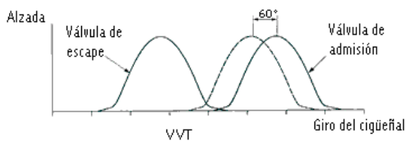
Fig. 7. Desplazamiento del cruce de válvulas del motor VVTI
