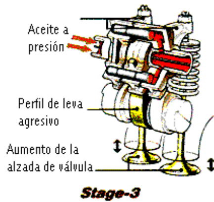
Fig. 13. i-VTEC. Estado 3
