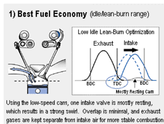
Fig. 9. i-VTEC. Estado 1
