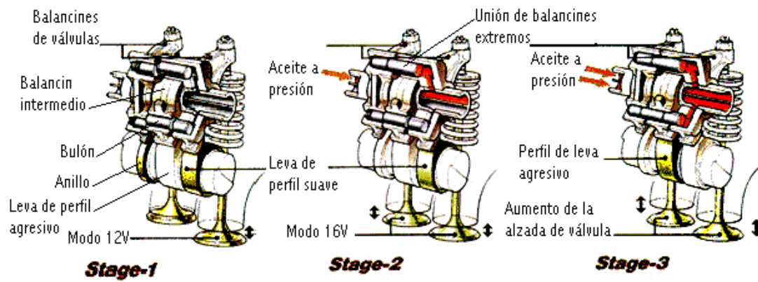
Fig. 15. i-VTEC. Estado 1,2, y 3
