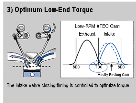
Fig. 12. i-VTEC. Estado 2
