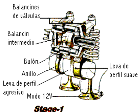
Fig. 8. i-VTEC. Estado 1
