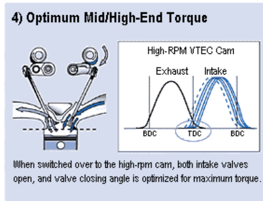
Fig. 14. i-VTEC. Estado 3
