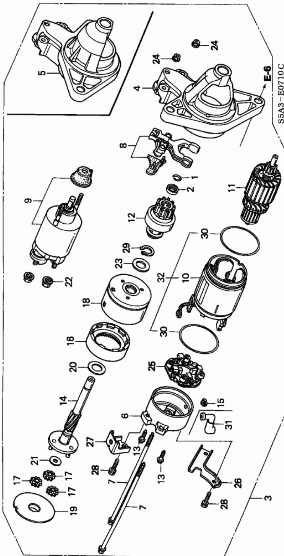
Figure 1: E-7-10 - STARTER MOTOR (DENSO)
