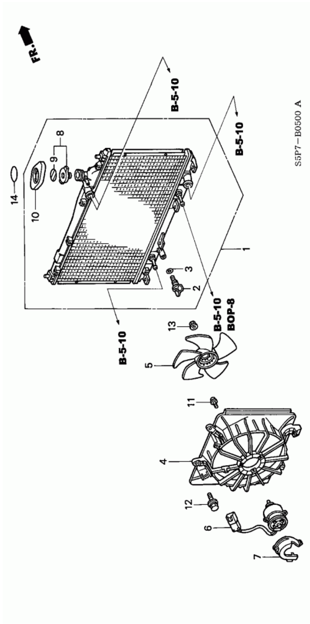
Figure 1: B-5 - RADIATOR (DENSO)
