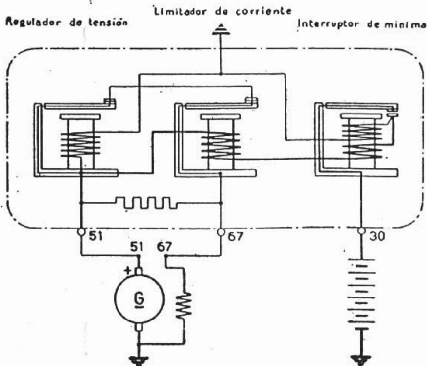
Esquema eléctrico del grupo de regulación.
