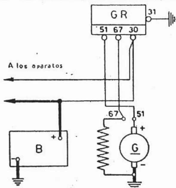
Esquema de las conexiones del grupo de regulación.
