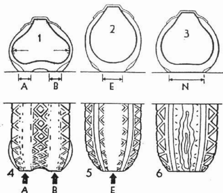
Desgaste irregular en las cubiertas.
