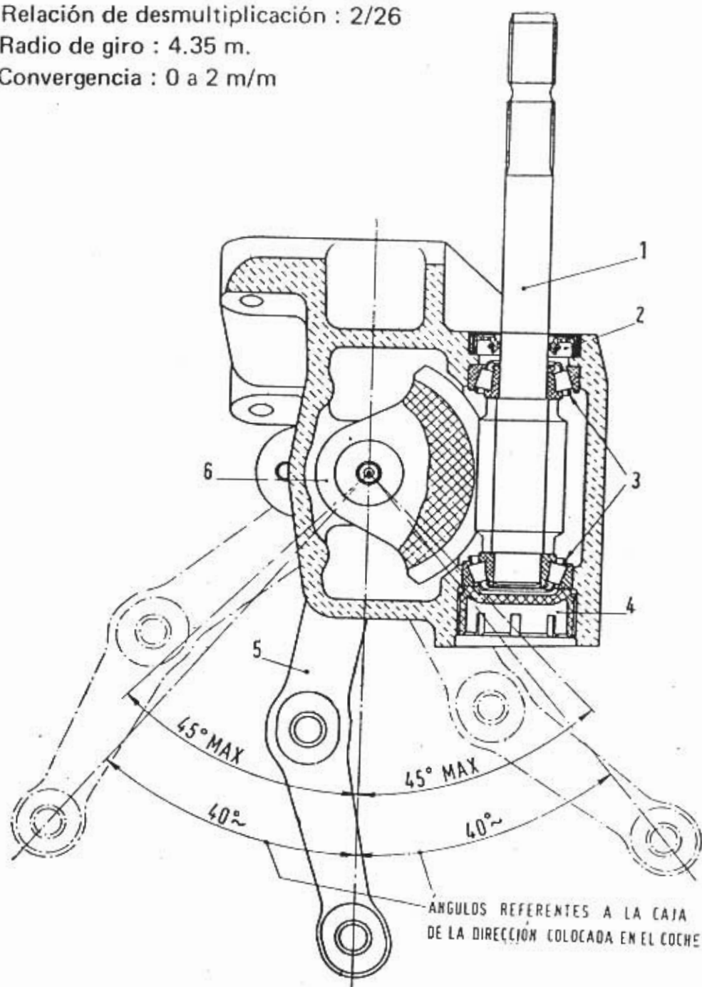
Sección de la caja de la dirección sobre el tornillo sinfín
