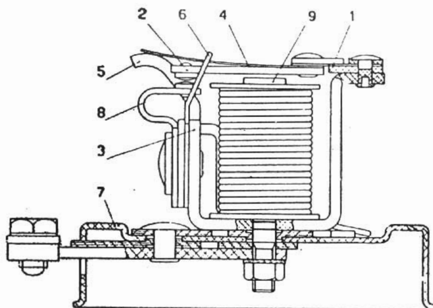
Interruptor de mínima del grupo de regulación.
