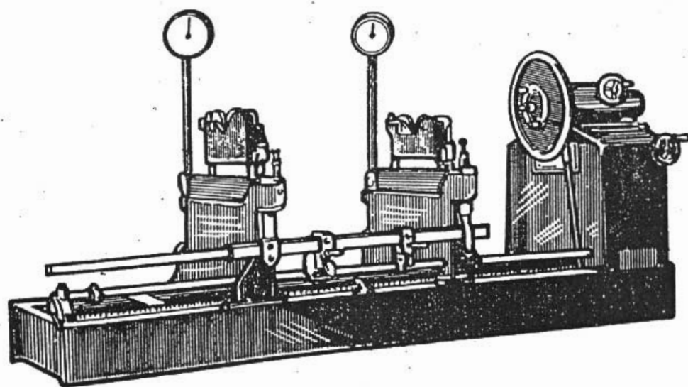
Máquina equilibradora del conjunto cigueñal, volante y embrague
