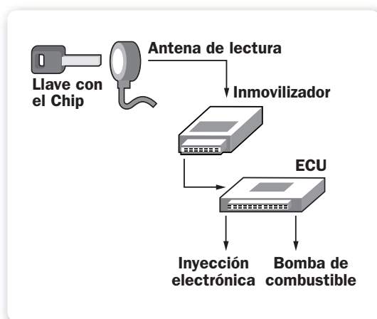
Figura 13. Bloques del sistema de comunicación de la llave con transponder.
