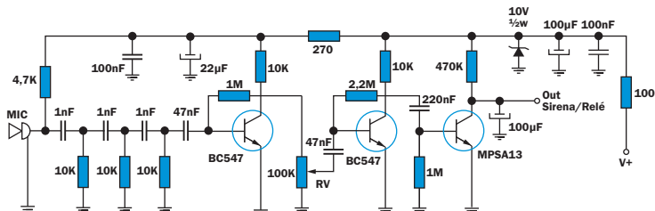
Figura 13. Para un mejor funcionamiento del circuito, debemos adherir el sensor (MIC) en la esquina superior del parabrisas o de la luneta.
