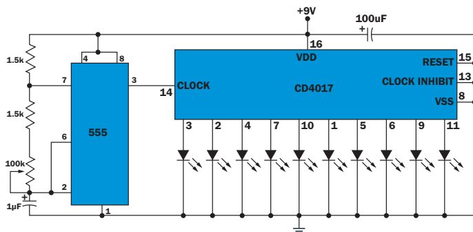
Figura 12. Podemos colocar este circuito en la parrilla delantera del vehículo o en la luneta, o montar varios circuitos formando un triángulo de baliza.
