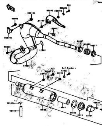
B-5 Muffler(s)
