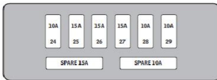
LOCALIZACIÓN: DETRÁS DE LA GUANTERA
