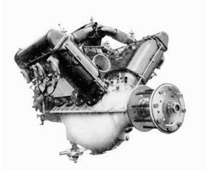
Moteur Hispano-Suiza type 8 F de 330 ch (Cliché catalogue constructeur, 1923).
