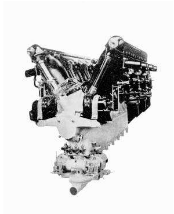
Moteur Hispano-Suiza type 12 M de 570 ch (1928). Catalogue constructeur.
