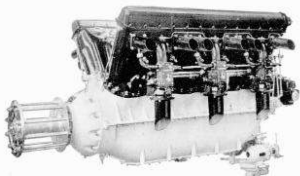
Moteur Hispano-Suiza type 12 Nb (1828). Catalogue constructeur.
