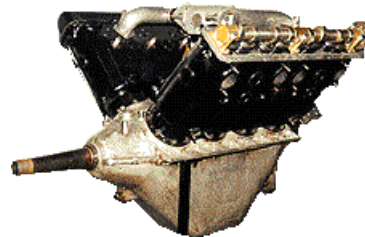
Hispano-Suiza 8A (1915).
