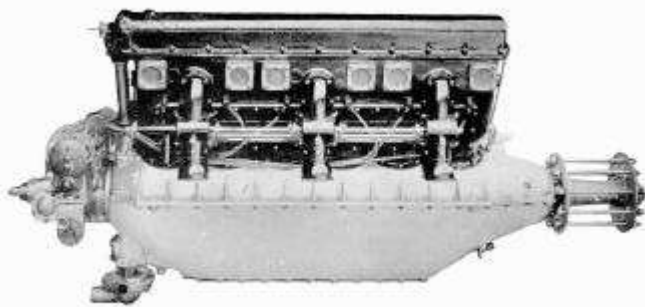
Moteur Hispano-Suiza type 12 Hbr en haut (réducteur ½) et 12 Hb de 500 ch (1925). (Catalogue constructeur).
