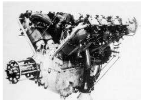
Le moteur Hispano-Suiza 8A de série en juin 1915 développe 150 ch.
