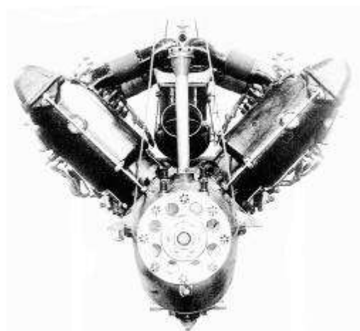
Moteur Hispano-Suiza 8Aa de 150 ch (1915).
