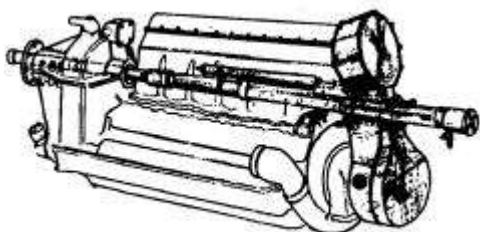
Moteur 12 Y avec canon Hispano de 20 mm.
