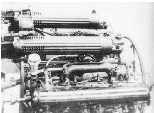
Moteur Hispano-Suiza du Sopwith Dolphin, montrant la disposition des deux mitrailleuses Vickers entre les deux rangées de cylindres. (Cliché Vickers).
