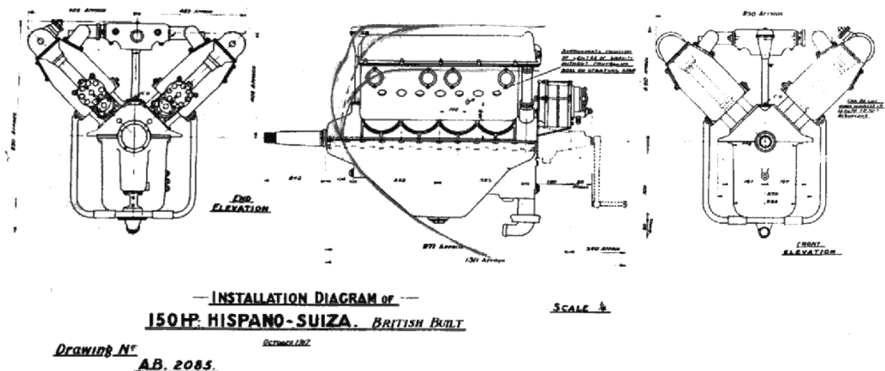
Plan trois vues du moteur Hispano-Suiza 8Aa de 150 ch (1915).
