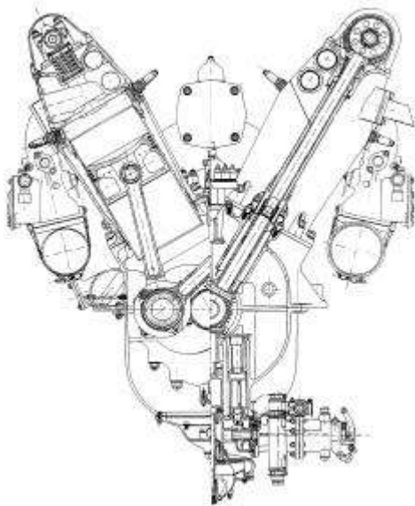
Moteur Hispano-Suiza 12 Xirs. (Cliché constructeur, 1933).
