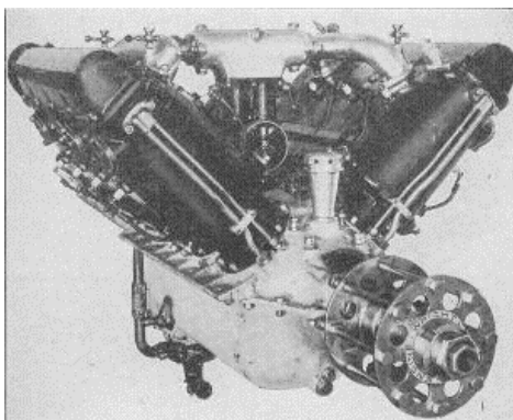
Moteur Hispano-Suiza 8Aa de 150 ch (1915).
