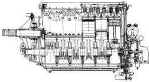
Moteur Klimov M-105 avec réducteur 2/3 et compresseur à deux étages. (Dessin OKB Klimov).
