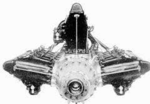
Moteur Hispano-Suiza type 18 Sbr, une mécanique destinée aux hydravions de compétition de la Coupe Schneider 1931. (Catalogue constructeur).
