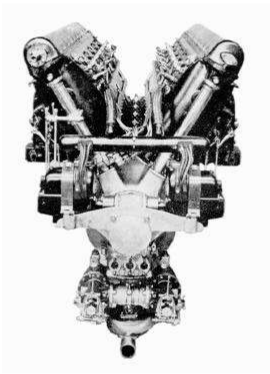
Moteur Hispano-Suiza type 12 Lbr de 600 ch (1928). Catalogue constructeur.
