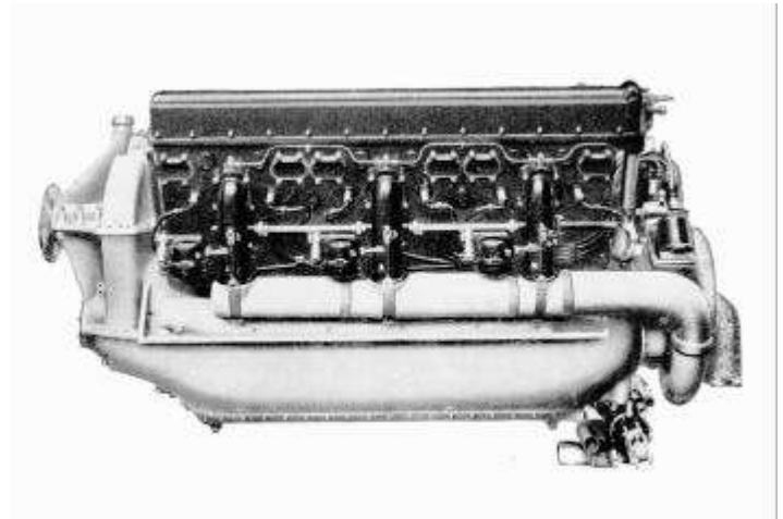
Moteur Hispano-Suiza suralimenté type 12 Ybrs de 800 ch (1932). Catalogue du constructeur.
