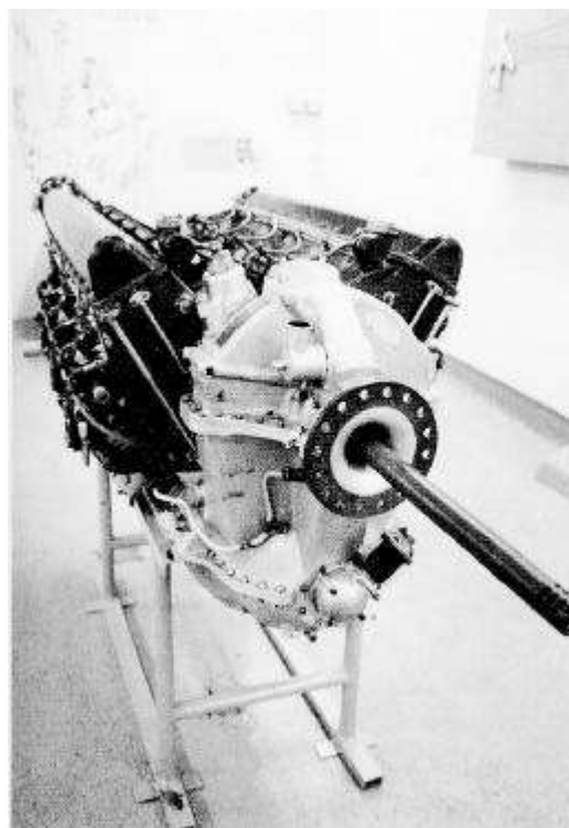
Moteur-canon Hispano-Suiza 12 Y-51 de 1050 ch. (Cliché Musée SNECMA).
