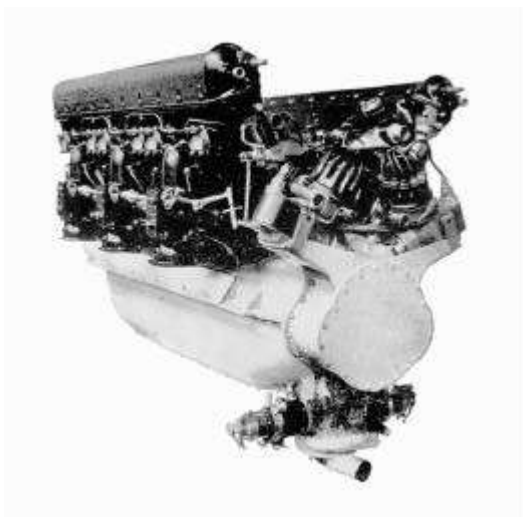
Moteur Hispano-Suiza suralimenté, type 12 Xbrs (1931). Catalogue du constructeur.
