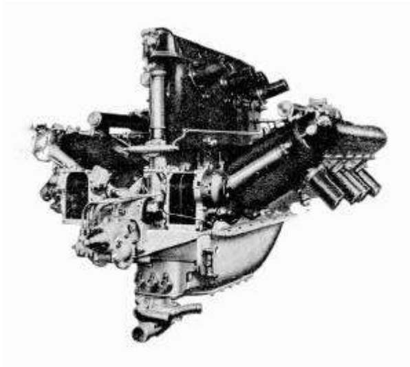
Moteur Hispano-Suiza type 12 Gb (1926). (Cliché catalogue constructeur 1932).
