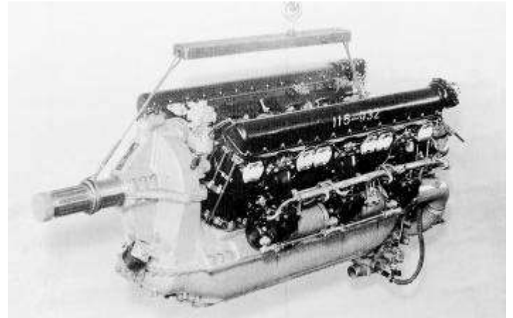
Moteur Klimov M-105 P de 1 100 ch.
