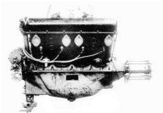
Moteur Hispano-Suiza 8Aa de 150 ch (1915).
