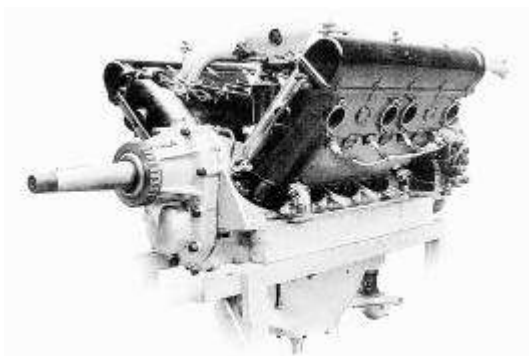
Moteur Hispano-Suiza 8Ba de 200 ch (1917).
