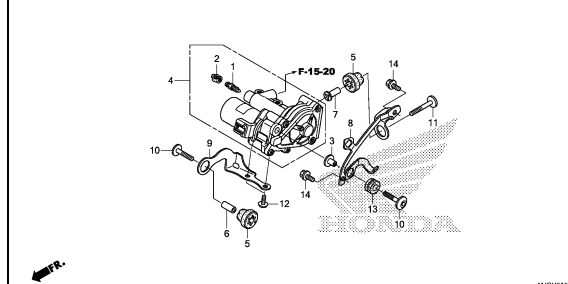
REAR POWER UNIT(CBR600RA)
