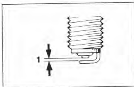
1. Holgura de la bujía
