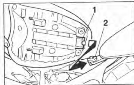
1. Salient 2. Soporte del asiento
