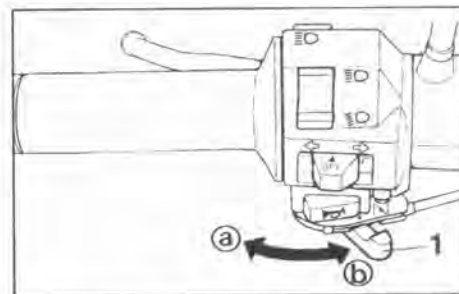
1. Palanca del estrangulador (choke) "a"
