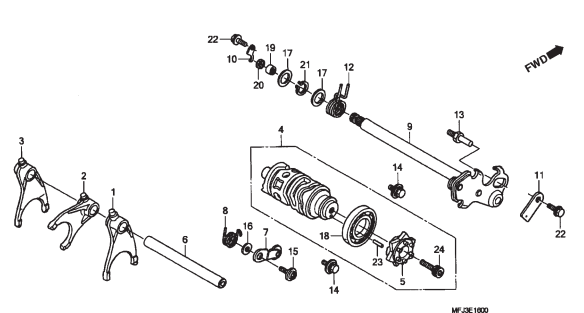
M-16 Tambor Seletor de Marchas
