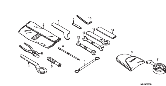
C-30 Ferramentas
