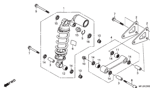
C-23 Amortecedor Traseiro
