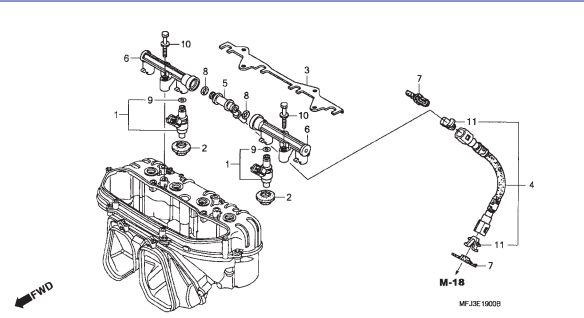
M-19 Injetor de Combustível
