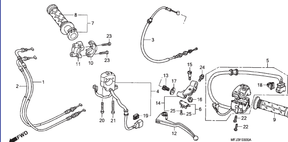
C-3 Alavanca do Guidão / Cabos / Interruptores
