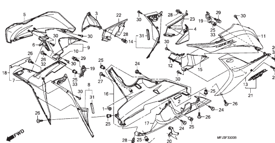
C-35-1 Emblema/Faixa (2)
