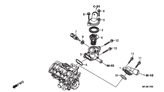
M-17 Termostato
