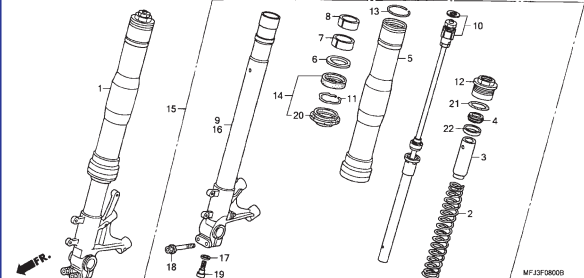
C-8 Garfo Dianteiro
