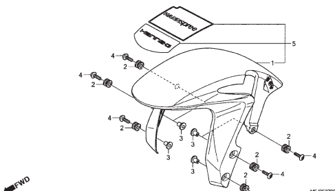
C-7 Pára-lama Dianteiro
