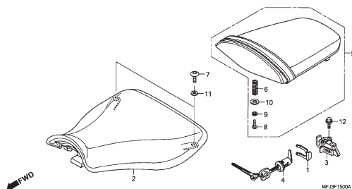
C-15 Assento
