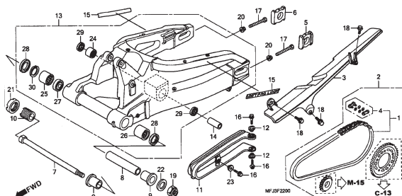
C-22 Garfo Traseiro
