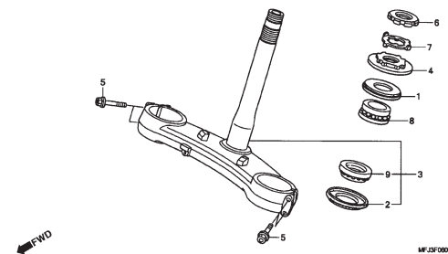
C-6 Coluna de Direção
