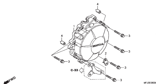
M-8 Tampa do Gerador
