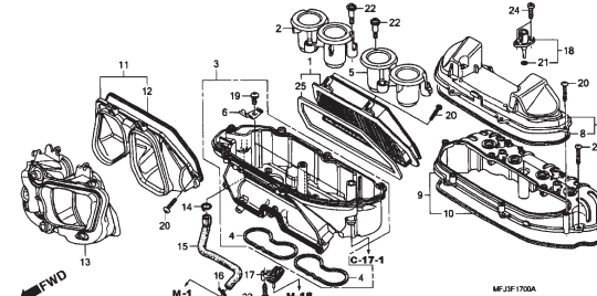
C-17 Filtro de Ar
