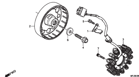
M-9 Gerador
