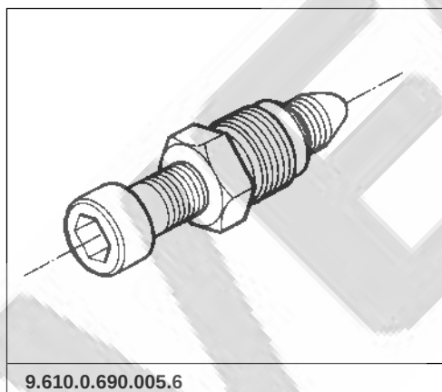
EXTRACTOR DEL PIÑÓN DE LA BOMBA DE INYECCIÓN CON AVANCE
