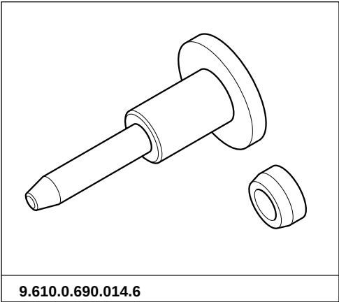
DISPOSITIVO PARA MONTAJE DE LAS GUÍAS DE LAS VÁLVULAS
