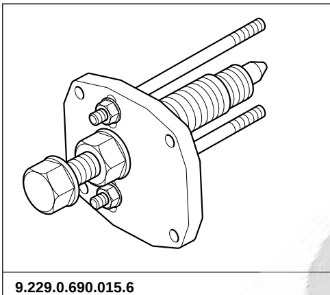
EXTRACTOR DEL PIÑÓN DE LA BOMBA DE INYECCIÓN
