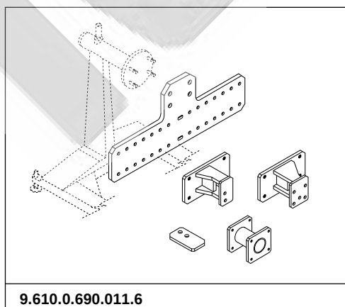
ADAPTADOR PARA EL SOPORTE DEL MOTOR
