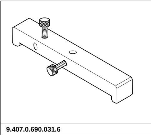
DISPOSITIVO PARA MEDICIÓN DE LA POSICIÓN DEL PISTÓN Y ALTURA DE LA CAMISA
