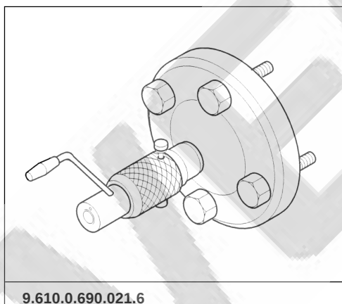
DISPOSITIVO PARA ASENTAMIENTO DE LA CAMISA
