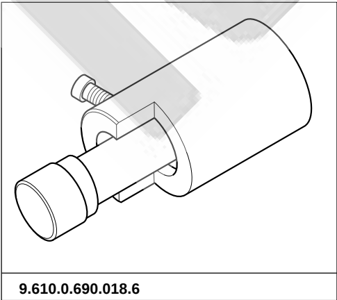
DISPOSITIVO PARA DESMONTAJE Y MONTAJE DEL BUJE DE LA BIELA
