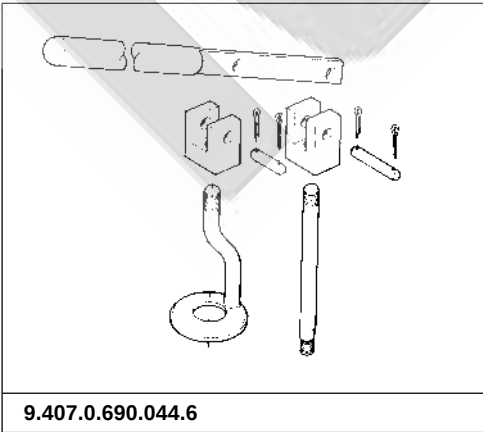
DISPOSITIVO PARA DESMONTAJE Y MONTAJE DE LOS RESORTES DE LAS VÁLVULAS EM LAS CULATAS
