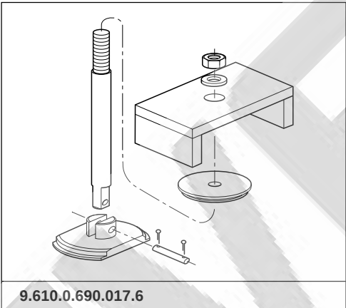
DISPOSITIVO PARA DESMONTAJE DE LA CAMISA DEL CILINDRO
