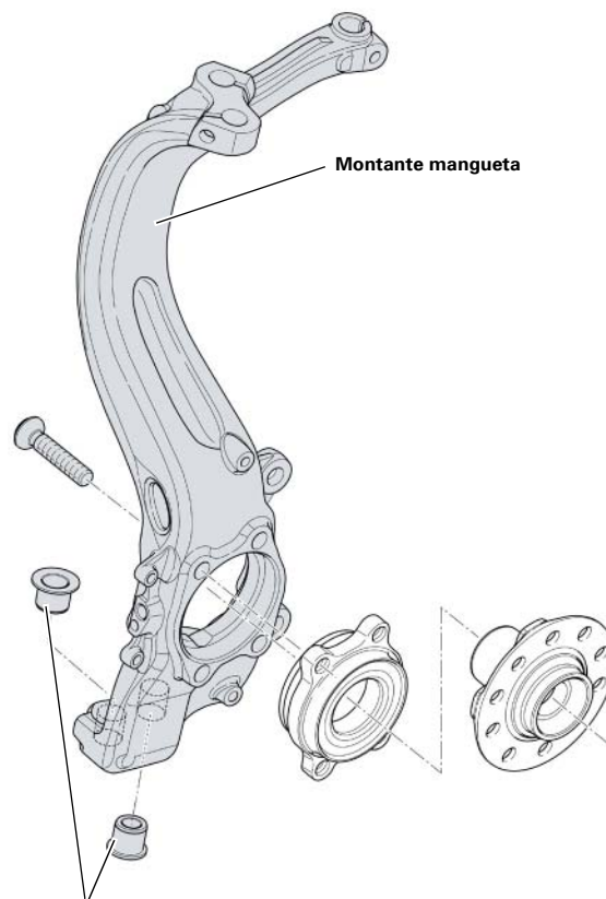
Casquillos para alojamiento de los brazos oscilantes
