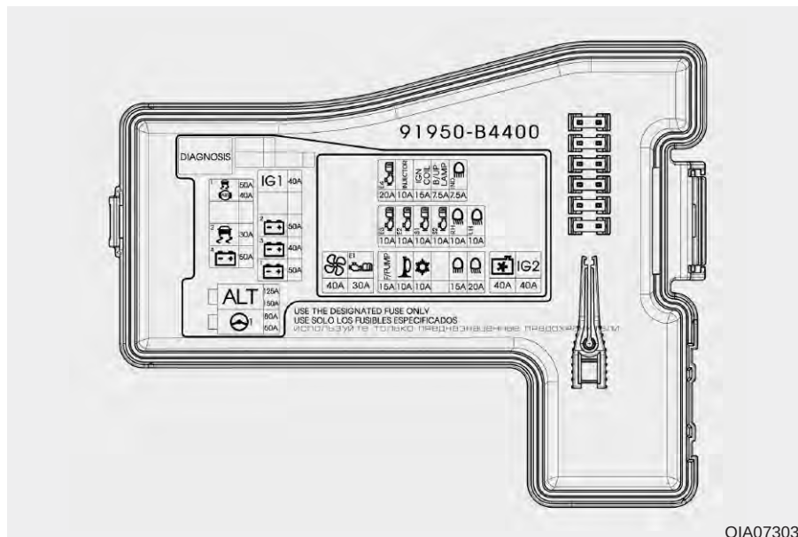
Panel de fusibles del compartimento del motor
