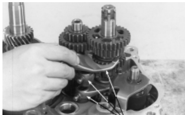
HORQUILLAS SELECTORAS
