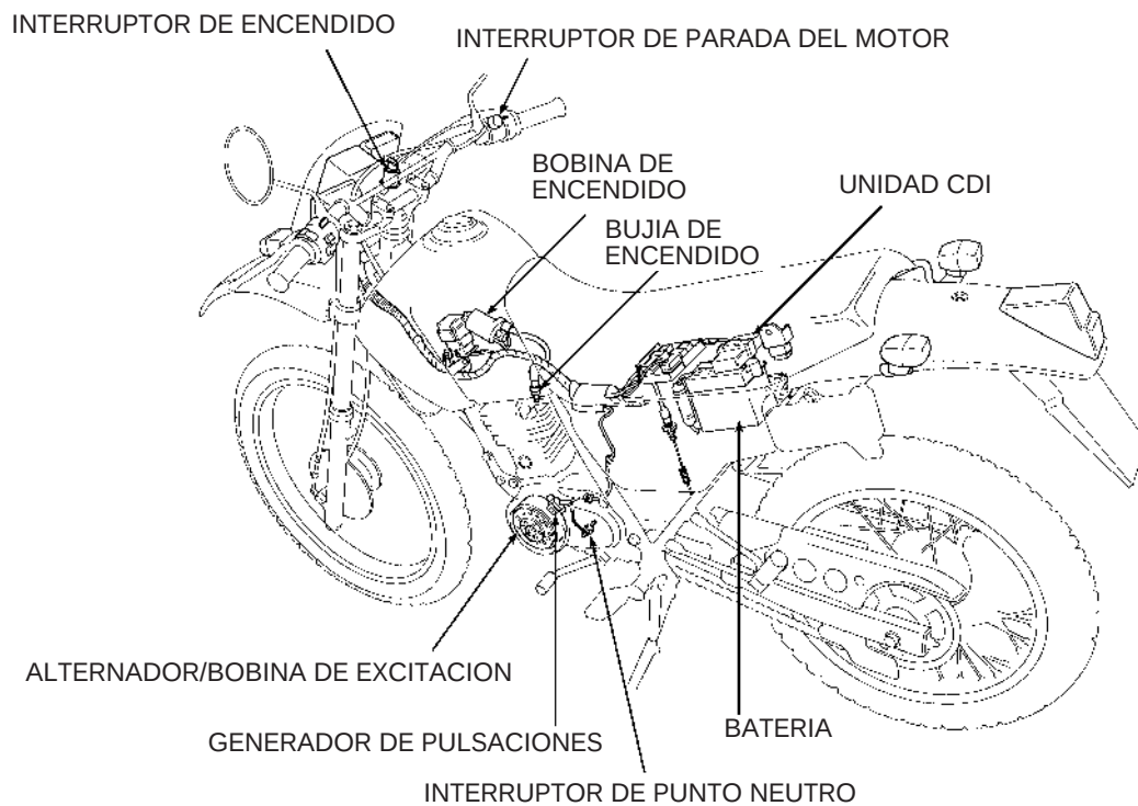
DIAGRAMA ELECTRICO:
