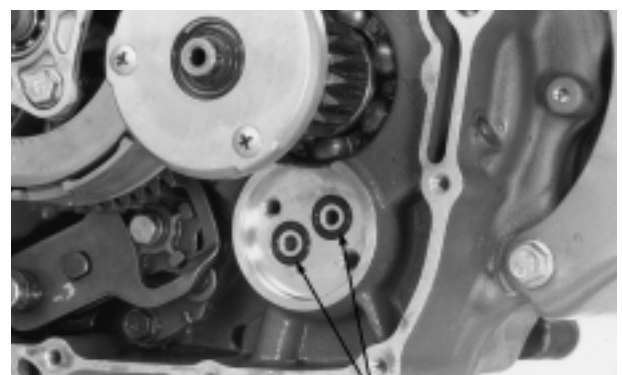
ANILLOS SELLADORES
