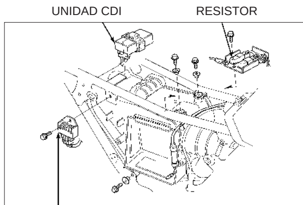
REGULADOR/RECTIFICADOR
