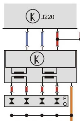
Circuito eléctrico
