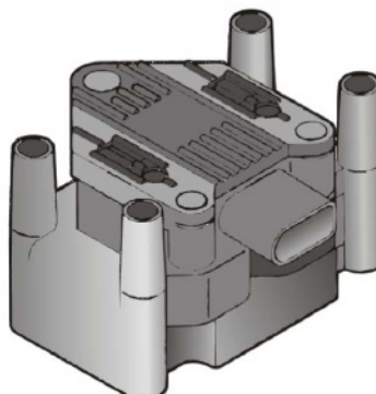
Transformador de encendido N152
