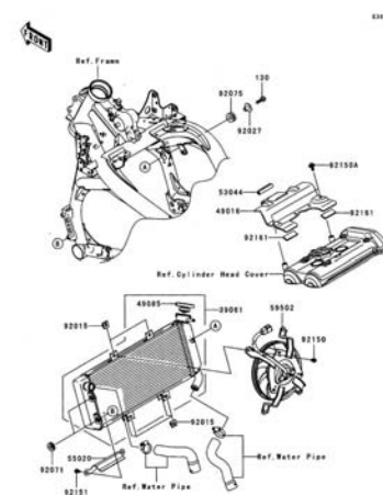
D-5 Radiador
