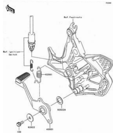
F-3 Brake Pedal
