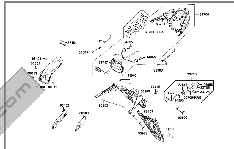
F18 GBARROS/PILOTO TRASERO (Pág. 115)
