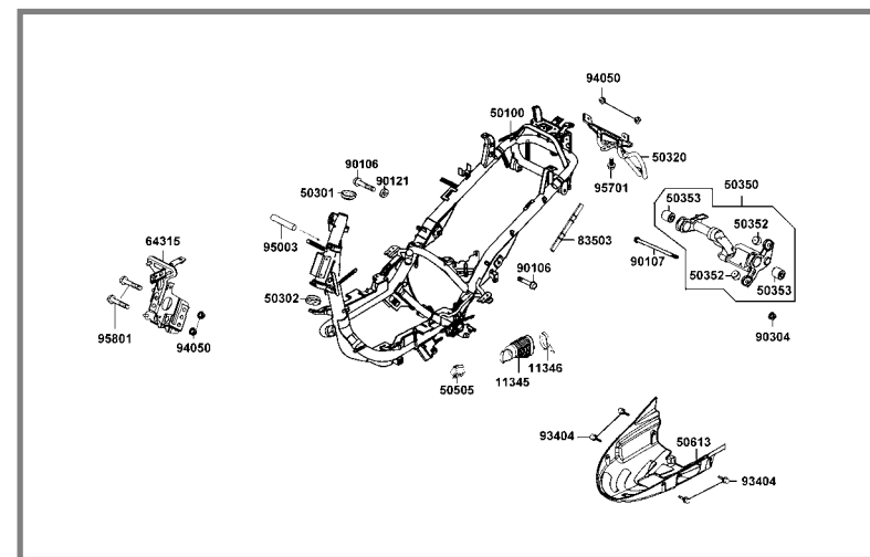
F20 CHASIS (Pág. 124)
