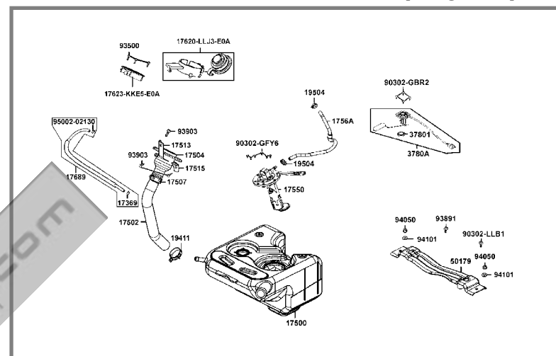
F10 DEPOSITO DE GASOLINA (Pág. 91)
