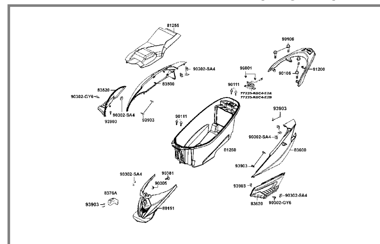
F12 CARROCERIA TRASERA (Pág. 97)
