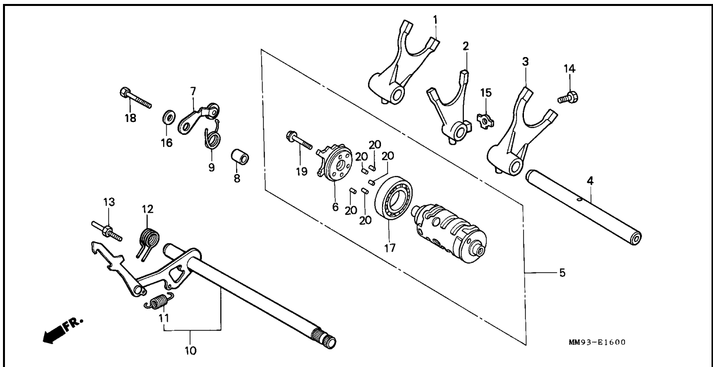
Bloque E-16 TAMBOR CAMBIO ENGRANAJES
