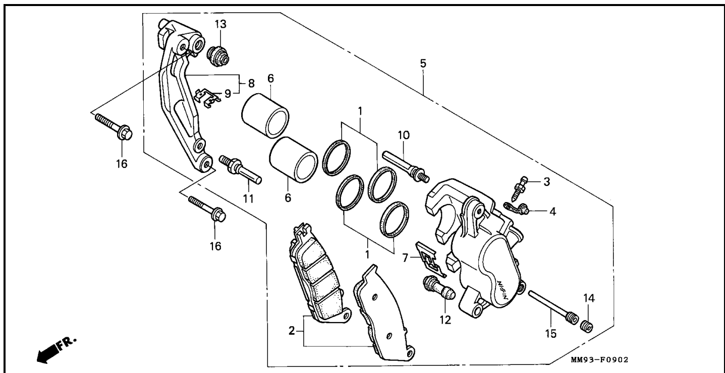
Bloque F-9-2 CALIBRE DE FRENO (XL600VR)
