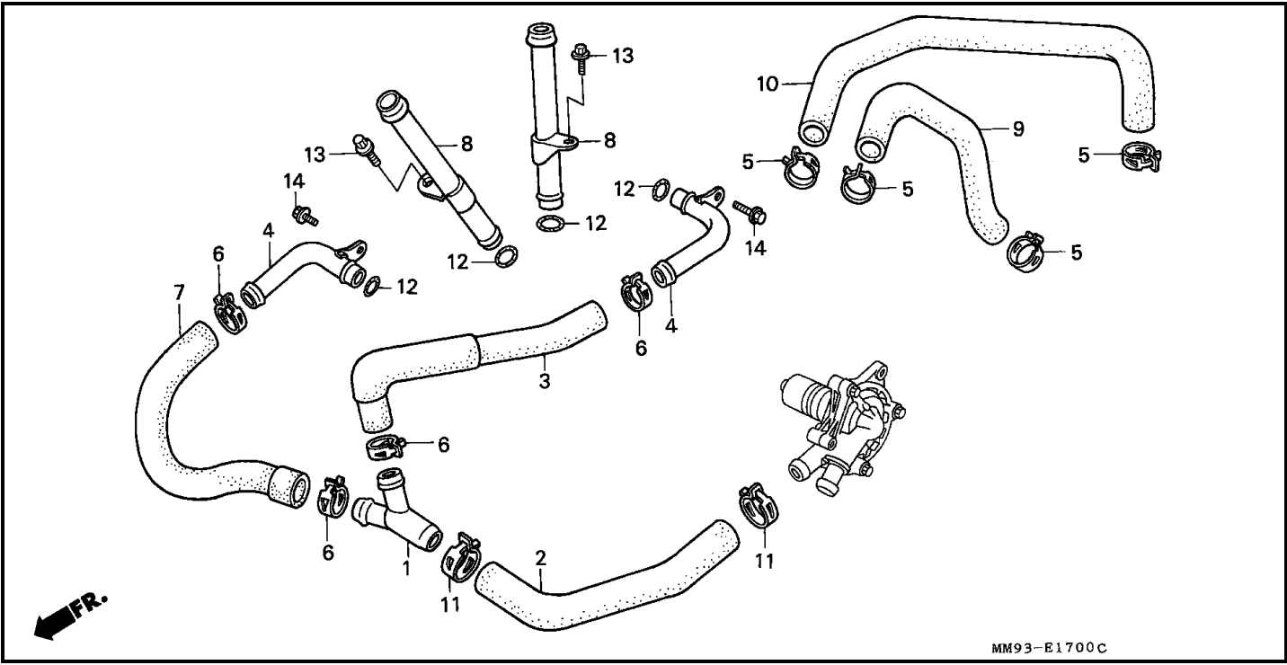
Bloque E-17 TUBERIA DE AGUA
