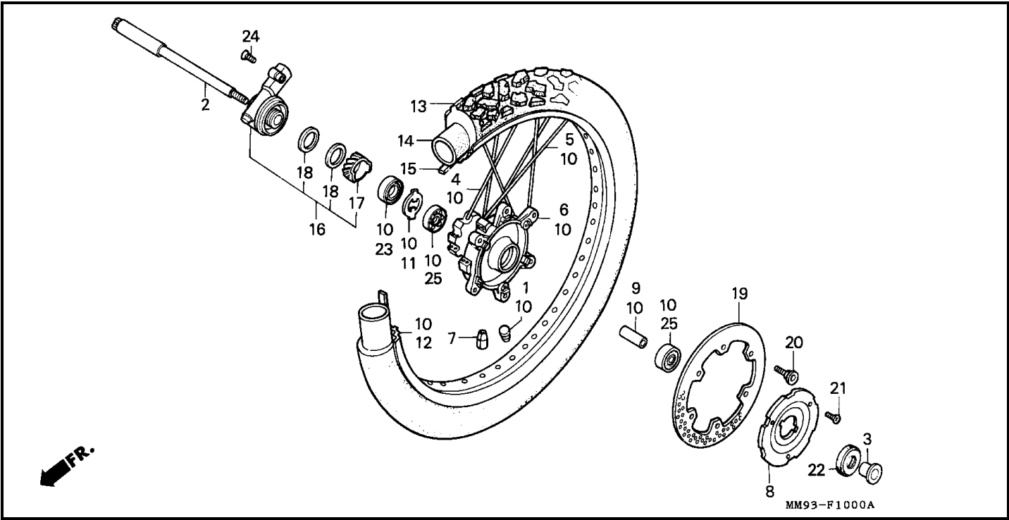
Bloque F-10 RUEDA DELANTERA
