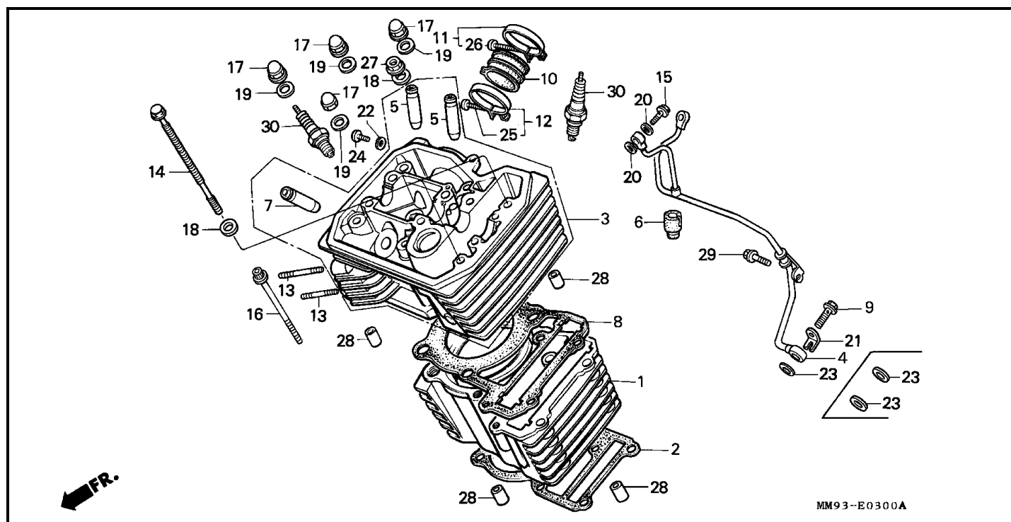
Bloque E-3 CILINDRO/CULATA DE CILINDRO (DELANTERO)
