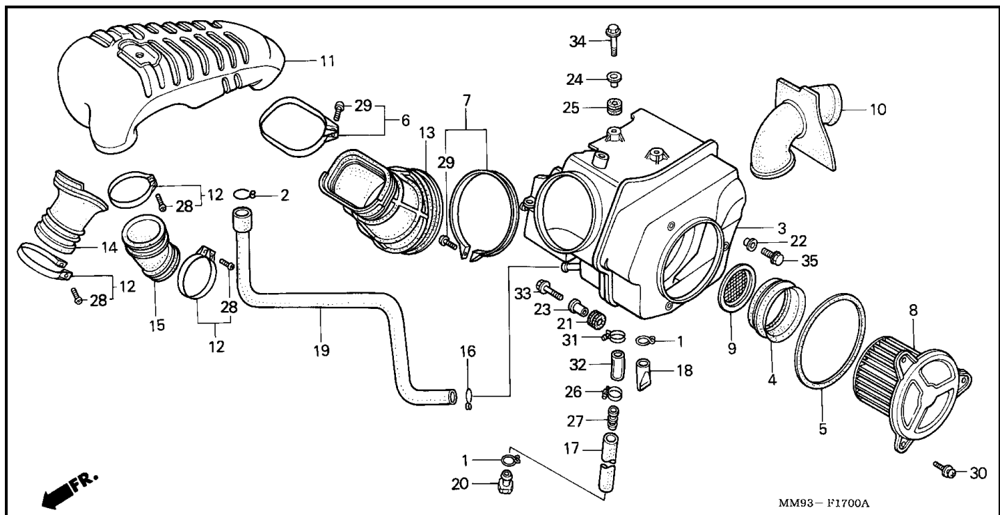
Bloque F-17 LIMPIADOR DE AIRE(1)
