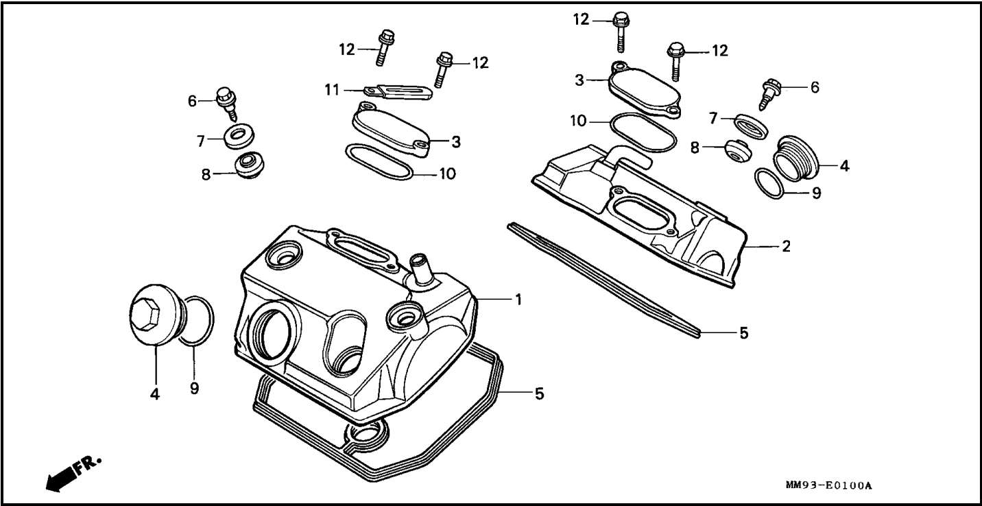
Bloque E-1 CUBIERTA CULATA CILINDRO
