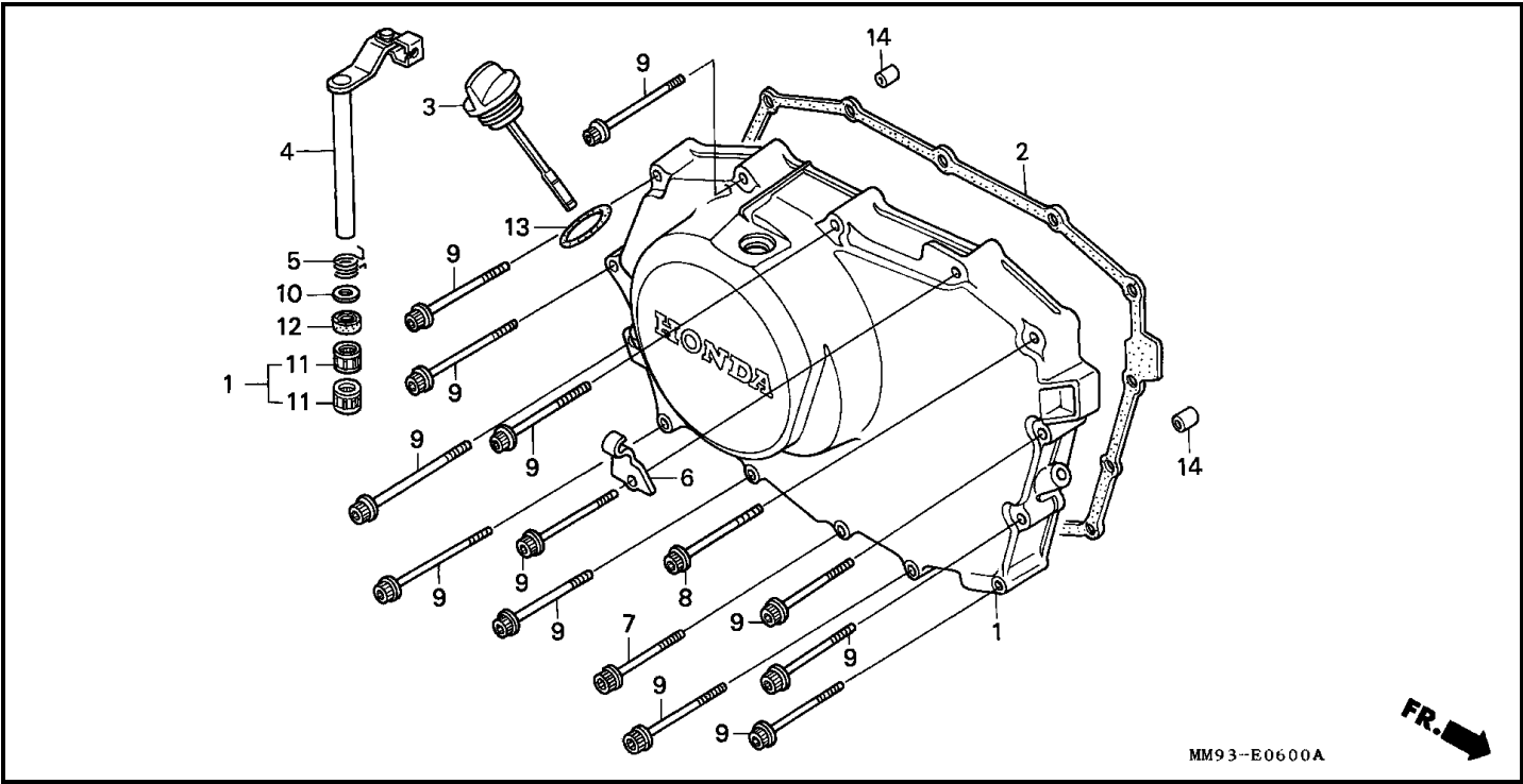
Bloque E-6 CUBIERTA DE CARTER DER.
