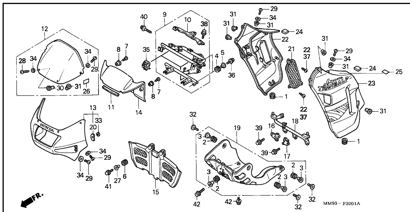
Bloque F-30-1 CAPO(2) (XL600VR)
