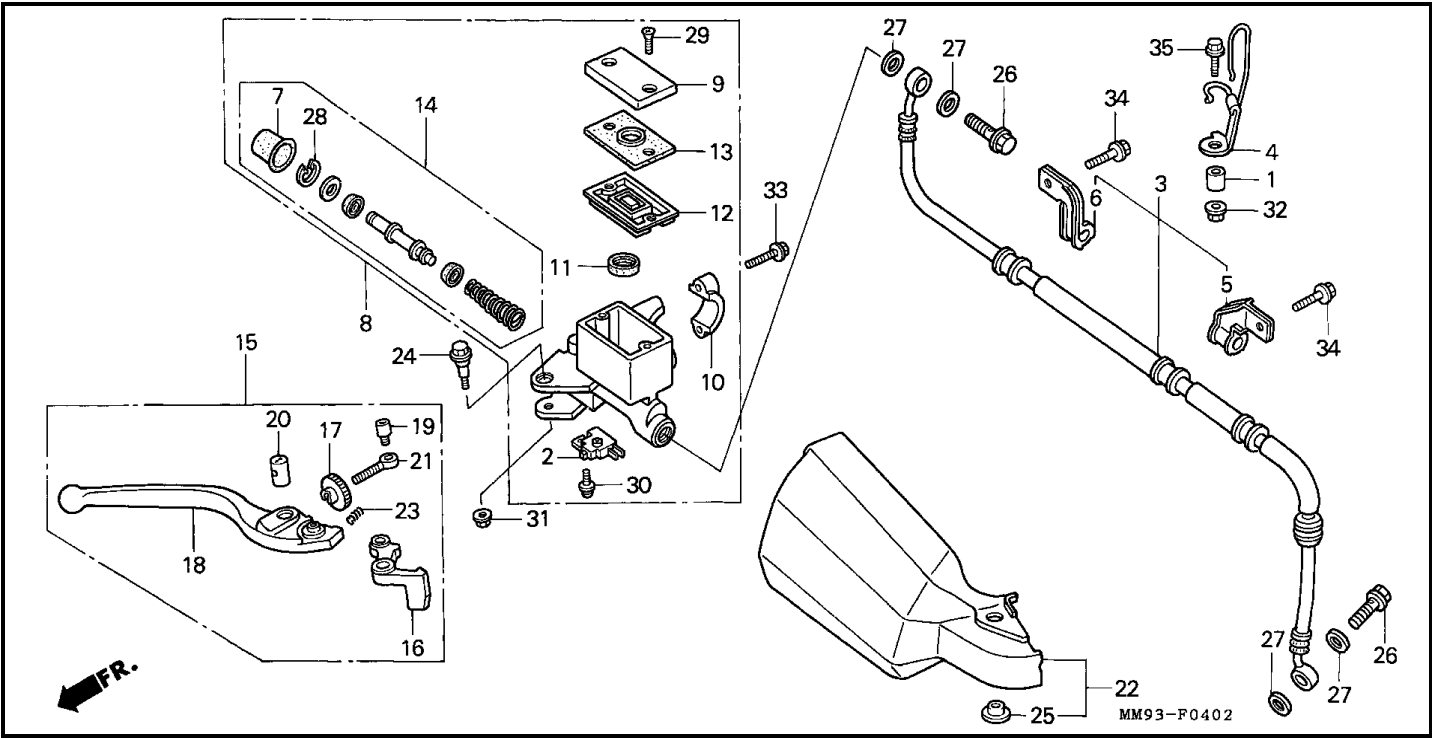
Bloque F-4-2 CILINDRO MAESTRO DE FRENO(XL600VR)
