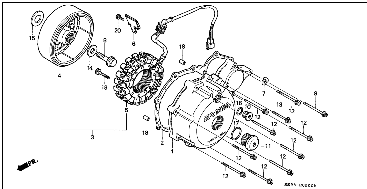
Bloque E-9 CUBIERTA DE CARTER IZQ./ GENERADOR
