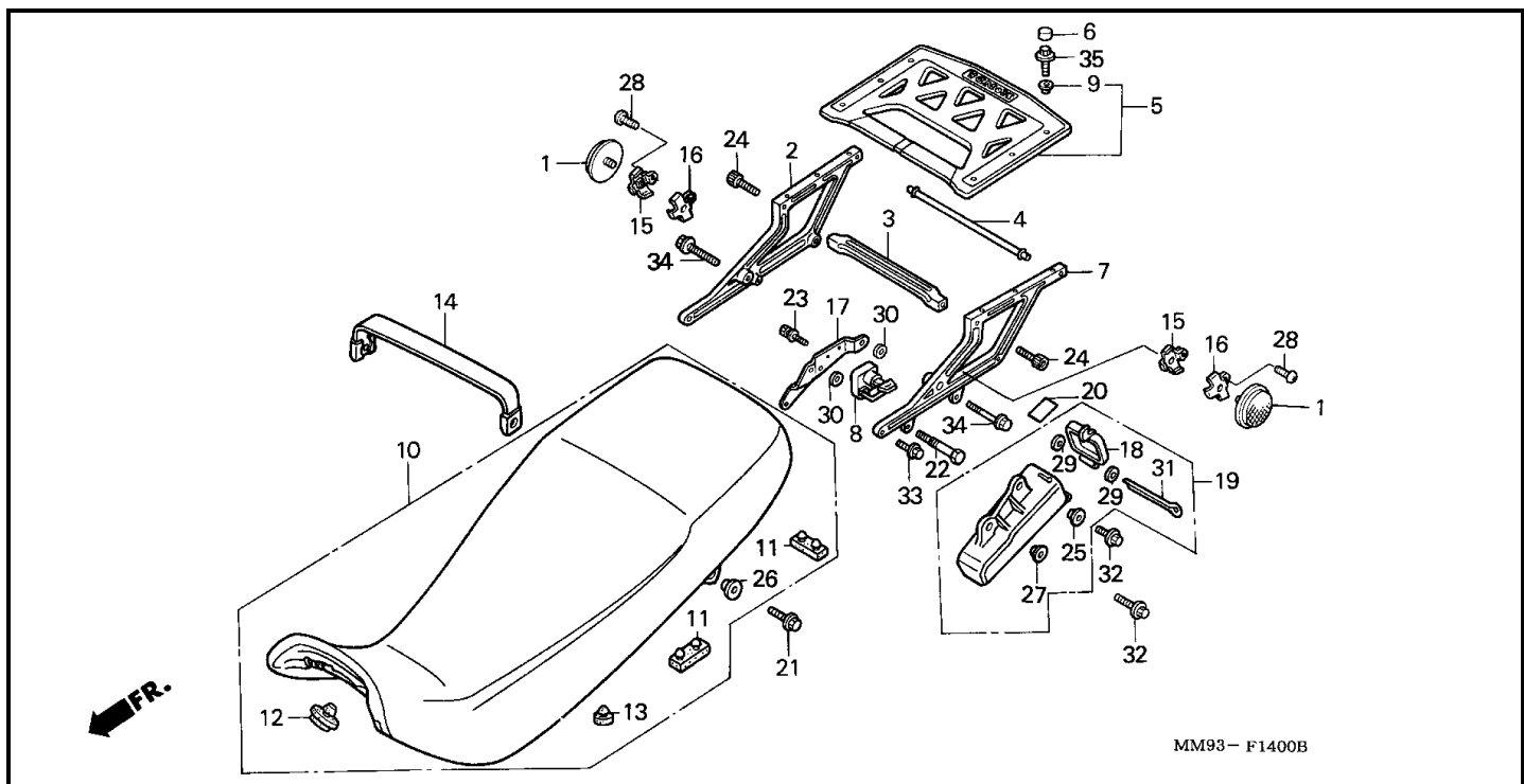
Bloque F-14 ASIENTO
