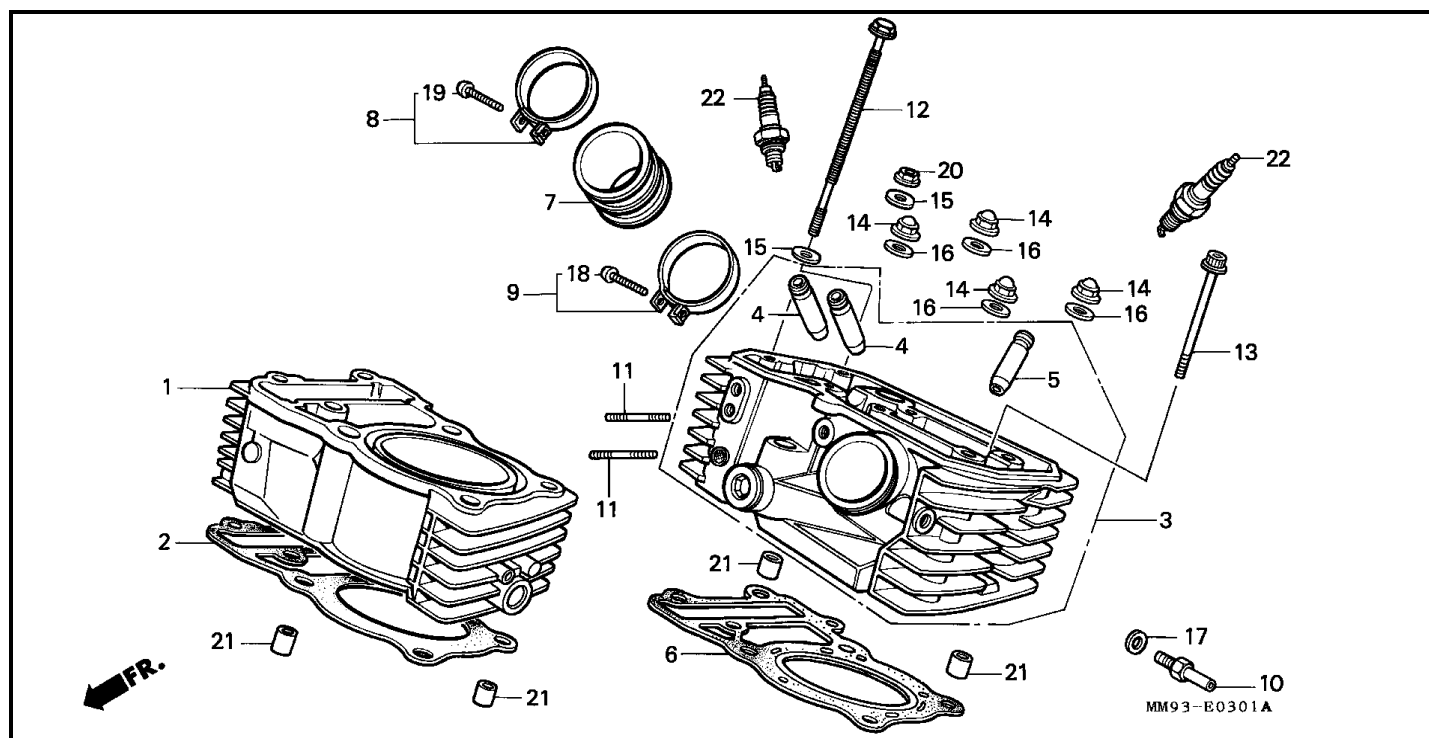
Bloque E-3-1 CILINDRO/CULATA DE CILINDRO (TRASERO)
