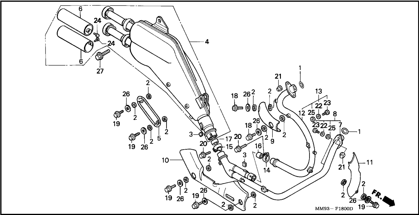
Bloque F-18 SILENCIADOR DE ESCAPE
