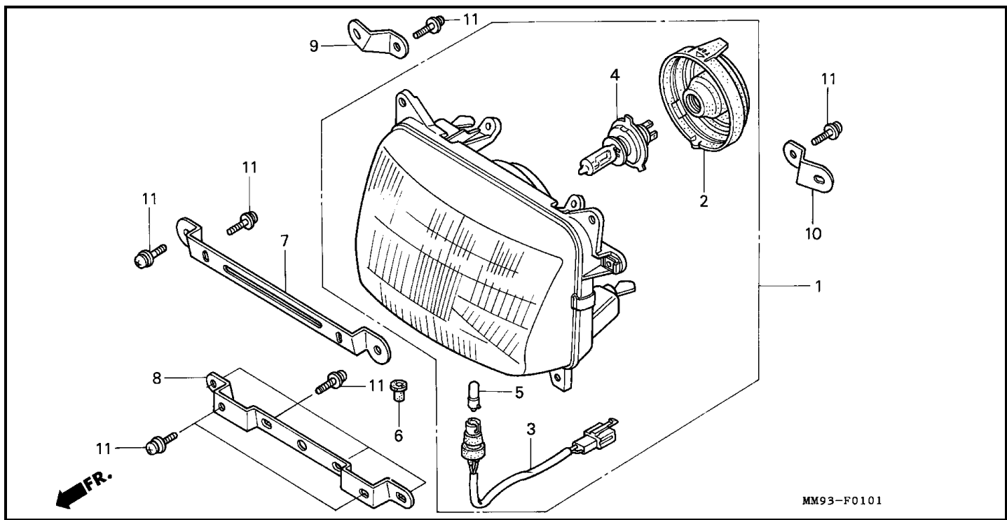
Bloque F-1-1 FARO DELANTERO(2) (XL600VR)
