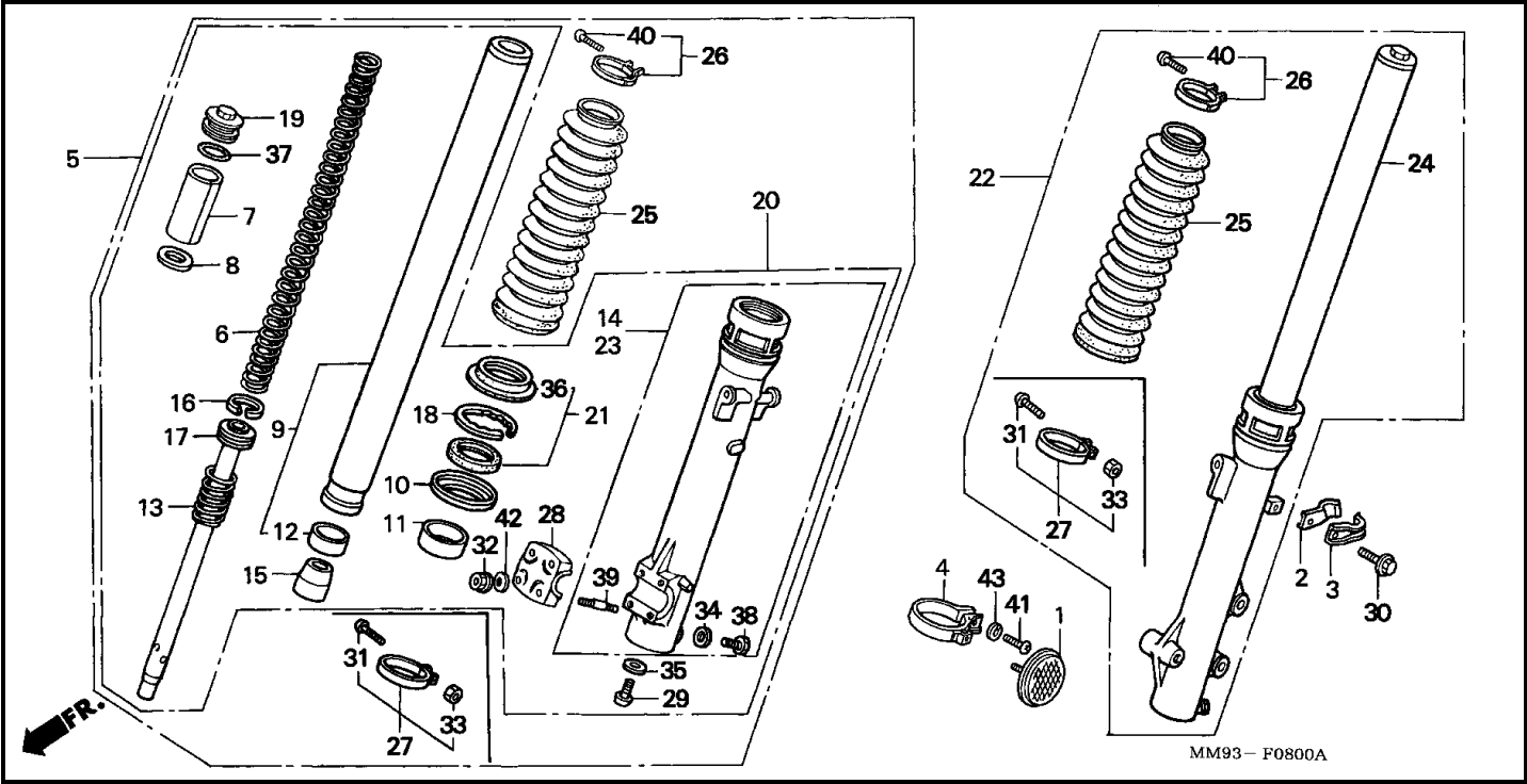
Bloque F-8 HORQUILLA DELANTERA
