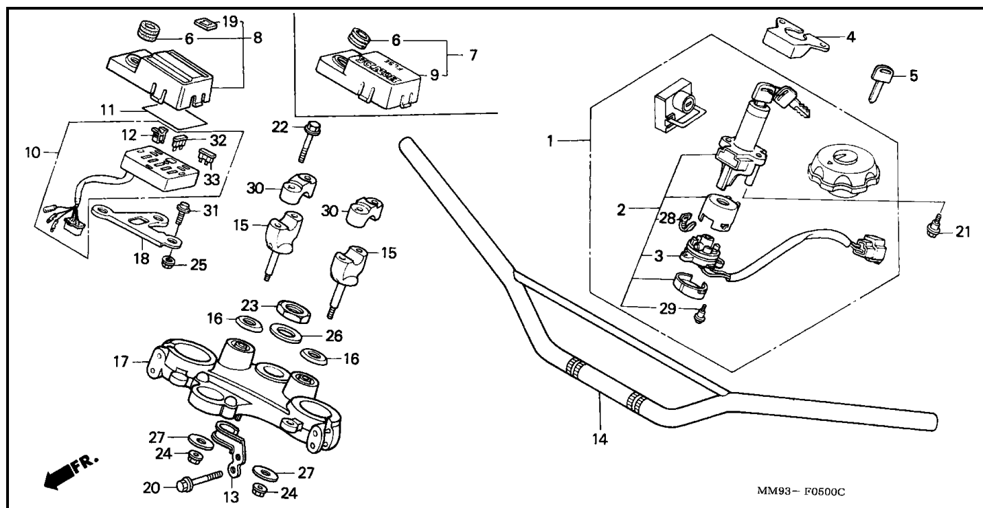
Bloque F-5 TUBERIA DE MANIJA/PUENTE SUPERIOR
