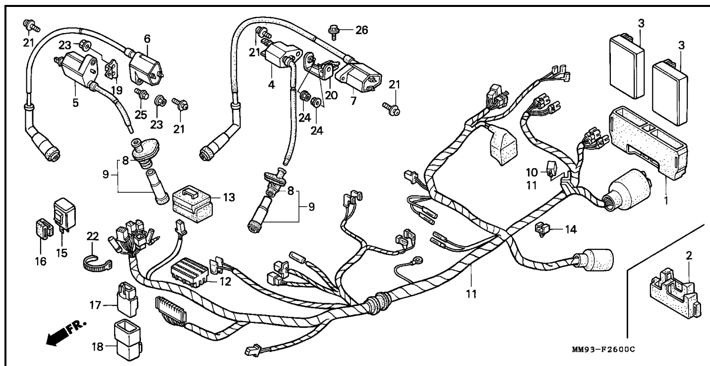
Bloque F-26 CONJUNTO DE ALAMBRES/ BOBINA DE ENCENDIDO
