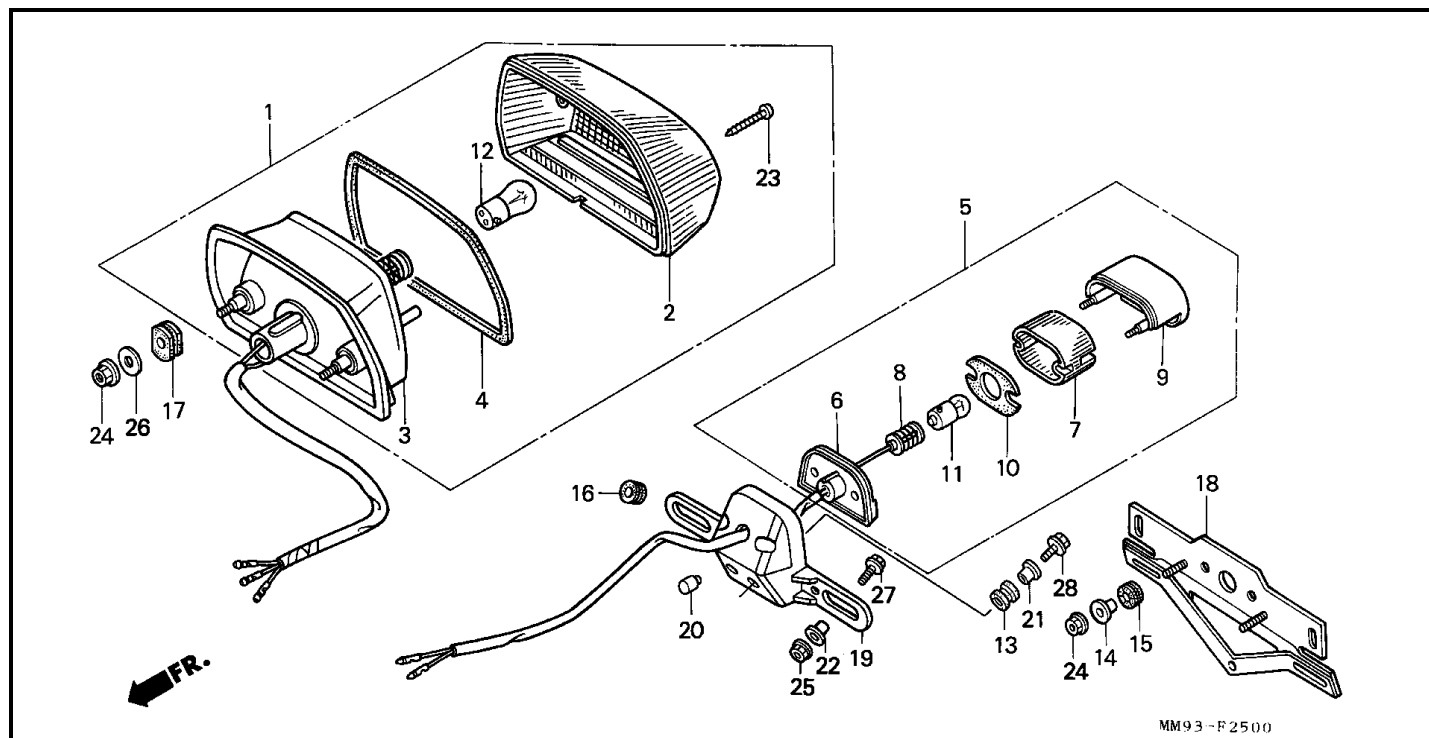
Bloque F-25 LUZ TRASERA
