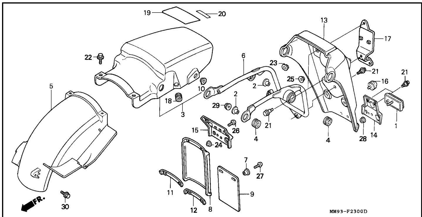
Bloque F-23 GUARDABARROS TRASERO
