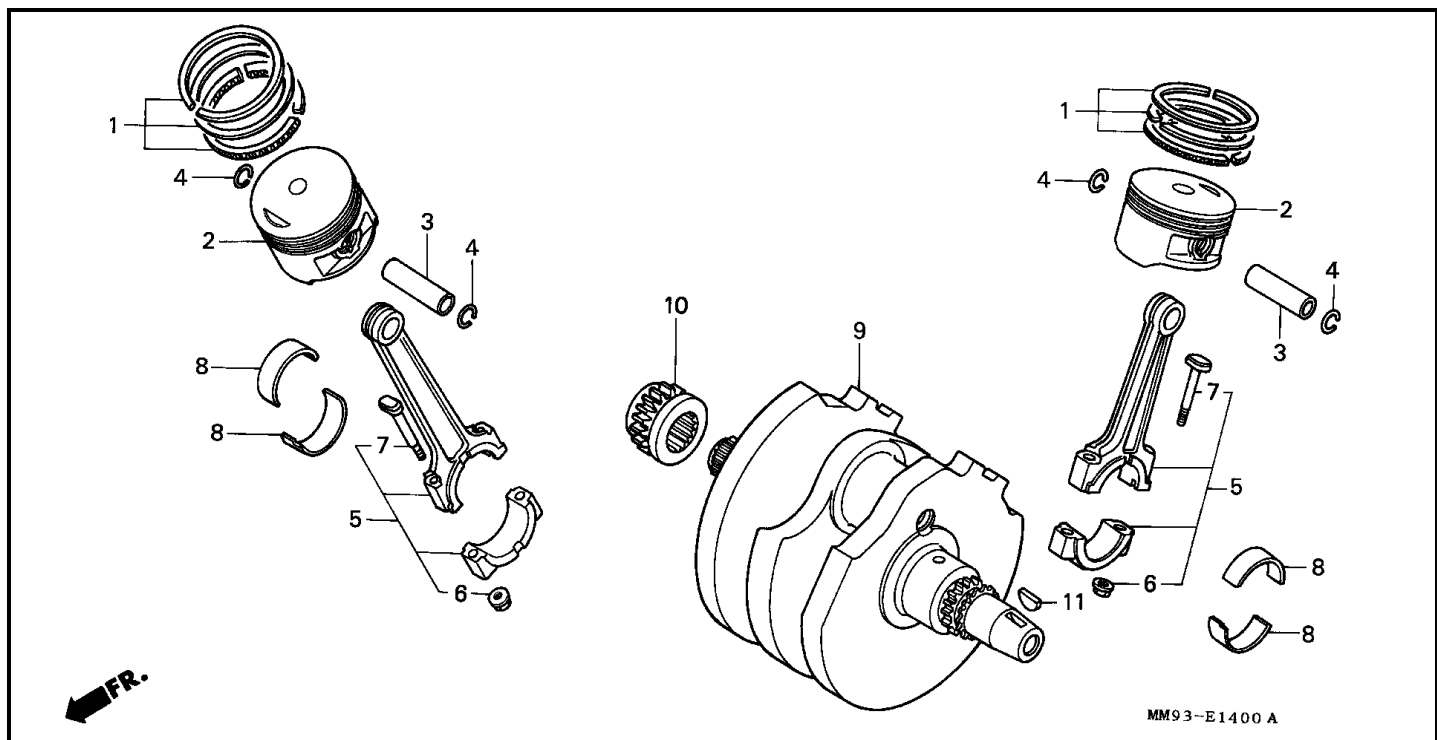
Bloque E-14 CIGUENAL/PISTON
