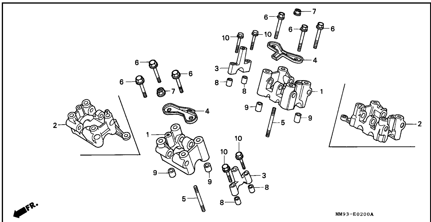
Bloque E-2 PORTADOR DE EJE DE LEVA
