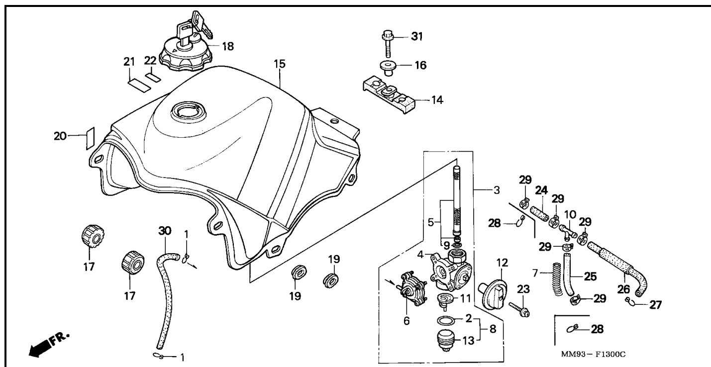
Bloque F-13 TANQUE DE COMBUSTIBLE
