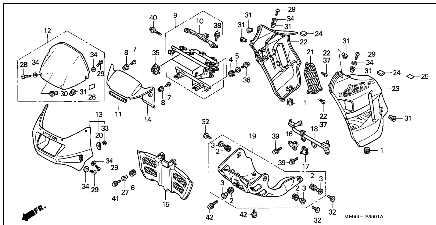
Bloque F-30-1 CAPO(2) (XL600VR)
