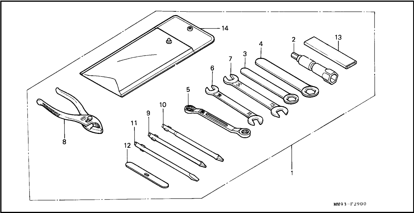
Bloque F-29 HERRAMIENTAS
