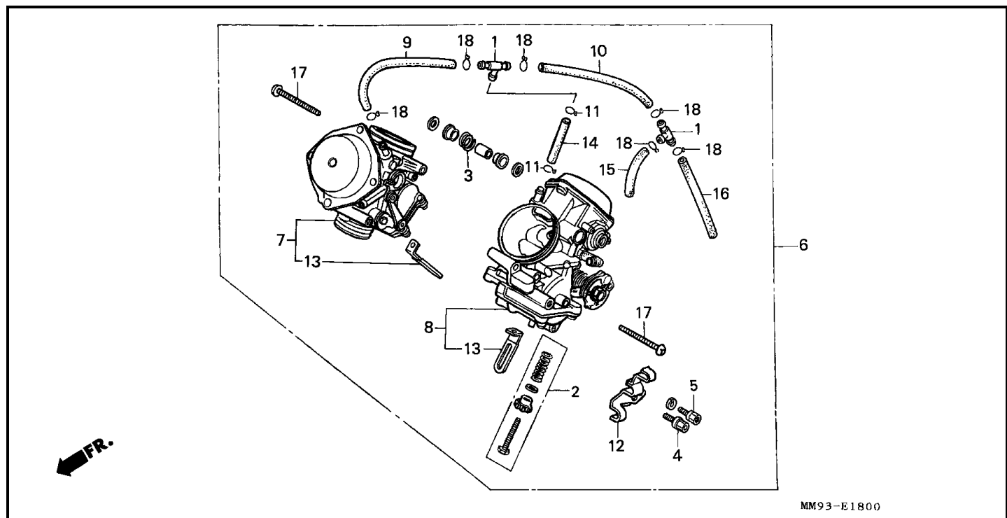
Bloque E-18 CARBURADOR(ENS.)
