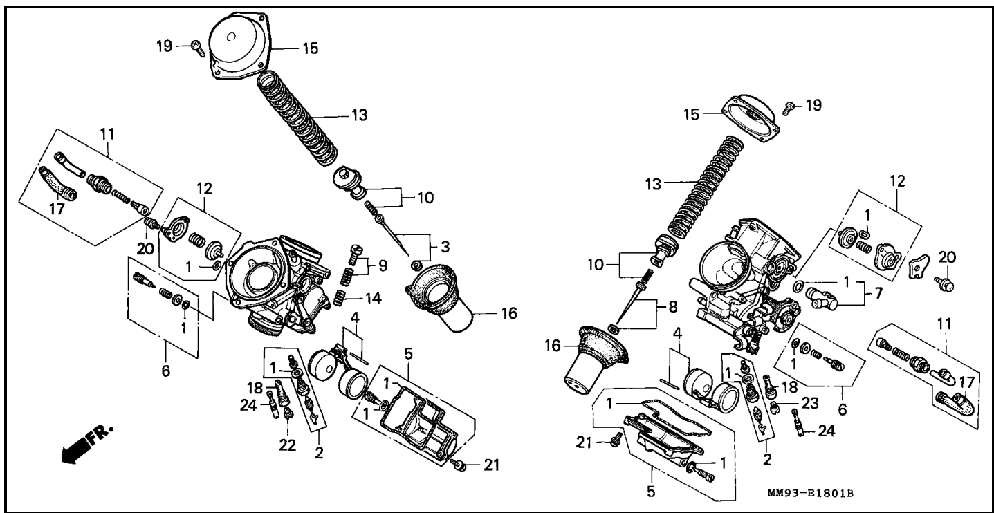
Bloque E-18-1 CARBURADOR (PARTES COMPONENTES)
