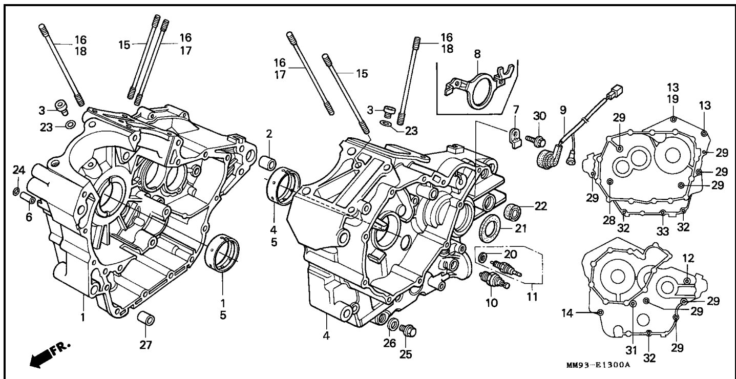
Bloque E-13 CARTER DE MOTOR
