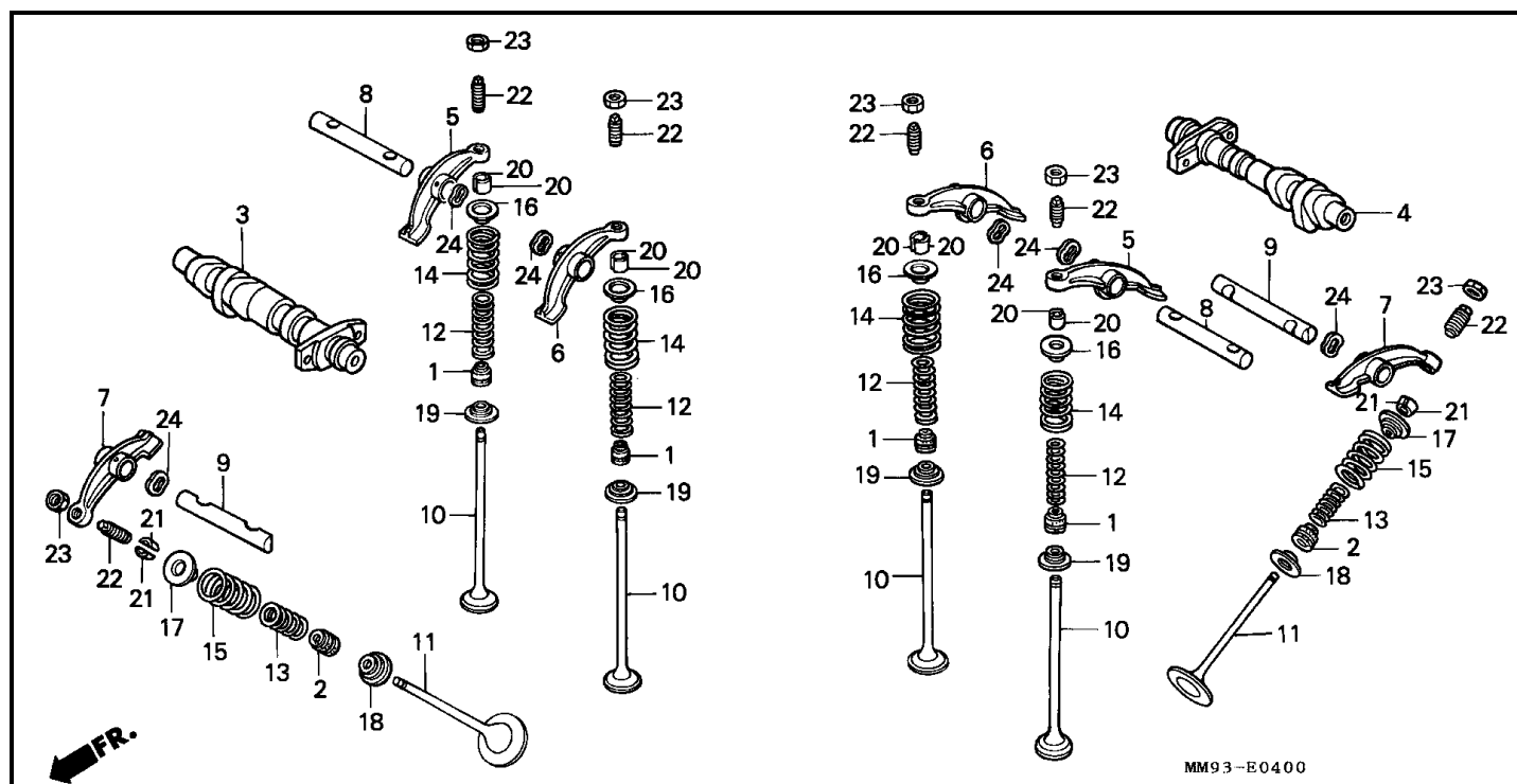
Bloque E-4 ARBOL DE LEVAS/VALVULA
