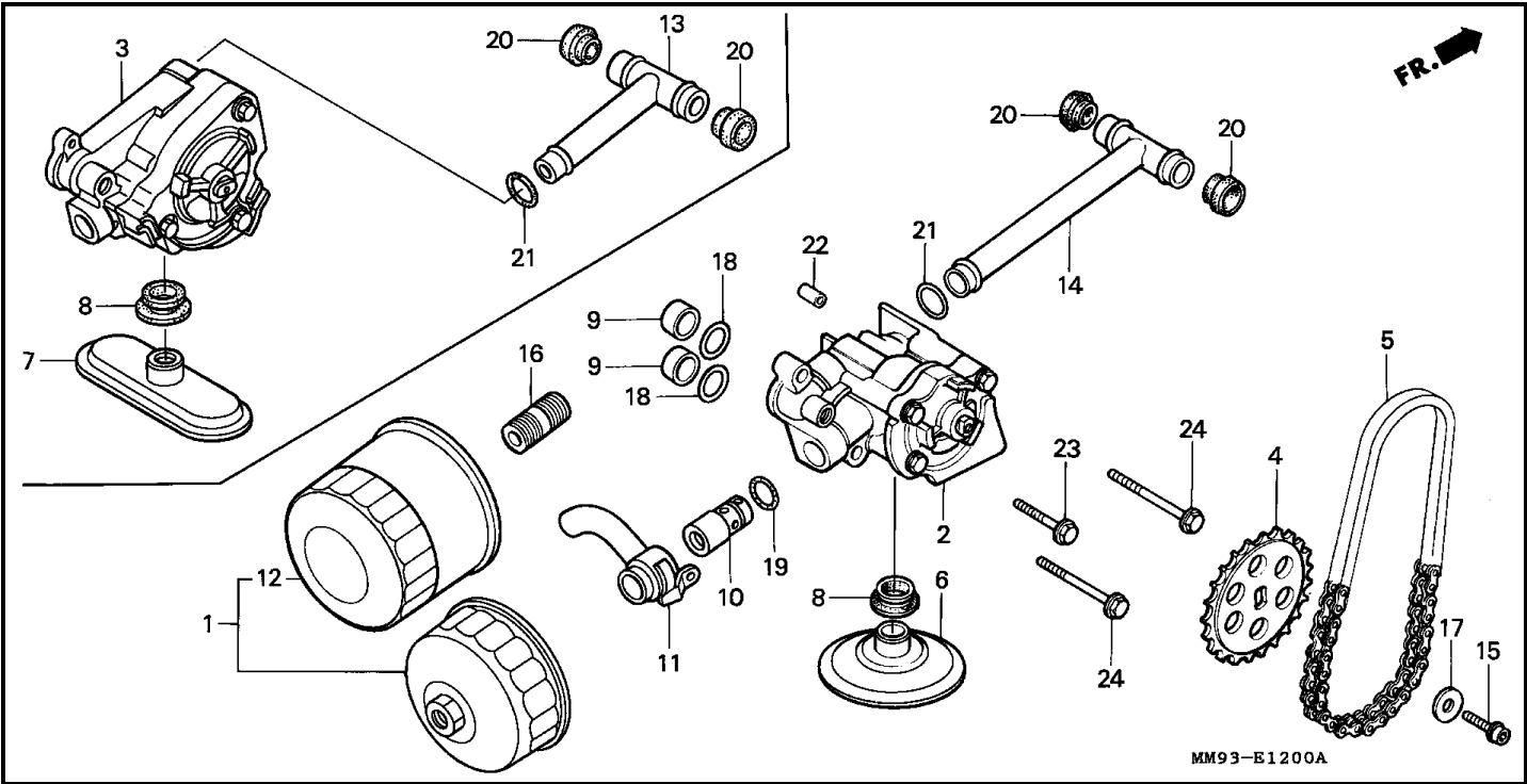
Bloque E-12 FILTRO DE ACEITE/BOMBA DE ACEITE
