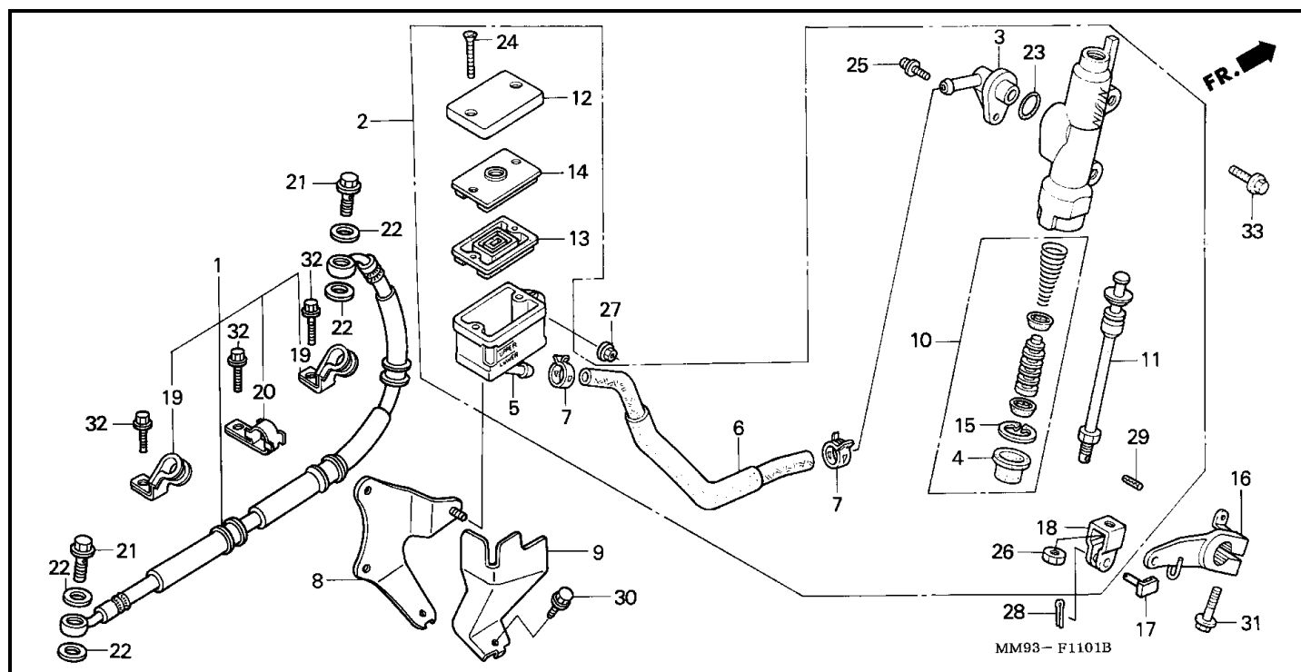
Bloque F-11-1 CILINDRO MAESTRO DE FRENO(XL600VM/VN/VP/VR)
