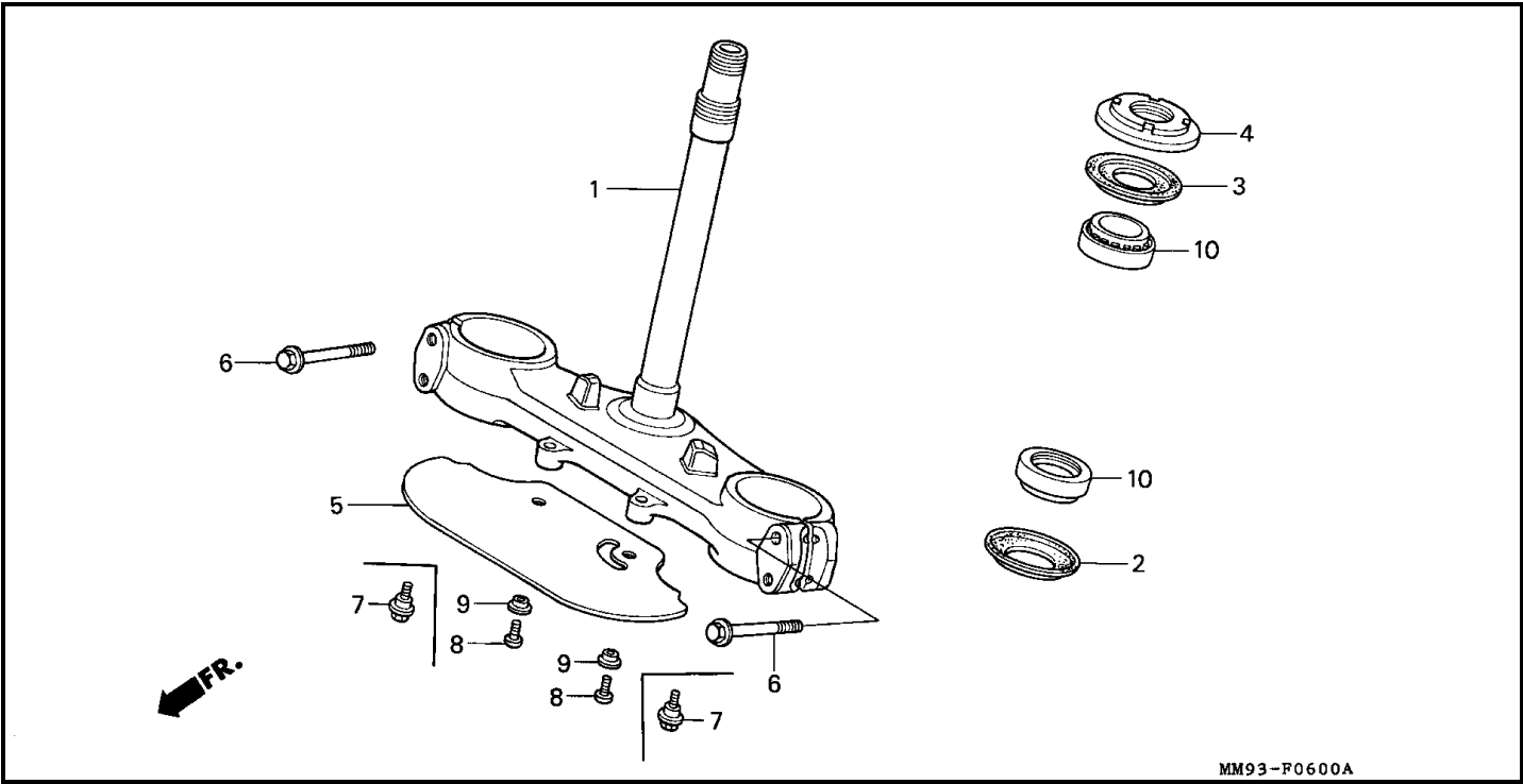
Bloque F-6 VASTAGO DE DIRECCION
