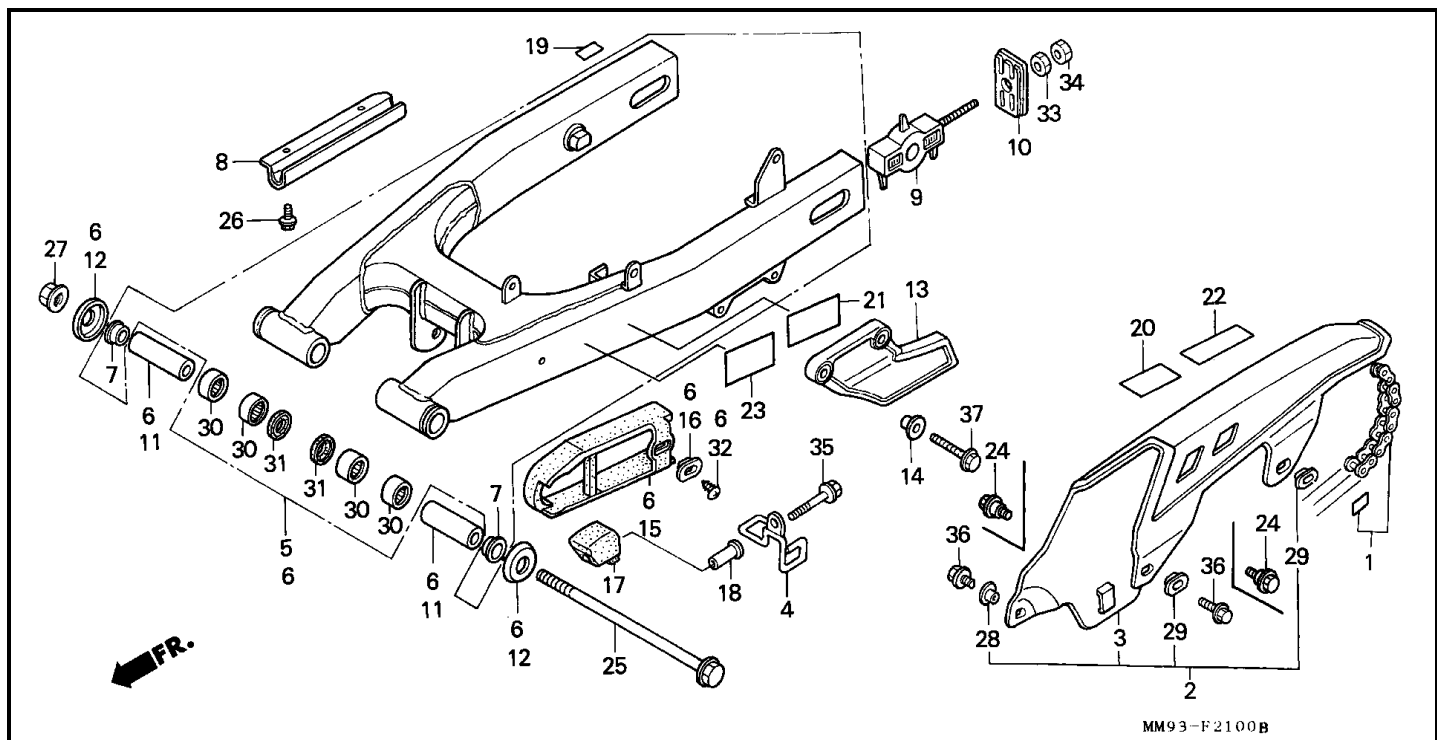
Bloque F-21 HORQUILLA TRASERA
