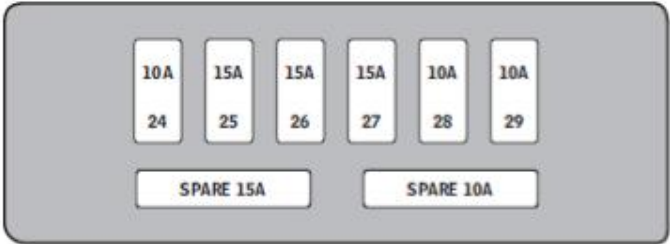
LOCALIZACIÓN: PARTE BAJA DE LA COLUMNA A, LADO DERECHO
