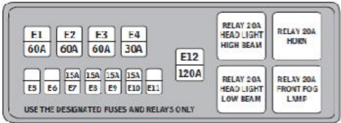
LOCALIZACIÓN: COMPARTIMIENTO DEL MOTOR (LADO DERECHO)
