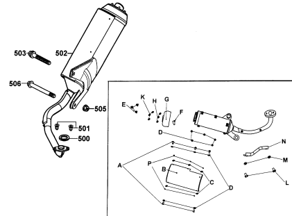
F14 TUBO DE ESCAPE -95-
