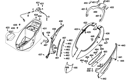
F12 PANEL CUERPO / COFRE -85-
