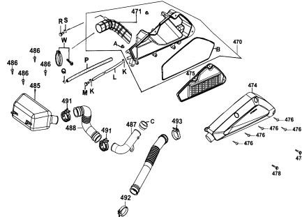
F13 FILTRO DE AIRE -91-
