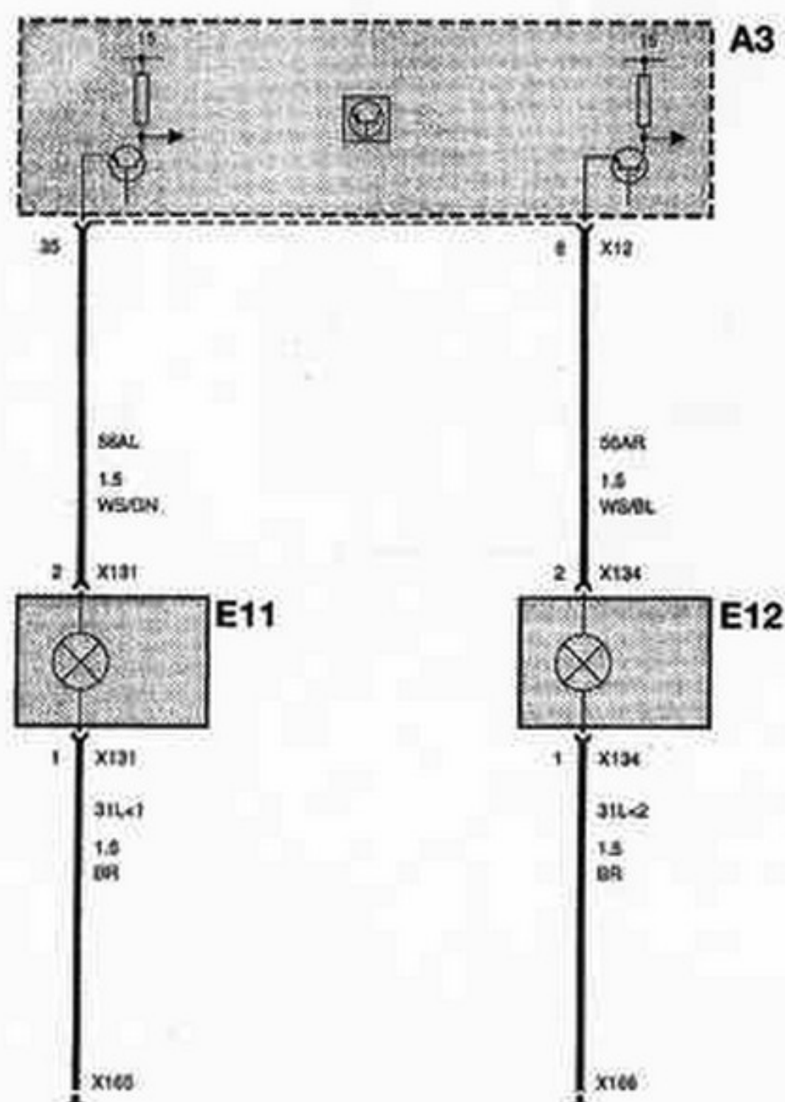
LUZ DE CARRETERA
