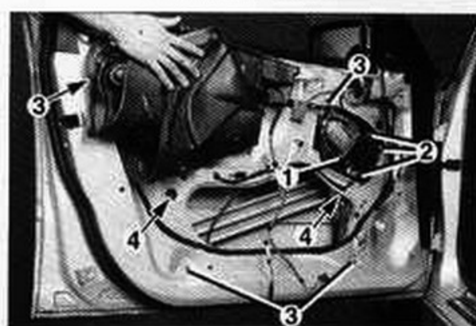
Desmontaje del mecanismo elevavinas delantero.
