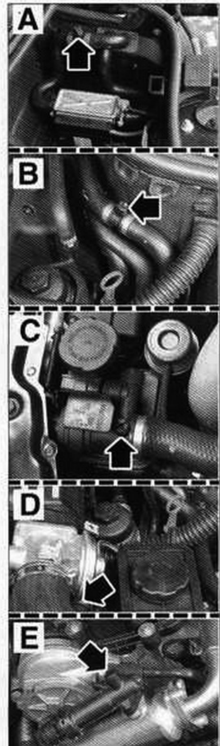
Situación de los tornillos de purga del circuito de refrigeración.
