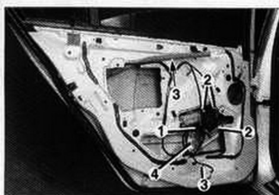
Desmontaje del mecanismo elevavinas trasero.
