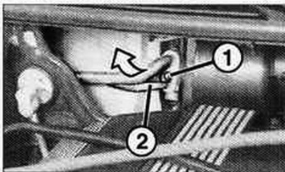
Desmontaje del tubo doble de climatización.
