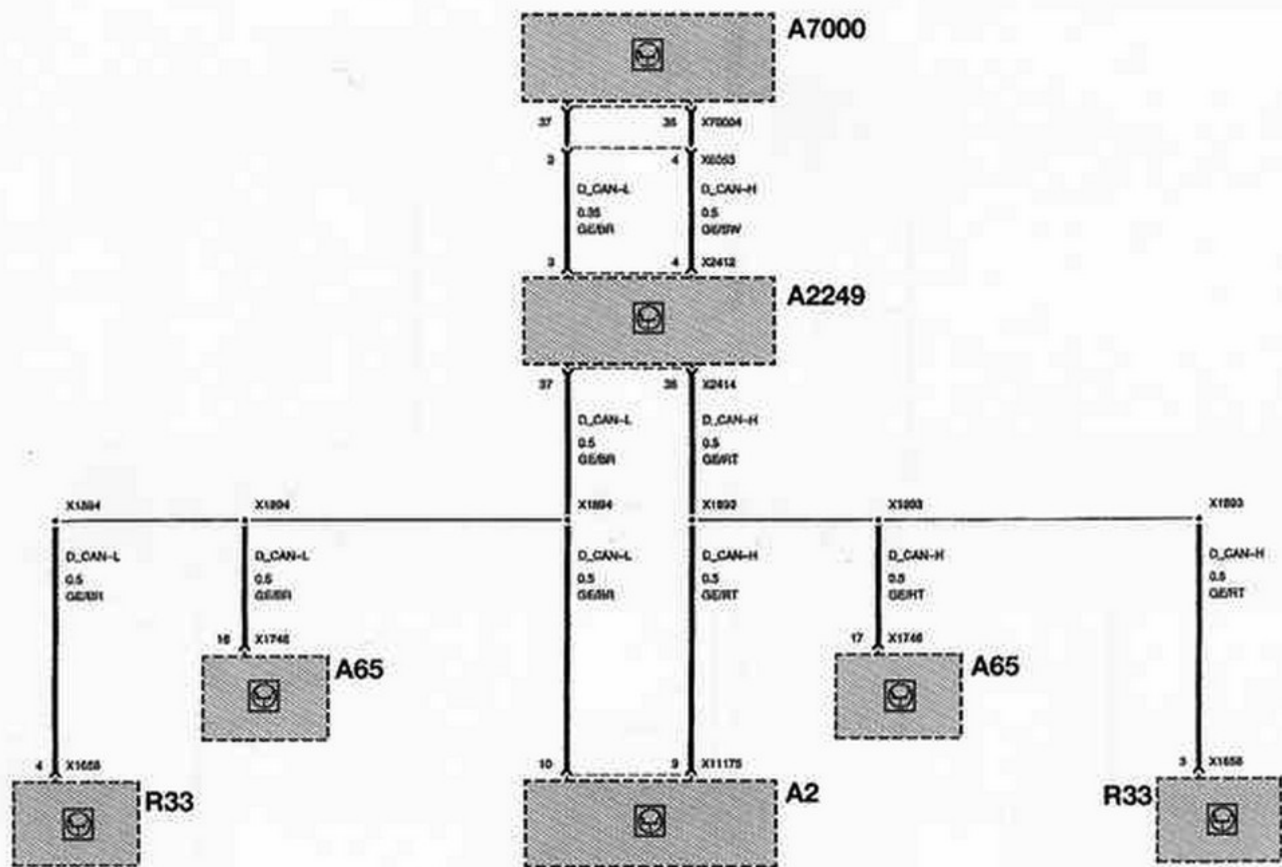
CUADRO DE INSTRUMENTOS. CONECTOR BUS CAN.
