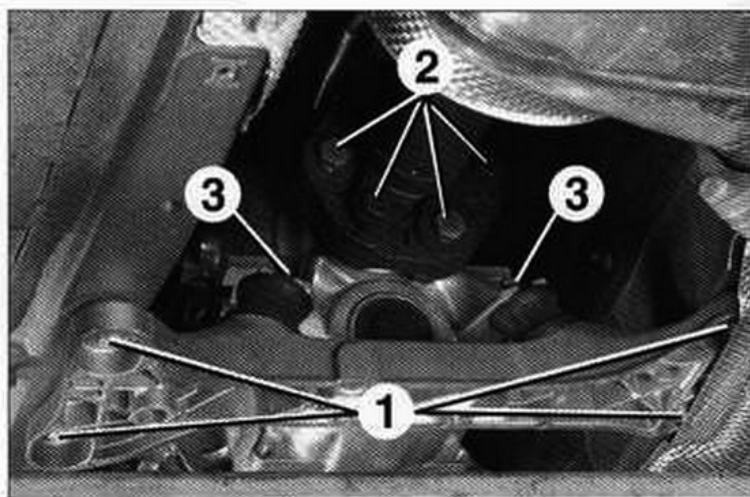
Desmontaje de la caja de velocidades.
