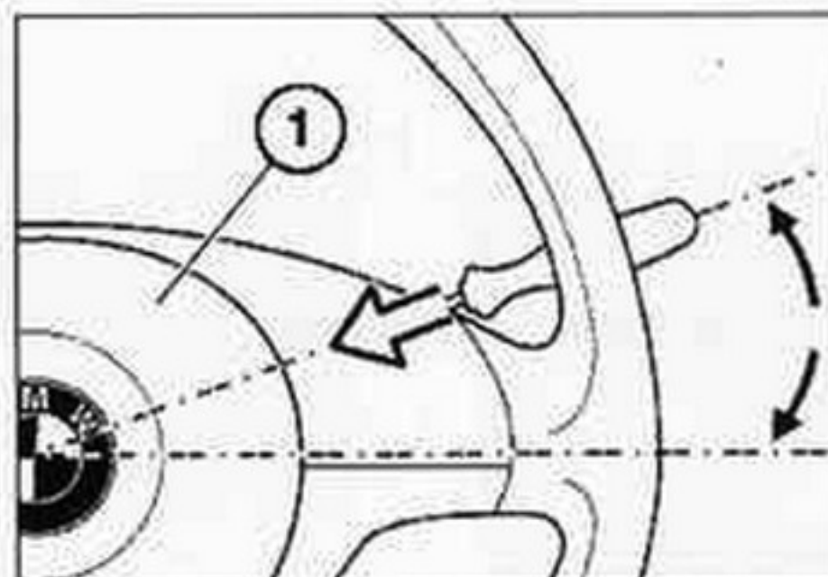
Desmontaje del airbag conductor (1).
