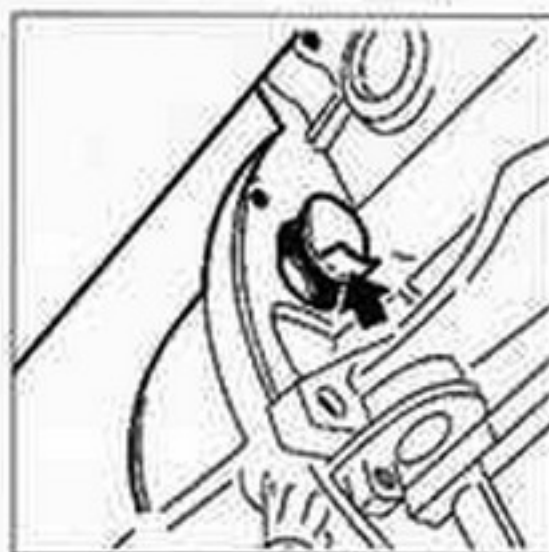
Desmontaje del capuchón del taladro de acceso a los tornillos de fijación del convertidor de par.
