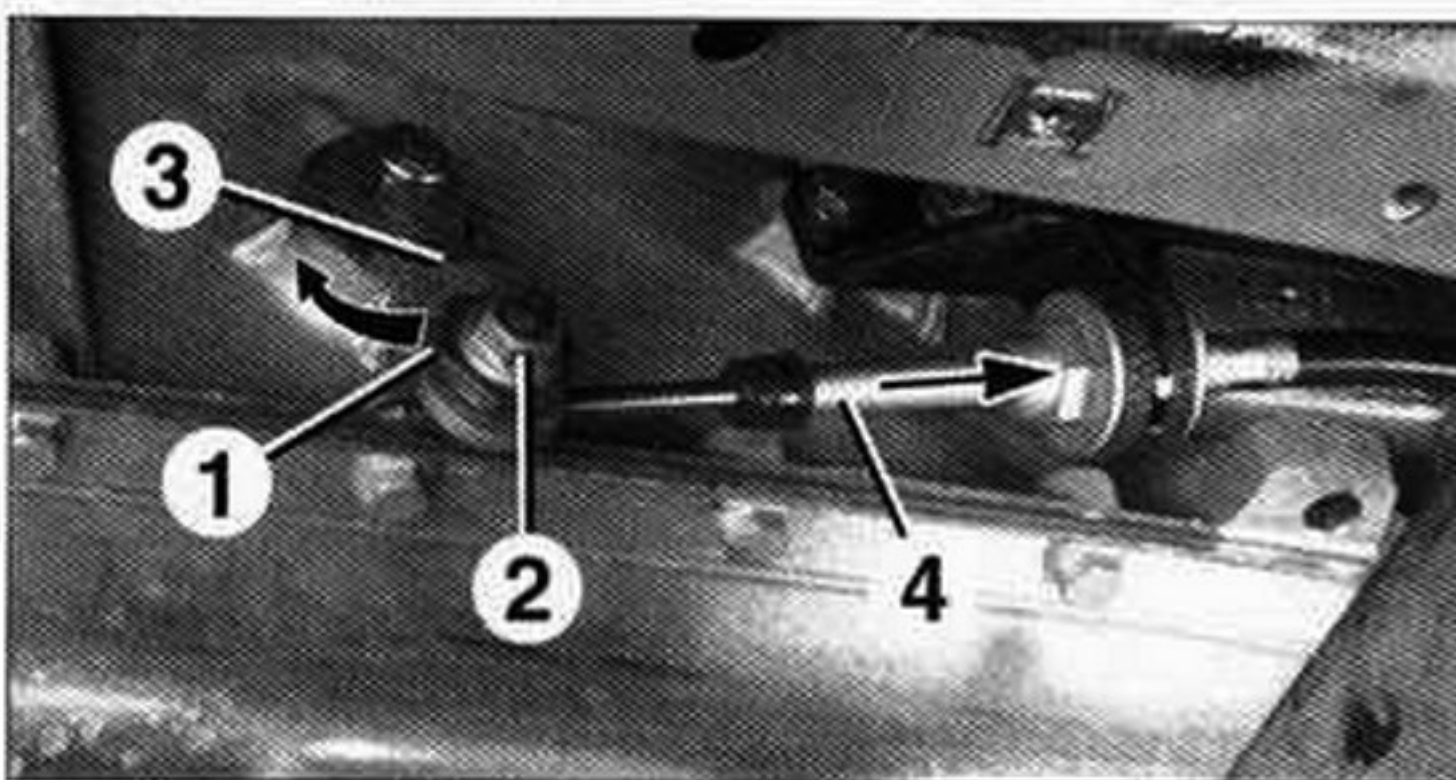
Método de reglaje del cable de selección.
