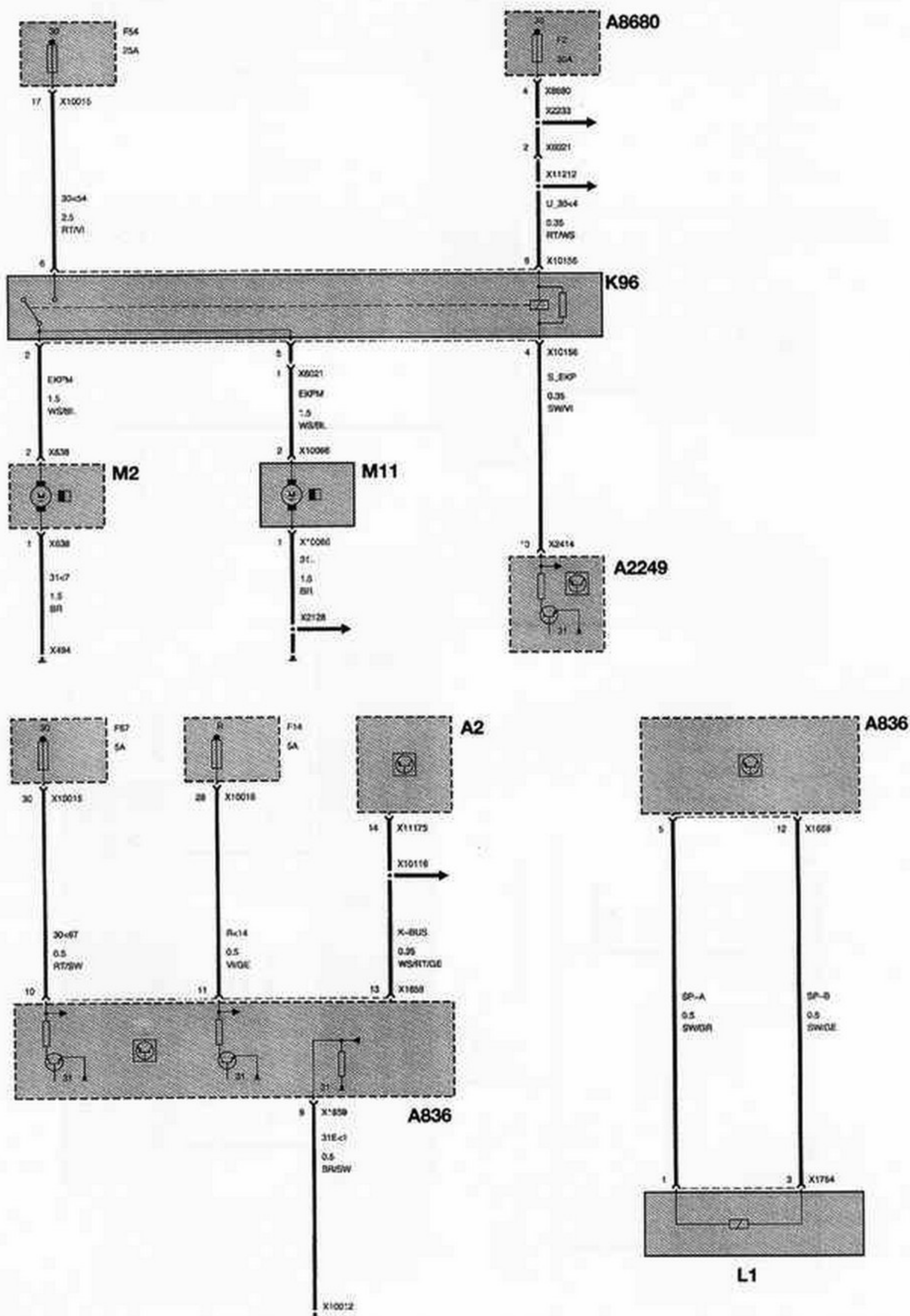
BOMBAS DE ALIMENTACION DE COMBUSTIBLE - SISTEMA ANTIARRANQUE
