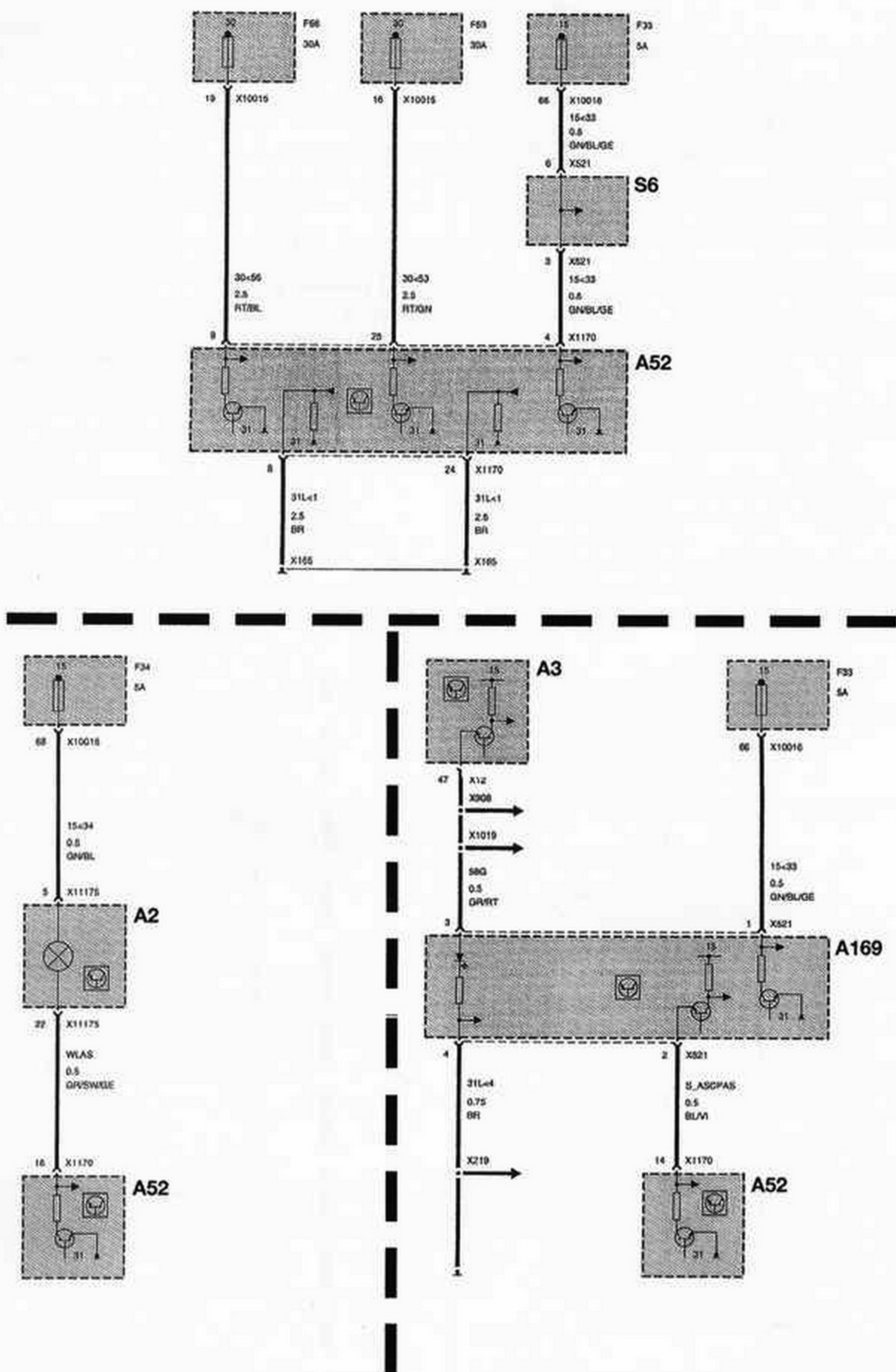
ALIMENTACION ABS, TESTIGO ABS EN CUADRO INSTRUMENTOS, TECLA ASC.
