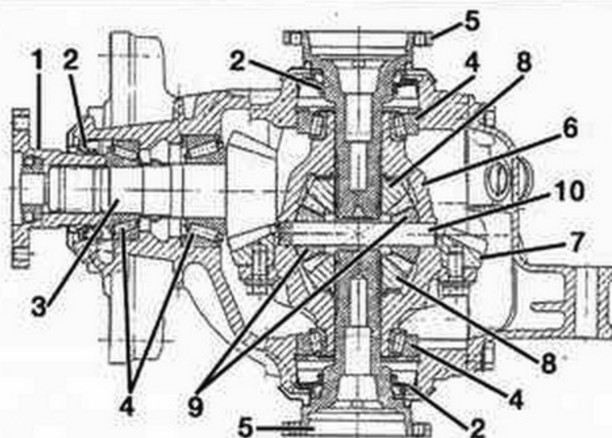
CORTE LONGITUDINAL DEL PUENTE TRASERO.
