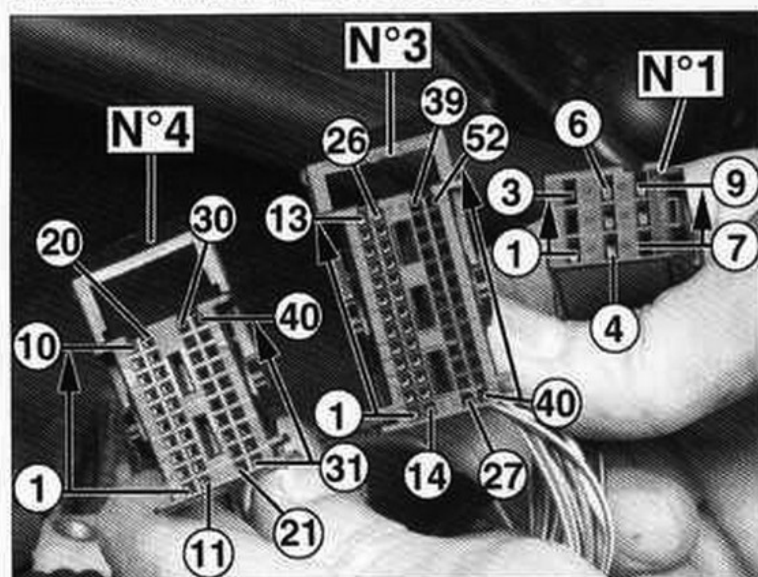
Identificación de los bornes de los conectores del calculador de gestión motor.
