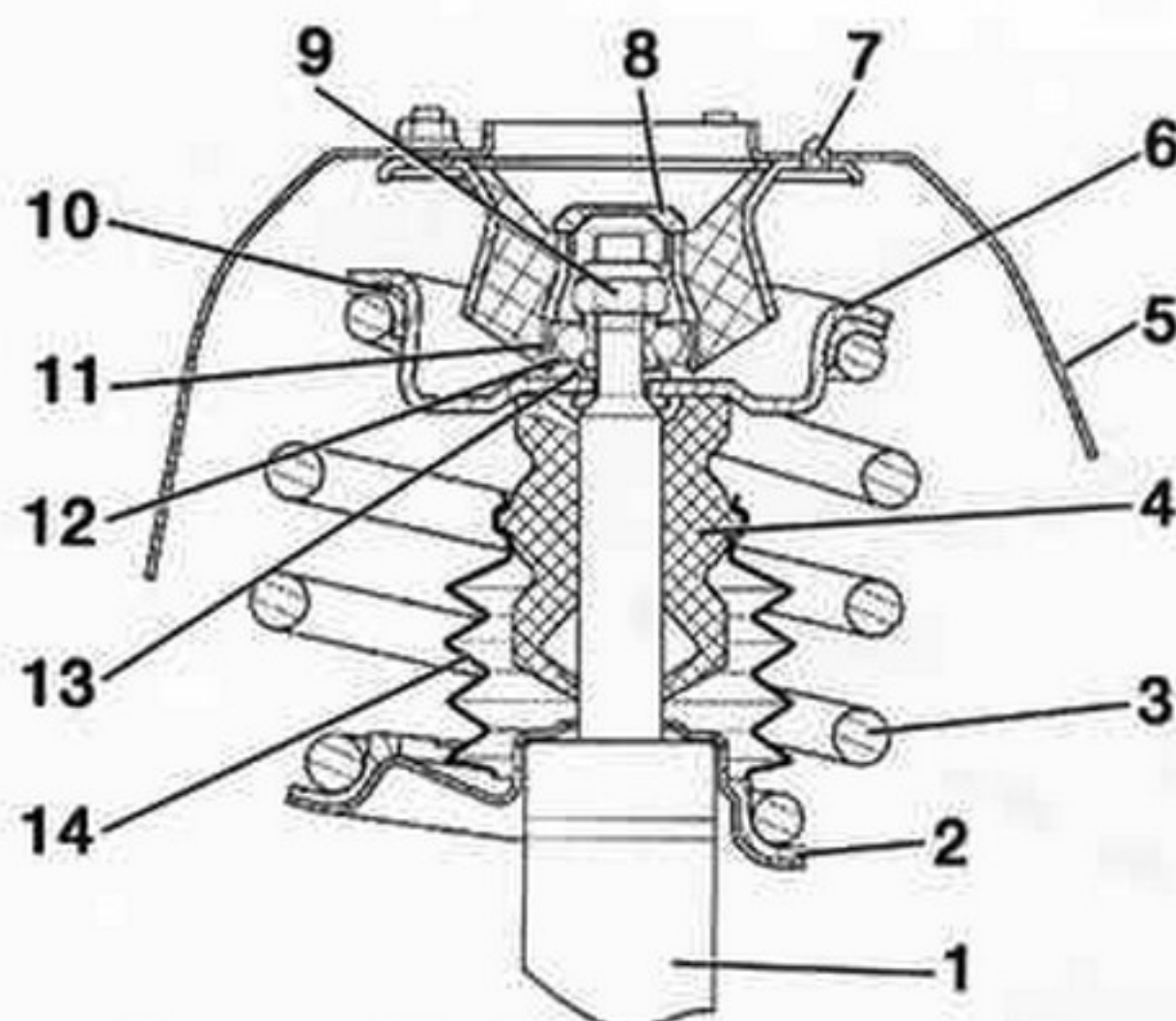
PIEZAS DE UN ELEMENTO DE SUSPENSION
