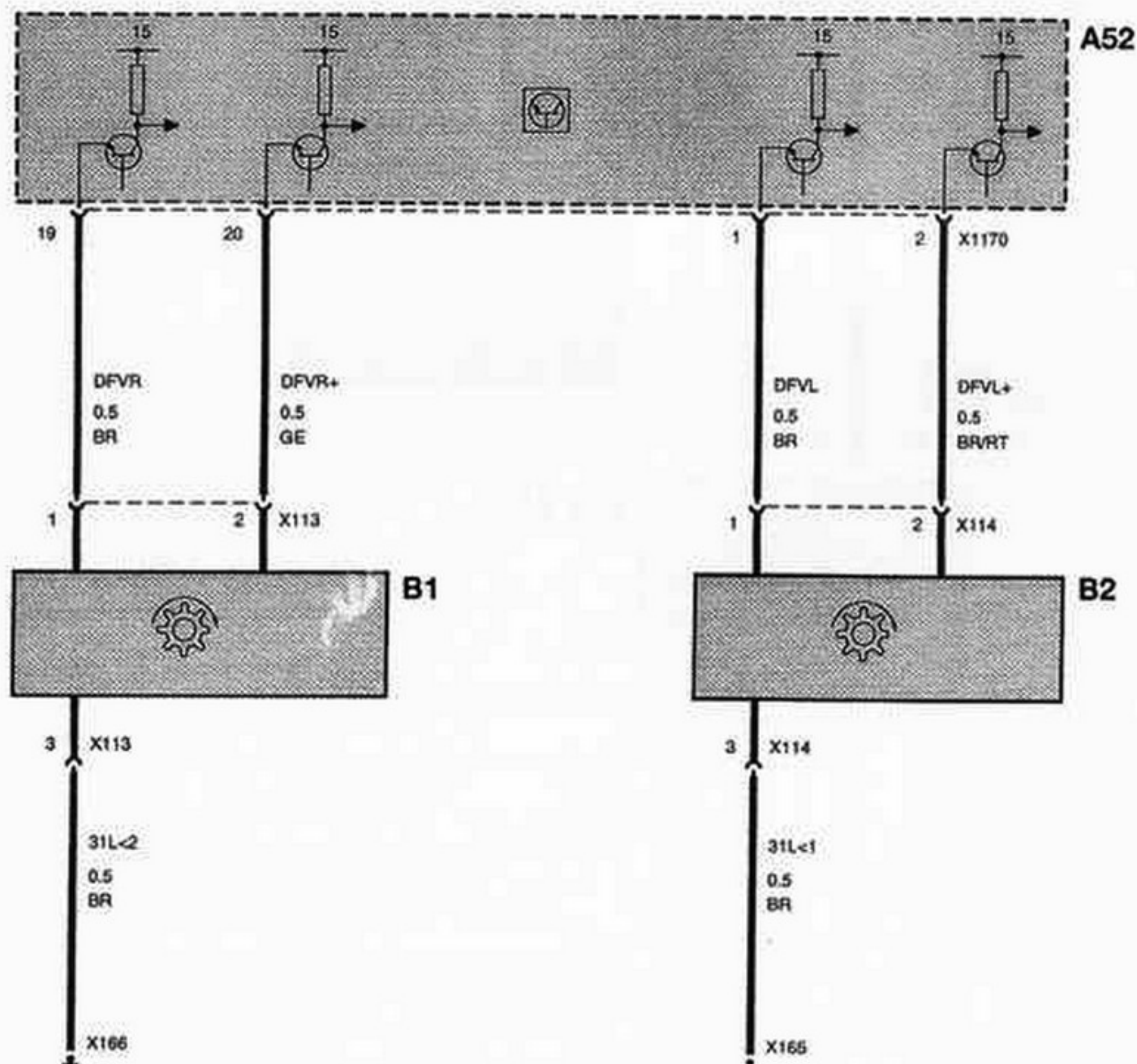
CAPTADORES DE VELOCIDAD DE RUEDAS
