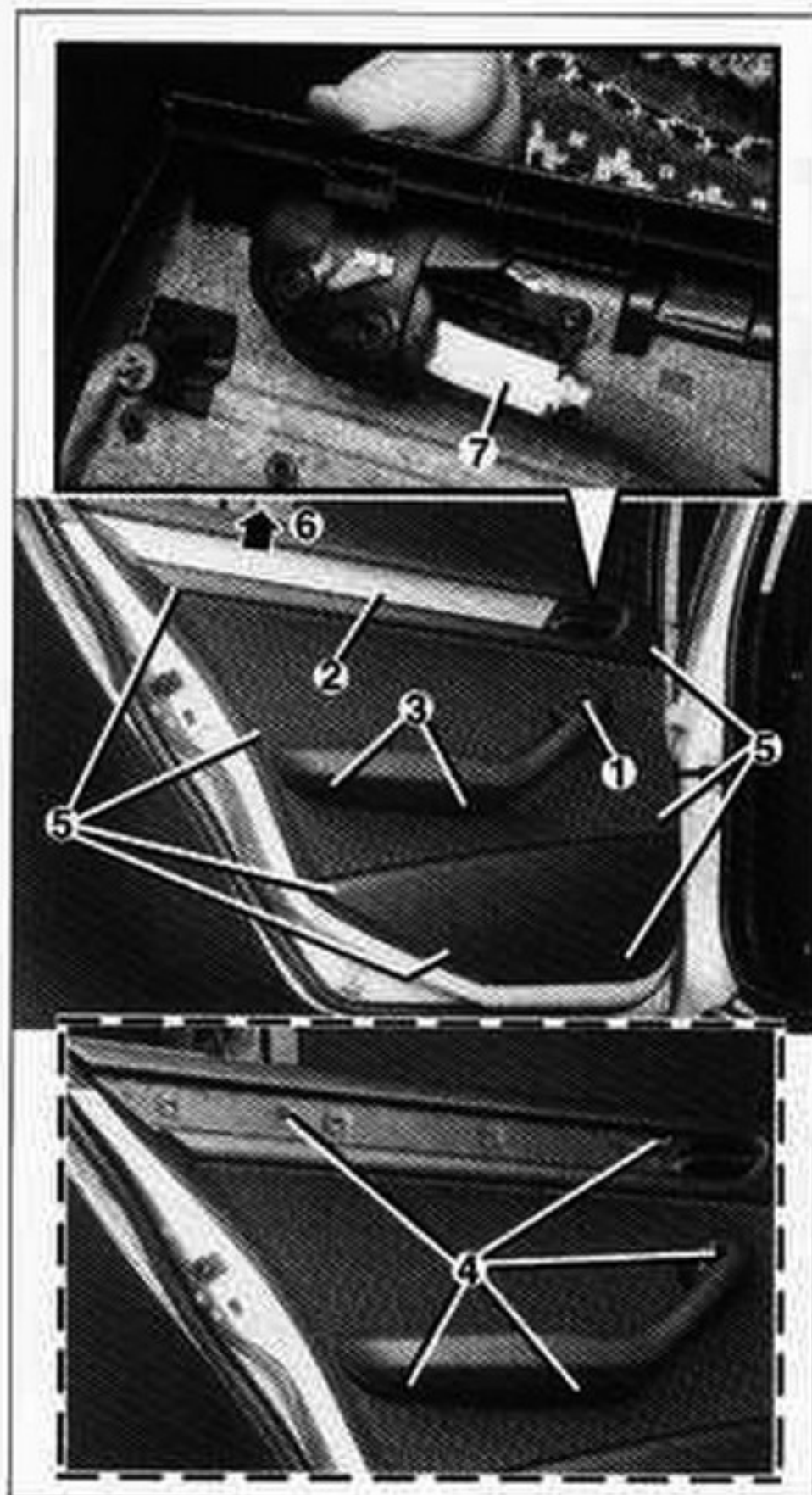
Desmontaje de la guarnición de puerta trasera.
