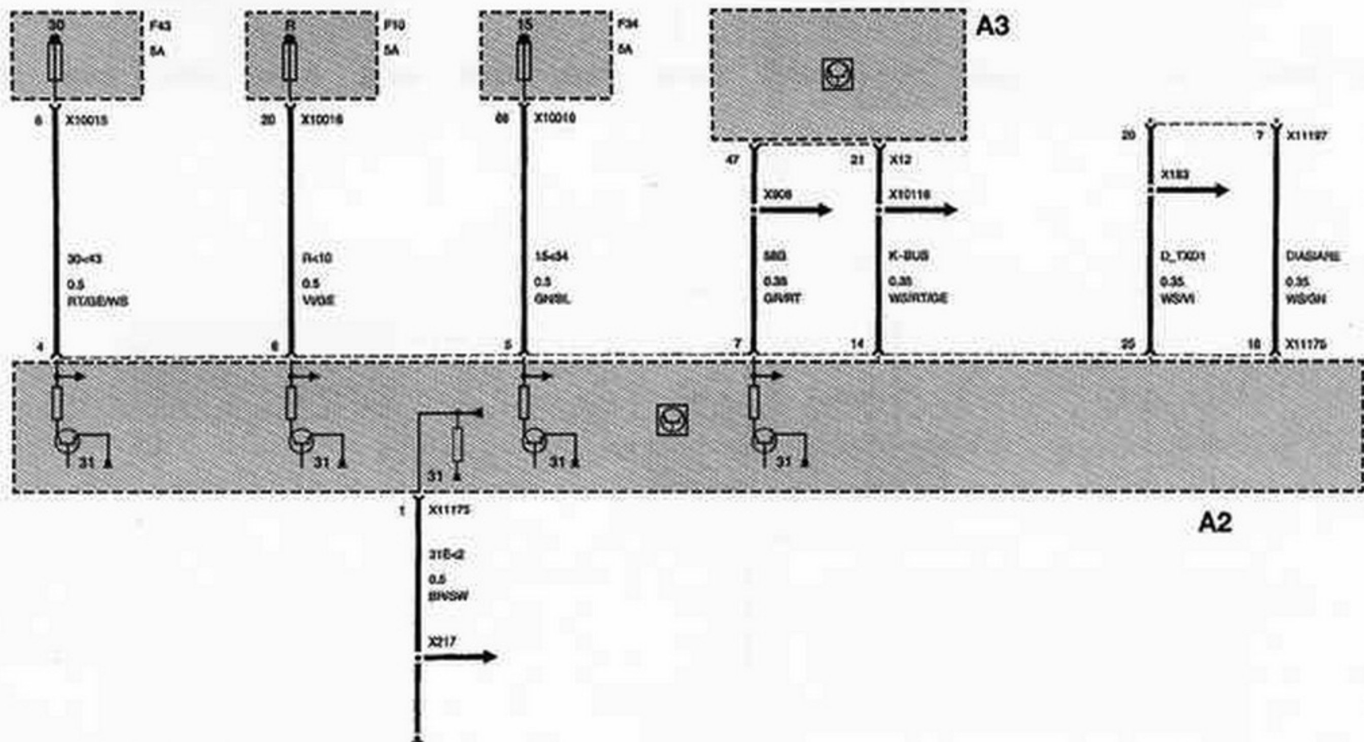
CUADRO DE INSTRUMENTOS. ALIMENTACION.
