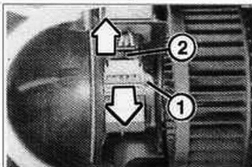
Desmontaje de la resistencia de motoventilador.
