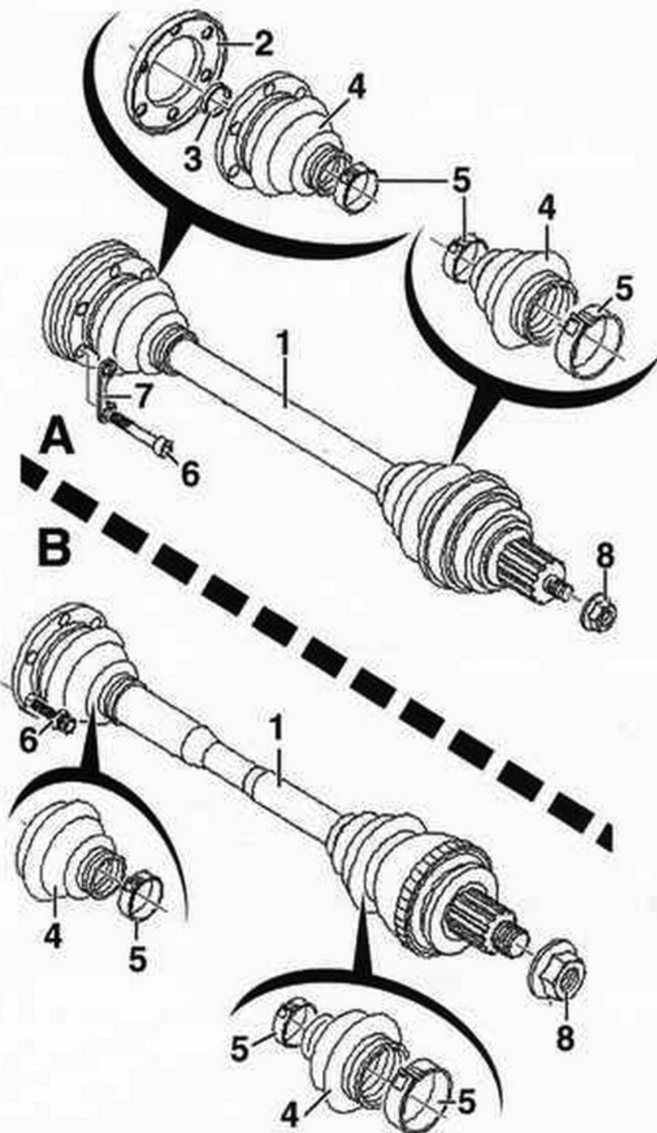
SEMIEJES DE RUEDA.
