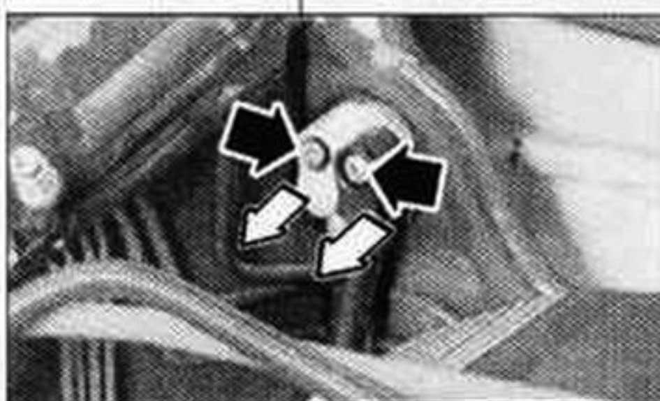
Desmontaje del tubo de aspiración de climatización.
