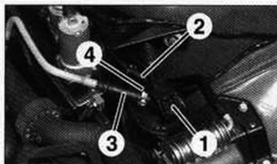
ALIMENTACION DE COMBUSTIBLE. 1. Tornillo de fijación del captador de presión de alimentación - 2. Tubería de alimentación que viene del depósito - 3. Tubería de alimentación hacia la bomba de alta presión - 4. Tornillo de sujeción del filtro.
