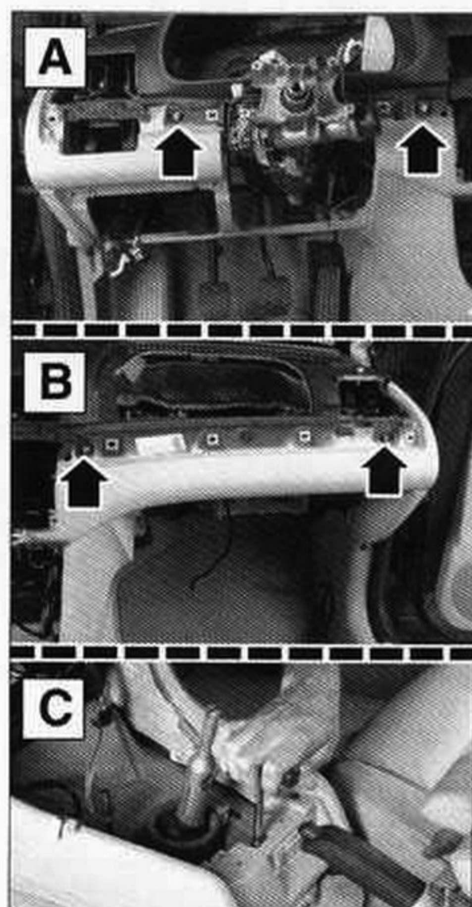
Situación de las tuercas de salpicadero.
