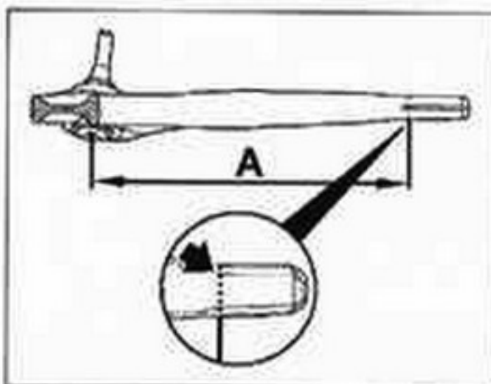
Medición de la cota "A" del triángulo.
