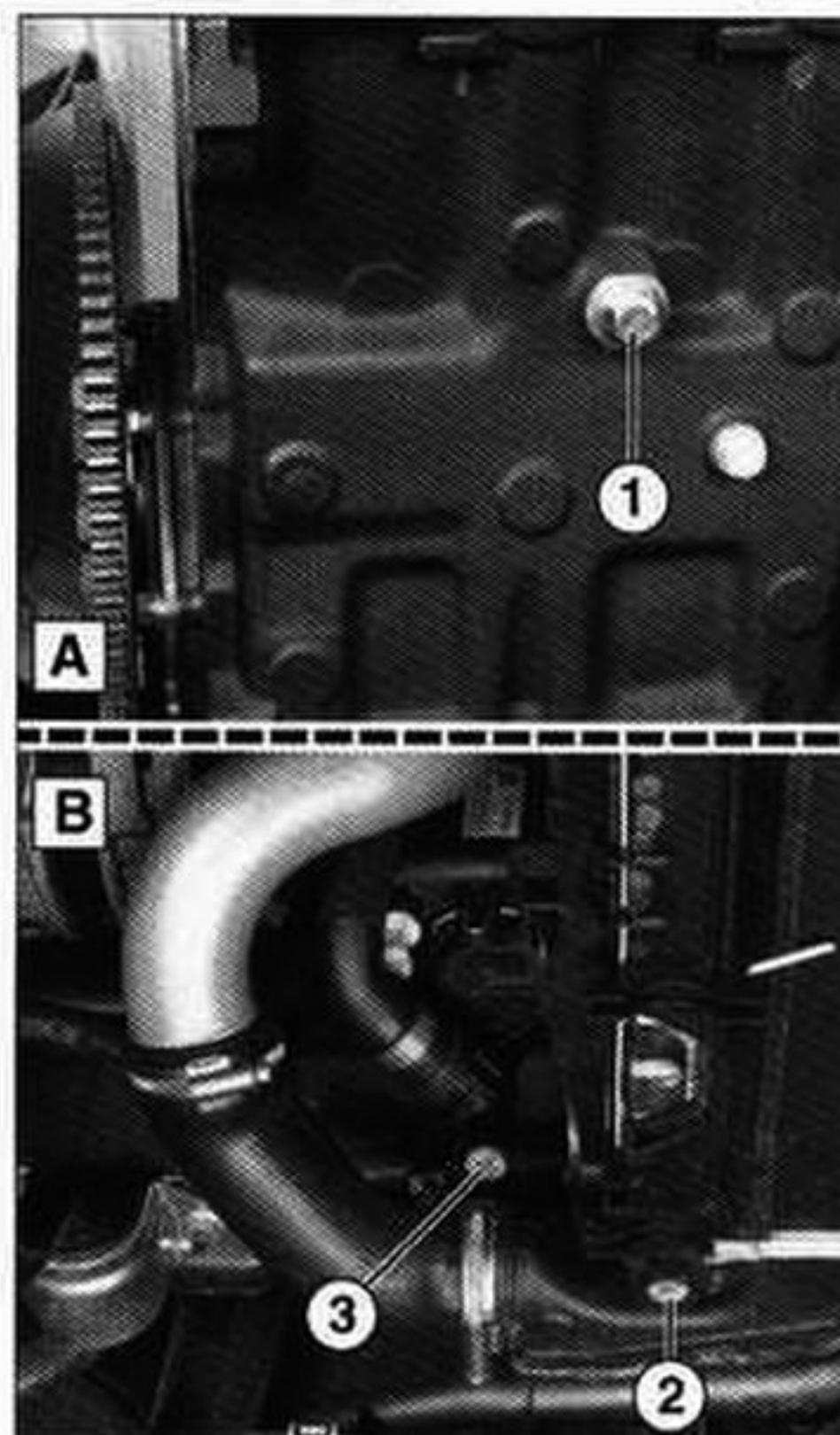
Vaciado del circuito de refrigeración.
