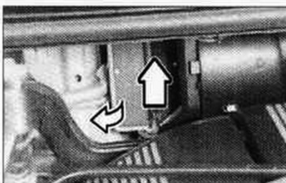
Desmontaje de la trampilla de aire reciclado.
