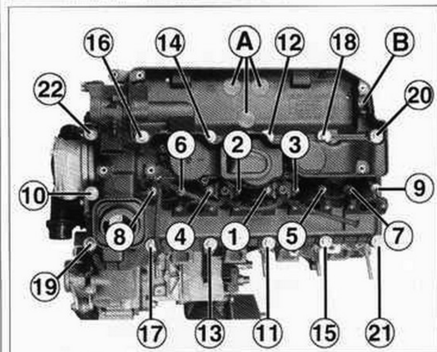
Tapa de culata.
