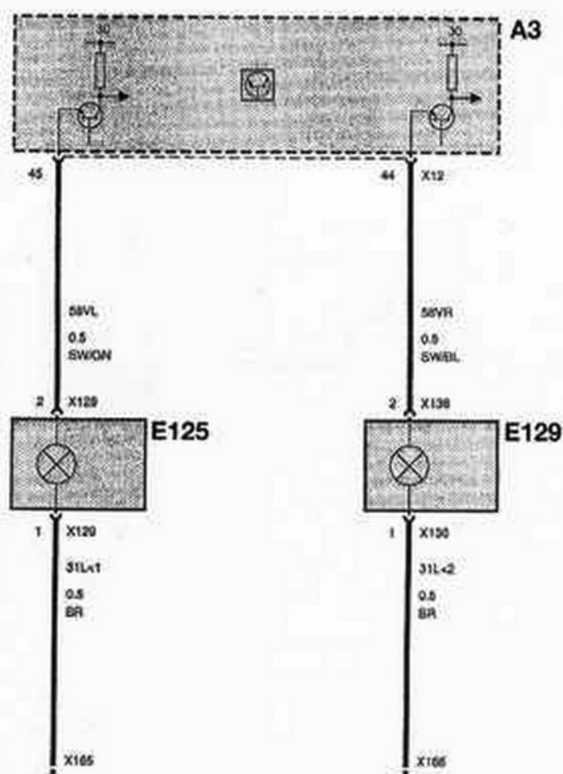
LUZ POSICION DELANTERA
