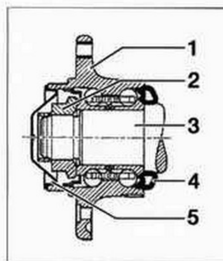
Corte de un cubo delantero.
