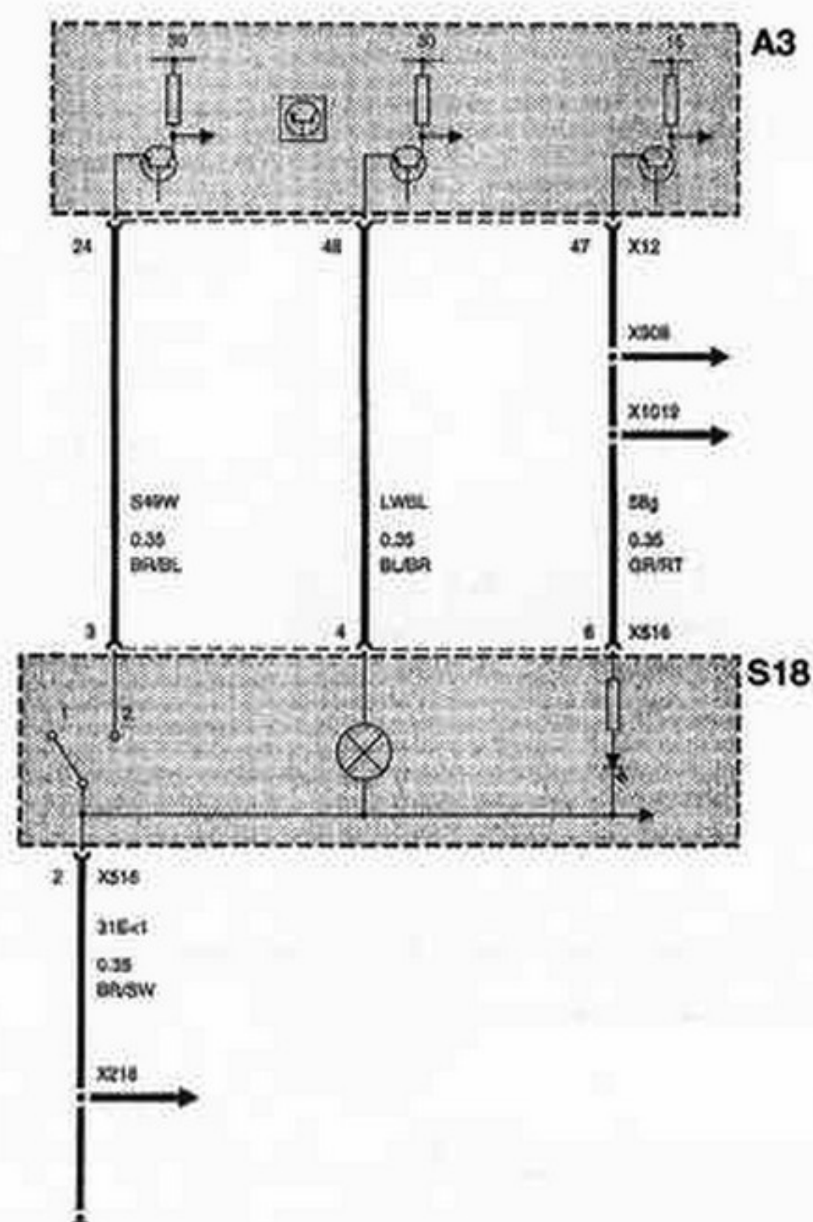
INTERRUPTOR INTERMITENTES EMERGENCIA
