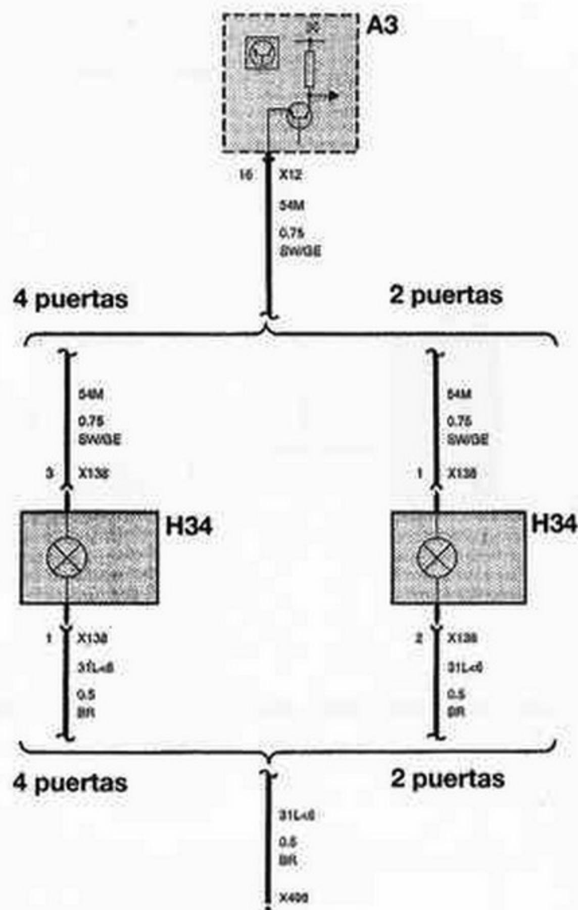
TERCERA LUZ STOP
