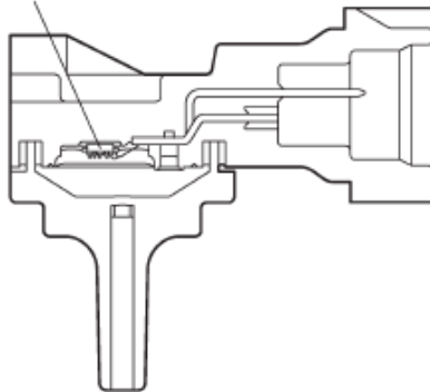
Unidad Sensor
