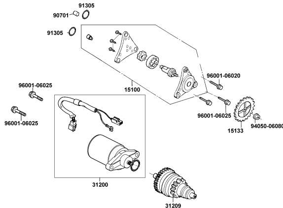
E07 MOTOR DE ARRAN. (Pág. 033)
