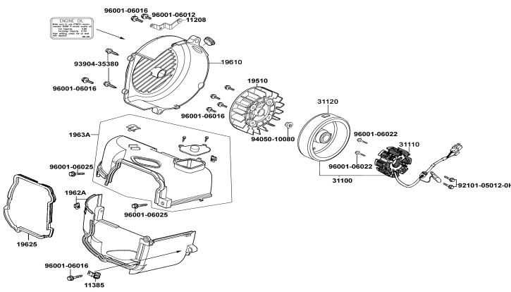
E08 ALTERNADOR (Pág. 035)
