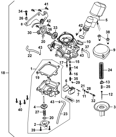
E05 CARBURADOR (Pág. 023)
