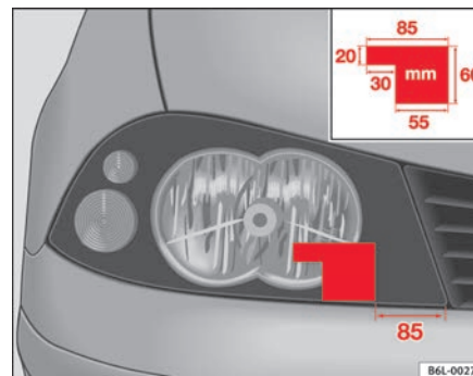
Fig. 107 Faro derecho
