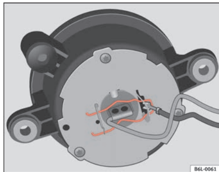
Fig. 151 Faros antiniebla
