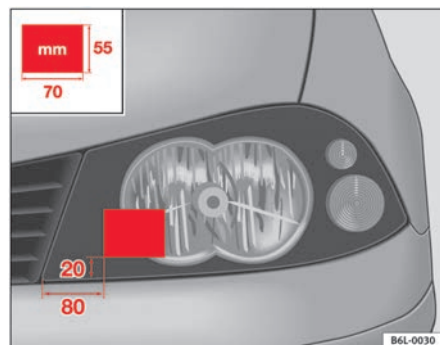
Fig. 110 Faro izquierdo
