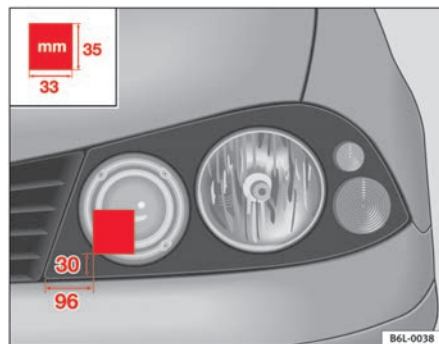
Fig. 118 Faro izquierdo
