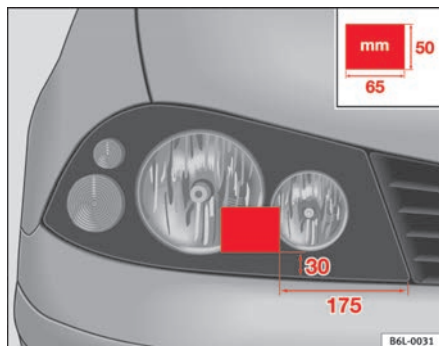
Fig. 111 Faro derecho
