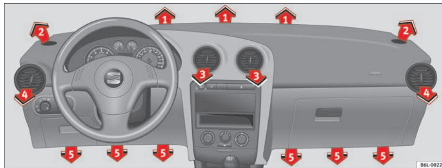
Fig. 89 Difusores de aire
