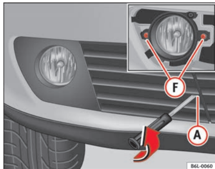
Fig. 150 Faros antiniebla
