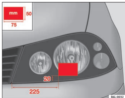
Fig. 112 Faro izquierdo
