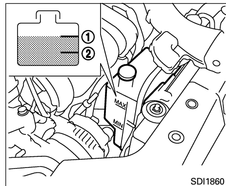
Motor HR16DE/MR18DE
