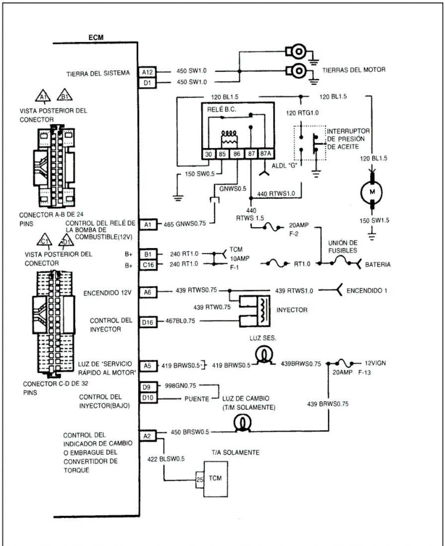
Fig. 2 Diagrama de Cableado del ECM(1 de 4)
