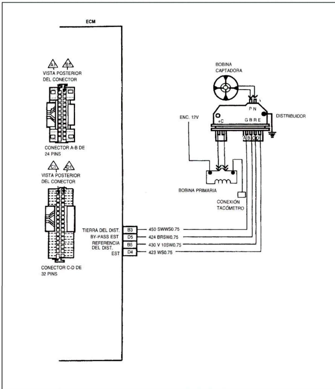
Fig. 4 Diagrama de Cableado del ECM(3 de 4)
