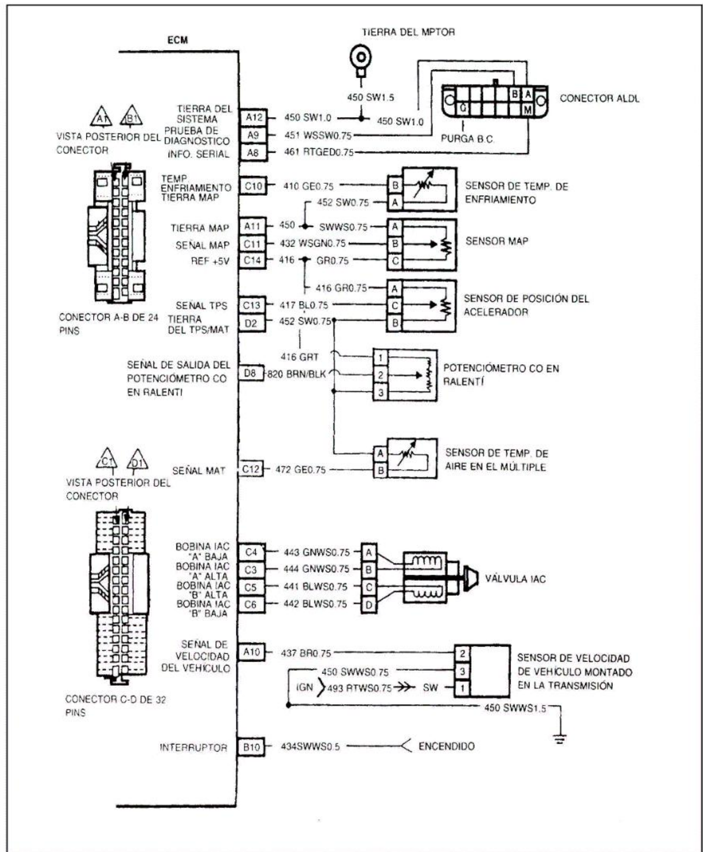
Fig. 3 Diagrama de Cableado del ECM(2 de 4)
