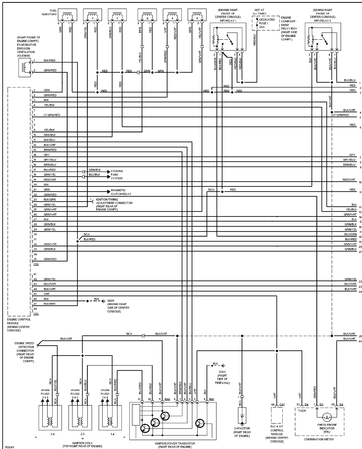
Fig. 37: Wiring Diagram (3000GT 3.0L DOHC - 1 Of 3)
