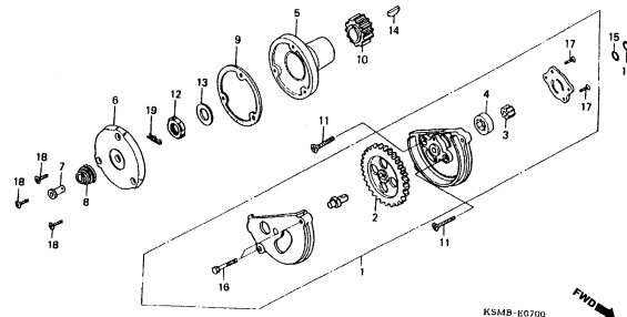
M-7 Bomba de Óleo / Oil Pump / Bomba de Aceite
