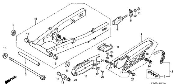
C-20 Garfo Traseiro / Swingarm / Horquilla Trasera
