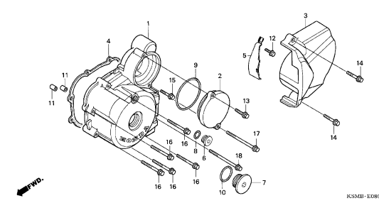
M-8 Tampa Lateral Esquerda / Left Crankcase Cover / Cubierta Izquierda del Cáster Motor
