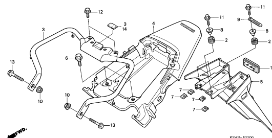
C-22 Pára-Lama Traseiro / Rear Fender / Parafango Trasero
