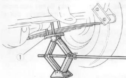
Front wheel jack-up Mise de la roue avant sur cric Levantando la rueda delantera Opkrikken van een voorwiel
