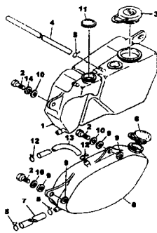
FIG.21 TANQUE DE ÓLEO
