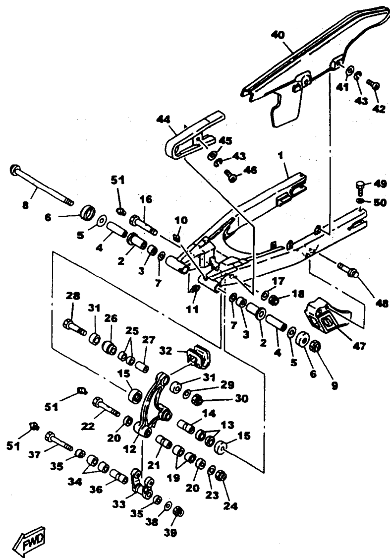
FIG. 22 - GARFO TRASEIRO
