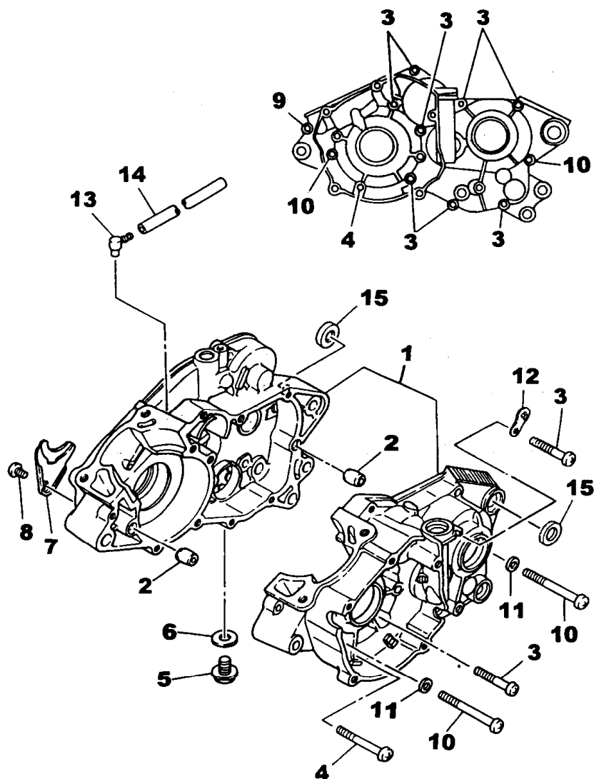
FIG. 09 - CARCAÇA DO MOTOR
