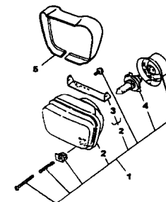
FIG.44 SISTEMA ELÉTRICO 2 P.51
