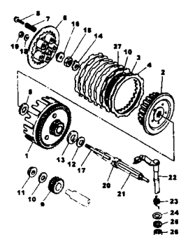
FIG.12 FRICÇÃO P.16
