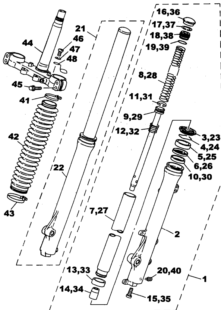
FIG. 25 - GARFO DIANTEIRO
