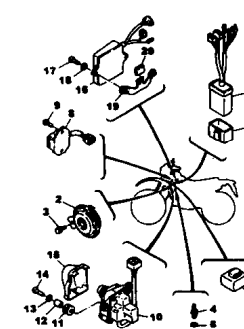
FIG.44 SISTEMA ELÉTRICO 2 P.51
