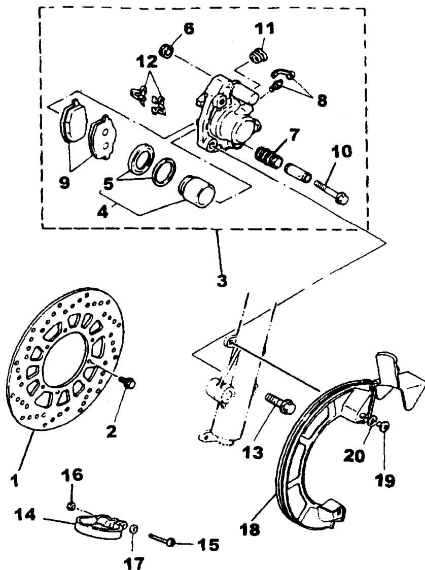
FIG. 29 - DISCO E PINÇA DE FREIO DIANTEIRO
