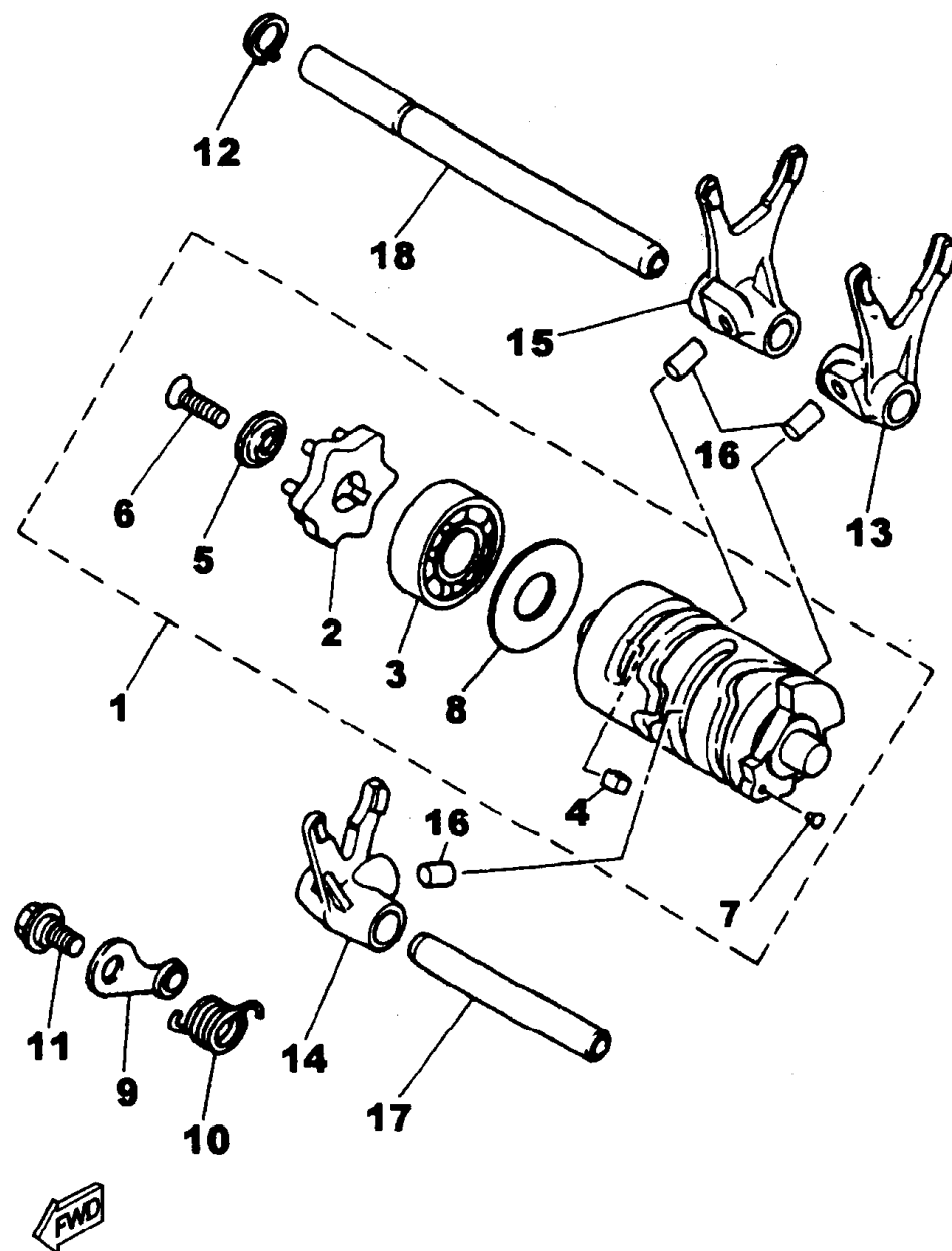
FIG. 15 - EIXO TRAMBULADOR
