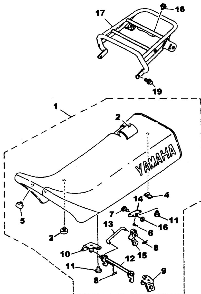
FIG. 27 - ASSENTO
