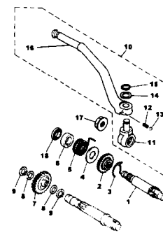
FIG.11 PEDAL DE PARTIDA P.15
