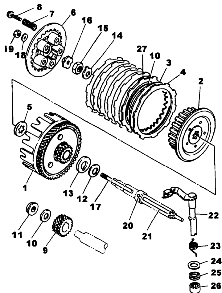
FIG. 12 - FRICÇÃO
