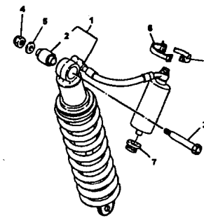
FIG.23 AMORTECEDOR TRASEIRO
