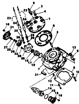
FIG.5 BOMBA DE ÓLEO P.8
