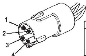
CONECTOR DEL SENSOR DE OXIGENO DE ENTRADA (LADO DEL MAZO)
