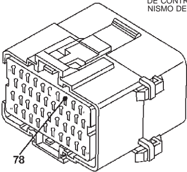
CONECTOR DEL MODULO DE CONTROL DEL MECA- NISMO DE TRANSMISION
