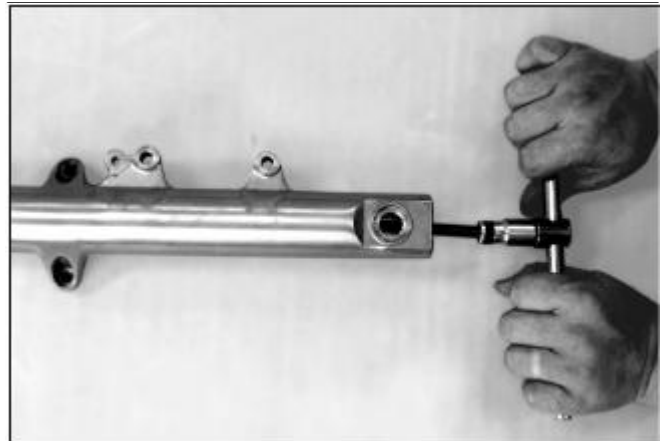
Bottom Case
