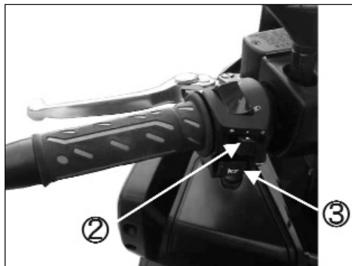
(2) Conmutador de intermitentes | (3) Botón del claxon
