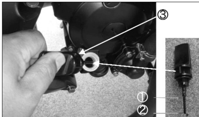
(1) Nivel máximo | (2) Nivel mínimo | (3) Varilla de nivel
