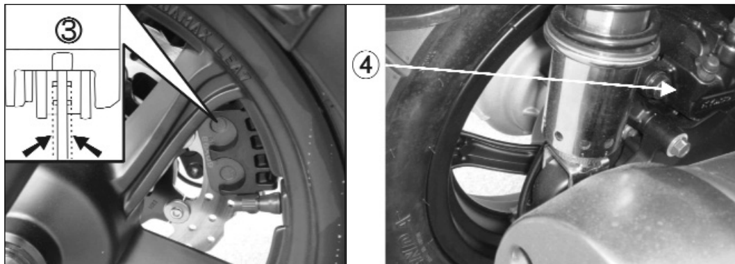
(Izda.) Desgaste pastillas freno delantero | (Dcha.) Desgaste pastillas freno trasero
