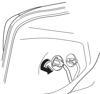
Luces de freno/cola (Tipo bombilla)
