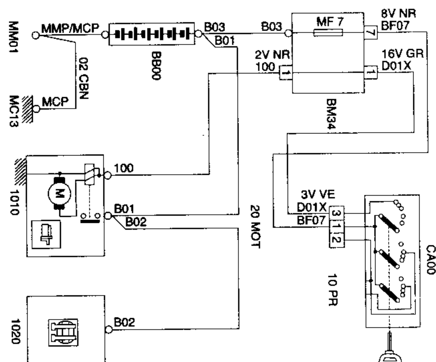
BB00 BATERÍA (MOTOR TU3JP)
