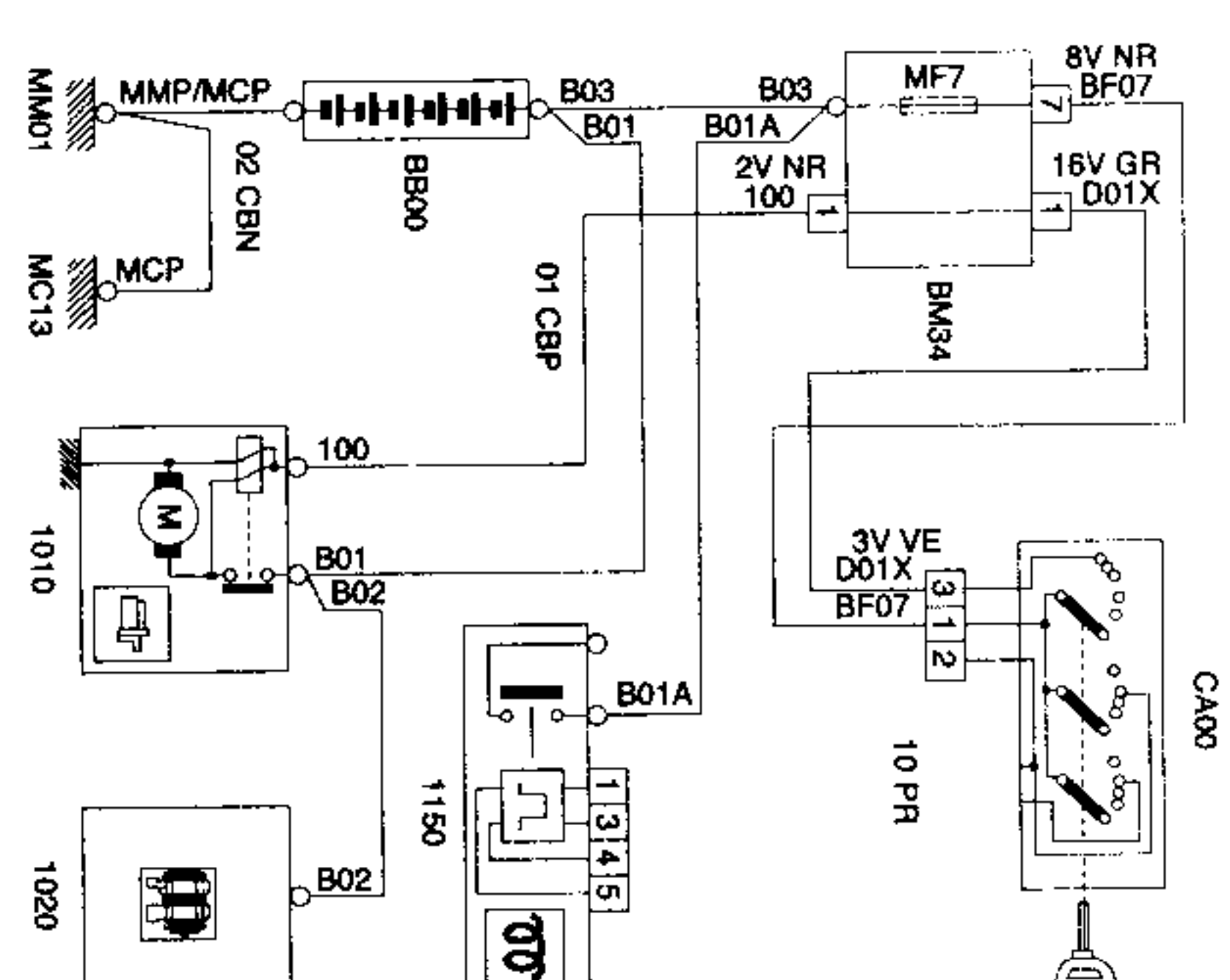
BB00 BATERÍA (MOTOR DW10TD)
