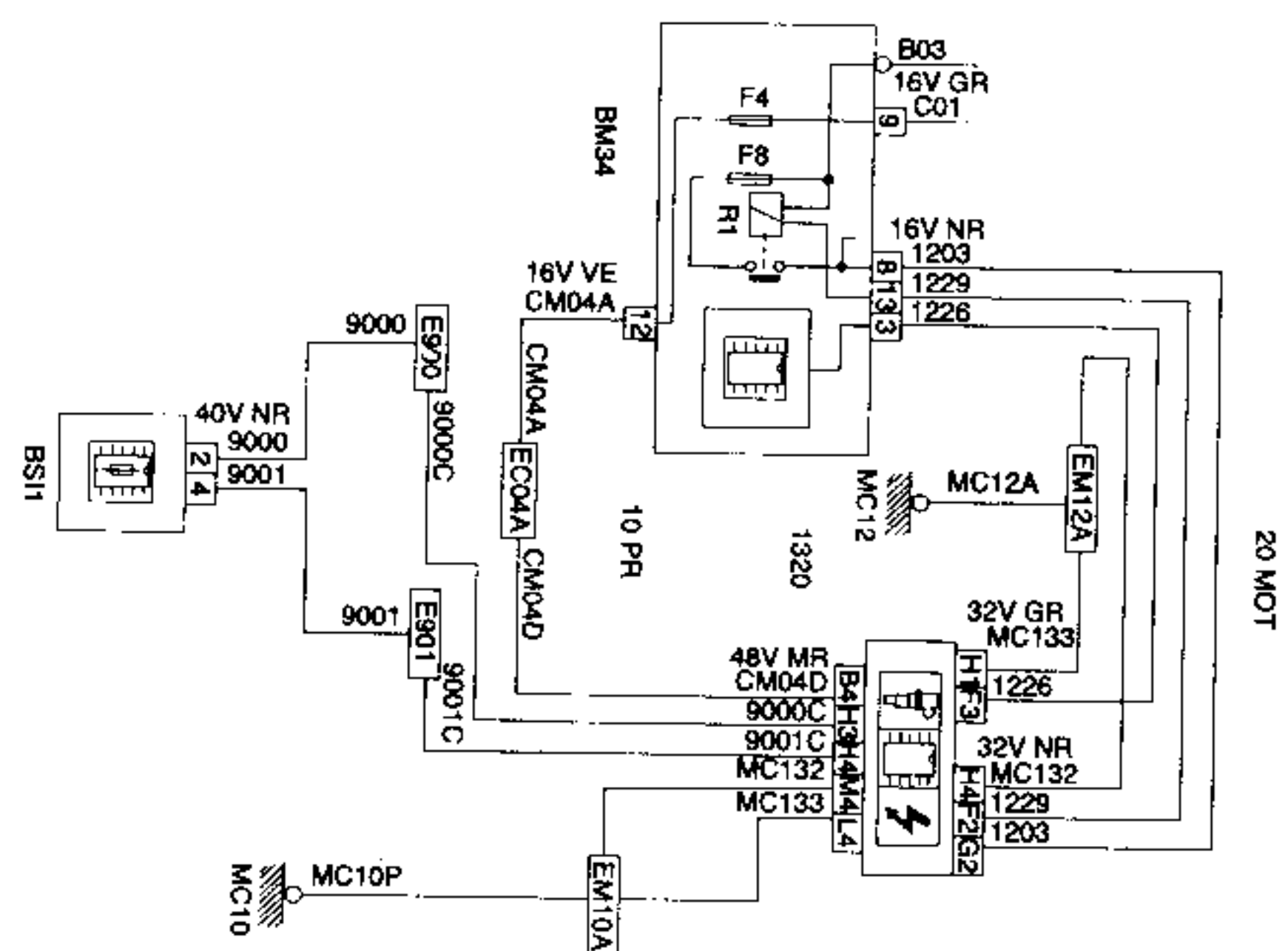
1320 CALCULADOR MOTOR (MOTOR TU5JP4 VERSIÓN EUROPA)
