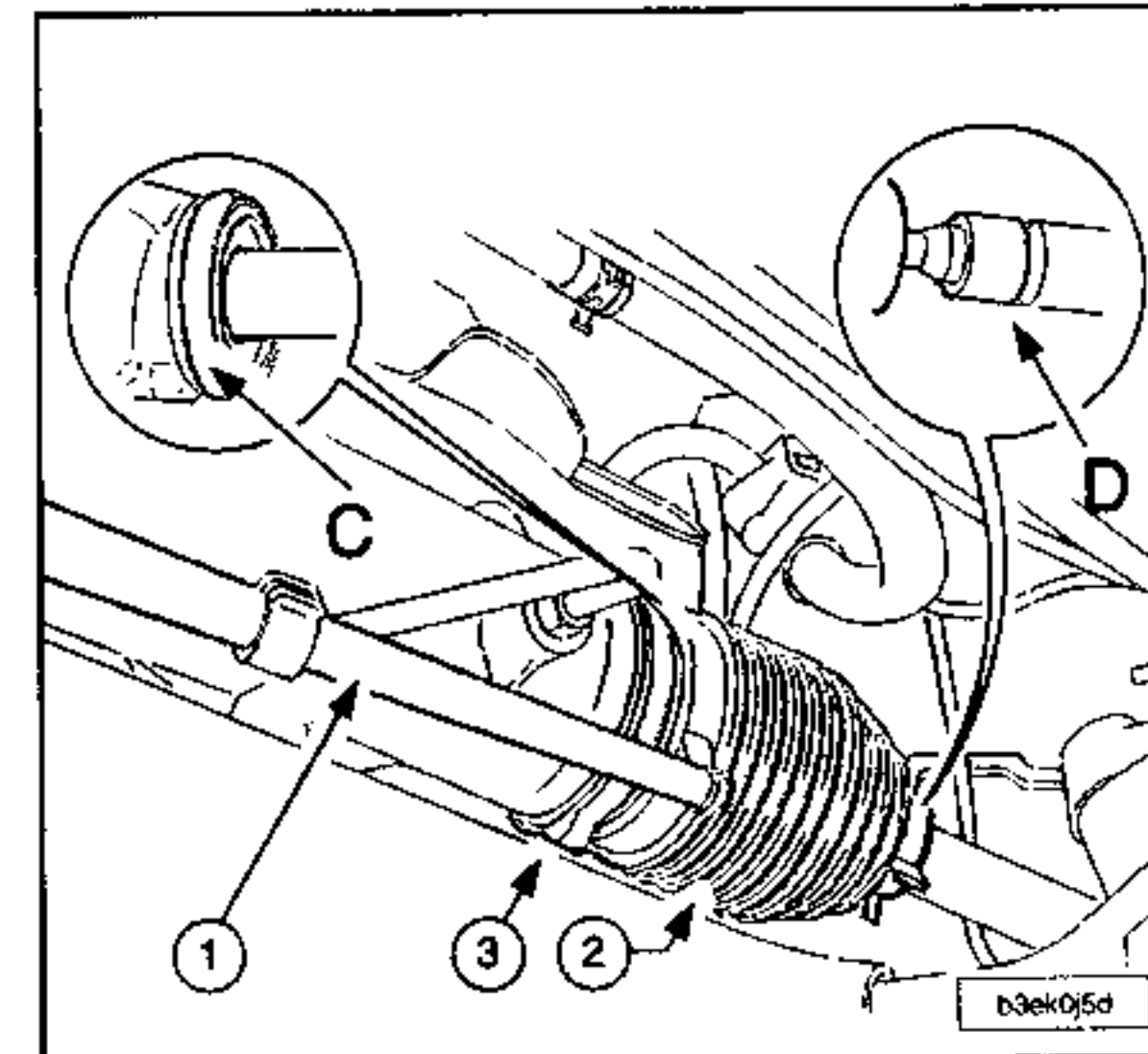
Montar un guardapolvos nuevo (2).
