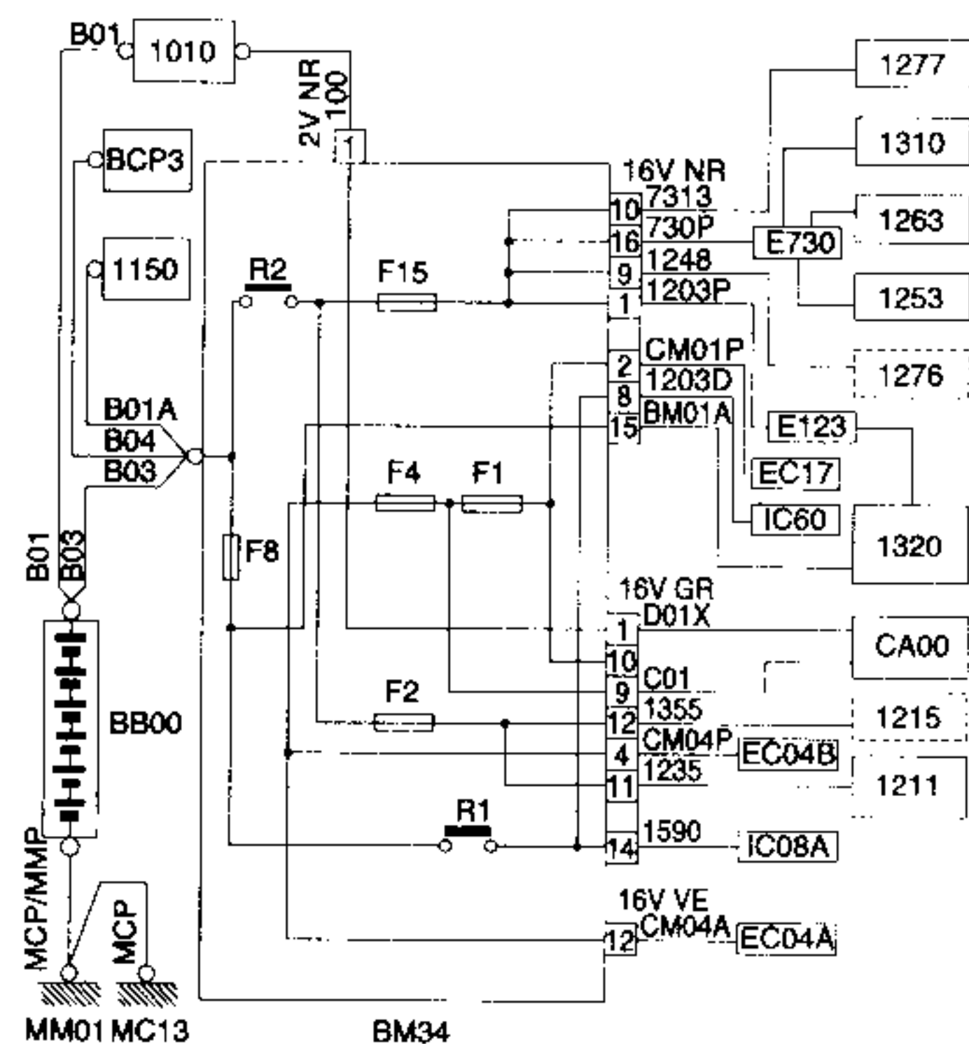
BM34 CAJETÍN DE SERVICIO MOTOR 34 FUSIBLES (MOTOR DW10TD CALCULADOR SIEMENS PARA DW10)
