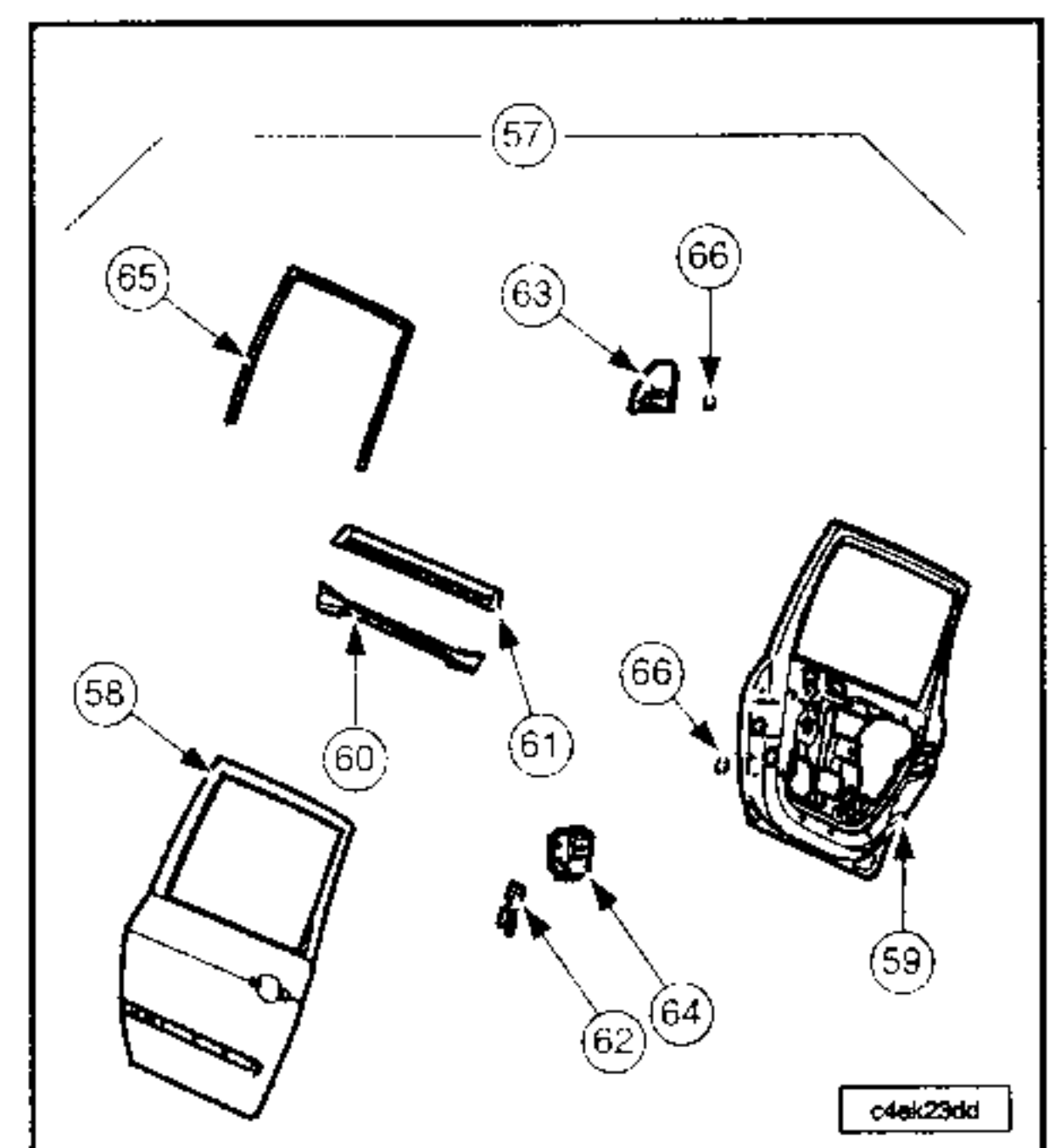
Break 5 puertas.
