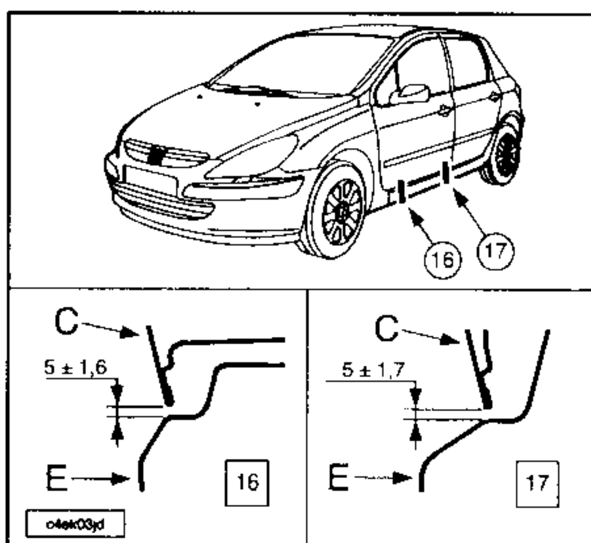
C.-Puerta. E.-Larguero.
