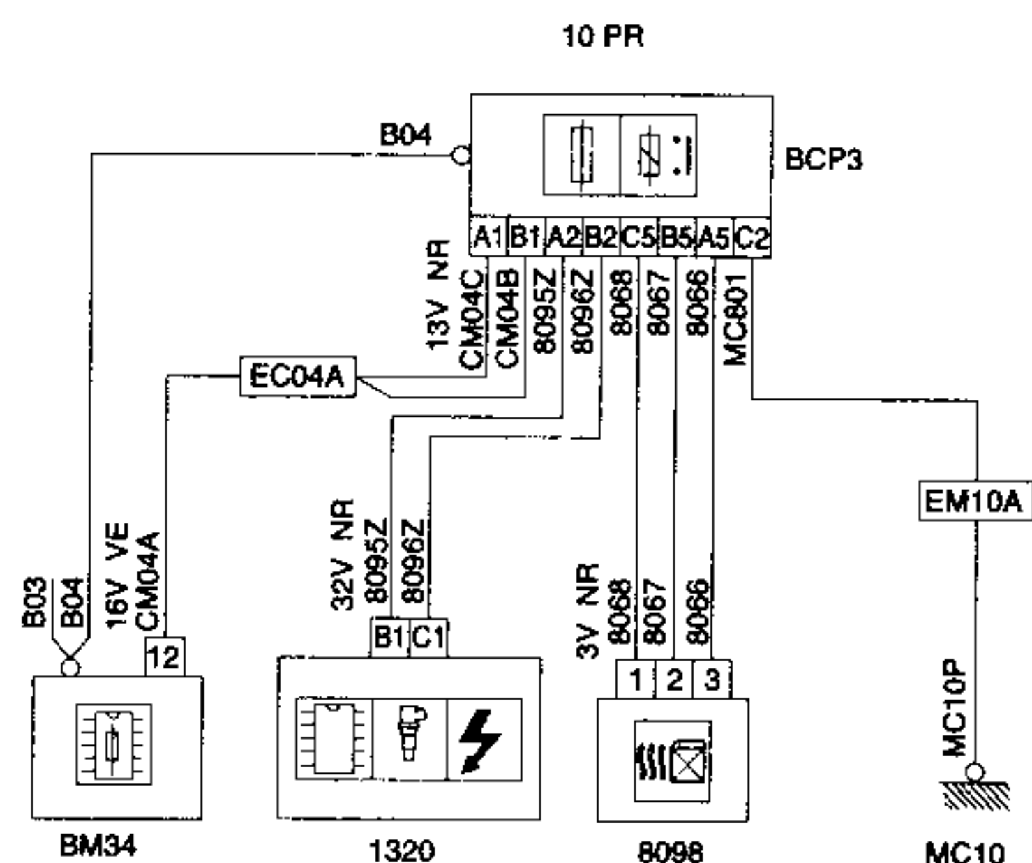
BCP3 CAJETÍN CONMUTACIÓN PROTECCIÓN 3º RELÉ (MOTOR DW10TD CALCULADOR SIEMENS PARA DW10)
