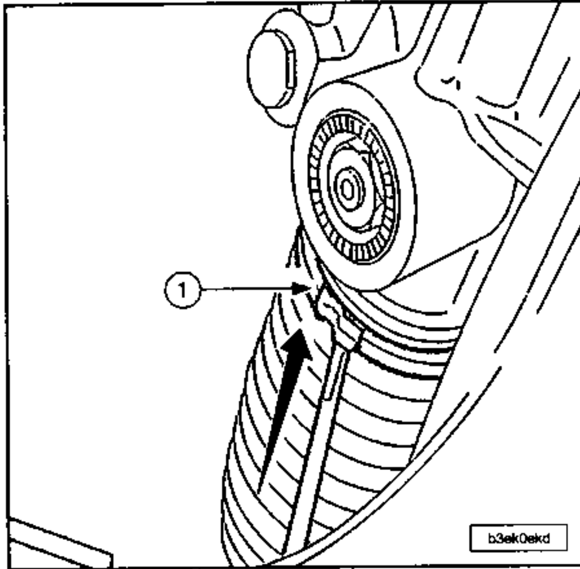
Quitar la abrazadera (1).
