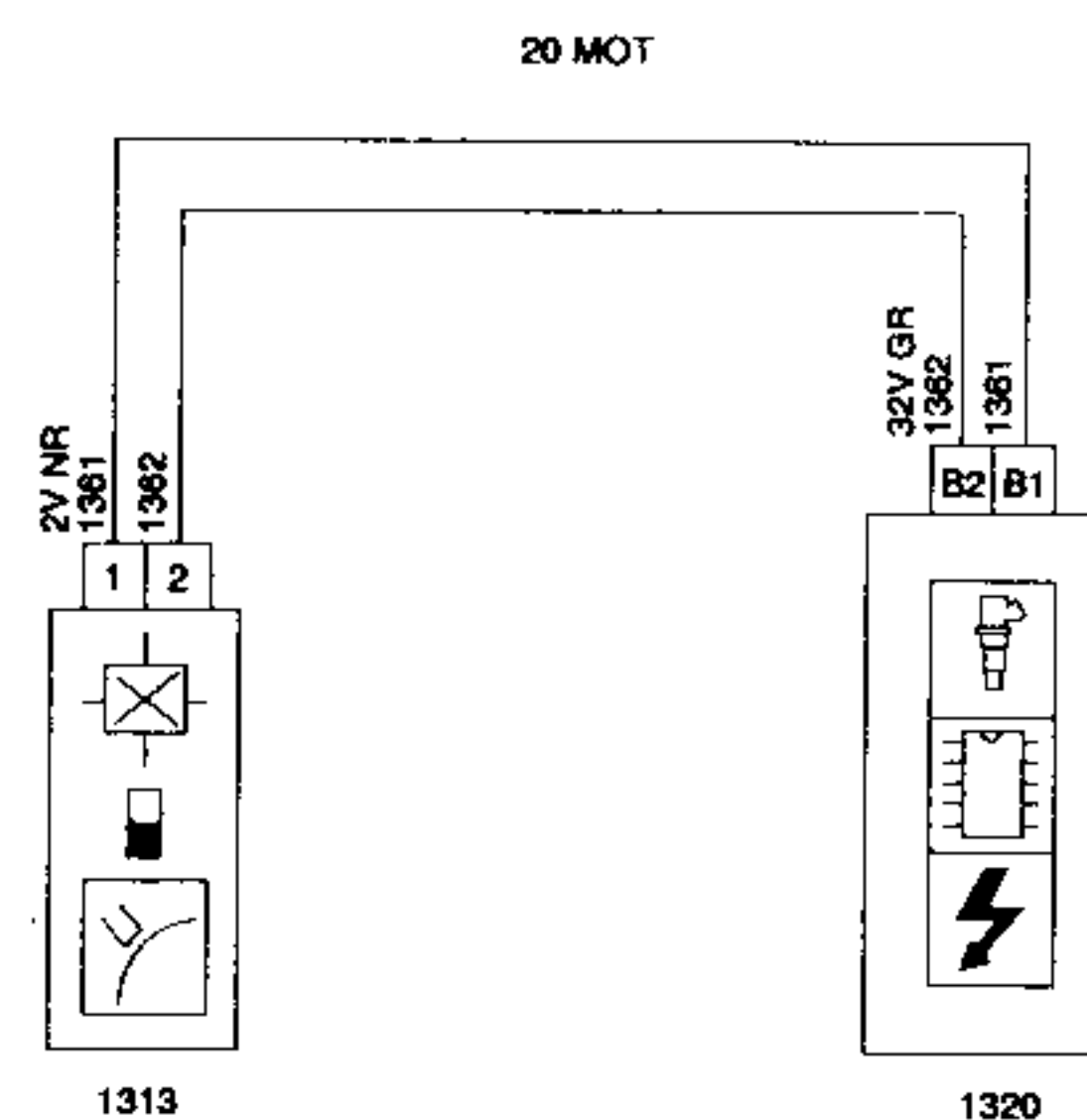
1313 CAPTADOR RÉGIMEN MOTOR (MOTOR TU5JP4 VERSIÓN EUROPA)
