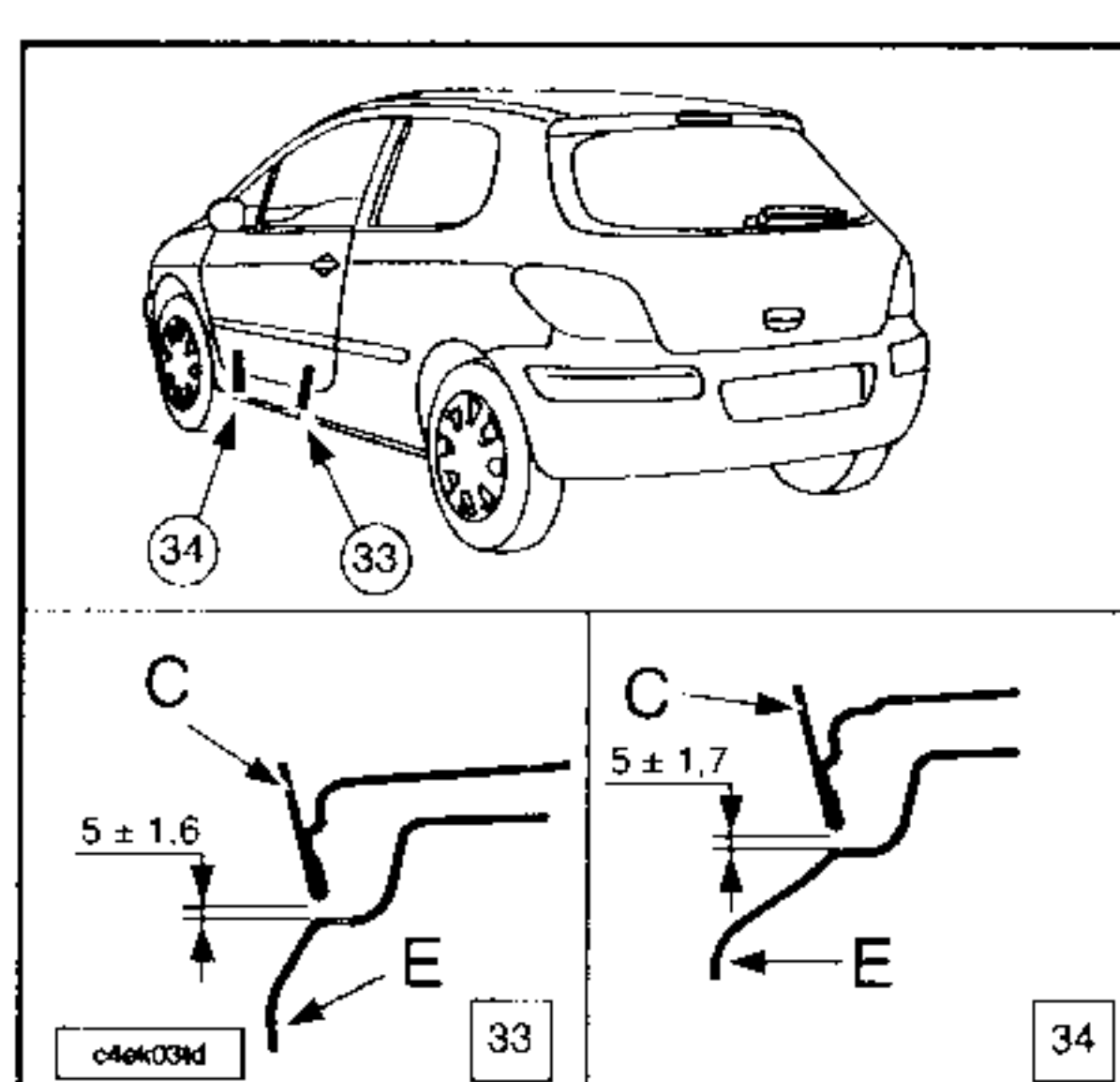
C.-Puerta. E.-Larguero.
