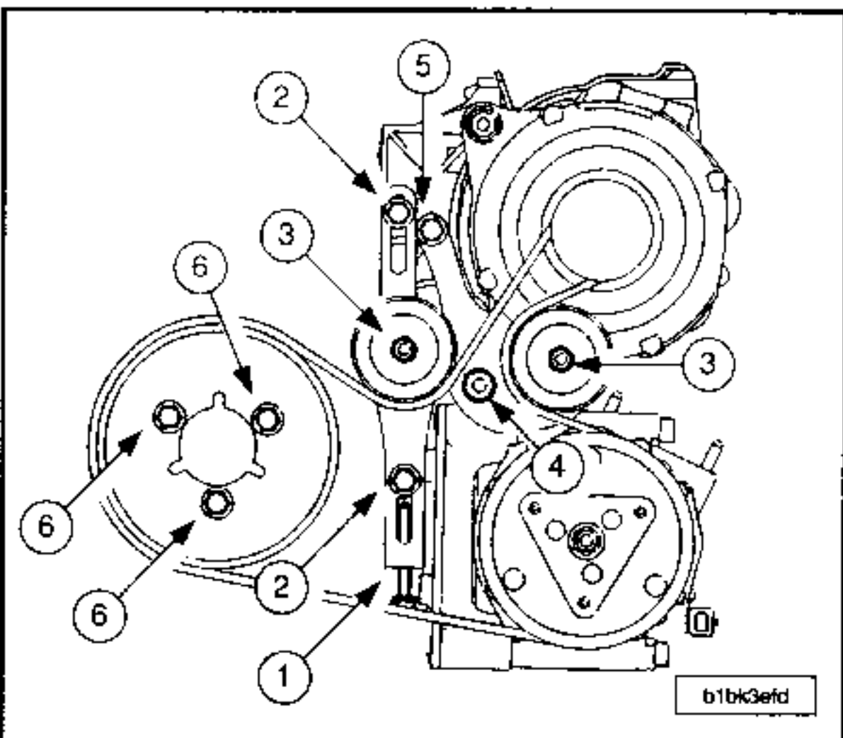
Aire acondicionado, motor TU3JP.
