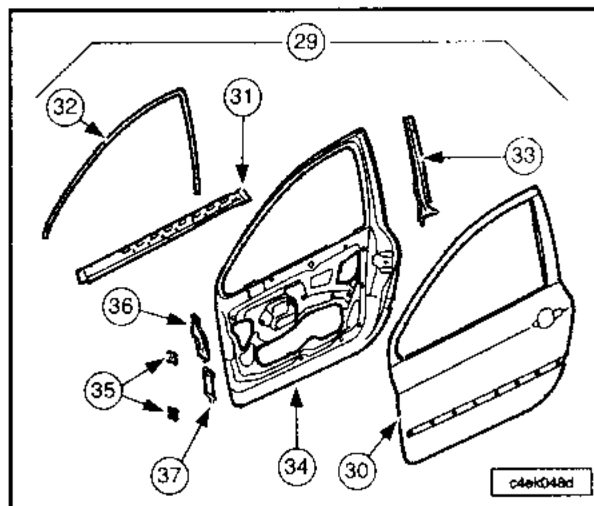
Berlina 3 puertas.
