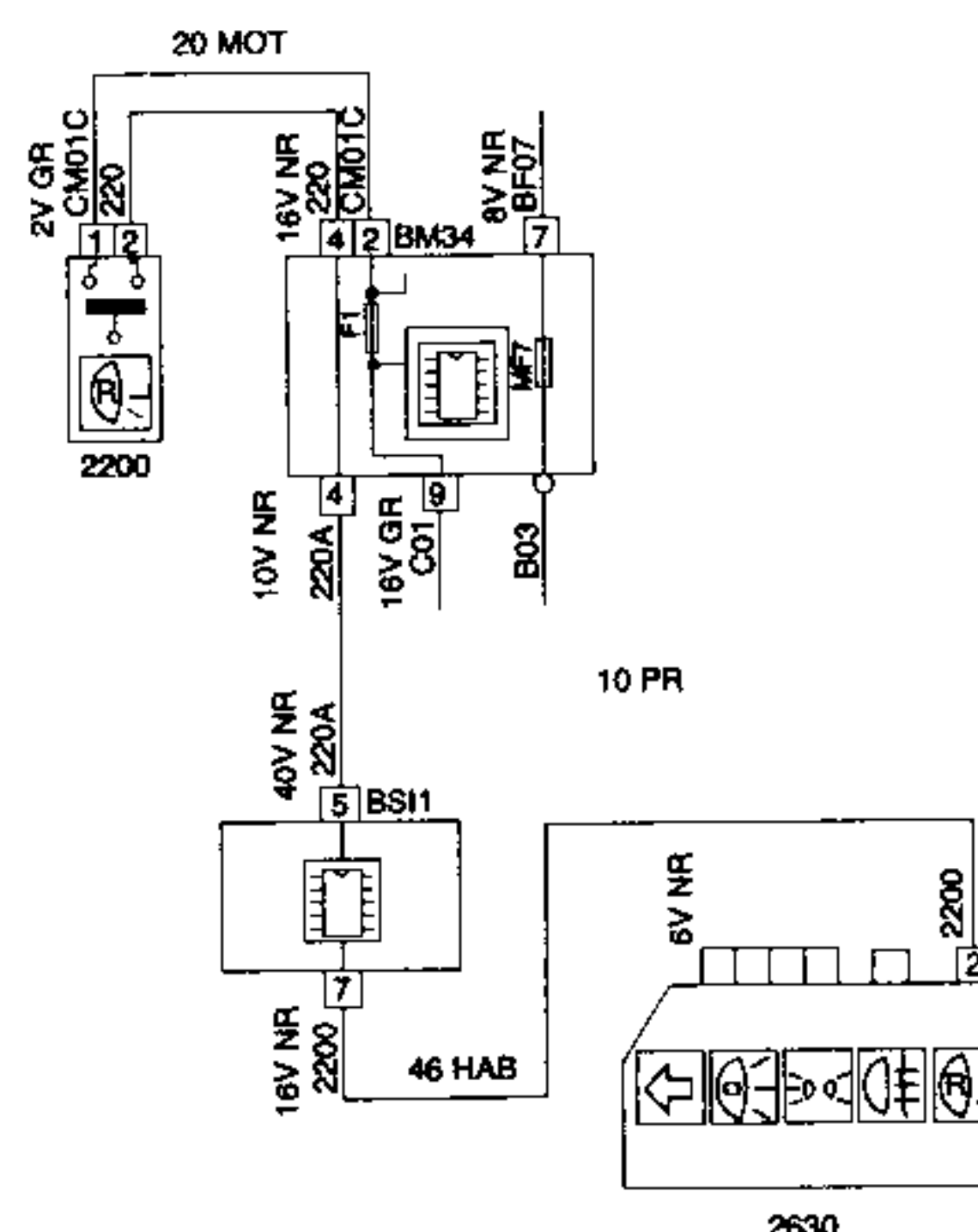
2200 CONTACTOR LUCES DE RETROCESO (MOTOR TU5JP4 VERSIÓN EUROPA)
