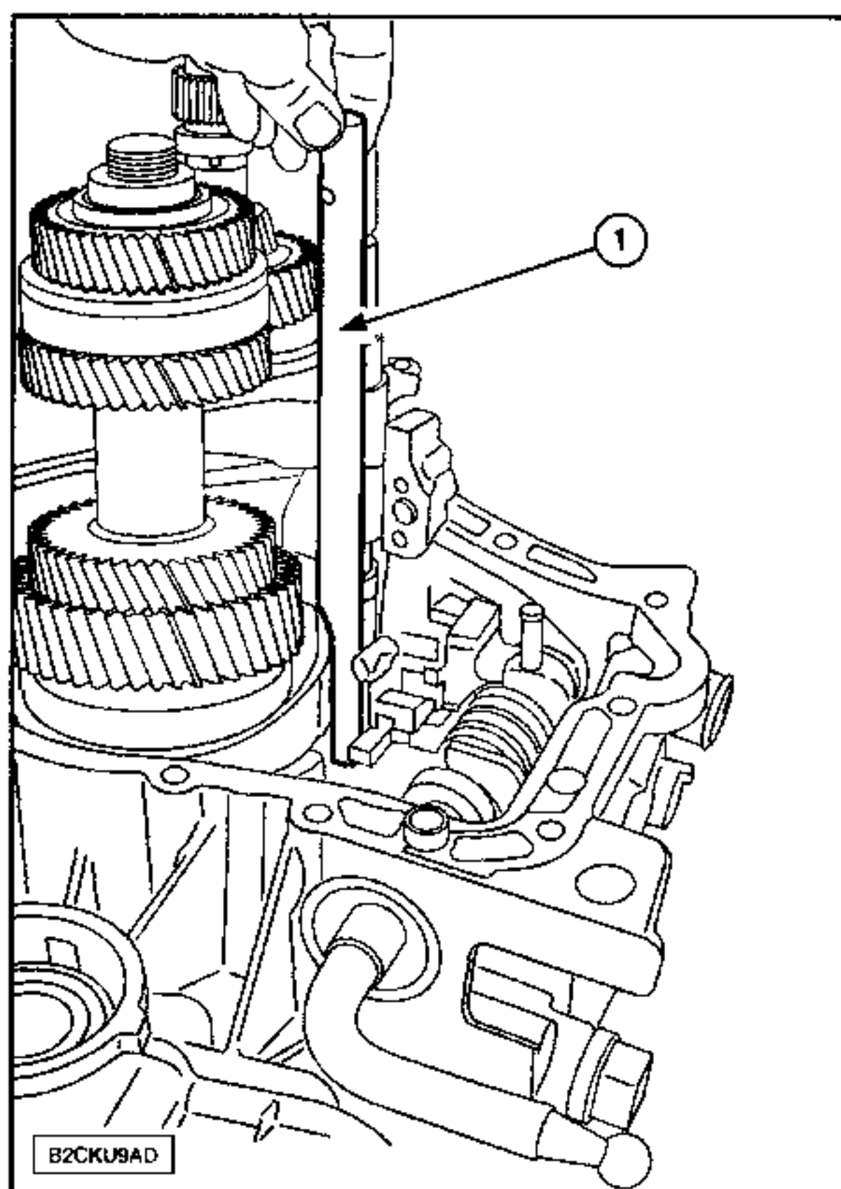
Montar el eje de horquilla de 5ª (1).
