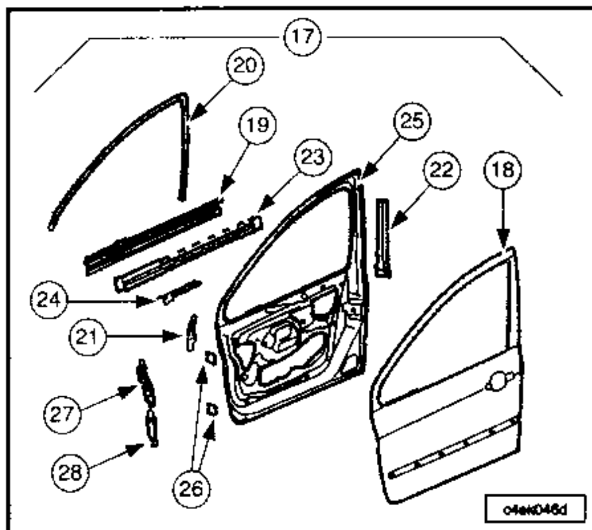
Berlina 5 puertas.
