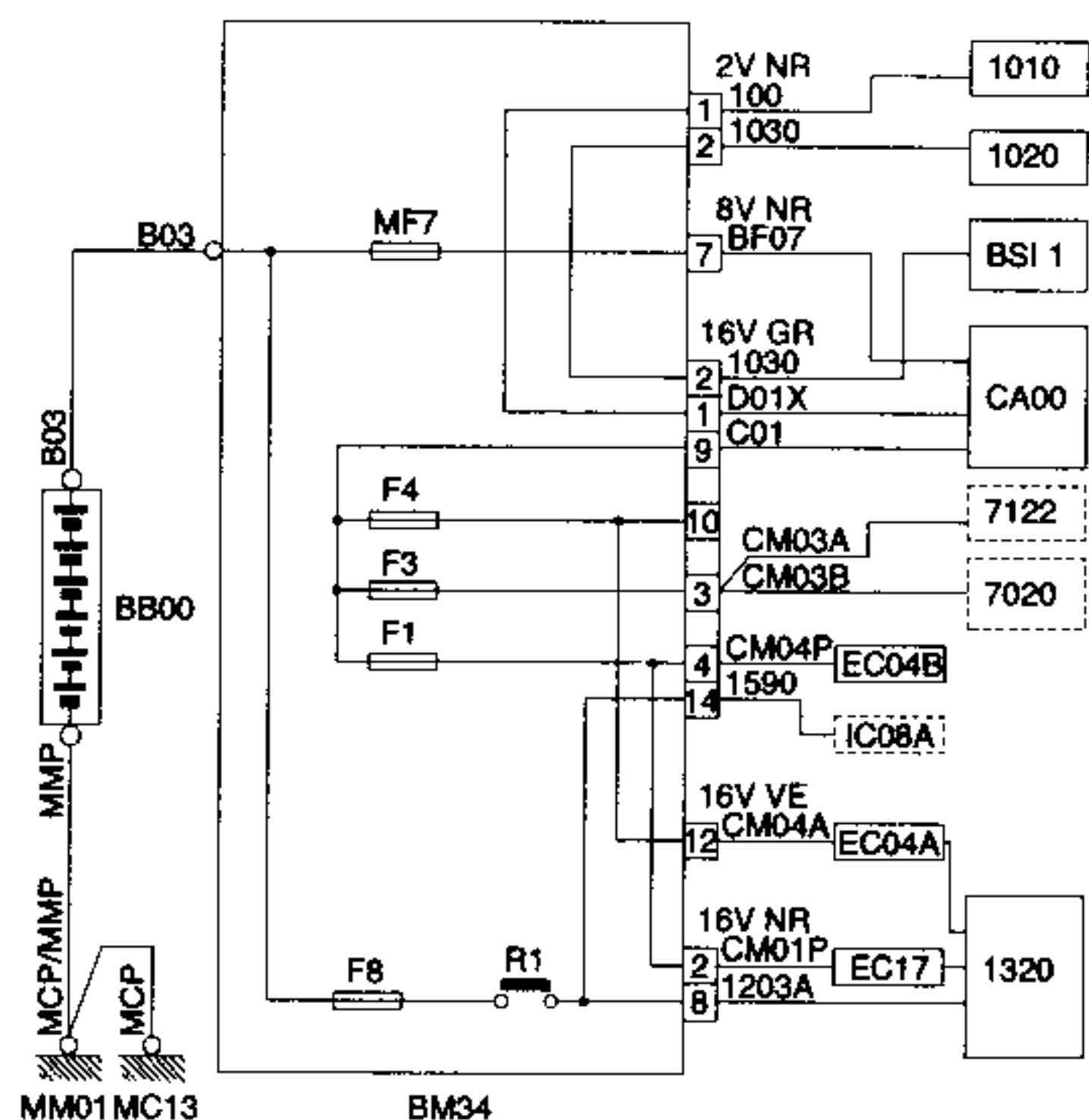
BM34 CAJETÍN DE SERVICIO MOTOR 34 FUSIBLES
