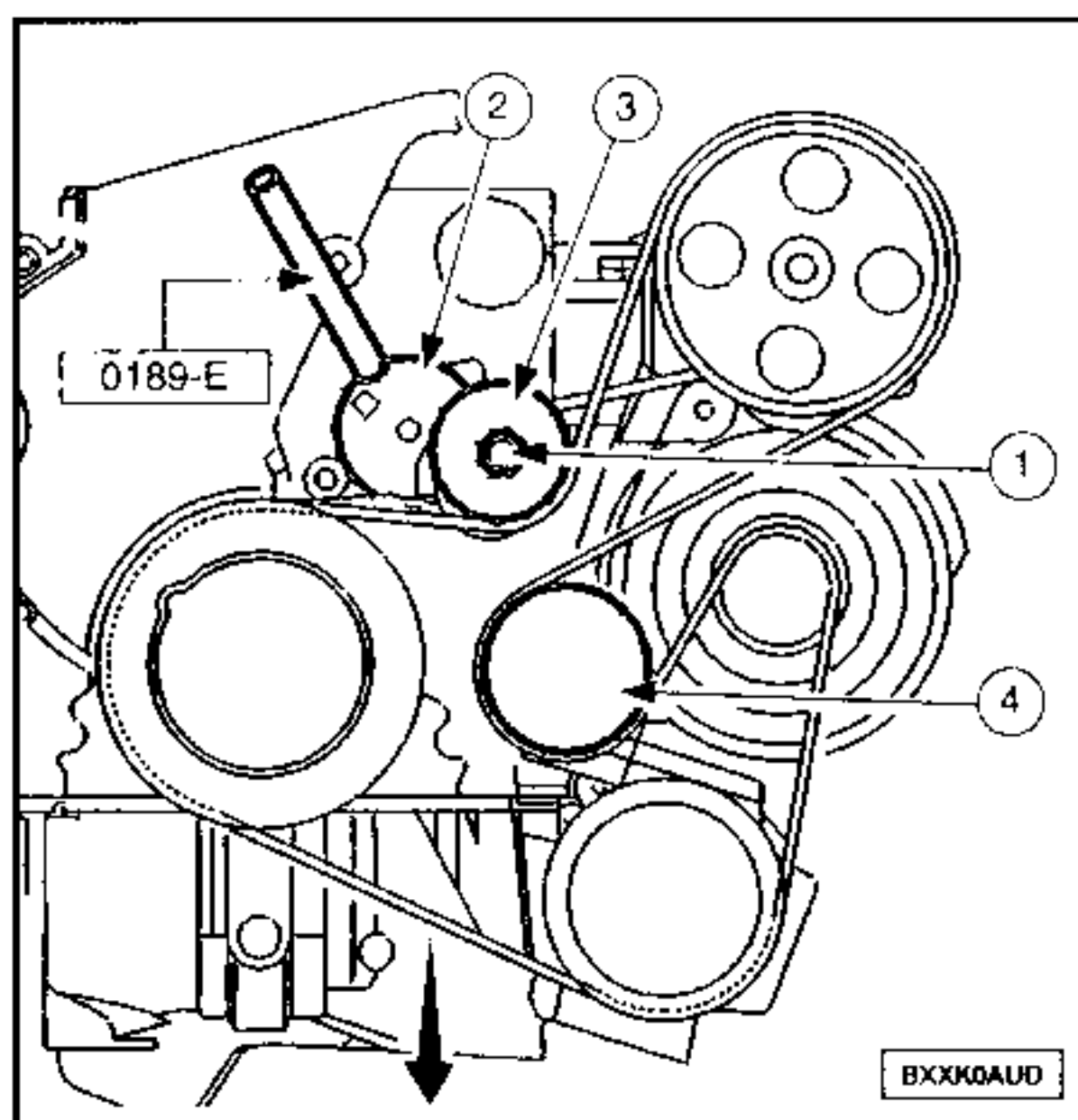
Motor EW10J4 (aire acondicionado).
