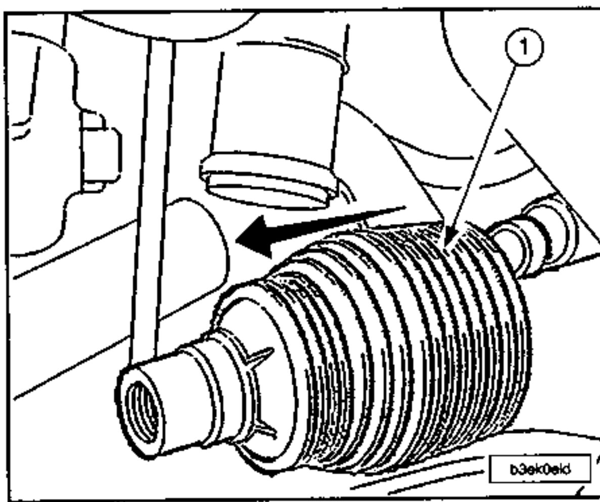
Sacar el guardapolvos de estanqueidad (1).
