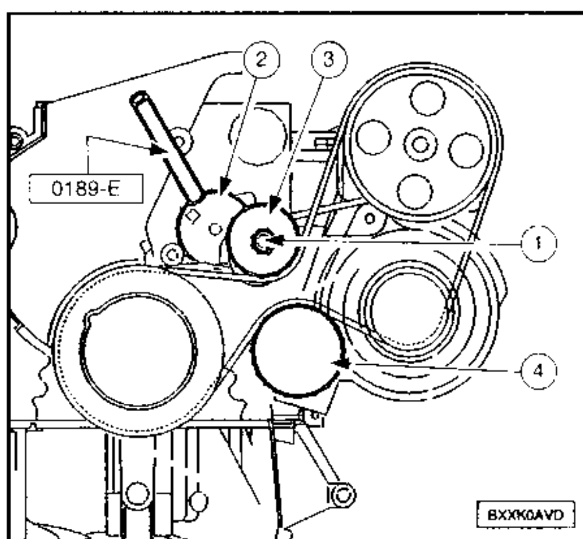
Motor EW10J4.
