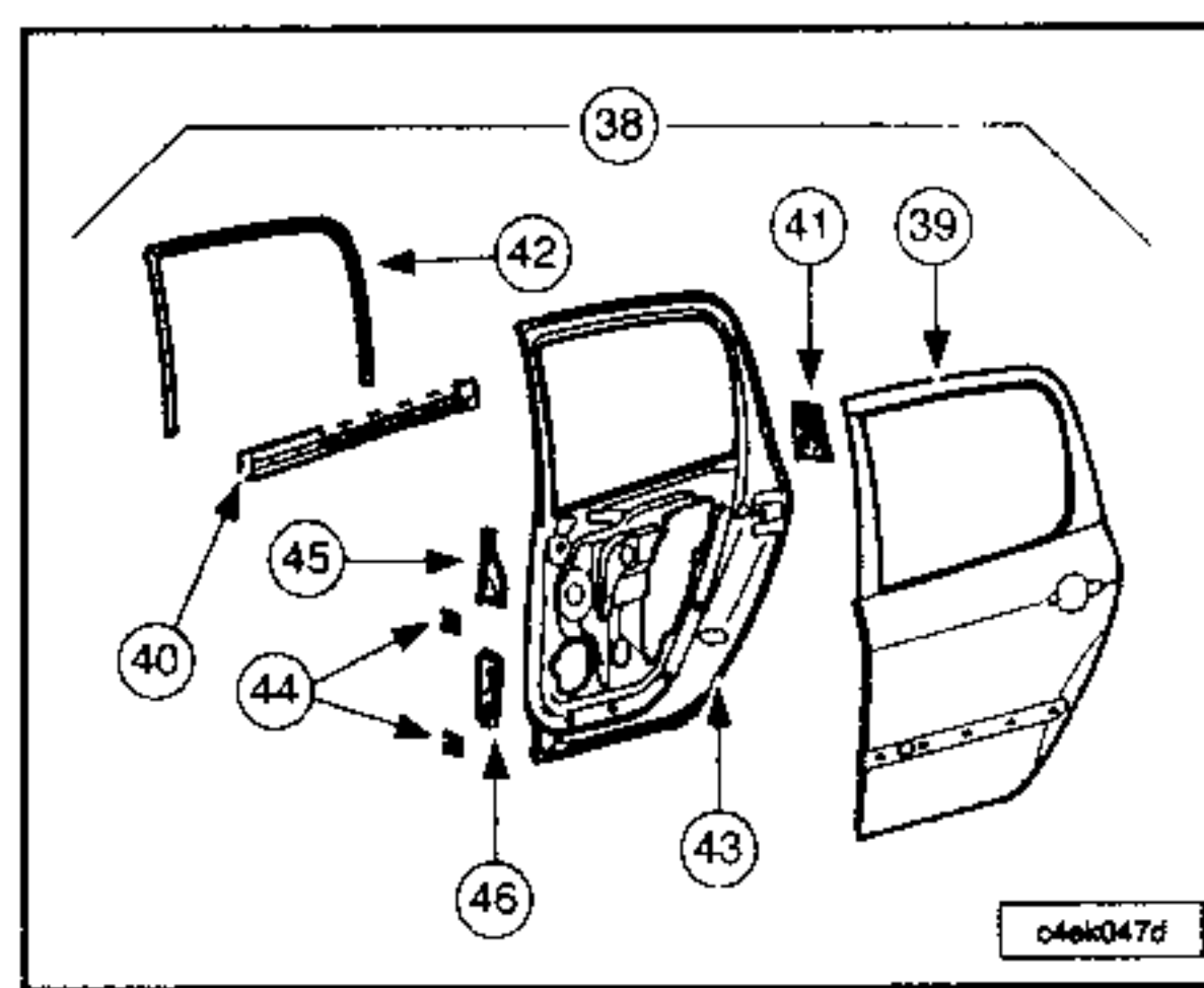
Berlina 5 puertas.
