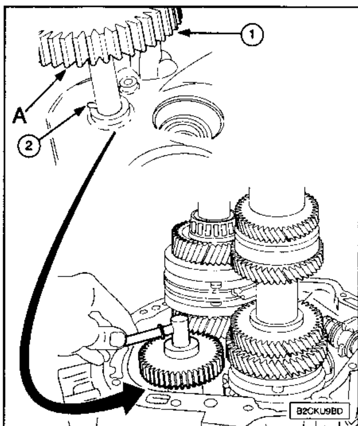
Montar el eje y el piñón de marcha atrás (1), entrada del dentado (A) hacia abajo.
