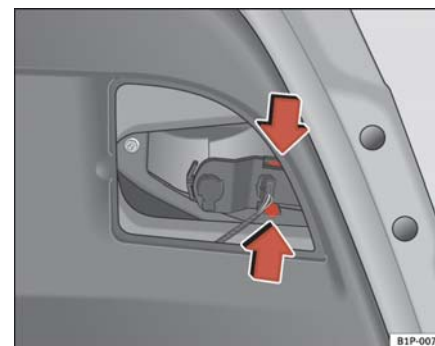
Fig. 165 Desmontaje del portalámparas
