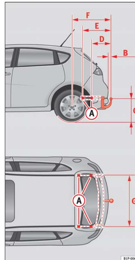
Fig. 132 Puntos de fijación del dispositivo de remolque
