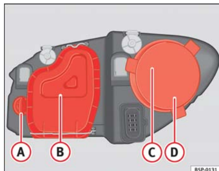
Fig. 155 Lámparas del faro principal
