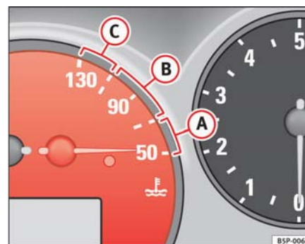
Fig. 34 Cuadro de instrumentos: indicador de la temperatura del líquido refrigerante del motor
