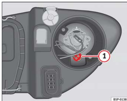
Fig. 162 Luz de población
