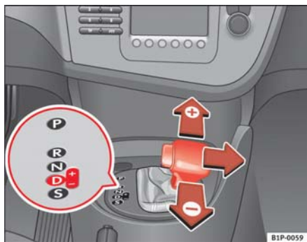
Fig. 121 Cambiar con tiptronic
