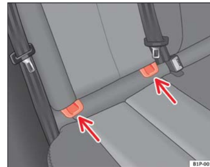
Fig. 30 Argollas de sujeción ISOFIX
