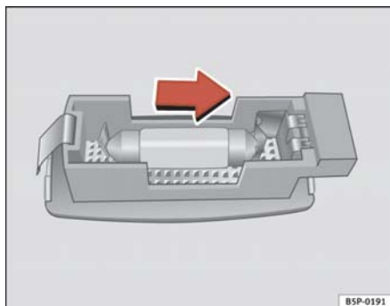
Fig. 172 Desmontaje luz del parasol
