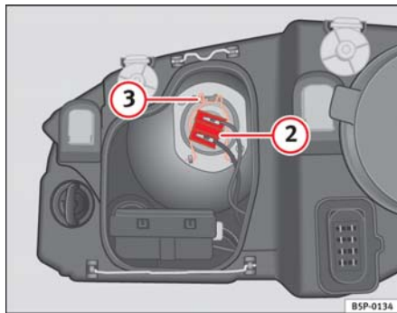
Fig. 158 Luz de cruce
