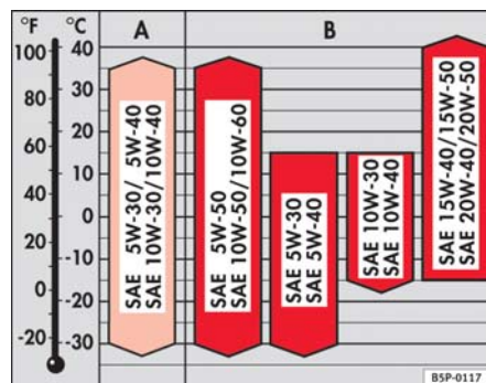
Fig. 136 Tipos de aceite de acuerdo a la temperatura
