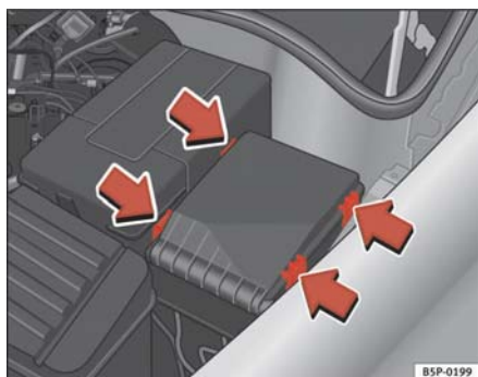
Fig. 154 Tapa de la caja de fusibles en el compartimento motor
