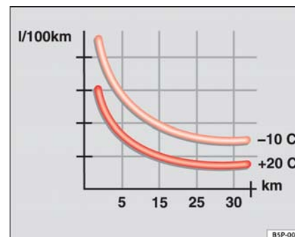
Fig. 131 Consumo de combustible (l/100 km) a dos temperaturas ambiente
