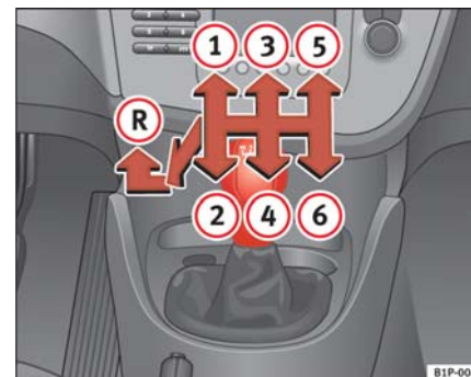
Fig. 116 Detalle de la consola central: esquema de un cambio manual de 6 marchas
