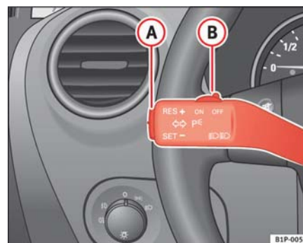
Fig. 126 Palanca de intermitentes y de luz de carretera: mando y tecla basculante para el regulador de velocidad
