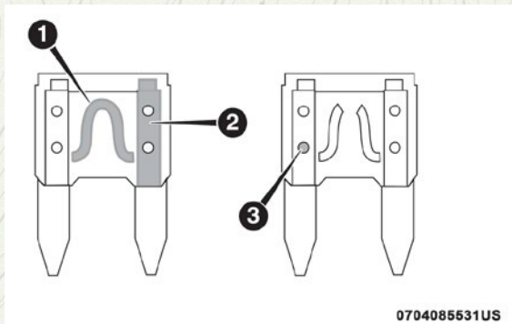
Hoja del fusible
