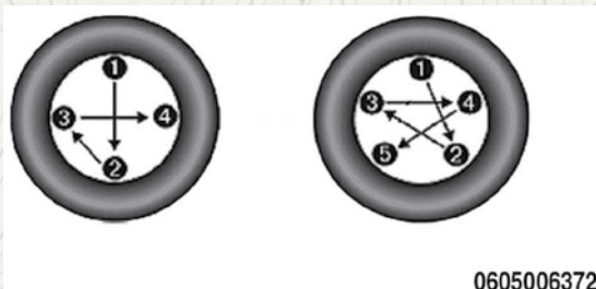
Patrón de apriete
