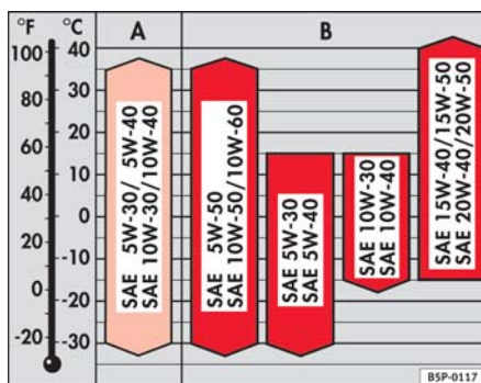
Fig. 143 Tipos de aceite de acuerdo a la temperatura
