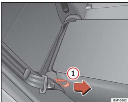
Fig. 89 Abatir o levantar el respaldo de los asientos posteriores
