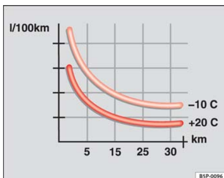
Fig. 138 Consumo de combustible (l/100 km) a dos temperaturas ambiente
