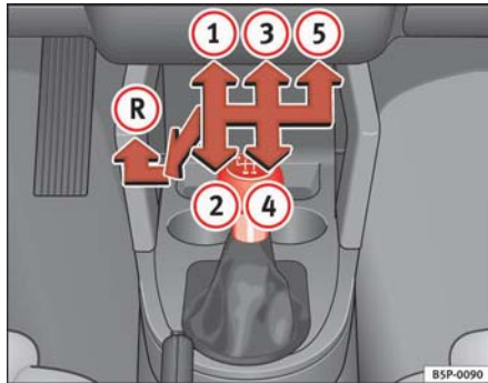
Fig. 122 Detalle de la consola central: esquema de un cambio manual de 5 marchas
