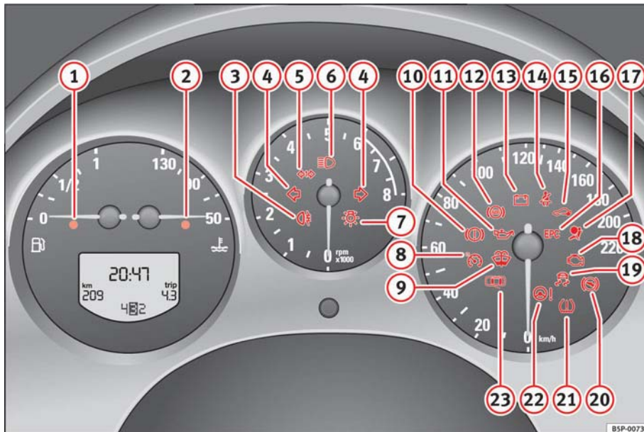
Fig. 43 Testigos de control y de advertencia del cuadro de instrumentos. Algunos de estos testigos pertenecen sólo a determinadas versiones del modelo o forman parte de equipamientos opcionales. ►
