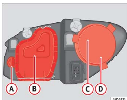
Fig. 165 Lámparas del faro principal
