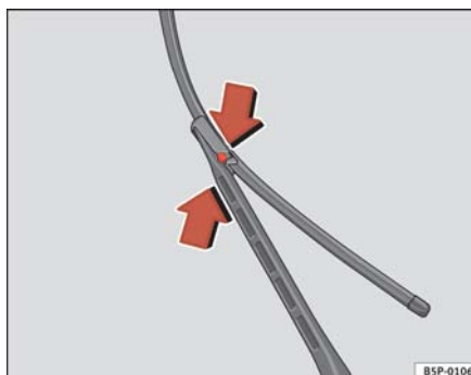
Fig. 149 Cambio de las escobillas del limpiaparabrisas
