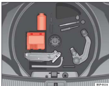
Fig. 156 Juego para reparación de neumáticos (Tyre Mobility System)
