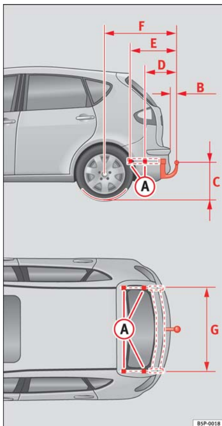
Fig. 139 Puntos de fijación del dispositivo de remolque
