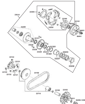
E-08: CLUTCH CENTRÍFUGO
