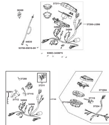
F-03: VELOCÍMETRO (RS-NAKED-DIGITAL)
