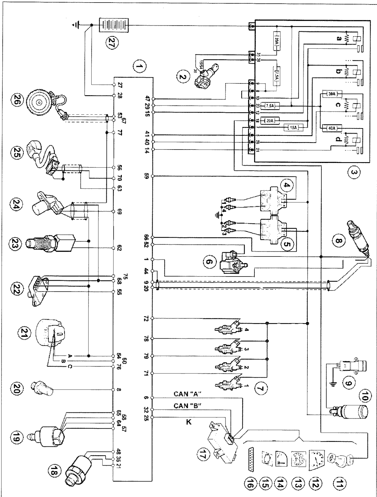
EQUIMA ELECTRICO SISTEMA INYECCION -ENCENDIDO
