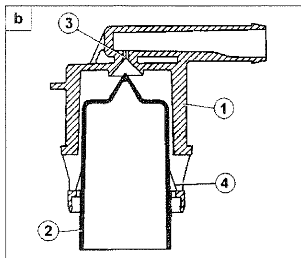
Secciones de la válvula fluctuante en las posiciones de trabajo a, b e c
