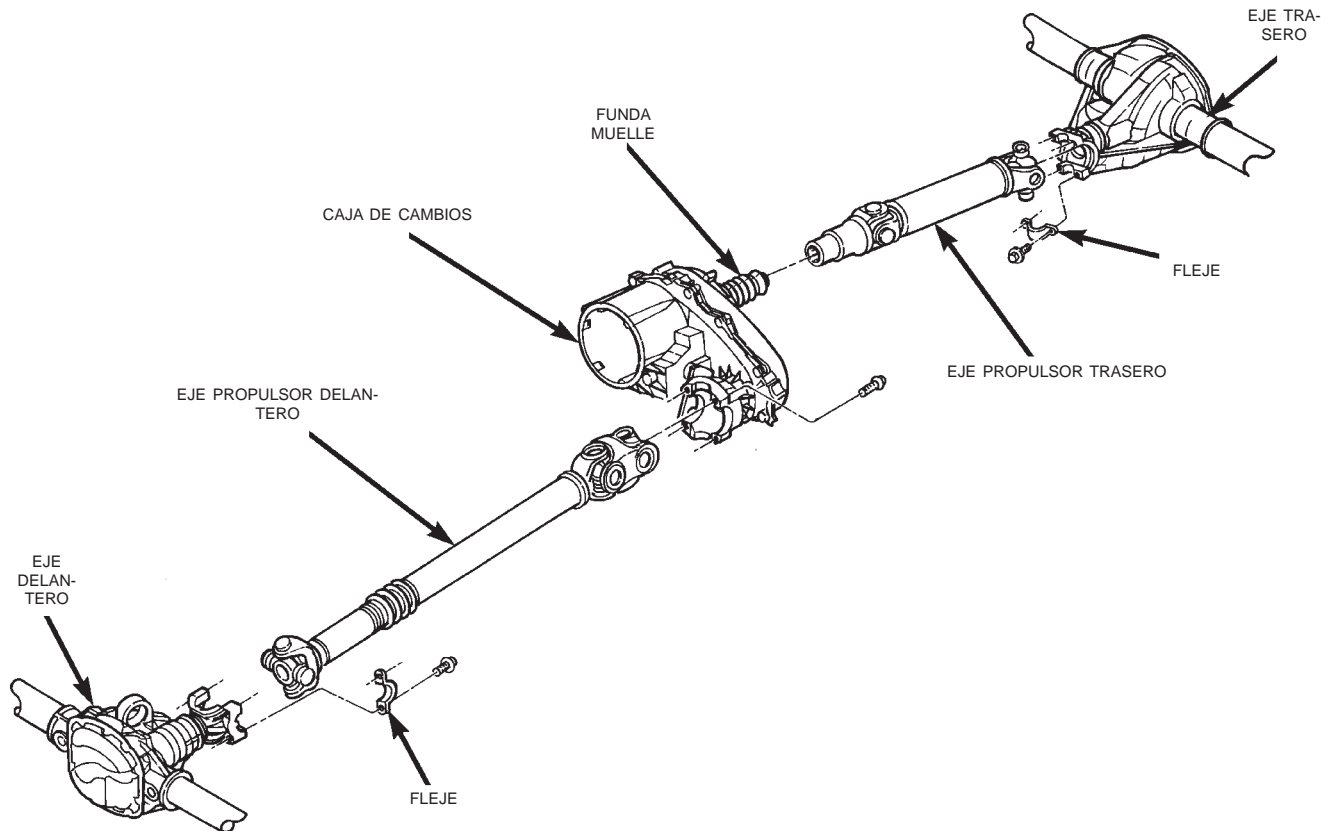
Fig. 1 Ejes propulsores delantero y trasero—4WD
