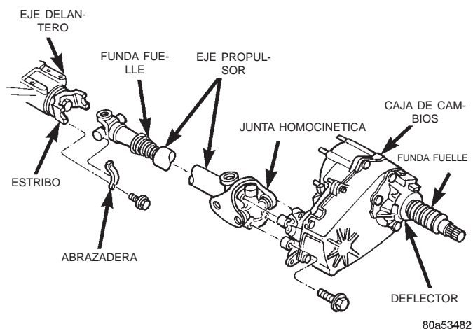
Fig. 12 Eje propulsor delantero
