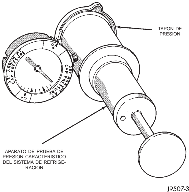
Fig. 14 Prueba a presión del tapón de presión del radiador—Característico
