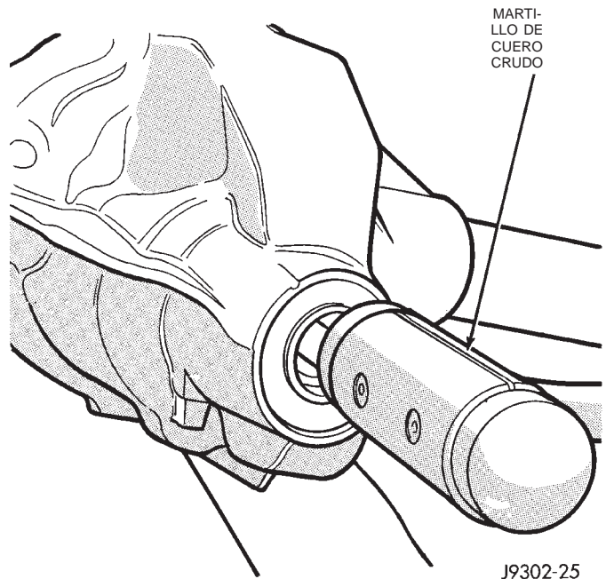
Fig. 35 Desmontaje del piñón satélite
