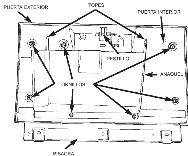
Fig. 18 Desmontaje e instalación de los componentes de la guantera
