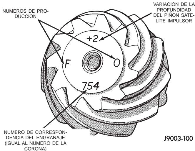
Fig. 51 Números de identificación del piñón satélite
