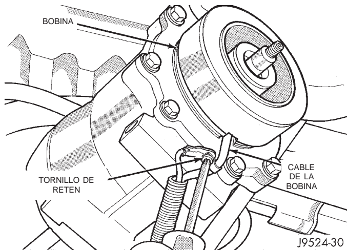
Fig. 28 Mazo de cables conductores de la bobina del embrague
