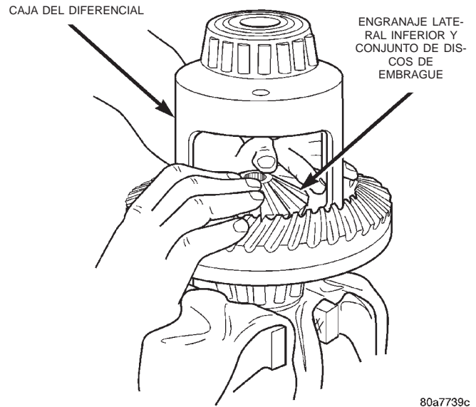
Fig. 49 Instalación de discos de embrague y engranaje lateral inferior
