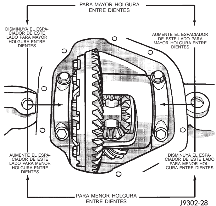
Fig. 78 Ajuste de espaciador de holgura entre dientes
