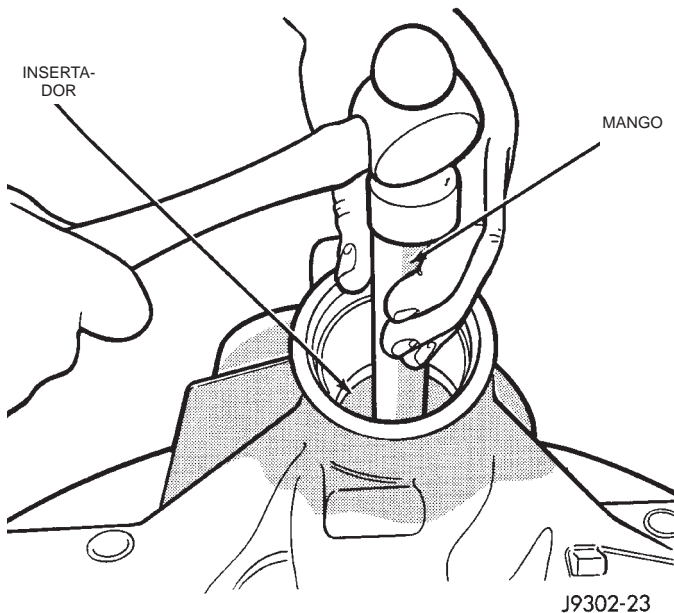
Fig. 31 Desmontaje de la cubeta del cojinete trasero
