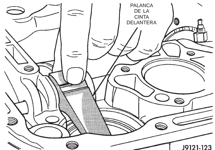
Fig. 92 Palanca de la cinta delantera
