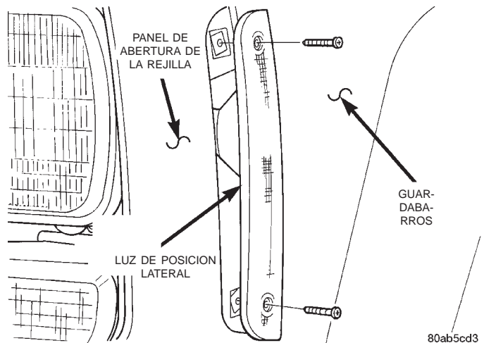
Fig. 5 Luz de posición lateral
