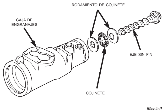
Fig. 21 Eje sin fin
