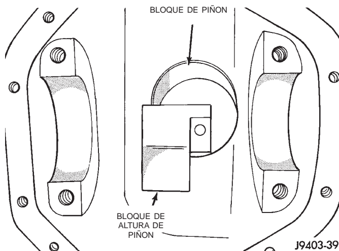
Fig. 47 Bloque de altura de piñón—Característico
