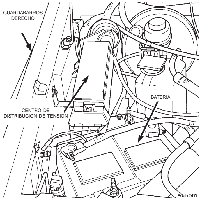
Fig. 9 Centro de distribución de tensión (PDC)
