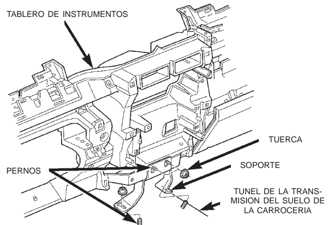
Fig. 22 Desmontaje e instalación del soporte de apoyo central del tablero de instrumentos
