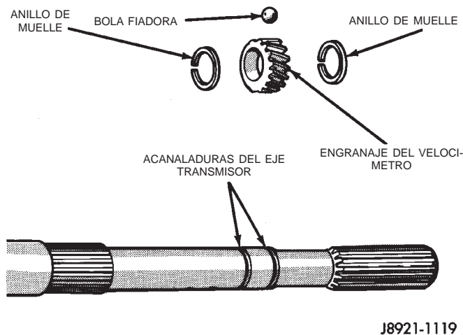
Fig. 40 Conjunto de engranaje propulsor del velocímetro
