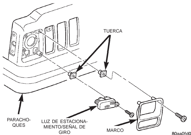
Fig. 4 Luz de estacionamiento/señal de giro
