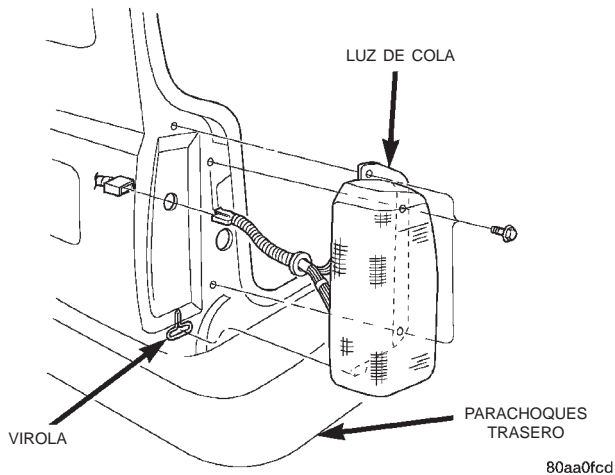
Fig. 6 Luz de cola
