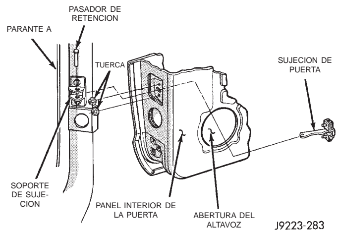
Fig. 28 Sujeción de la puerta (tope de retención)
