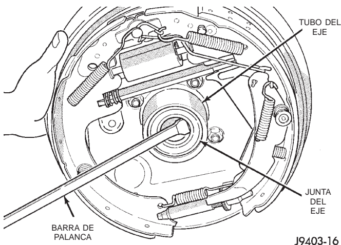
Fig. 10 Desmontaje de junta del eje
