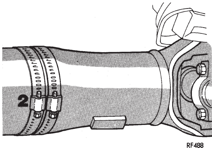
Fig. 6 Dos tornillos de abrazadera en la misma posición
