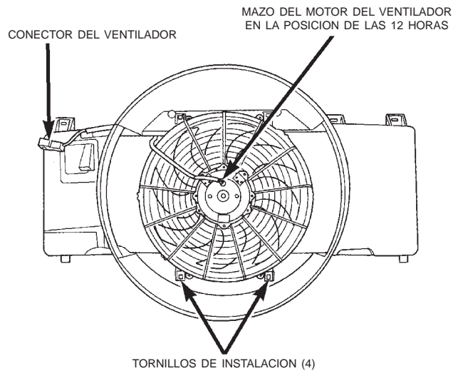
Fig. 37 Orientación e instalación del módulo del ventilador
