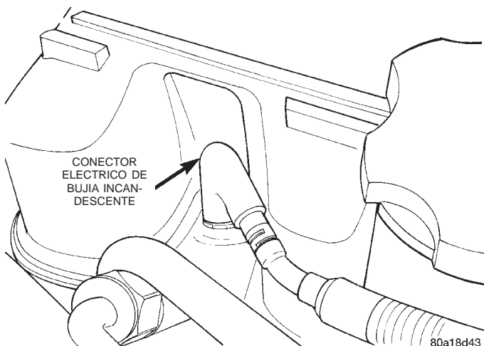
Fig. 23 Conector eléctrico de bujía incandescente
