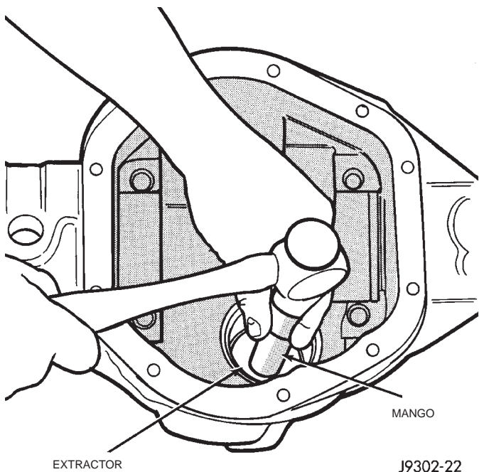
Fig. 30 Desmontaje de la cubeta del cojinete delantero
