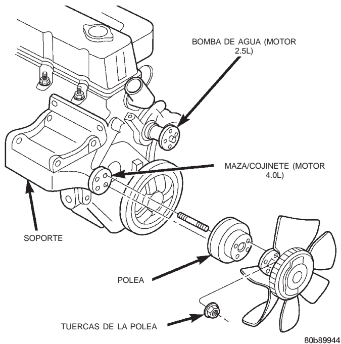
Fig. 50 Ventilador de refrigeración instalado en el soporte
