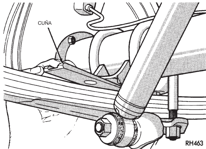
Fig. 36 Ajuste del ángulo en los muelles de láminas
