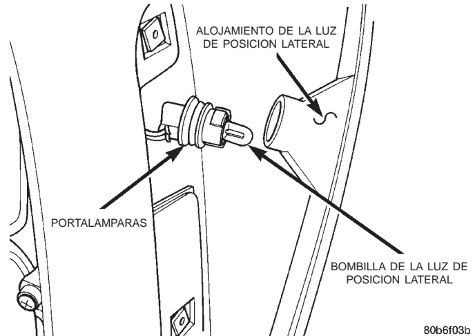
Fig. 4 Luz de posición lateral
