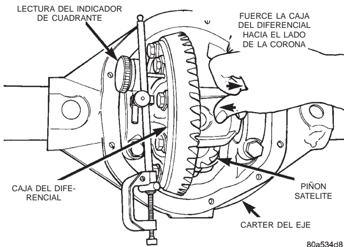
Fig. 58 Sujeción de caja del diferencial y lectura del indicador de cuadrante
