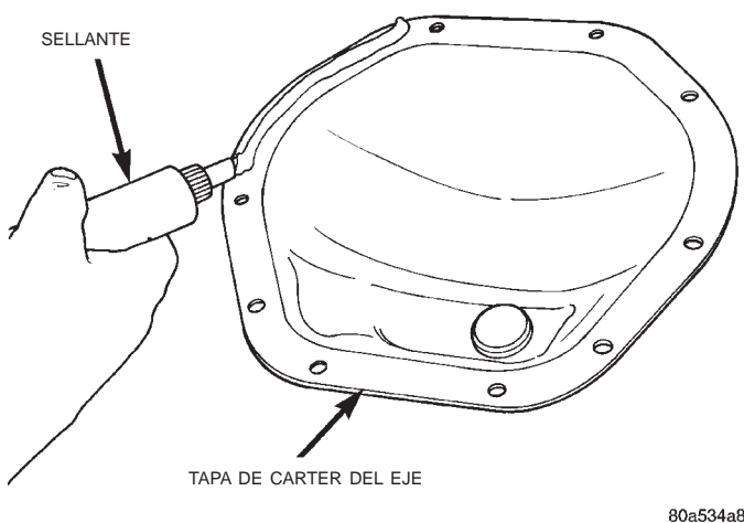
Fig. 7 Aplicación de sellante
