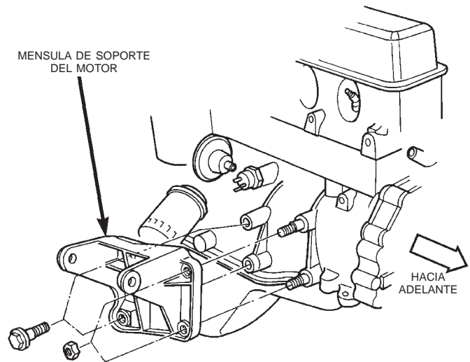
Fig. 23 Ménsula de soporte del motor—Lado derecho
