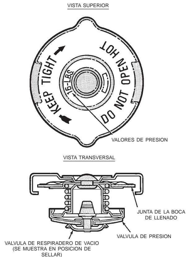
Fig. 4 Tapón y boca de llenado de presión del radiador—Característico
