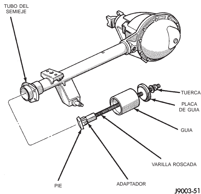
Fig. 11 Extractor de cojinetes del semieje
