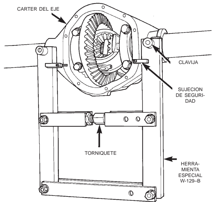
Fig. 17 Instalación del separador del cárter del diferencial
