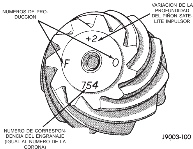
Fig. 44 Números de identificación del piñón satélite
