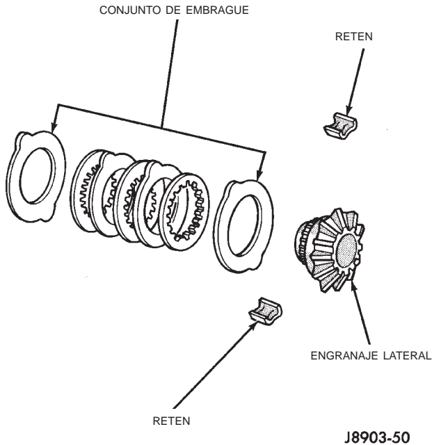
Fig. 48 Conjunto de discos de embrague
