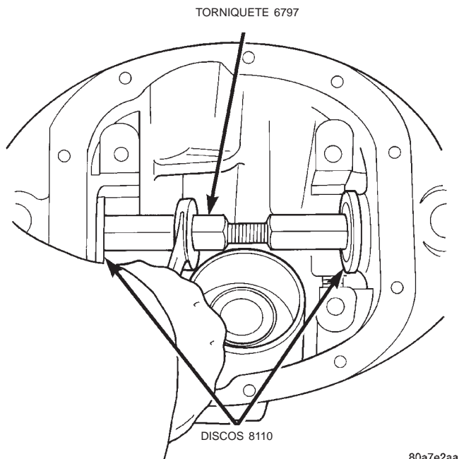
Fig. 25 Instalación de junta de aceite
