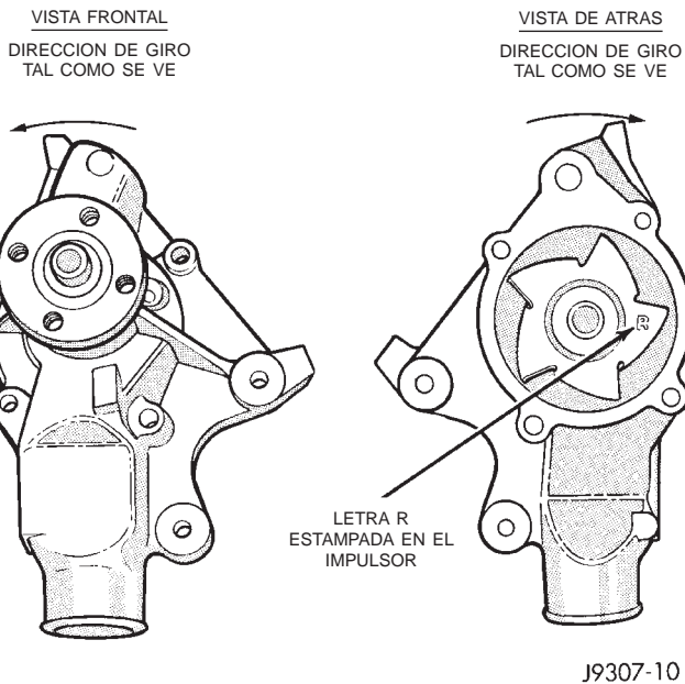
Fig. 5 Bomba de agua de giro inverso—Característico
