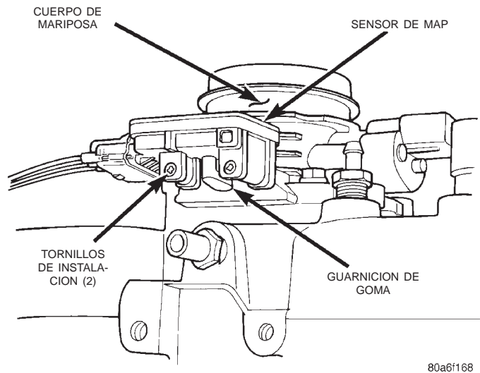
Fig. 49 Instalación del sensor de MAP
