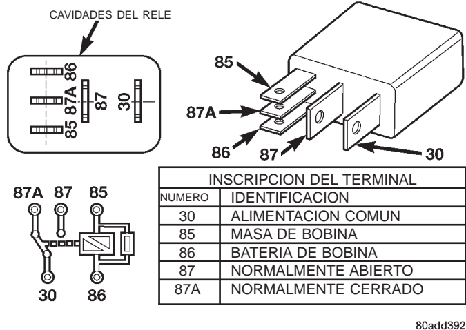
Fig. 11 Relé tipo 2
