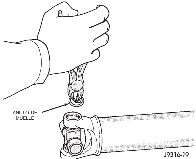
Fig. 17 Desmontaje de anillo de muelle
