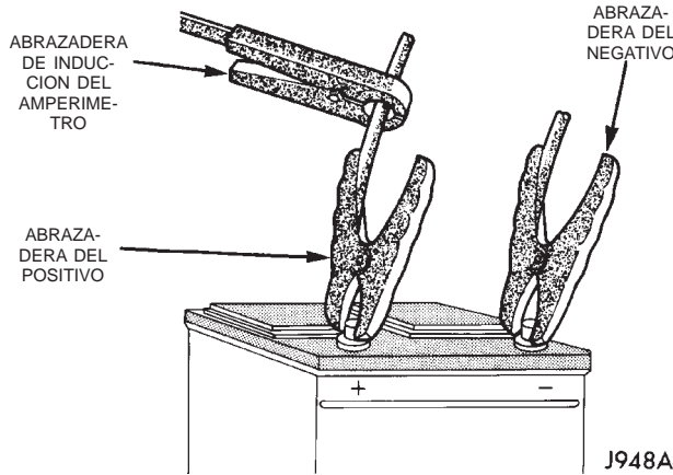
Fig. 7 Conexiones del probador de carga Voltímetro y amperímetro - Características
