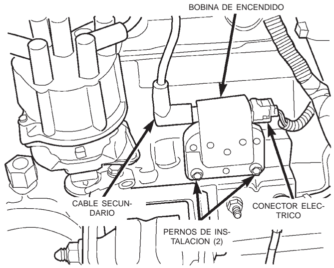
Fig. 7 Bobina de encendido—Motor 4.0L
