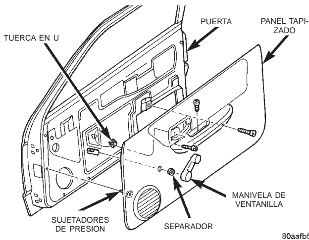
Fig. 7 Desmontaje e instalación del panel tapizado de la puerta delantera - Ventanilla manual
