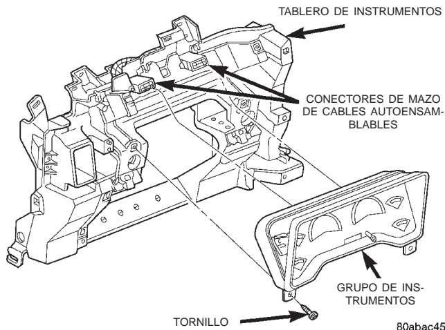
Fig. 12 Desmontaje e instalación del grupo de instrumentos
