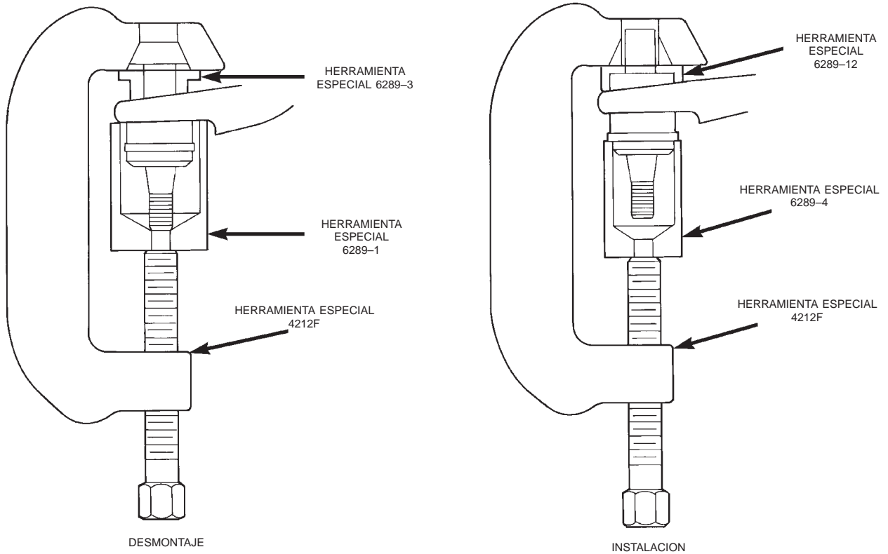
Fig. 15 Desmontaje e instalación del perno de rótula inferior
