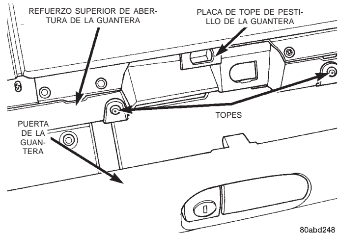
Fig. 16 Desmontaje e instalación de topos de la guantera
