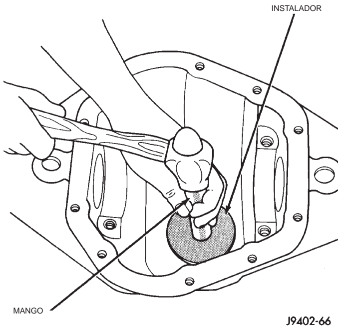
Fig. 40 Instalación de la cubeta del cojinete trasero del piñón
