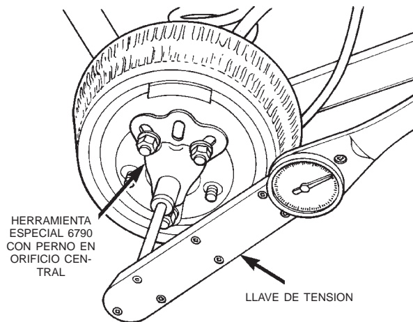
Fig. 6 Prueba del Trac-LoK™—Característica
