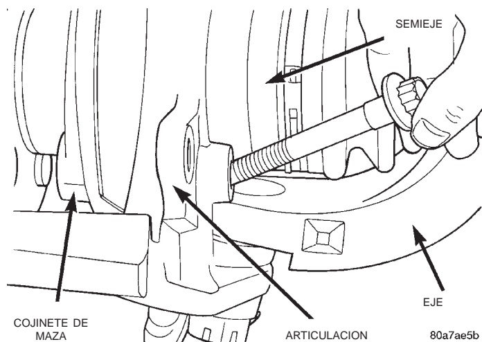
Fig. 11 Pernos del cojinete de maza
