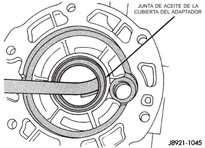
Fig. 14 Desmontaje de la junta de la cubierta del adaptador
