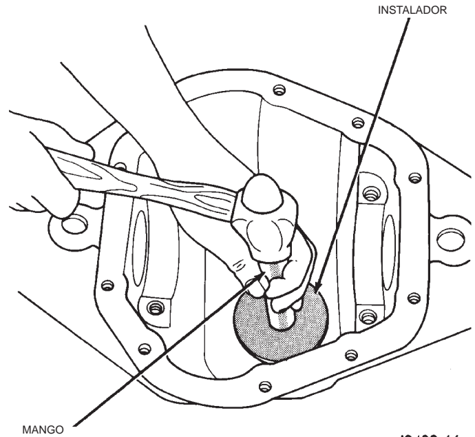
Fig. 30 Instalación de la cubeta del cojinete trasero del piñón
