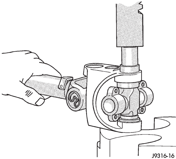
Fig. 33 Colocación de tapa de cojinete
