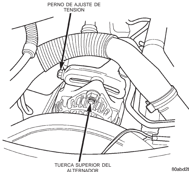
Fig. 48 Soporte de ajuste de tensión de la correa del generador
