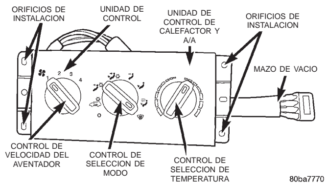
Fig. 37 Desmontaje e instalación del calefactor y A/A
