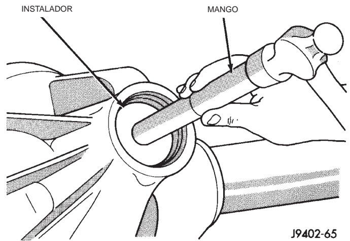
Fig. 31 Instalación de la cubeta del cojinete delantero del piñón
