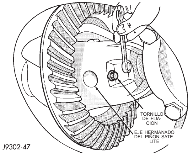
Fig. 40 Tornillo de fijación del eje hermano
