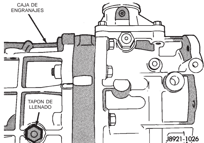
Fig. 4 Localización del tapón del orificio de llenado
