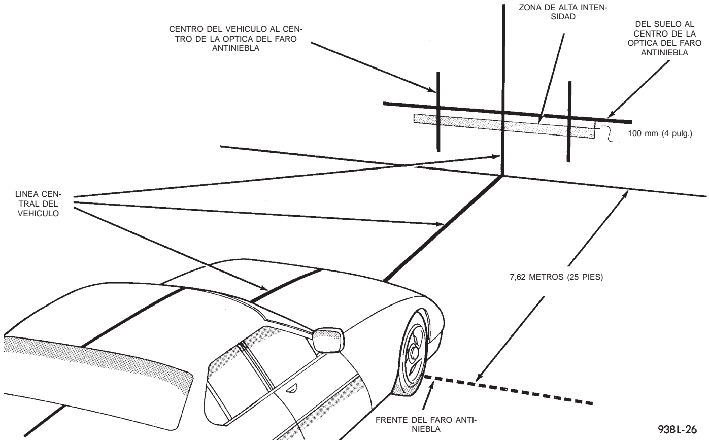
Fig. 4 Alineación de faro antiniebla — Característica
