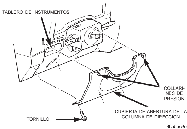
Fig. 4 Desmontaje e instalación de cubierta de abertura de la columna de dirección
