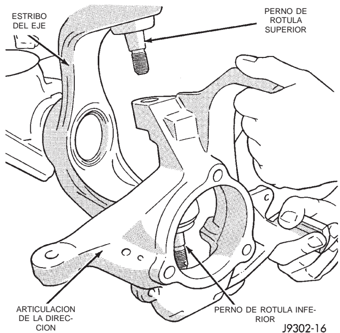
Fig. 13 Desmontaje e instalación de la articulación de dirección
