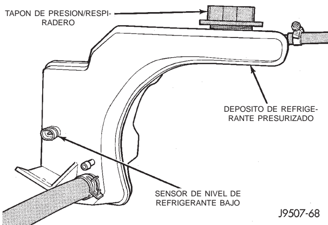
Fig. 13 Depósito de refrigerante y tapón de presión/respiradero
