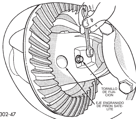
Fig. 49 Tornillo de fijación de eje engranado del piñón satélite
