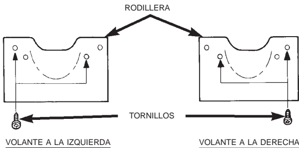
Fig. 6 Localización de los tornillos de instalación de la rodillera 80abac42
