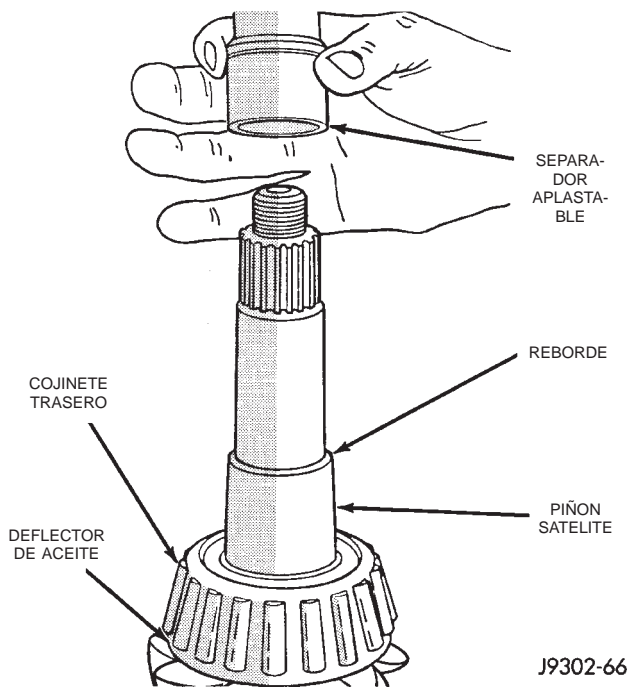
Fig. 44 Separador de ajuste previo aplastable
