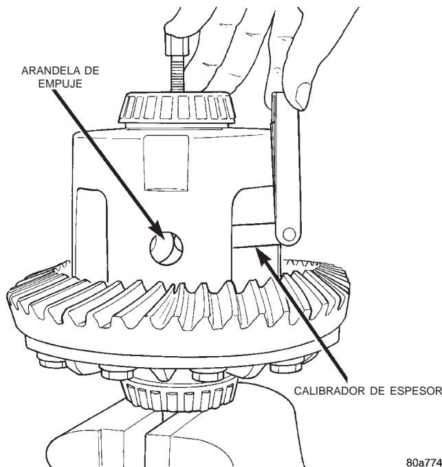
Fig. 58 Desmontaje de arandela de empuje de piñón satélite
