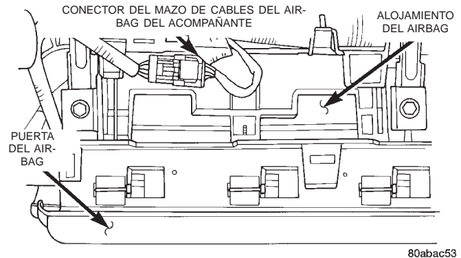
Fig. 9 Conector del módulo del airbag del lado del acompañante
