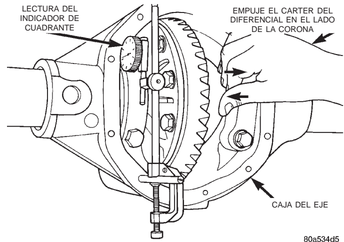
Fig. 76 Sujeción del cárter del diferencial y lectura del indicador de cuadrante
