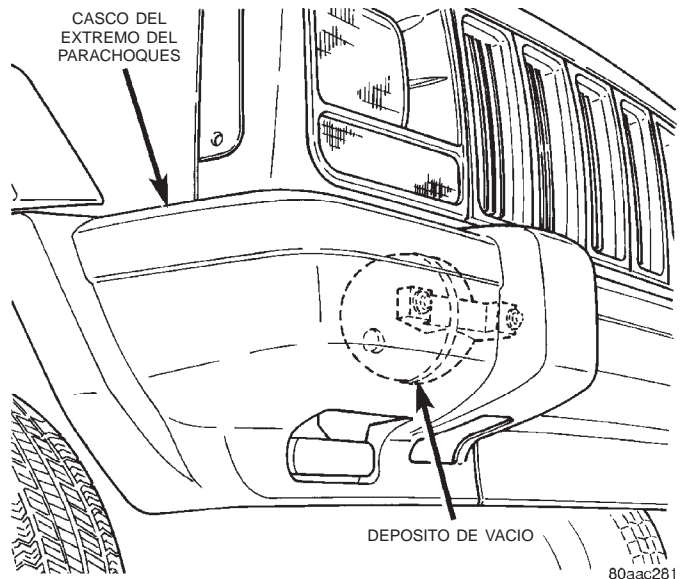
Fig. 6 Localización del depósito de vacío
