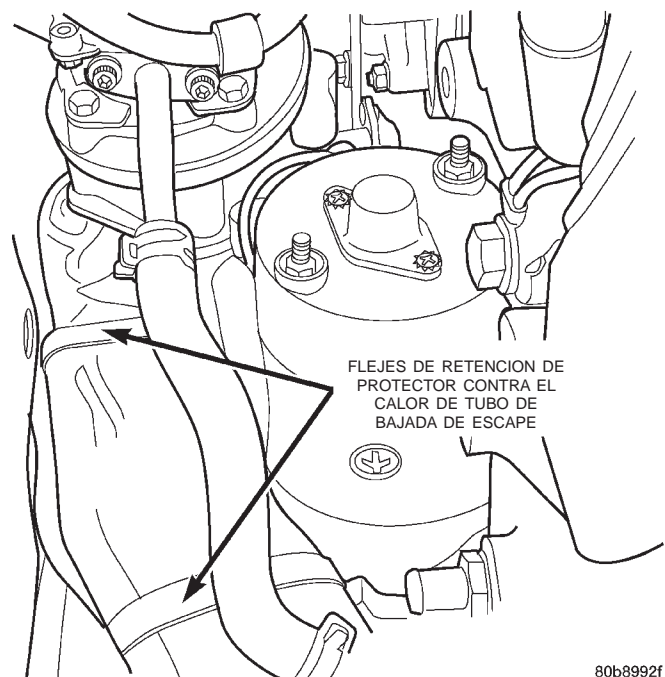
Fig. 6 Protector contra el calor del tubo de bajada de escape
