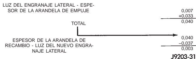
Fig. 61 Cálculos del engranaje lateral
