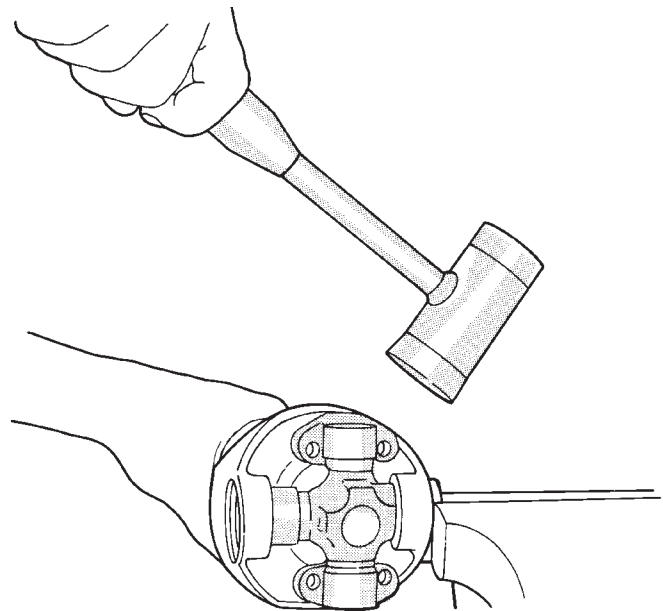
Fig. 23 Extracción del cojinete
