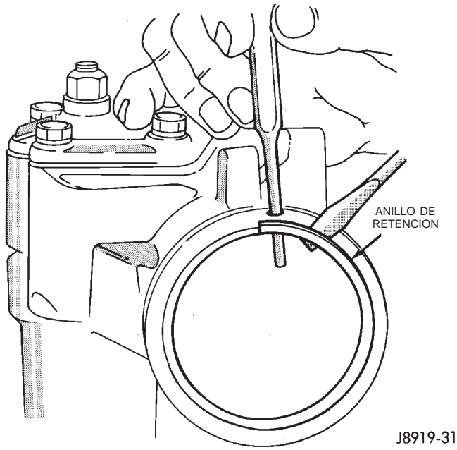
Fig. 3 Anillo de retención del tapón de cierre
