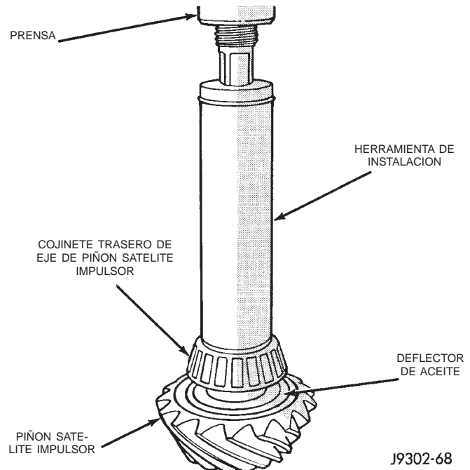
Fig. 36 Instalación de cojinete trasero del piñón
