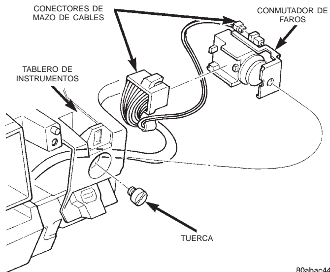
Fig. 11 Desmontaje e instalación del conmutador de faros
