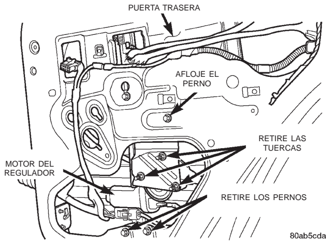
Fig. 59 Ventanilla de la puerta trasera
