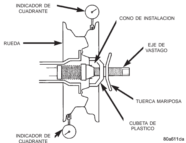
Fig. 3 Descentramiento radial
