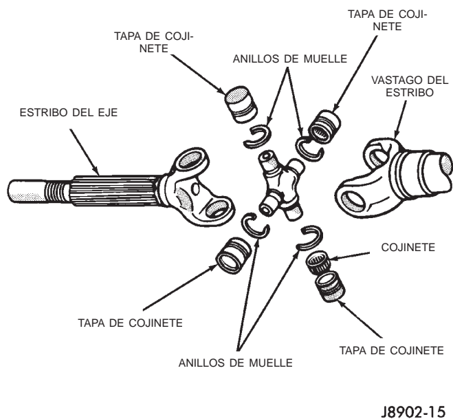
Fig. 4 Articulación universal exterior del semieje
