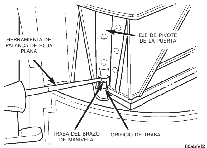
Fig. 57 Desmontaje e instalación de la palanca de la puerta de modo-característico
