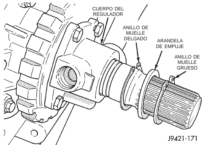
Fig. 36 Anillos de muelle y separador
