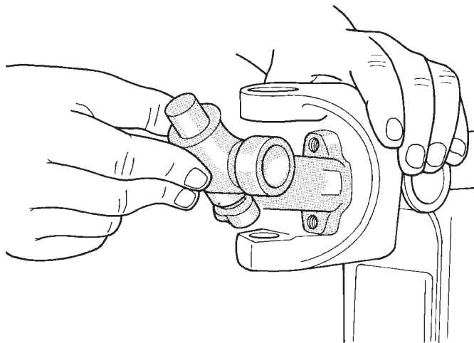
Fig. 32 Instalación de la cruceta restante
