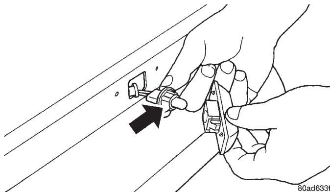
Fig. 3 Luz repetidora lateral
