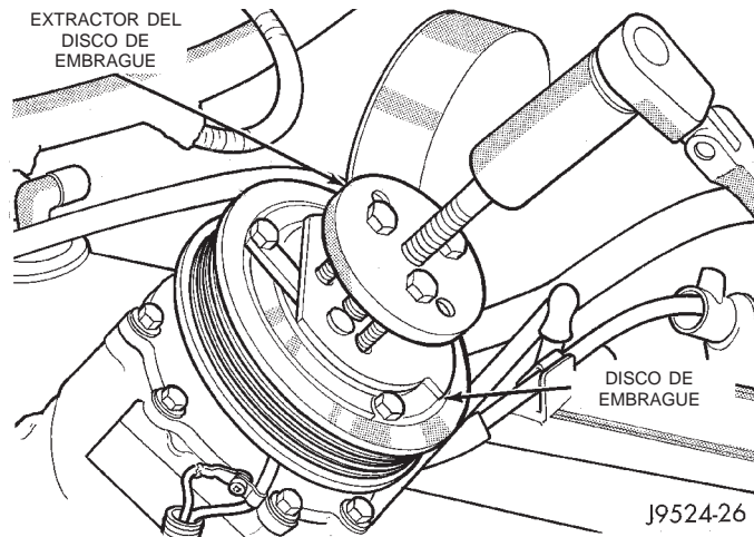
Fig. 24 Desmontaje del disco de embrague
