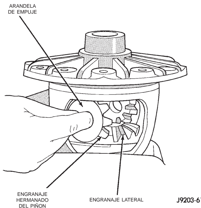
Fig. 41 Desmontaje de engranajes hermanados del piñón
