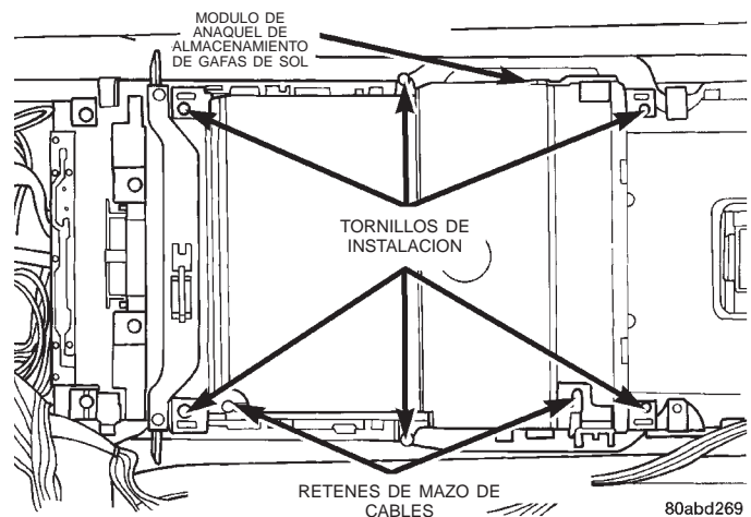
Fig. 6 Desmontaje e instalación de anaquel de almacenamiento de gafas de sol
