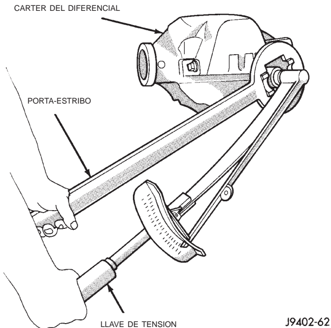
Fig. 15 Apriete de la tuerca del eje del piñón
