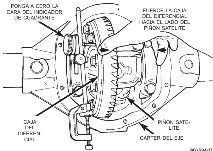
Fig. 57 Sujeción de la caja del diferencial y puesta a cero del indicador de cuadrante
