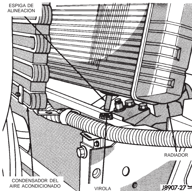
Fig. 35 Espigas de alineación del radiador—Características
