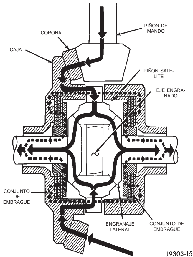
Fig. 5 Funcionamiento del diferencial de desplazamiento limitado Trac-lok™
