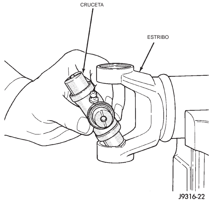
Fig. 20 Instalación de la cruceta en el estribo
