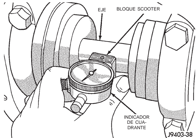
Fig. 49 Medición de profundidad de piñón satélite—Característica
