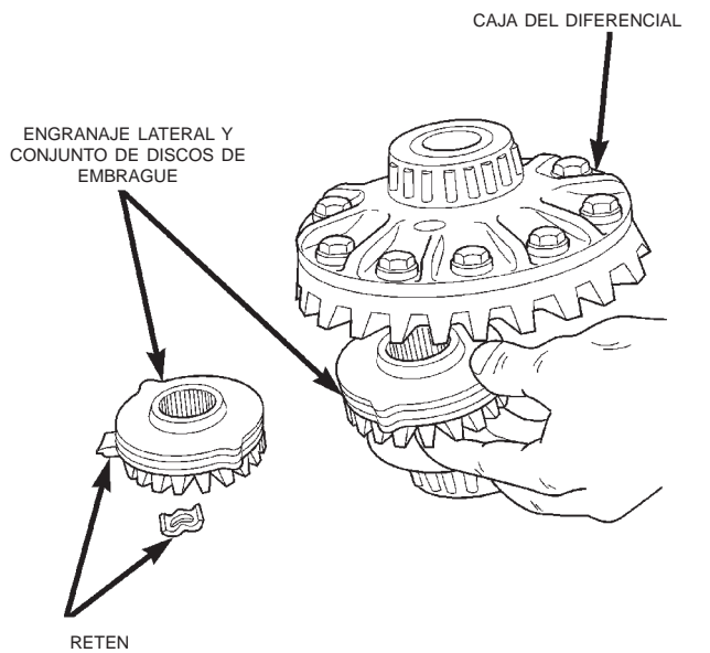
Fig. 60 Desmontaje de engranaje lateral y disco de embrague
