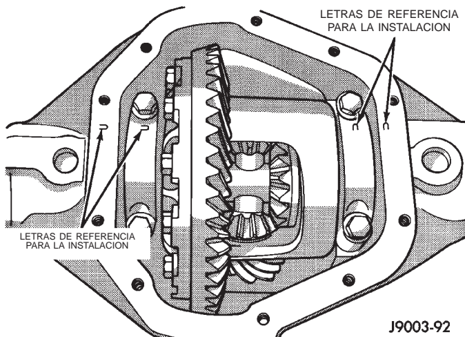
Fig. 22 Letras de referencia de la tapa de cojinete del diferencial
