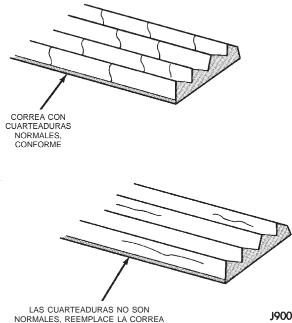
Fig. 10 Esquemas de desgaste de la correa
