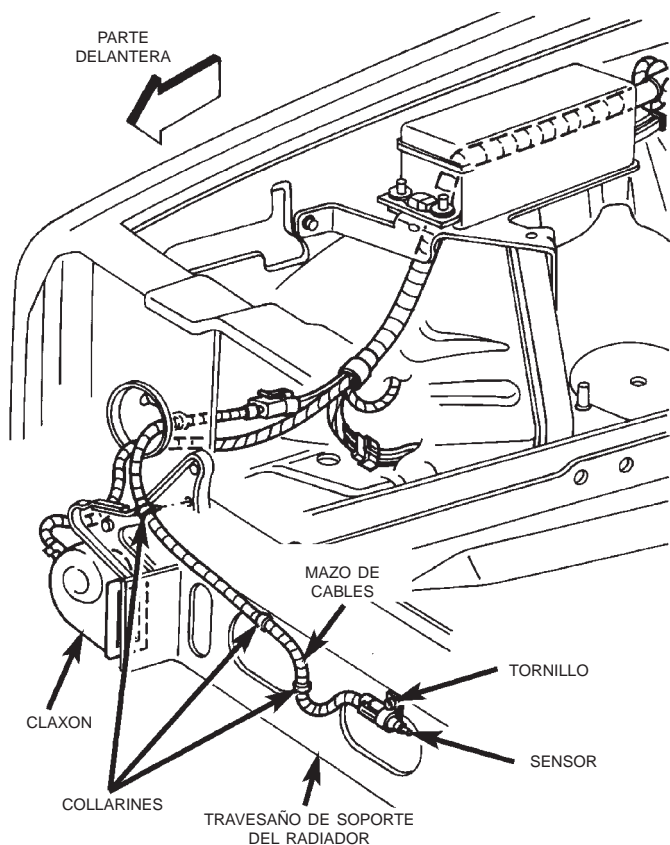
Fig. 7 Desmontaje e instalación del sensor de temperatura ambiente
