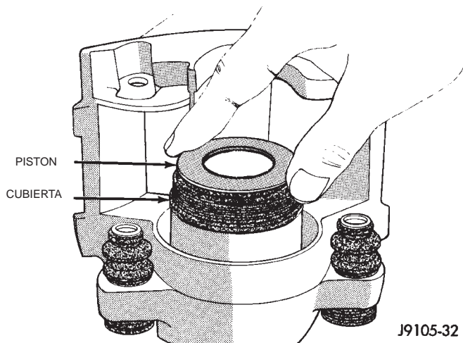
Fig. 53 Instalación del pistón del calibrador
