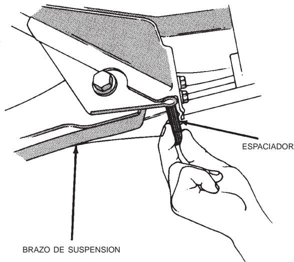
Fig. 36 Ajuste del ángulo en los muelles de láminas
