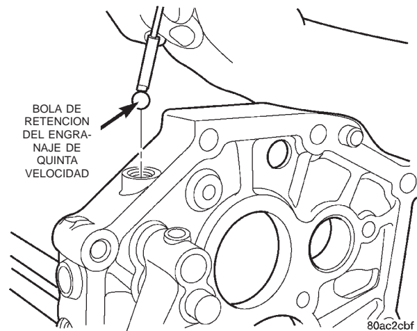
Fig. 68 Desmontaje de bola de retención del engranaje de quinta velocidad
