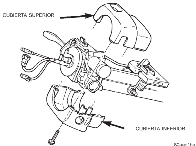
Fig. 3 Cubiertas de la columna
