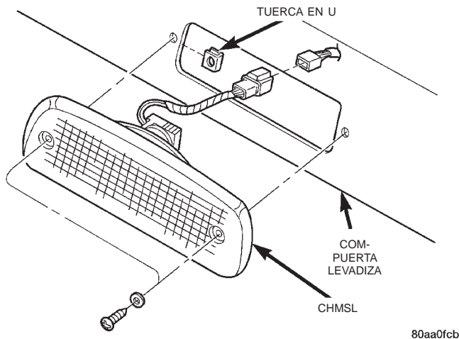
Fig. 7 Luz de stop central superior
