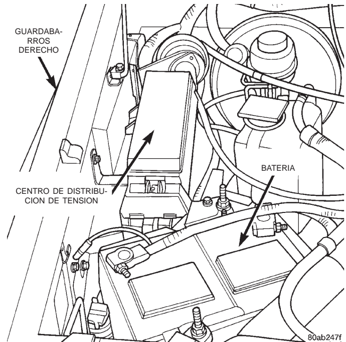
Fig. 30 Centro de distribución de tensión
