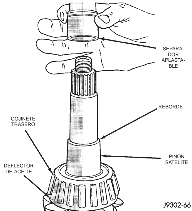
Fig. 38 Separador aplastable
