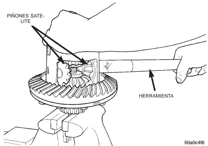
Fig. 46 Desmontaje de piñones satélite
