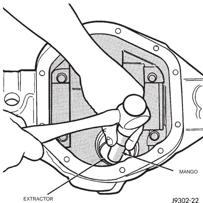
Fig. 26 Desmontaje de la cubeta del cojinete delantero
