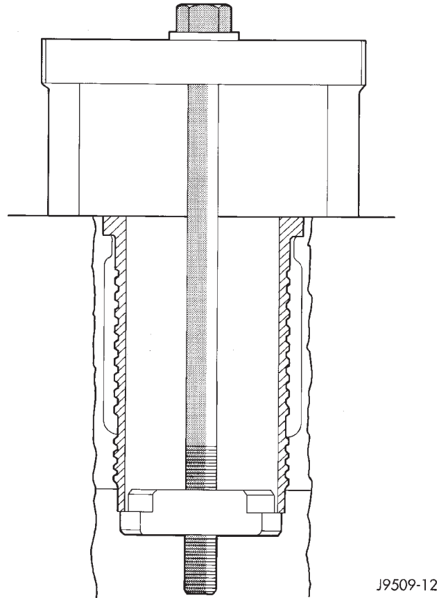
Fig. 62 Herramienta de desmontaje de camisas
