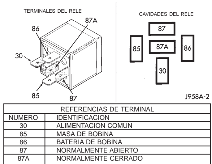
Fig. 3 Relé de encendedor de cigarrillos
