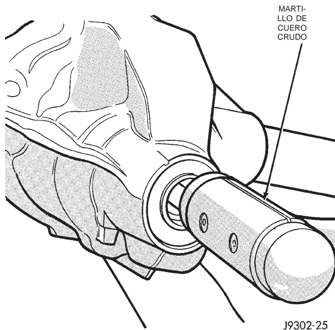
Fig. 13 Desmontaje del piñón satélite
