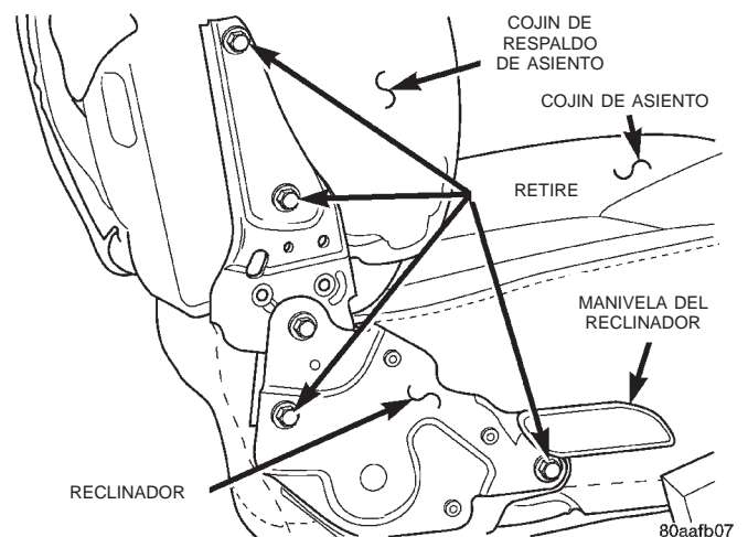
Fig. 13 Reclinator de asiento individual conformado
