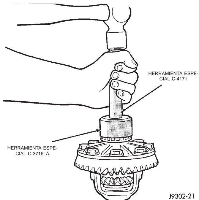
Fig. 24 Instalación de cojinetes laterales del diferencial
