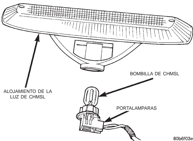
Fig. 6 Bombilla de CHMSL
