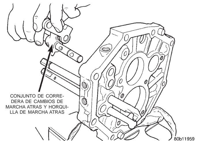
Fig. 70 Desmontaje de corredera de cambios de marcha atrás
