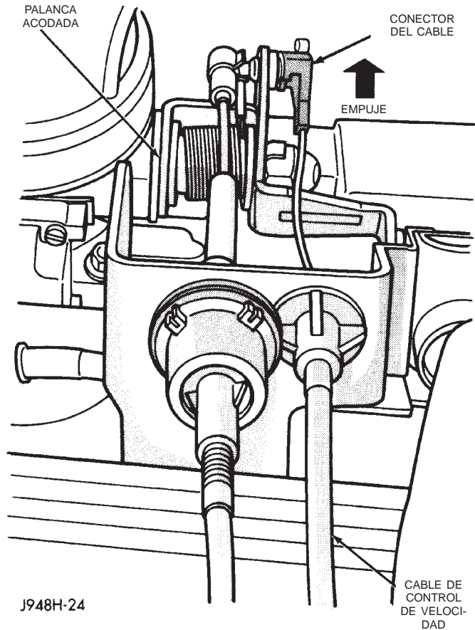
Fig. 4 Cable del servo a la palanca acodada— desmontaje e instalación
