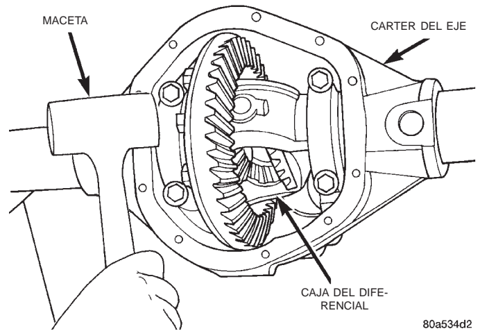
Fig. 52 Calce de cojinete lateral del diferencial en el lado del piñon satélite
