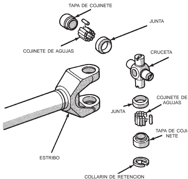
Fig. 3 Articulación universal sencilla
