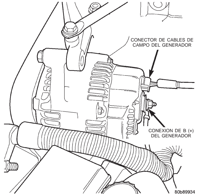
Fig. 1 Terminales del generador
