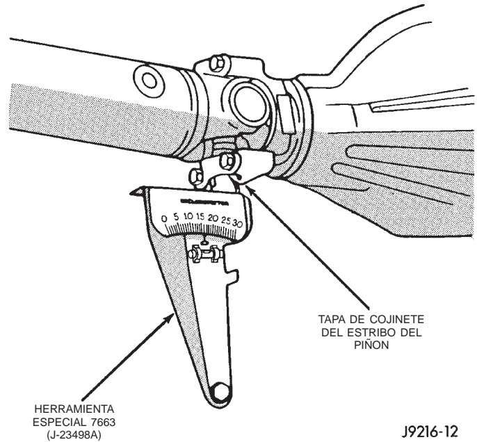
Fig. 10 Medición del ángulo (de impulsión) trasero (B)
