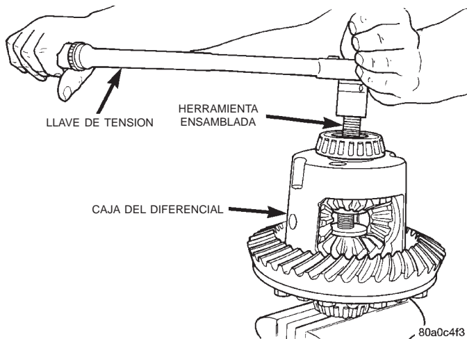
Fig. 44 Apriete de herramienta compresora de muelles Belleville
