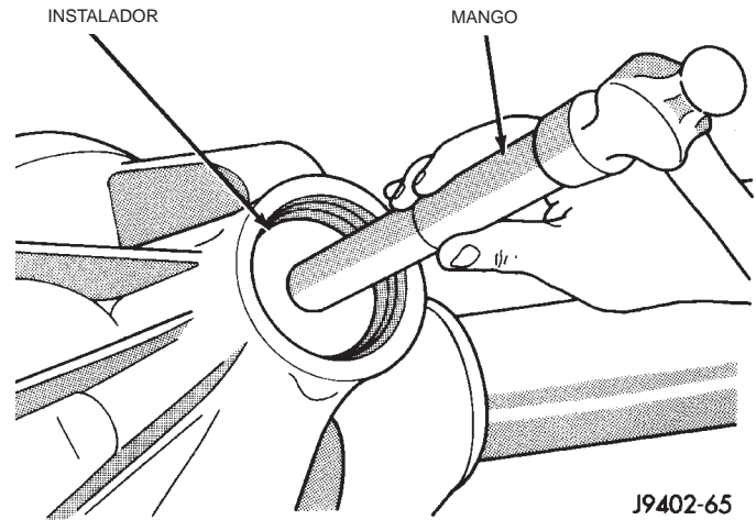
Fig. 41 Instalación de la cubeta del cojinete delantero del piñón
