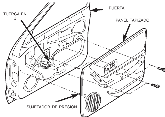
Fig. 23 Panel tapizado de la puerta delantera—Elevallas eléctrico
