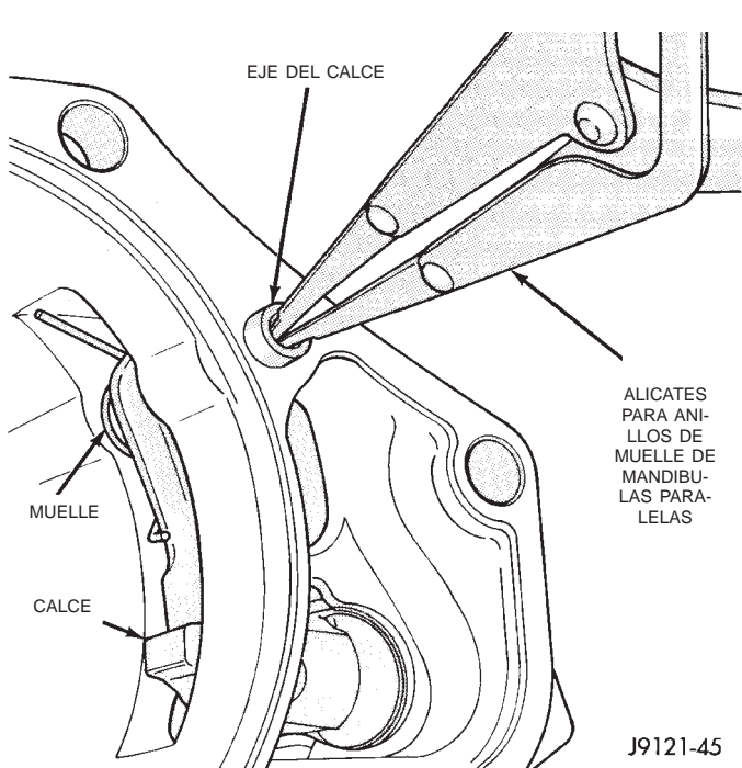
Fig. 170 Calce de estacionamiento, eje y muelle
