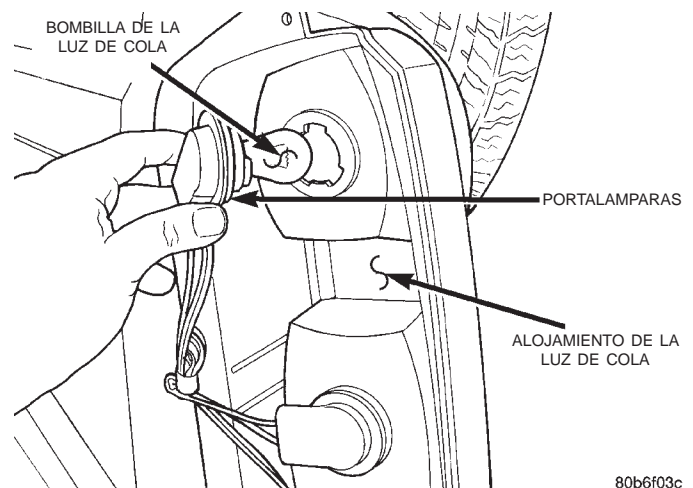
Fig. 5 Desmontaje del portalámparas
