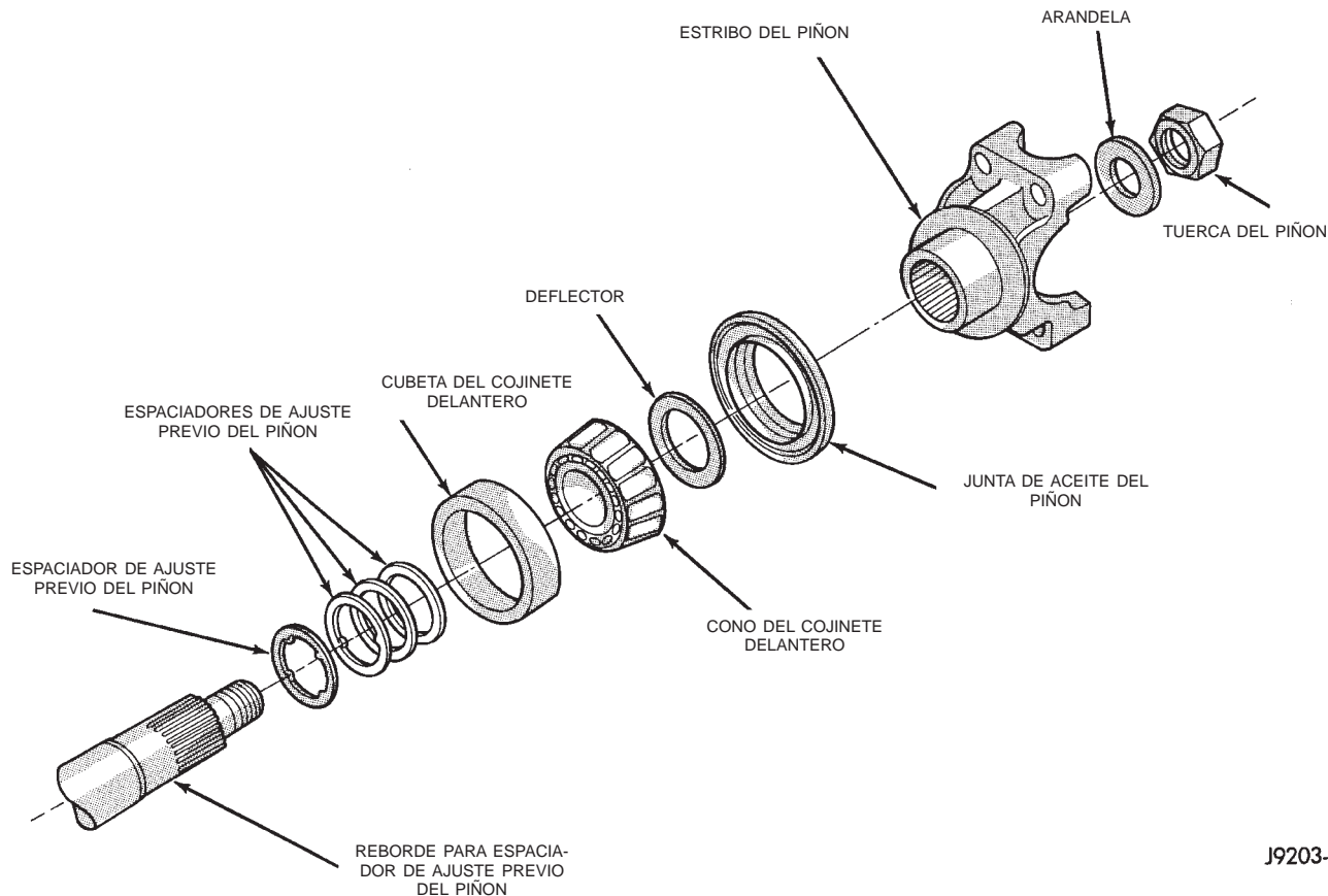
Fig. 37 Espaciadores de ajuste previo—Caraterísticos
