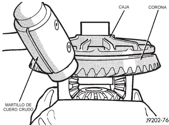
Fig. 32 Desmontaje de la corona
