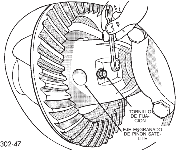
Fig. 36 Tornillo de fijación de eje engranado del piñón satélite
