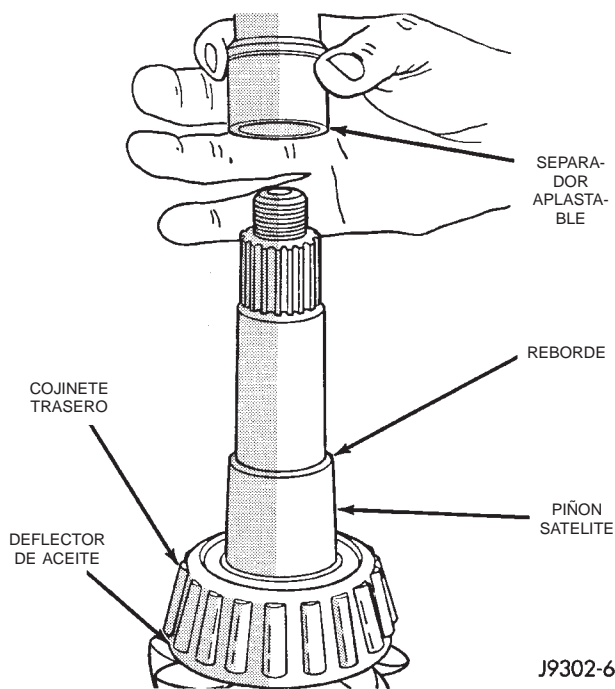
Fig. 34 Separador de ajuste previo aplastable
