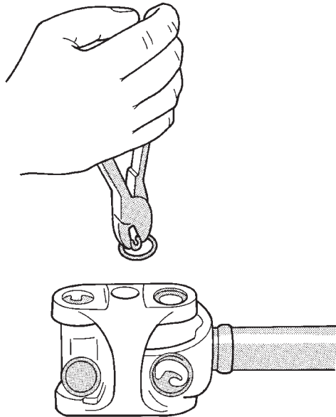
Fig. 22 Desmontaje de anillos de muelle
