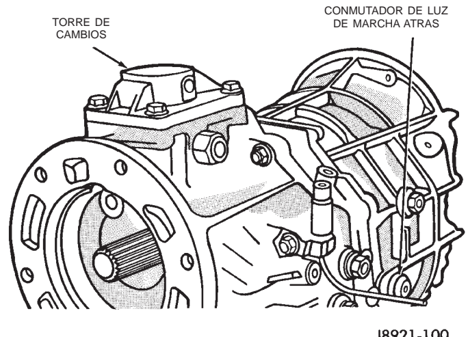
Fig. 50 Instalación de torre de cambios y conmutador de luz de marcha atrás
