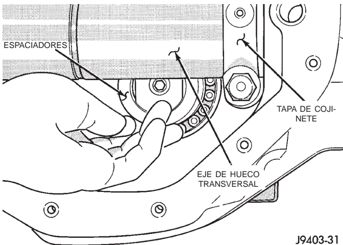
Fig. 56 Selección de espaciador (es) de profundidad
