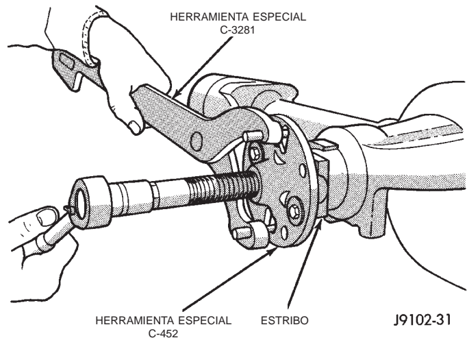
Fig. 34 Desmontaje del estribo del piñón
