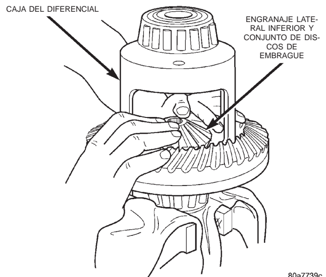
Fig. 62 Instalación de discos de embrague y engranaje lateral inferior
