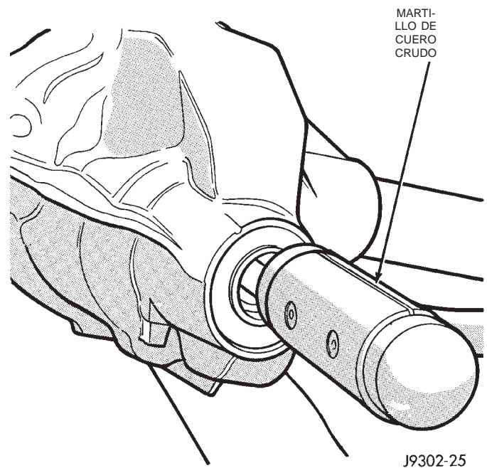
Fig. 29 Desmontaje del piñón satélite
