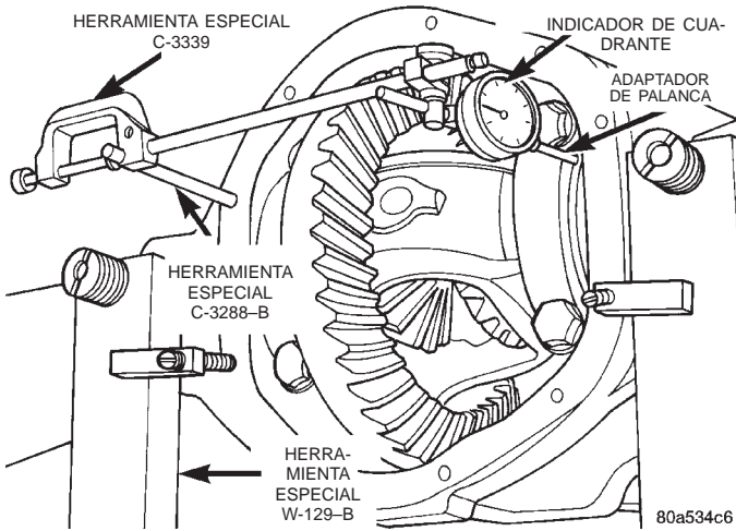
Fig. 18 Instalación del indicador de cuadrante
