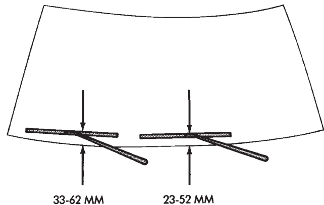
Fig. 5 Desmontaje e instalación del brazo del limpiador
