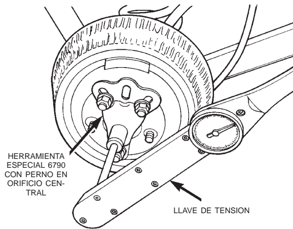
Fig. 5 Prueba del Trac-lok™—Característica
