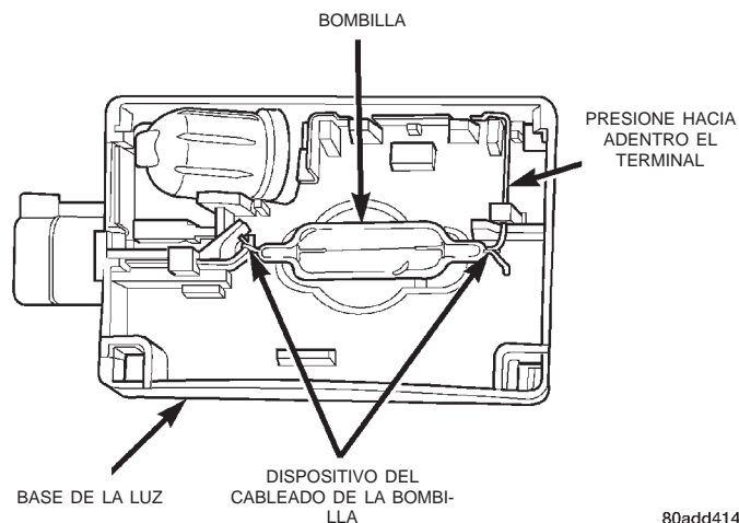
Fig. 8 Bombilla de la luz de debajo del capó
