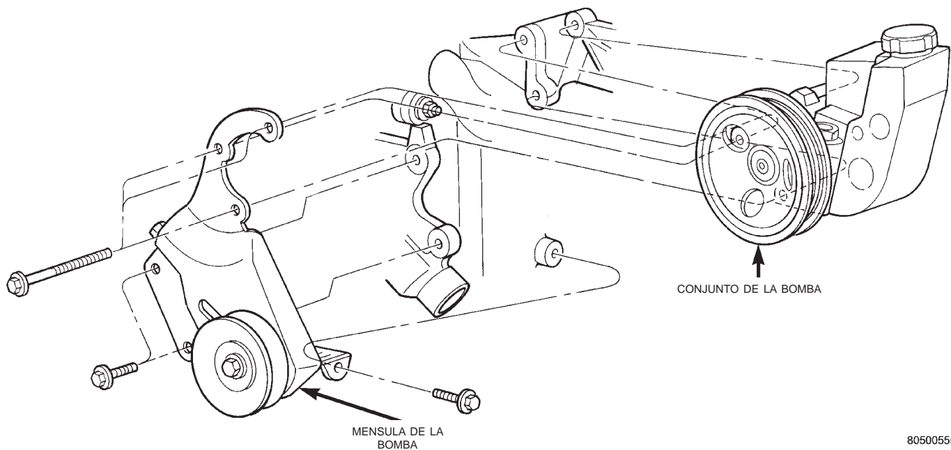
Fig. 24 Fijación de la bomba de la dirección asistida-4.0L
