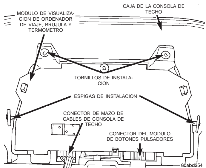
Fig. 4 Desmontaje e instalación de módulo de visualización de ordenador de viaje, brújula y termómetro
