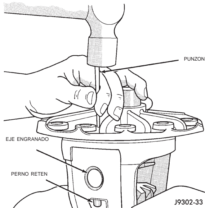
Fig. 40 Desmontaje de pasador de rodillo de eje engranado
