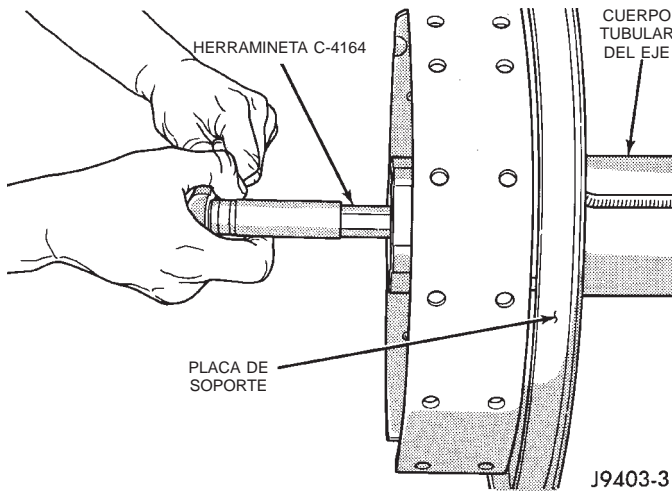
Fig. 18 Herramienta para ajustador roscado
