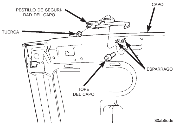
Fig. 7 Pestillo de seguridad del capó
