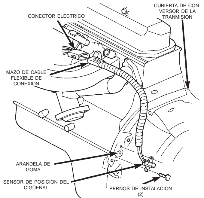
Fig. 22 Sensor de posición del cigüeñal—Motor de 2.5L 4 cilindros con transmisión automática
