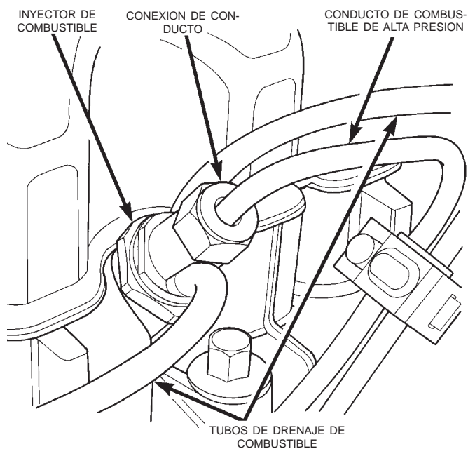
Fig. 40 Inyector de combustible—característico
