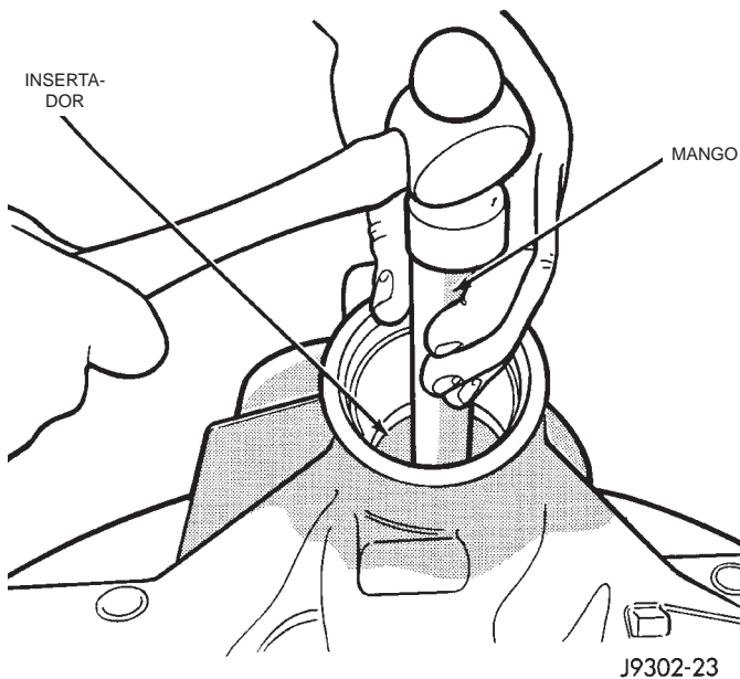
Fig. 37 Desmontaje de la cubeta del cojinete trasero
