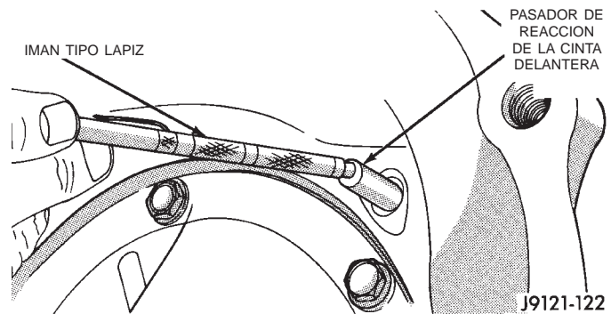
Fig. 91 Pasador de reacción de la cinta delantera
