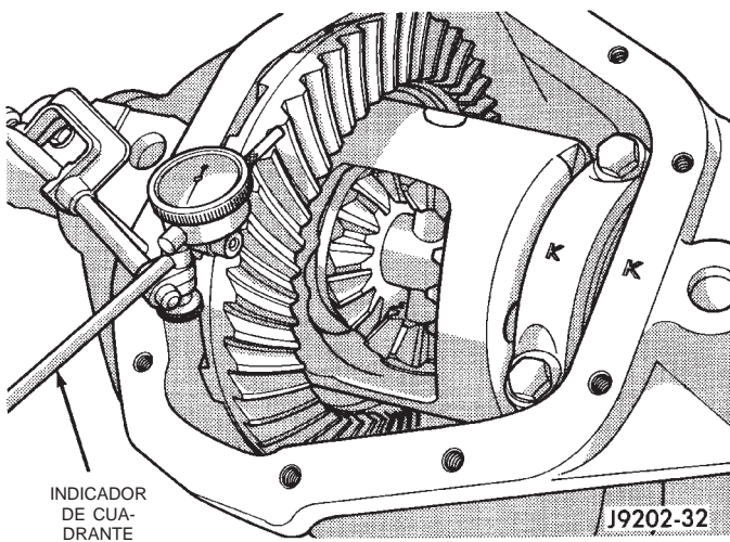
Fig. 77 Medición de holgura entre dientes de la corona
