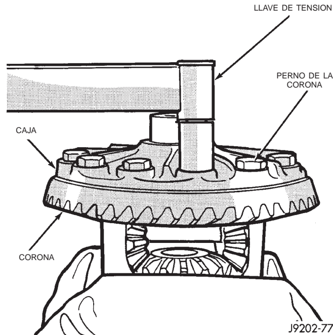
Fig. 23 Instalación de pernos de la corona
