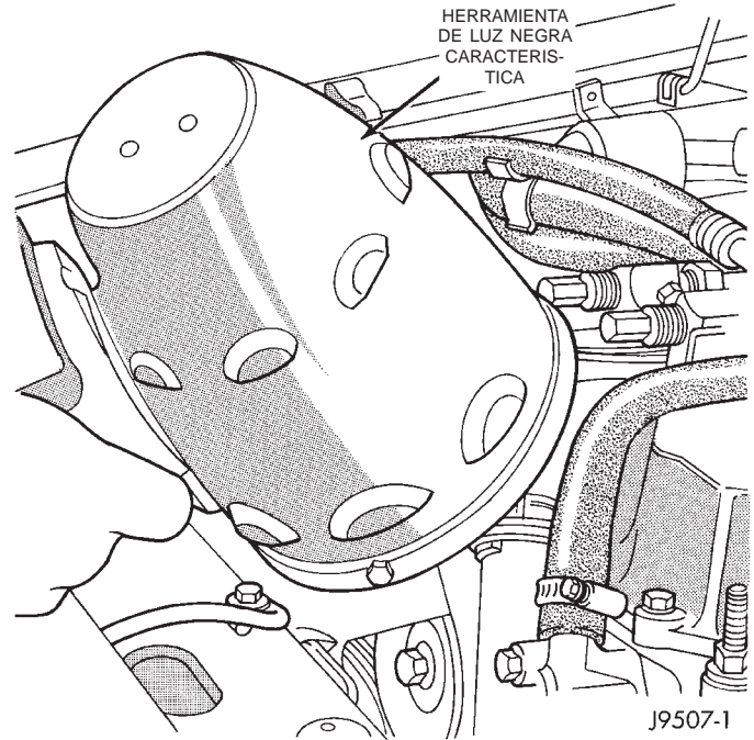
Fig. 9 Detección de fugas utilizando luz negra—Característica
