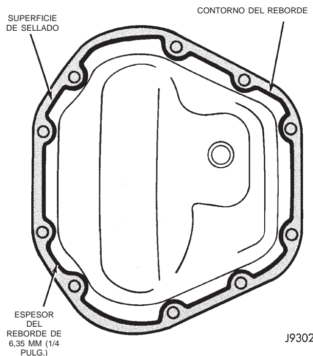
Fig. 3 Tapa de cárter con sellante característica
