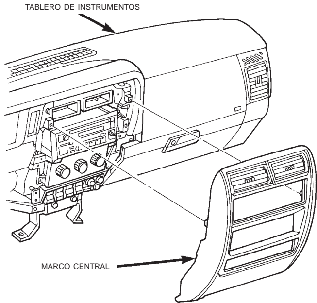
Fig. 7 Desmontaje e instalación del marco central en el tablero de instrumentos 80ab87bc
