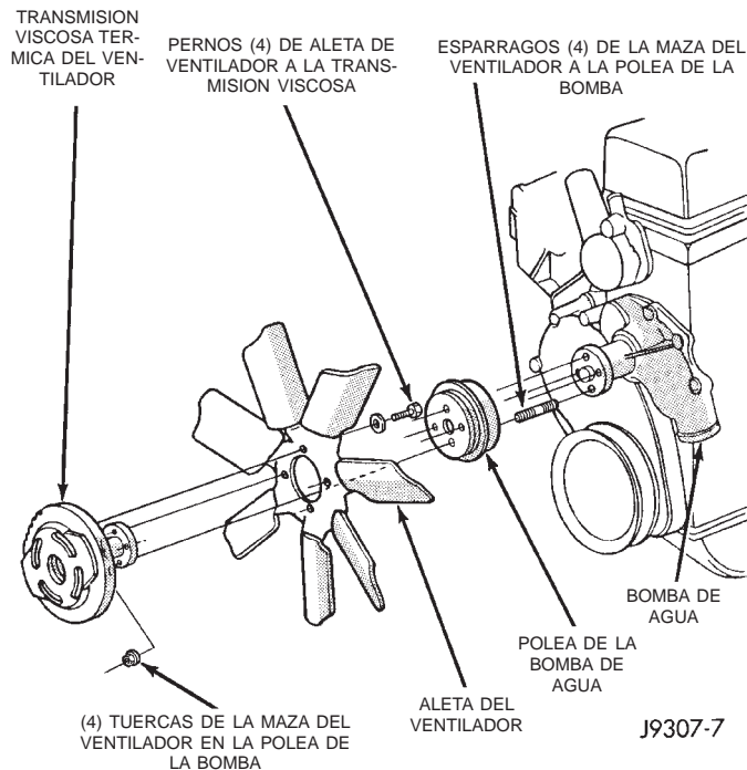
Fig. 20 Tuercas de instalación del ventilador
