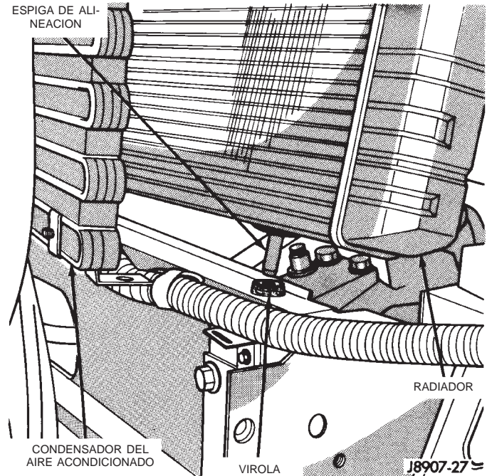
Fig. 16 Espigas de alineación del radiador—Características
