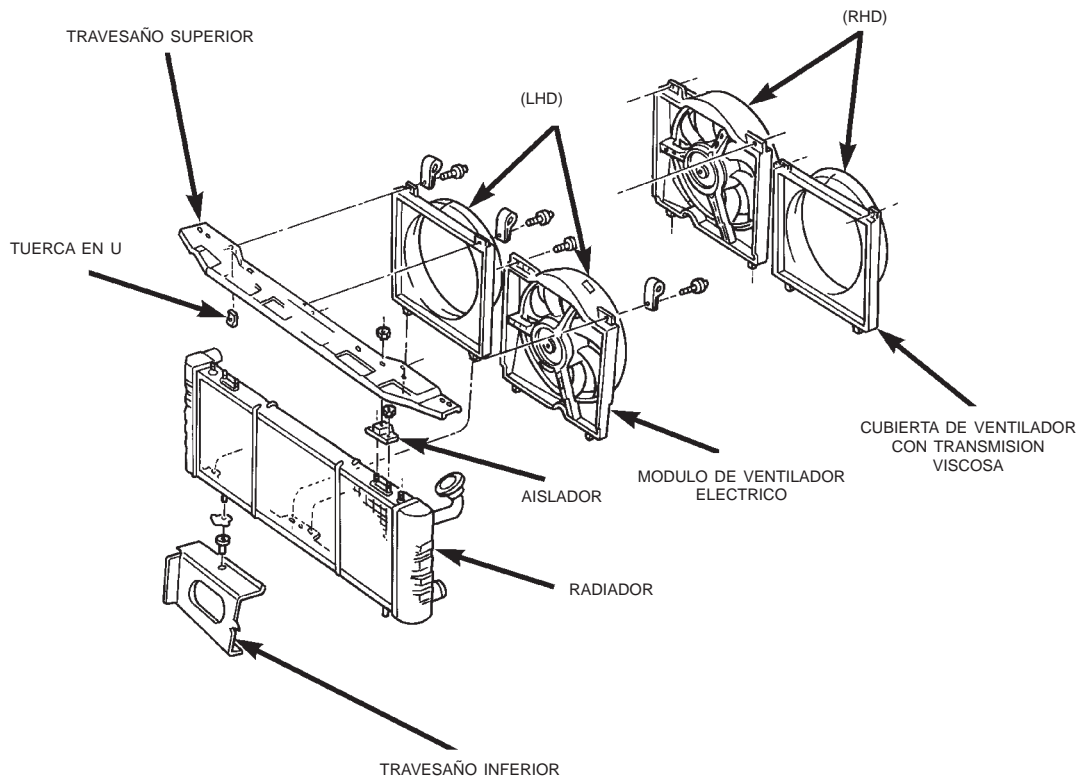
Fig. 33 Desmontaje e instalación del radiador—Motores 4.0L
