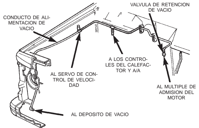
Fig. 58 Alimentación de vacío
