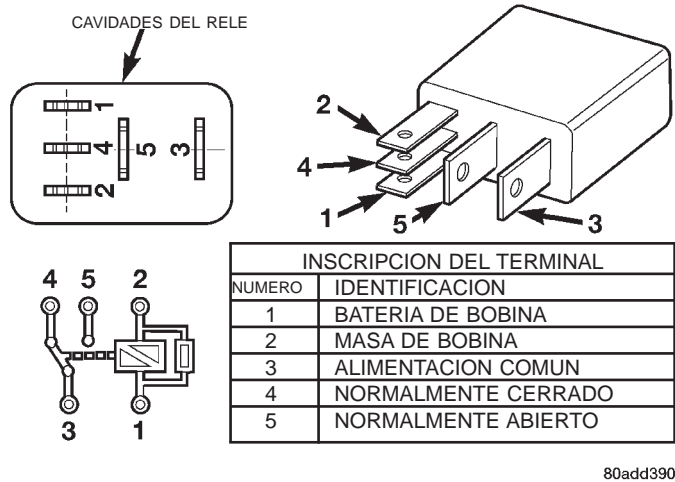
Fig. 12 Relé tipo 3
