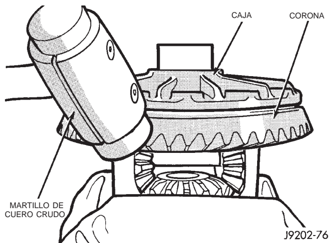
Fig. 26 Desmontaje de la corona
