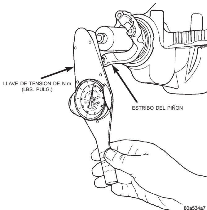
Fig. 39 Comprobación de torsión de rotación del piñón satélite
