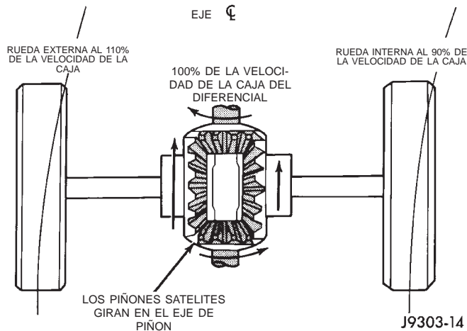
Fig. 3 Funcionamiento del diferencial—En los giros
