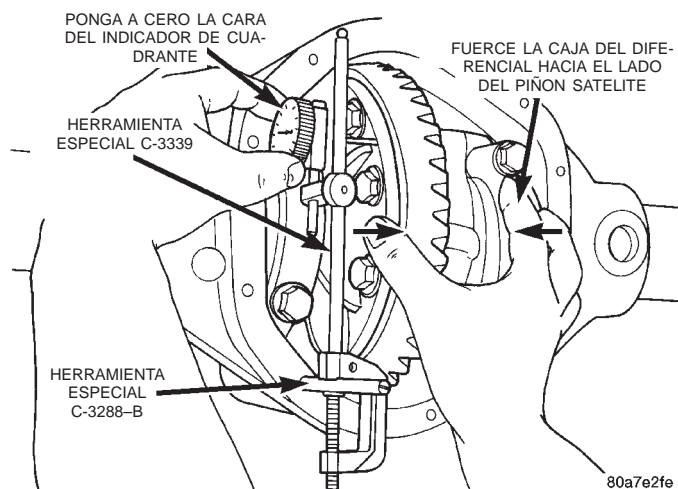
Fig. 55 Sujeción de la caja del diferencial y puesta a cero del indicador de cuadrante
