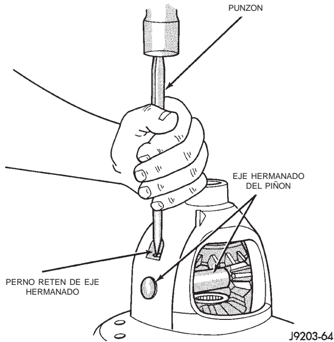
Fig. 42 Instalación de pasador de rodillo del eje hermano
