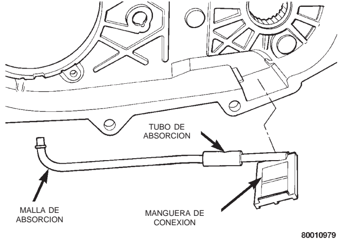
Fig. 20 Desmontaje del tubo de absorción de aceite
