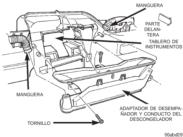
Fig. 64 Adaptador de desempañador y conducto del descongelador
