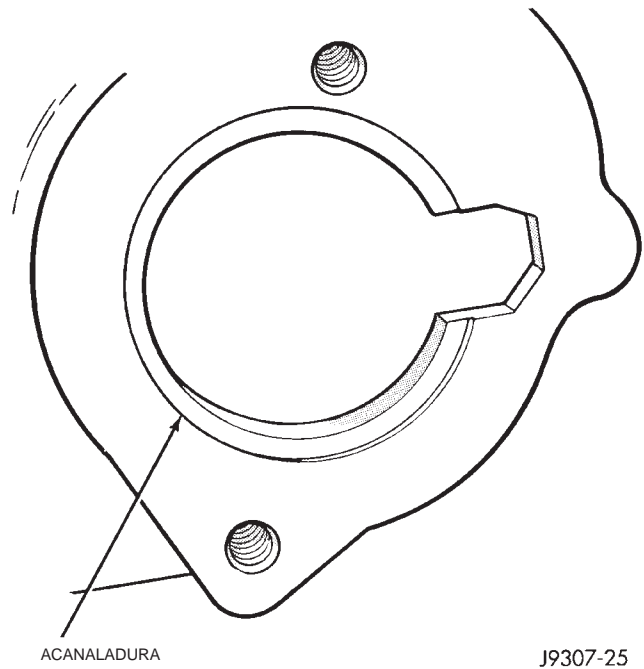
Fig. 27 Escotadura del termostato
