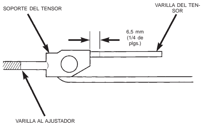
Fig. 61 Medición de la varilla del tensor
