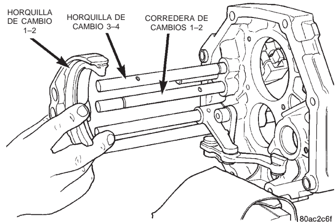
Fig. 85 Instalación de horquilla de cambio 1-2
