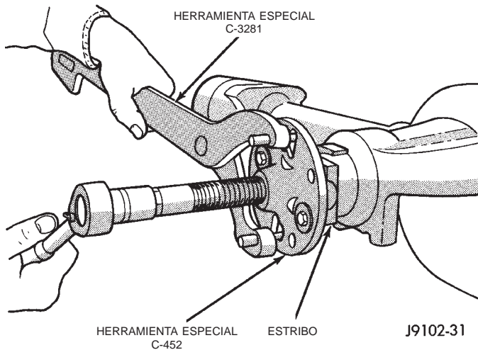
Fig. 6 Desmontaje del estribo del piñón
