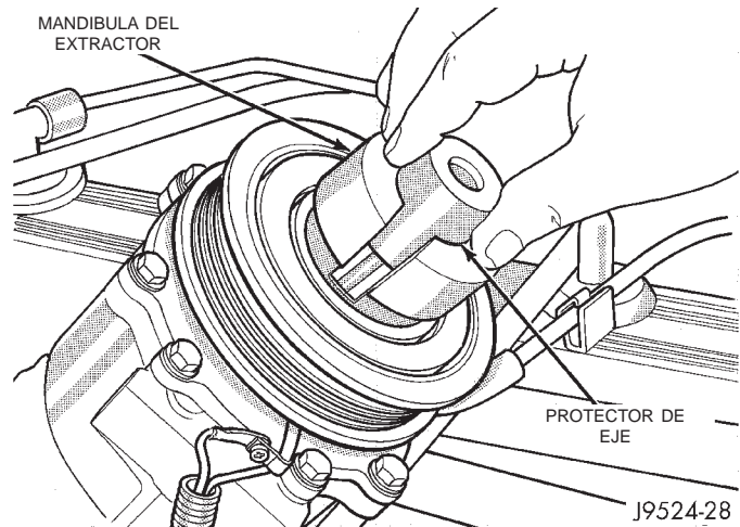
Fig. 26 Protector de eje y extractor
