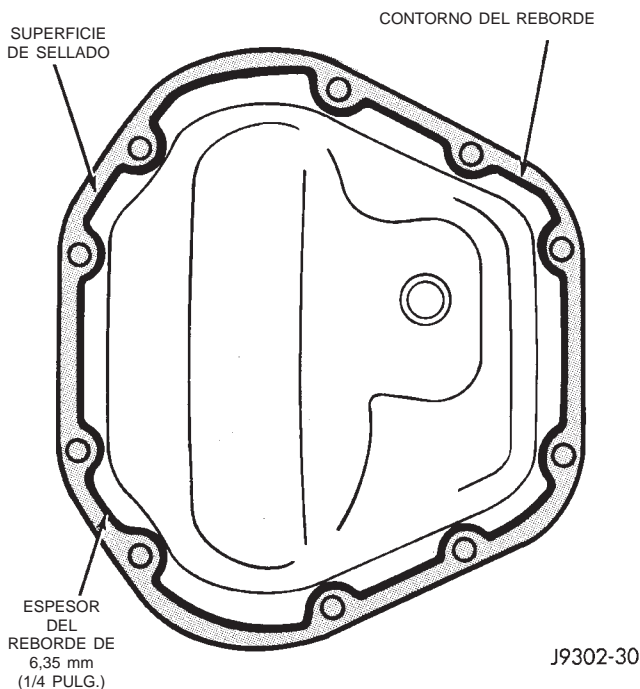
Fig. 48 Tapa de cárter característica con sellante
