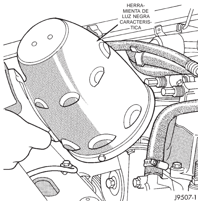
Fig. 11 Detección de fugas utilizando luz negra—Característico
