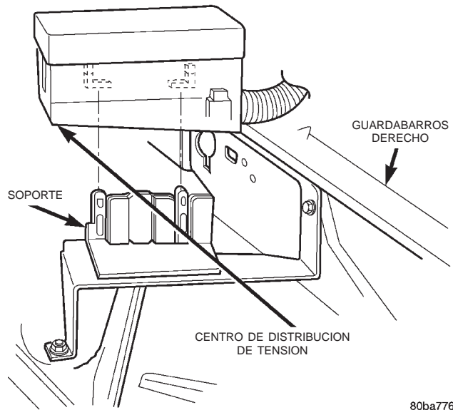
Fig. 4 Desmontaje e instalación del centro de distribución de tensión
