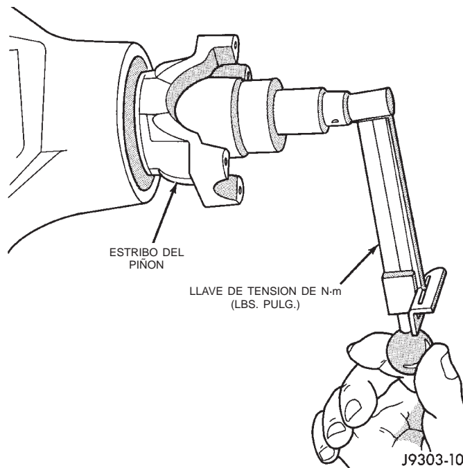
Fig. 10 Comprobación de torsión de rotación del piñón
