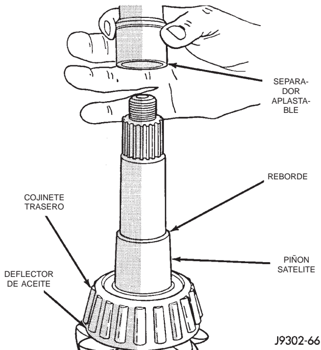
Fig. 14 Separador de ajuste previo aplastable
