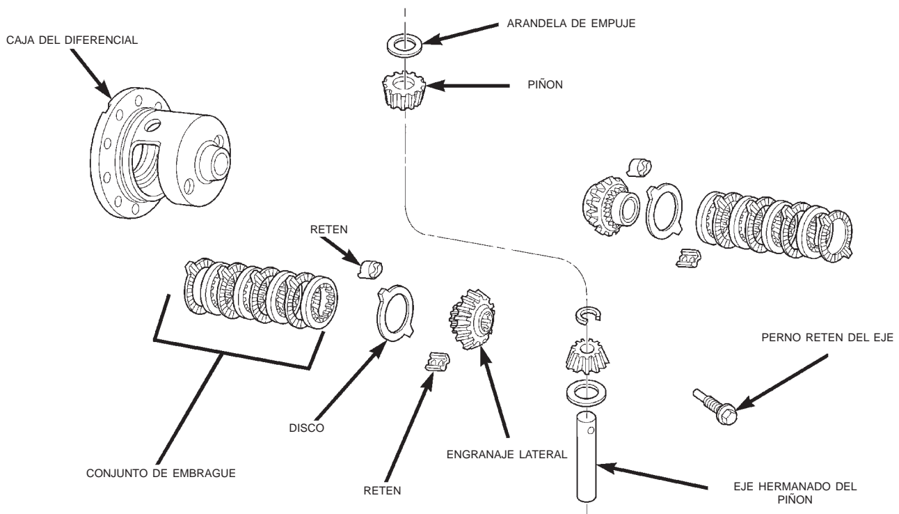
Fig. 51 Componentes del diferencial Trac-lok™
