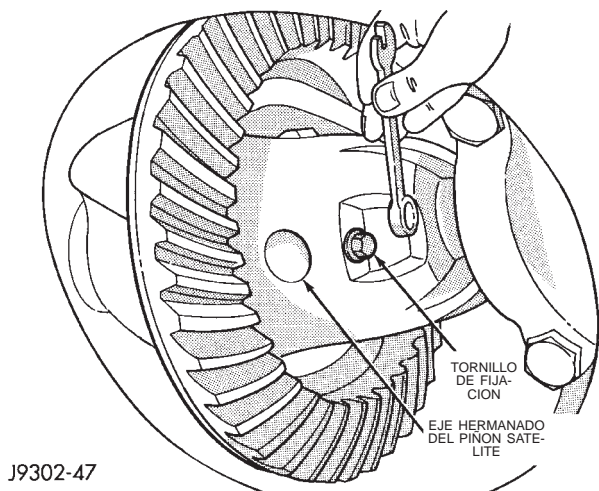
Fig. 53 Tornillo de fijación del eje hermano
