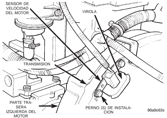
Fig. 6 Localización del sensor de velocidad del motor
