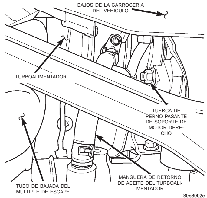
Fig. 2 Manguera de retorno de aceite del turboalimentador — Posición y orientación
