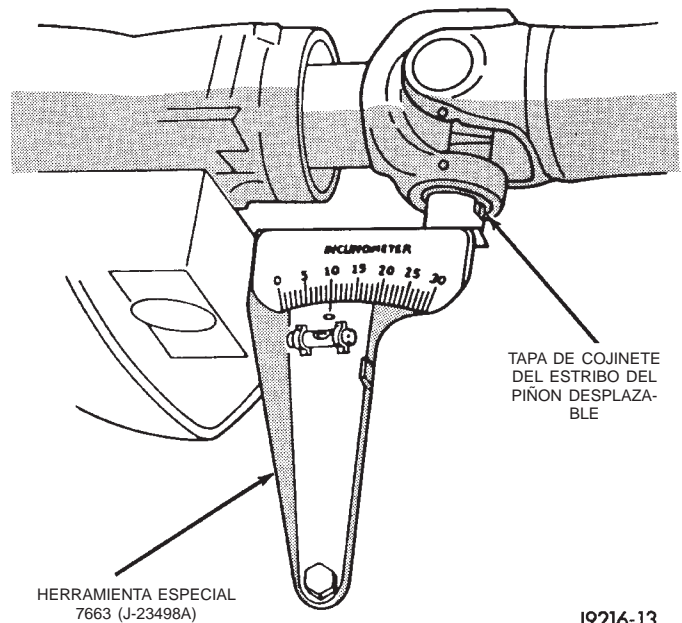
Fig. 8 Medidor del ángulo (de transmisión) delantero (A)
