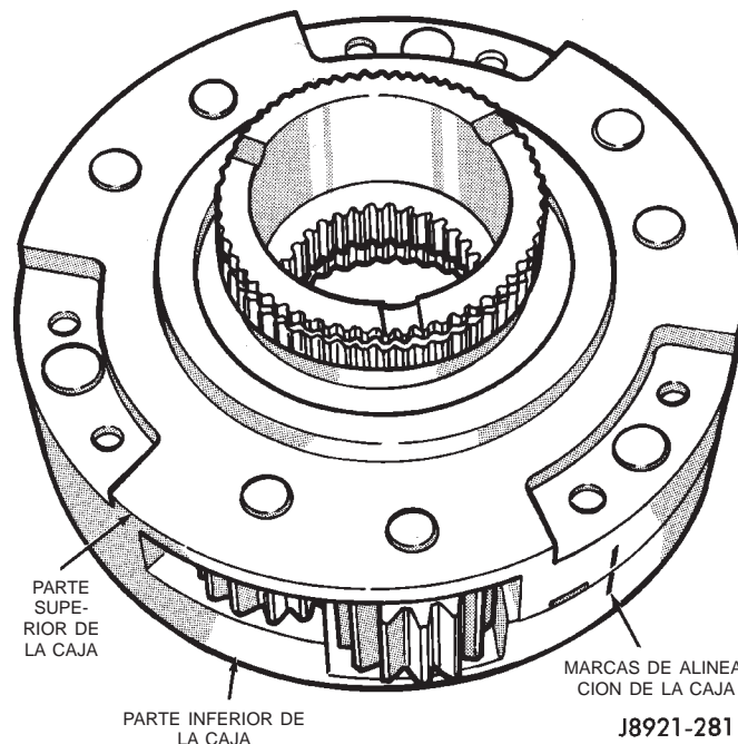
Fig. 63 Ensamblaje de la caja del diferencial ENSAMBLAJE DE ENGRANAJE IMPULSOR/DE BAJA
