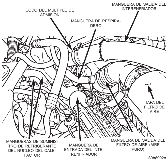
Fig. 1 Compartimiento del motor - LHD — Diesel
