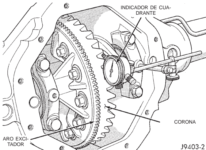
Fig. 58 Medición de la holgura entre dientes de la corona
