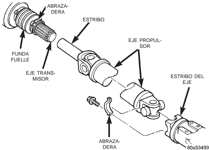
Fig. 15 Eje propulsor trasero
