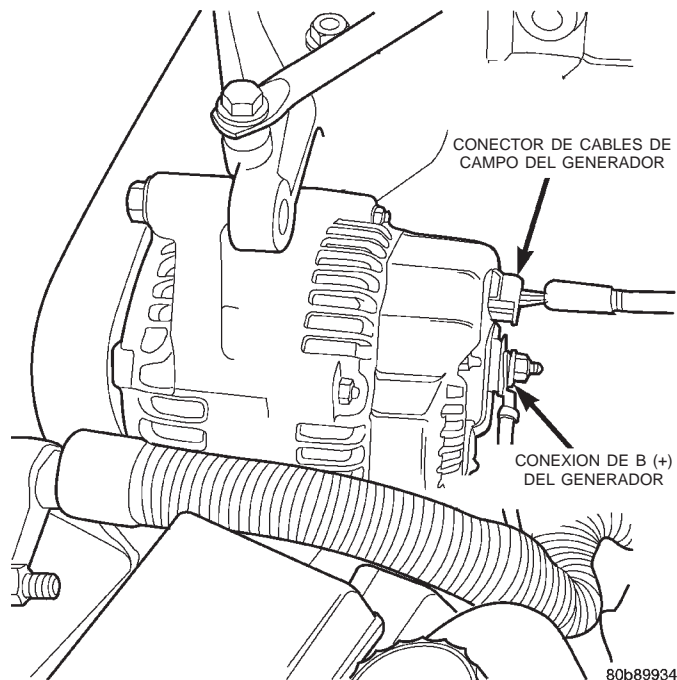
Fig. 4 Terminales del generador
