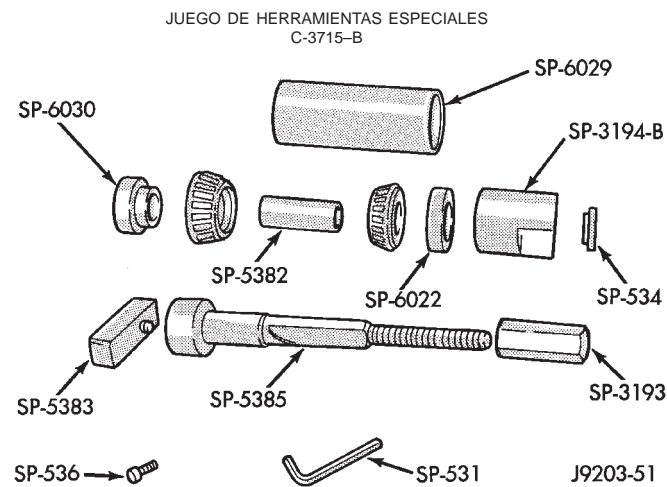
Fig. 53 Herramientas de ajuste de piñón de eje 8 1/4
