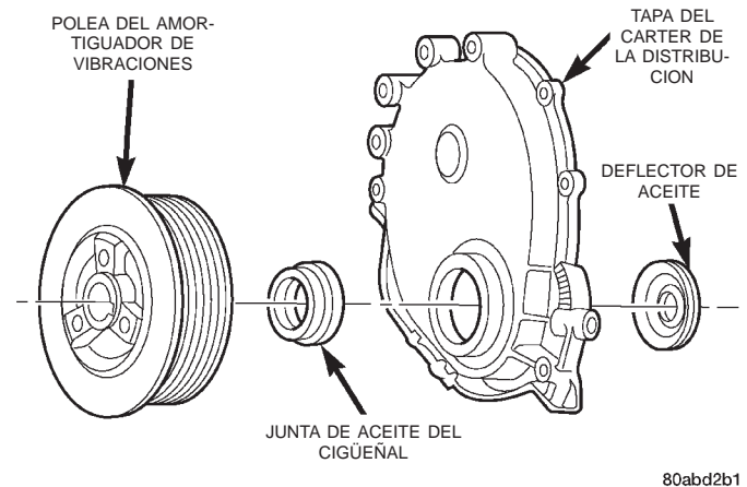
Fig. 39 Componentes de la tapa del cárter de la distribución
