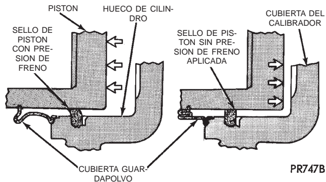
Fig. 3 Compensación del desgaste del forro con el sello de pistón
