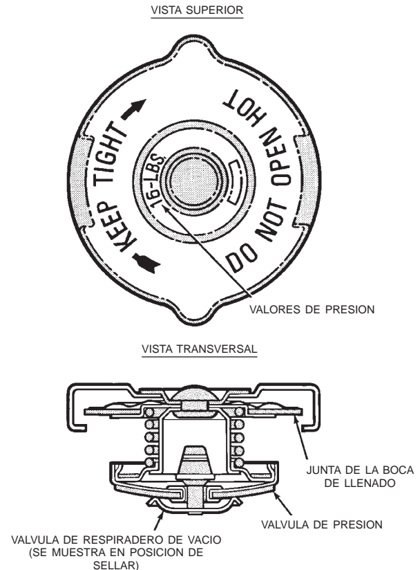
Fig. 13 Tapón de presión del radiador
