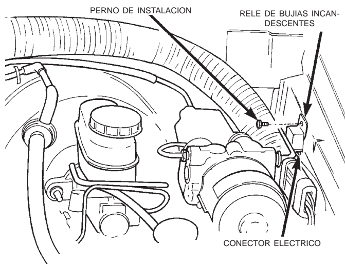
Fig. 13 Localización del relé de bujías incandescentes
