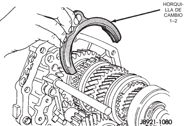
Fig. 73 Desmontaje de las horquillas de cambio
