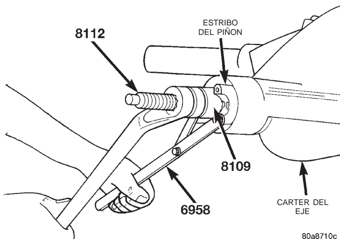
Fig. 9 Instalación del estribo del piñón
