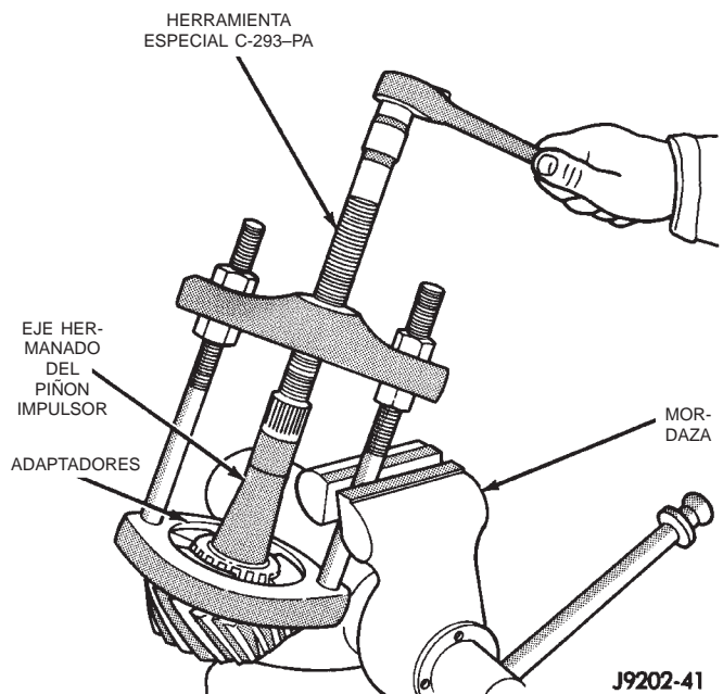
Fig. 39 Desmontaje del cojinete trasero
