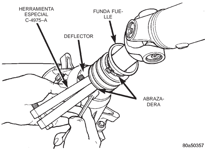
Fig. 16 Cierre de la abrazadera de la junta guardapolvo—Característica
