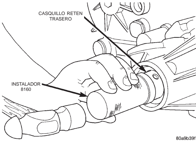
Fig. 9 Instalación del casquillo retén trasero
