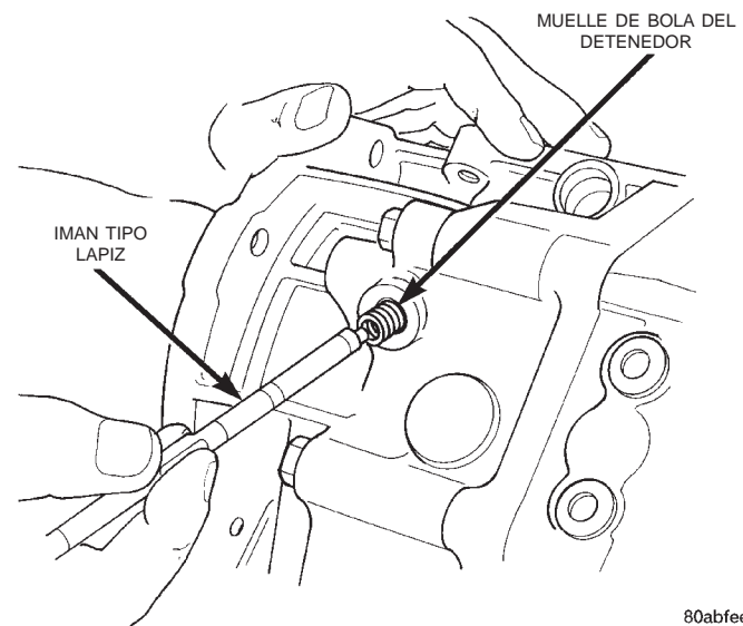
Fig. 45 Instalación de muelle del detenedor
