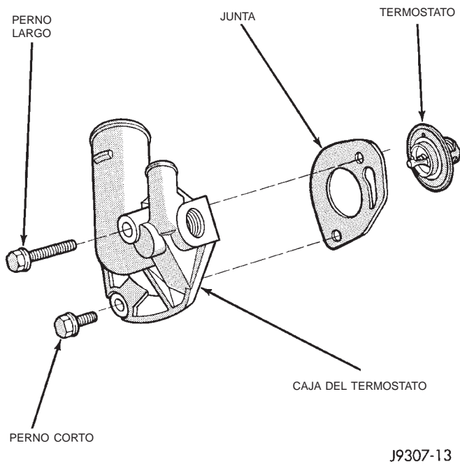
Fig. 26 Desmontaje e instalación del termostato
