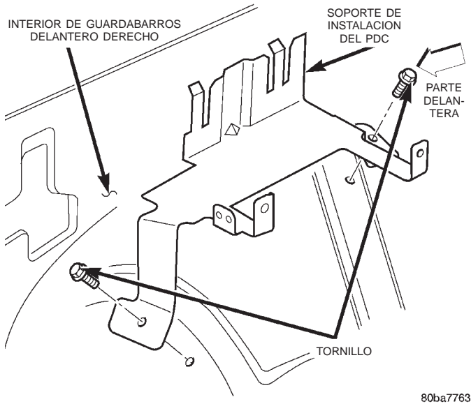
Fig. 5 Desmontaje e instalación del soporte de instalación del PDC
