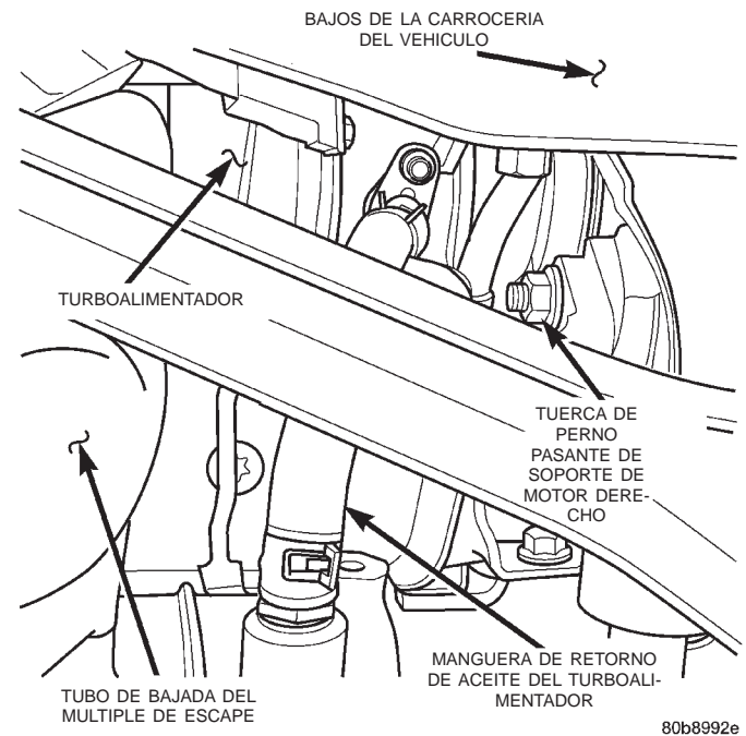
Fig. 3 Conducto de retorno de aceite del turboalimentador
