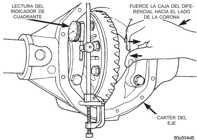
Fig. 56 Sujeción de caja del diferencial y lectura del indicador de cuadrante
