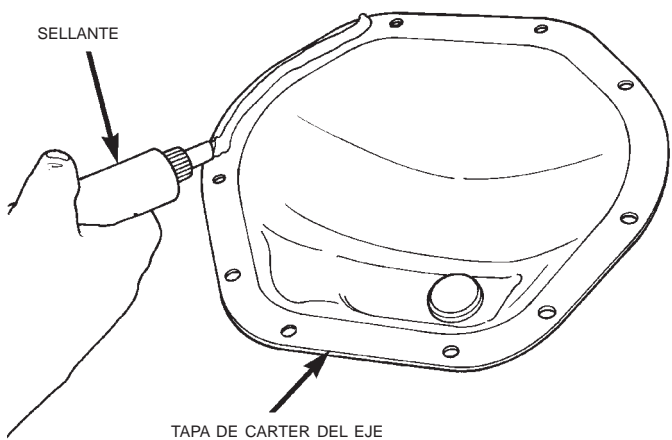
Fig. 6 Aplicación de sellante
