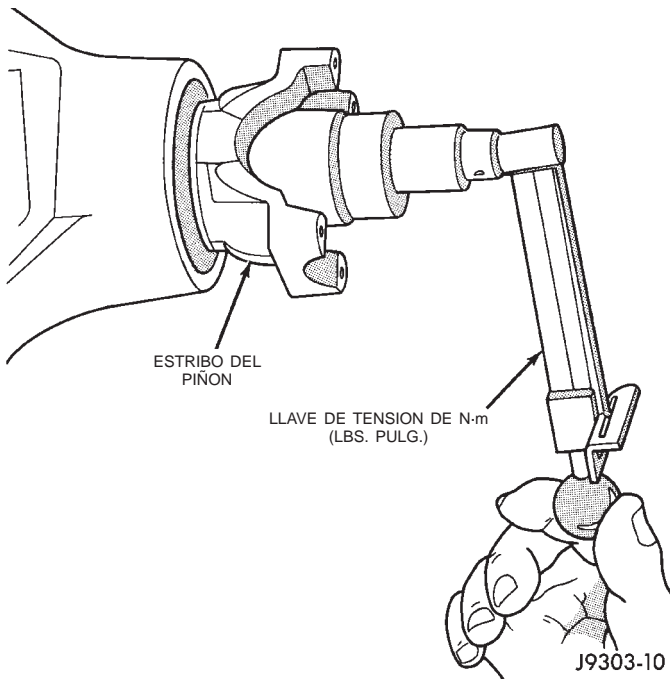
Fig. 35 Comprobación de torsión de rotación del piñón satélite
