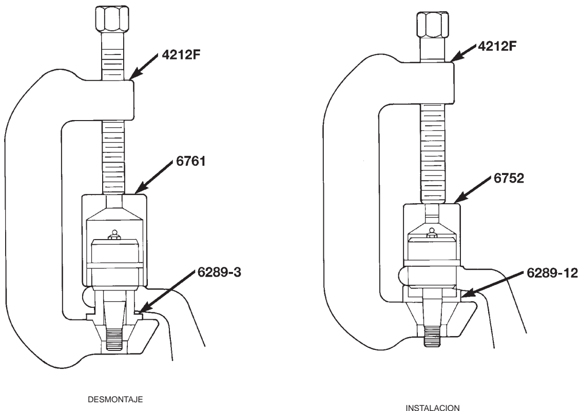
Fig. 14 Desmontaje e instalación del perno de rótula superior
