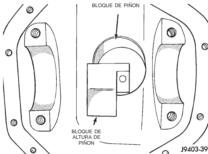
Fig. 67 Bloque de altura de piñón—Característico
