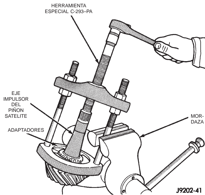
Fig. 29 Desmontaje del cojinete trasero
