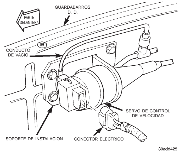
Fig. 1 Localización del servo de control de velocidad
