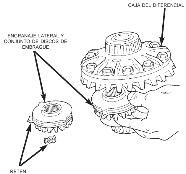
Fig. 47 Desmontaje de engranaje lateral y disco de embrague
