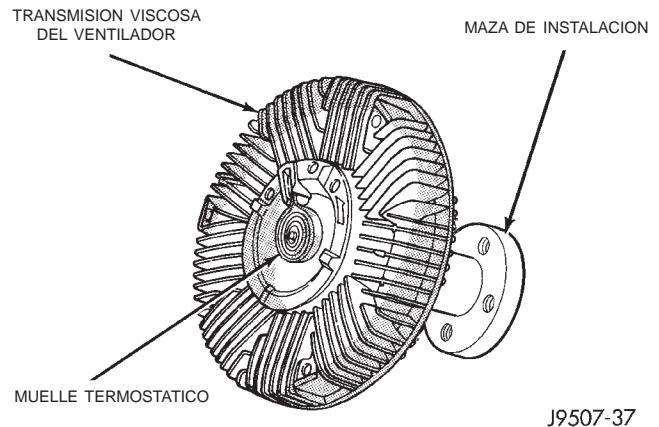
Fig. 8 Transmisión viscosa del ventilador característica
