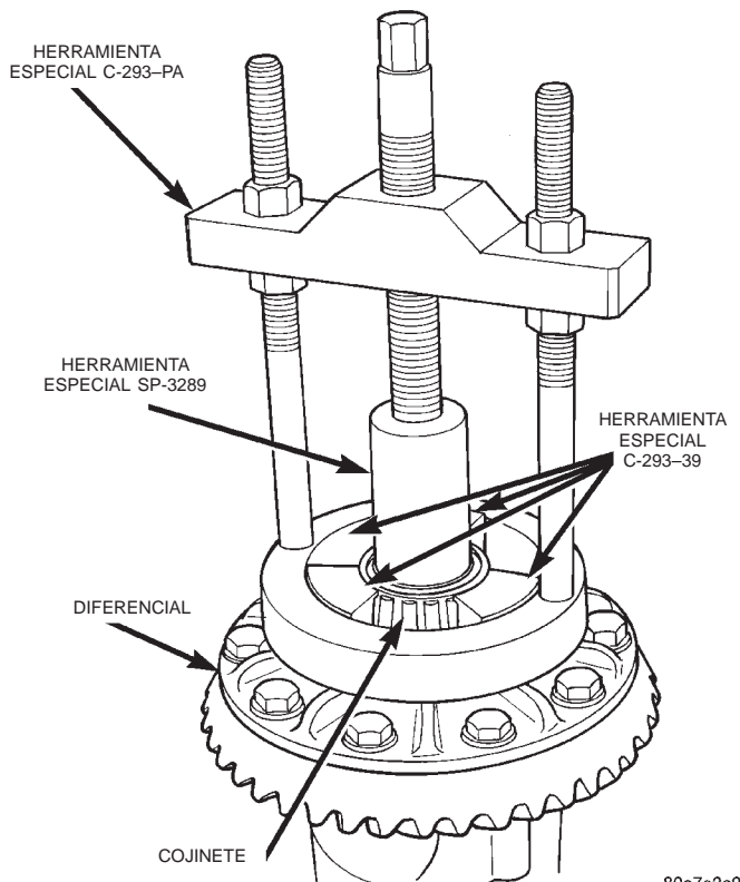
Fig. 23 Desmontaje de cojinete del diferencial
