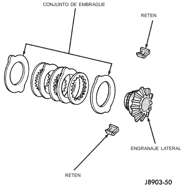
Fig. 61 Conjunto de discos de embrague
