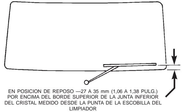
Fig. 8 Instalación de brazo de limpiador trasero
