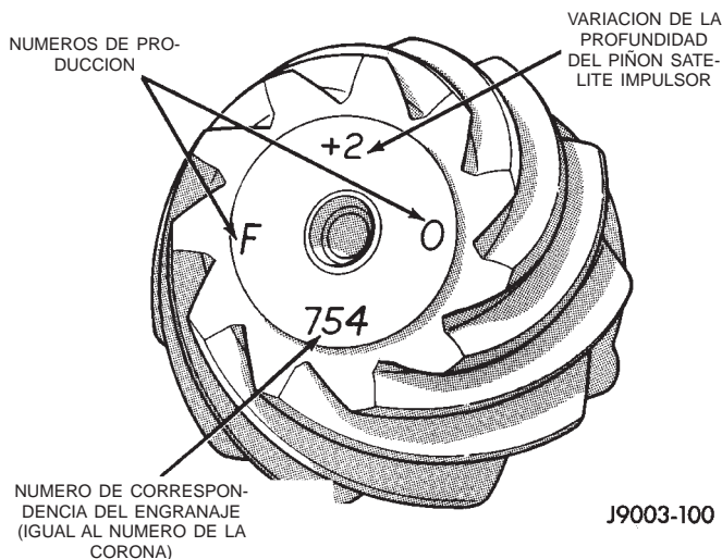
Fig. 64 Números de identificación del piñón satélite
