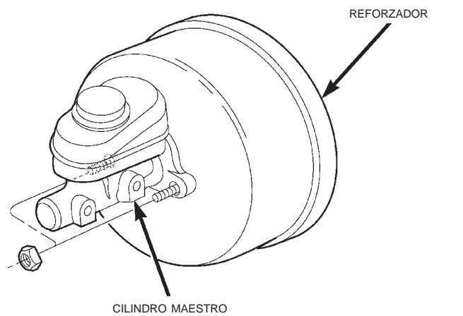
Fig. 21 Cilindro maestro
