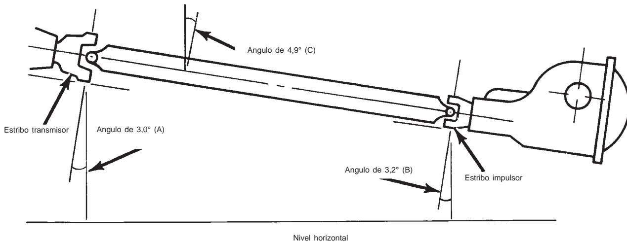
Fig. 10 Medición del ángulo (de impulsión) trasero (B)
