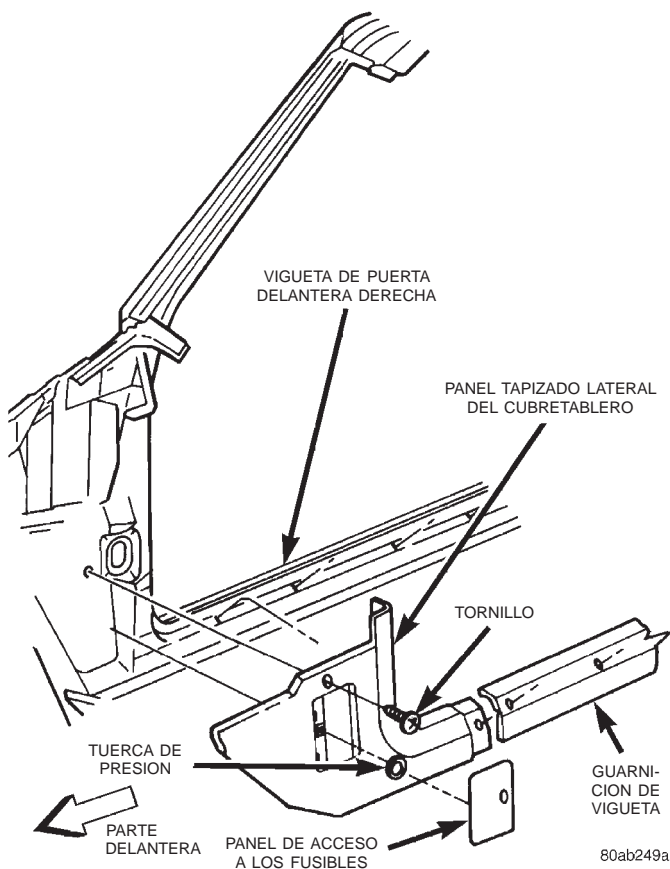
Fig. 6 Desmontaje e instalación de panel tapizado interior lateral del cubretablero derecho
