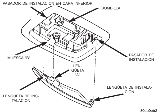
Fig. 10 Óptica de luz de zona de carga
