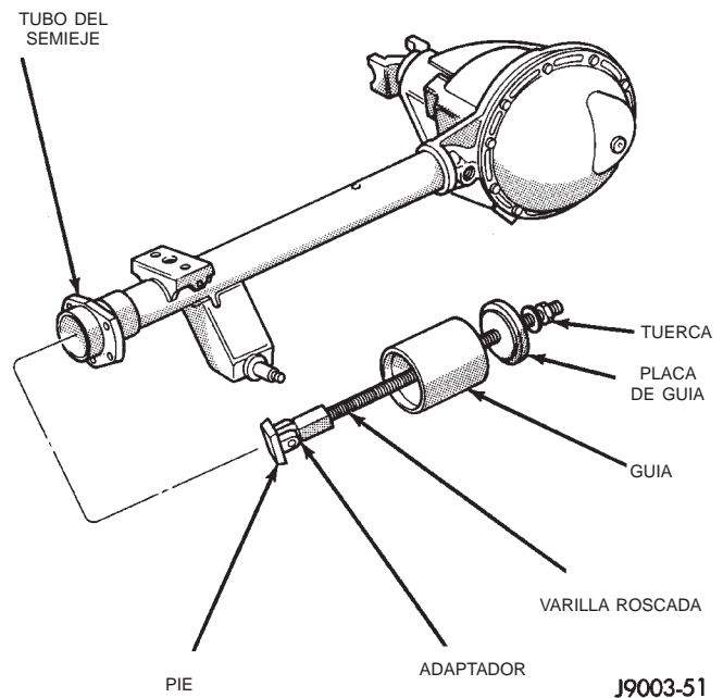
Fig. 21 Extractor de cojinetes del semieje
