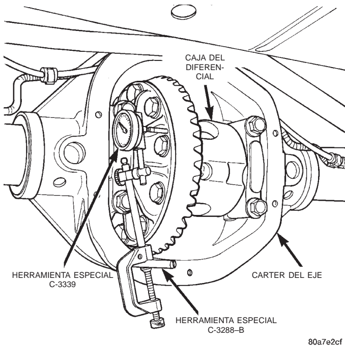
Fig. 54 Medición de juego lateral del diferencial
