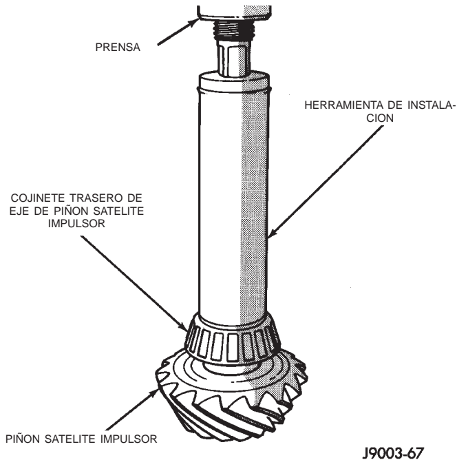
Fig. 43 Instalación de cojinete trasero del eje
