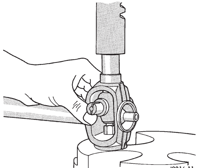
Fig. 28 Presión de tapa de cojinete
