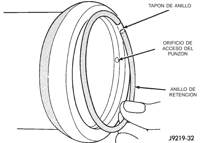
Fig. 5 Instalación del anillo de retención
