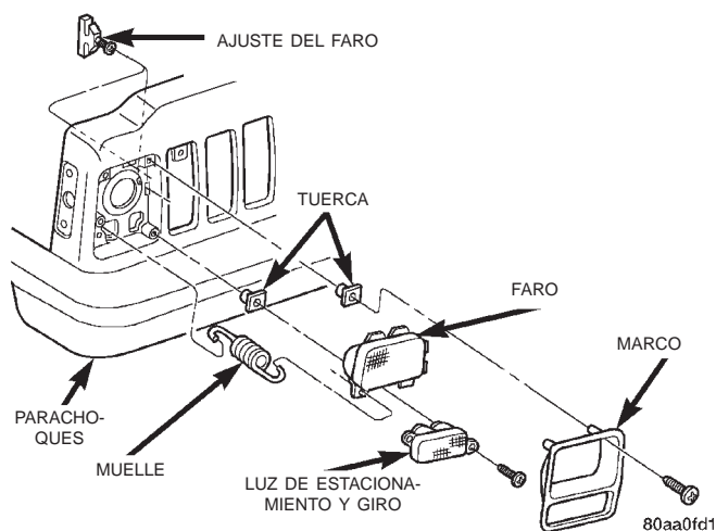
Fig. 1 Marco del faro
