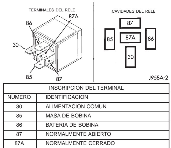
Fig. 10 Relé tipo 1
