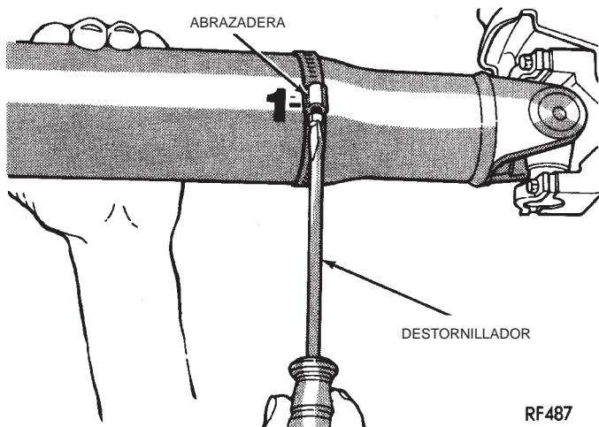
Fig. 5 Tornillo de abrazadera en la posición 1
