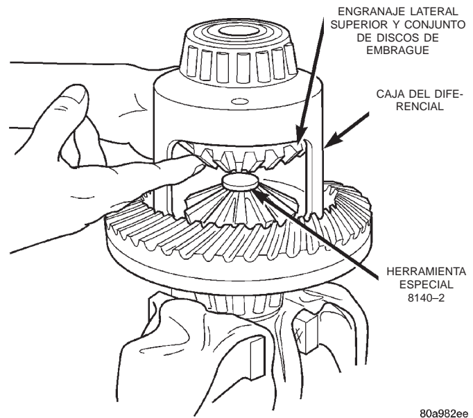
Fig. 50 Instalación de discos de embrague y engranaje lateral superior
