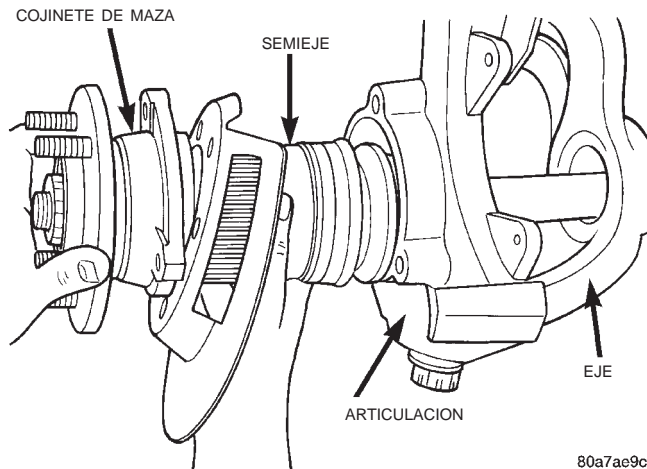
Fig. 12 Conjunto de cojinete de maza y eje
