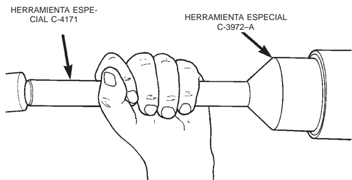
Fig. 8 Instalación de junta del piñón
