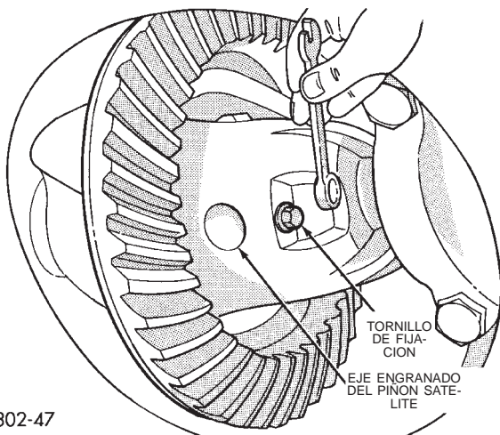
Fig. 8 Tornillo de fijación del eje engranado
