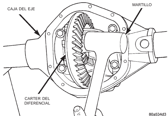
Fig. 73 Asentamiento de los cojinetes laterales falsos de diferencial en el lado de la corona
