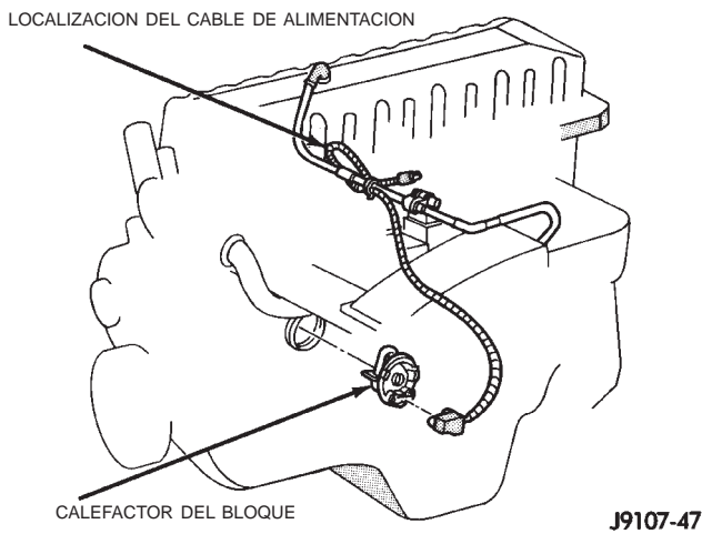
Fig. 40 Calefactor y cable— Motor de 4.0L y 6 cilindros
