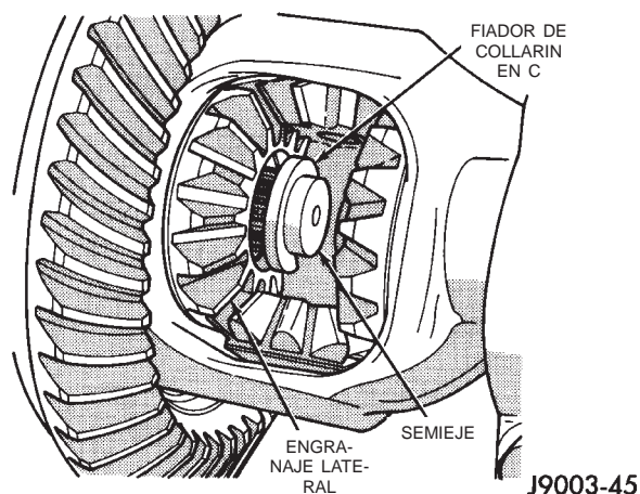
Fig. 20 Fiador de collarín en C del semieje
