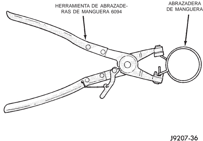
Fig. 5 Herramienta de abrazaderas de manguera
