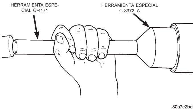
Fig. 15 Instalación de la junta del piñón
