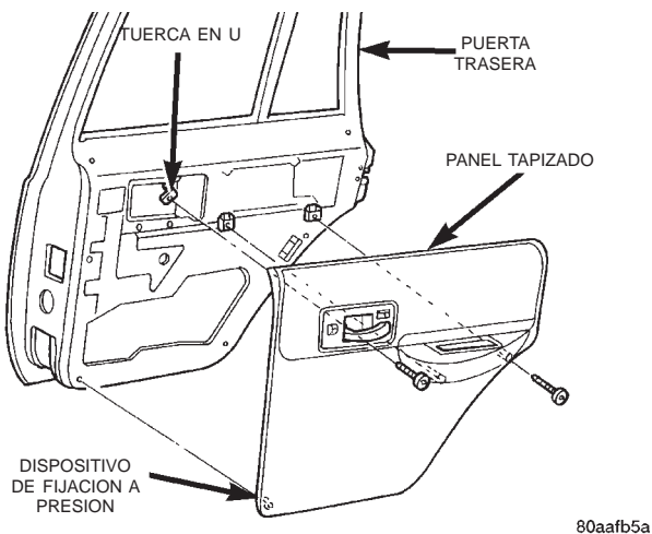
Fig. 6 Desmontaje e instalación de panel tapizado de puerta trasera
