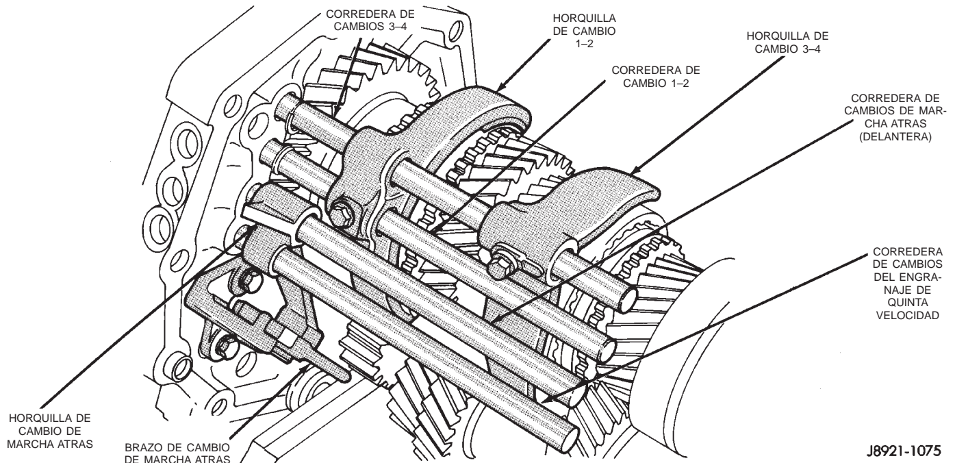
Fig. 67 Identificación de corredera de cambios
