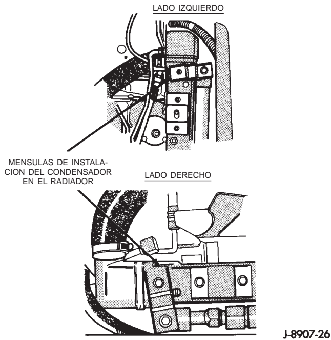
Fig. 29 Ménsulas de instalación del condensador en el radiador
