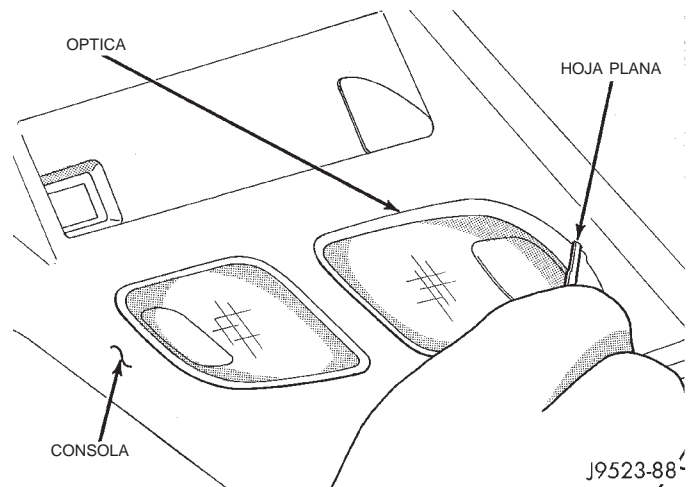
Fig. 10 Bombilla de luz de lectura
