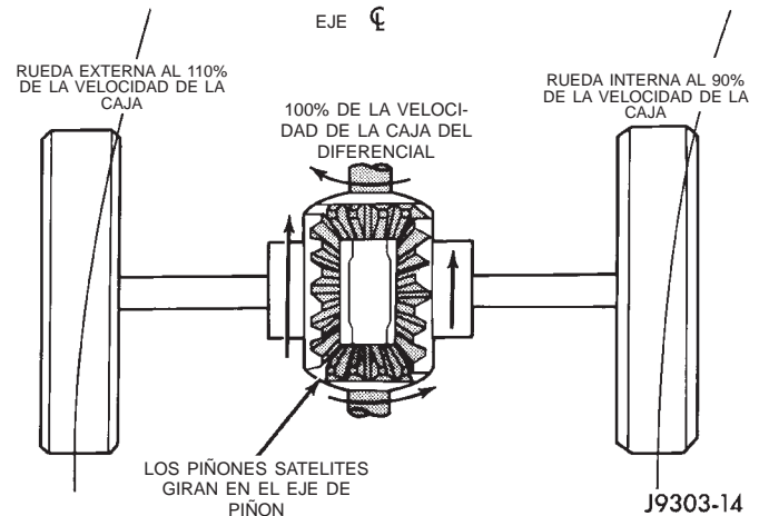
Fig. 4 Funcionamiento del diferencial—En los giros
