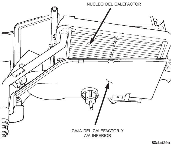
Fig. 62 Desmontaje e instalación del núcleo del calefactor
