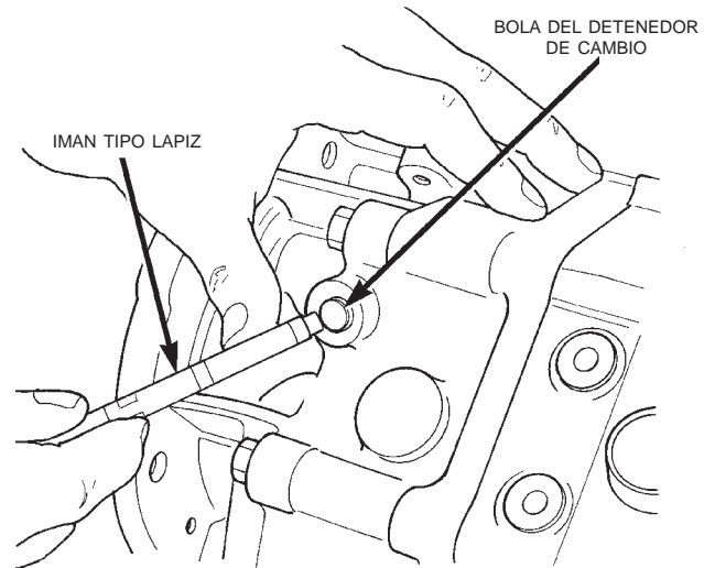
Fig. 44 Instalación de bola del detenedor
