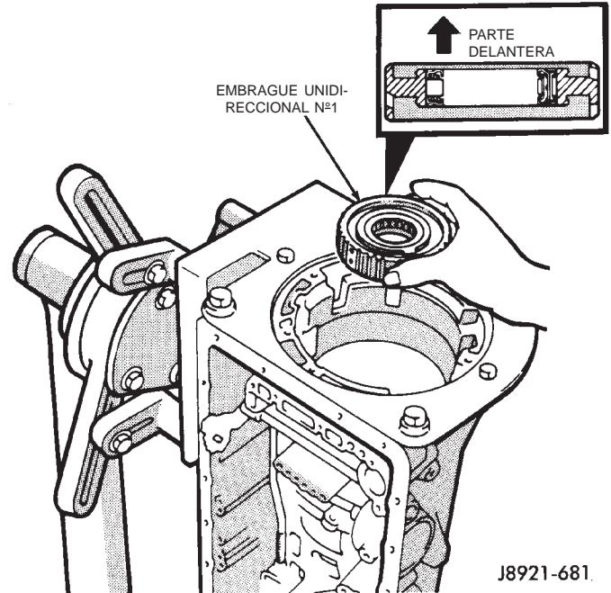
Fig. 137 Instalación del embrague unidireccional n°1
