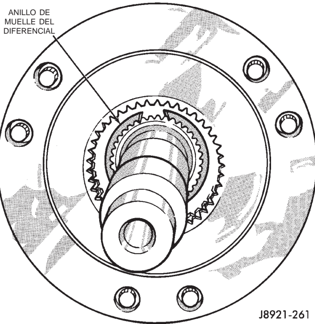
Fig. 73 Instalación del anillo de muelle del diferencial
