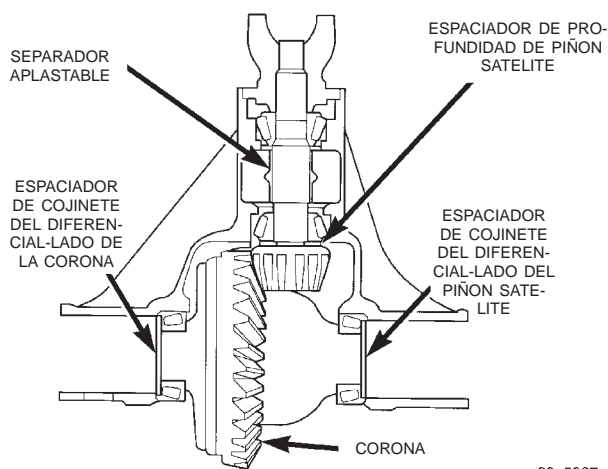
Fig. 70 Posiciones de espaciadores de ajuste del eje
