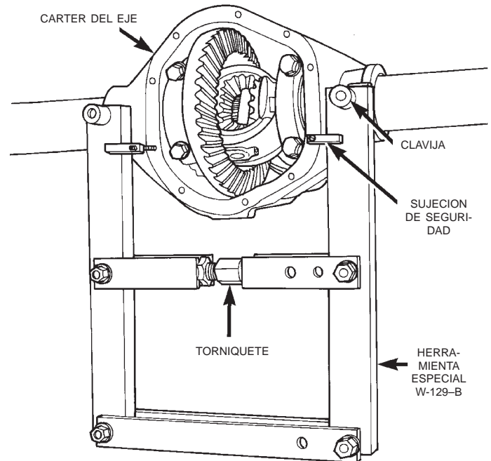
Fig. 28 Instalación de separador del cárter del eje
