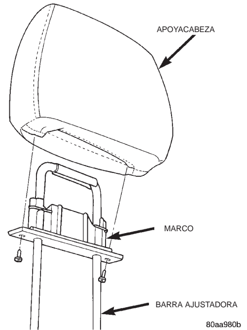
Fig. 5 Apoyacabeza
