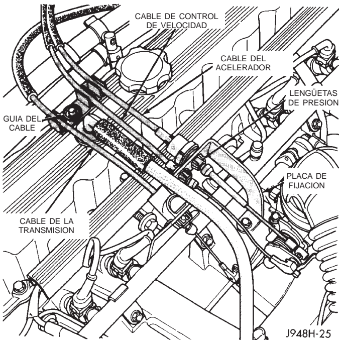
Fig. 5 Lengüetas de presión en la placa de fijación del cable
