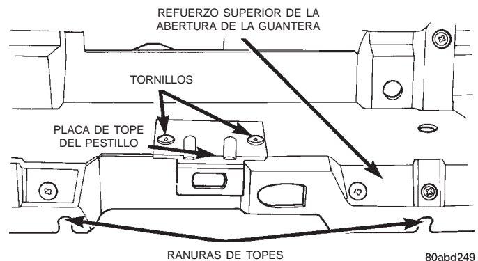
Fig. 20 Desmontaje e instalación de placa de tope del pestillo de la guantera
