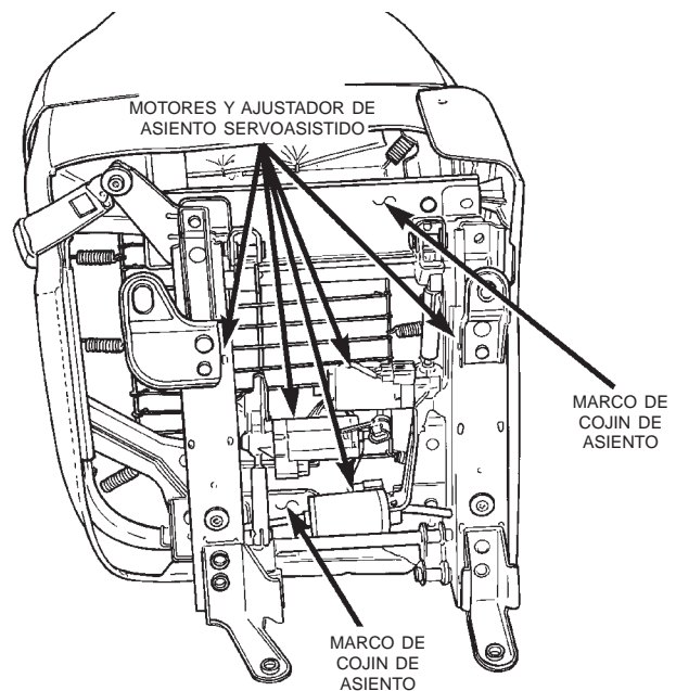
Fig. 4 Desmontaje e instalación de asiento servoasistido
