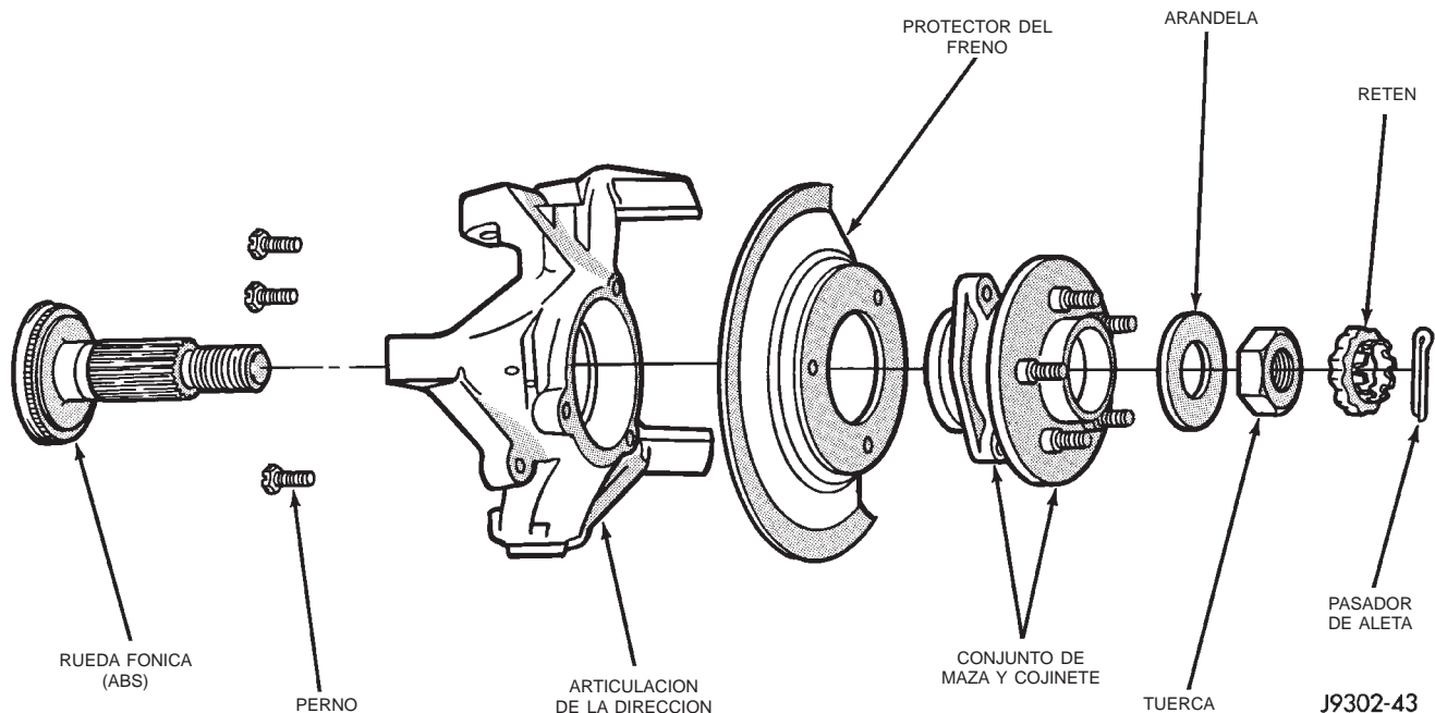
Fig. 10 Maza, articulación y semieje
