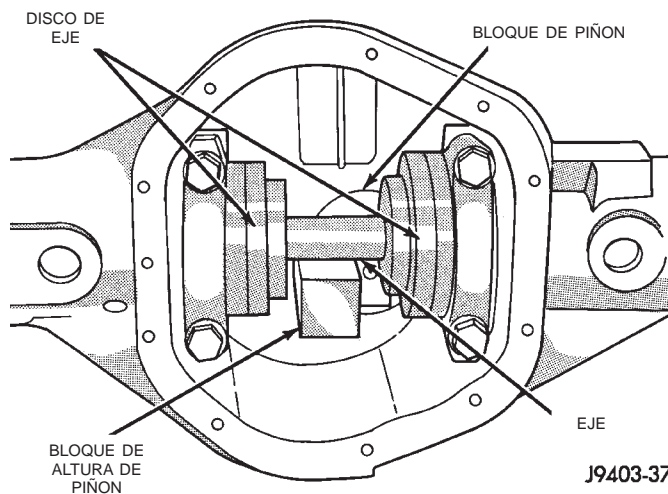
Fig. 68 Herramientas de calibración en el cárter—Característico
