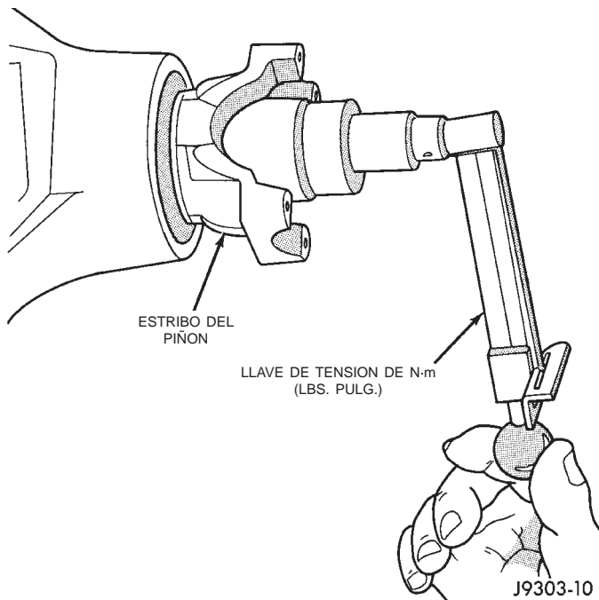
Fig. 18 Comprobación de torsión de rotación del piñón satélite
