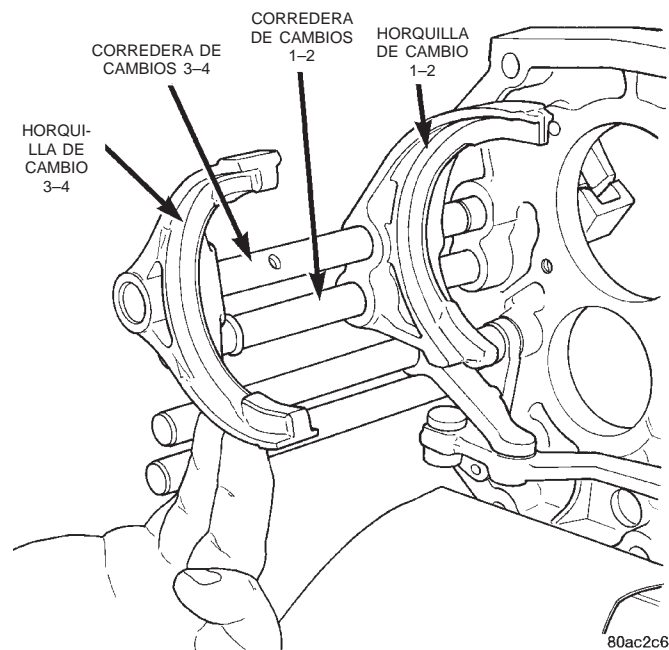
Fig. 86 Instalación de horquilla de cambio 3-4
