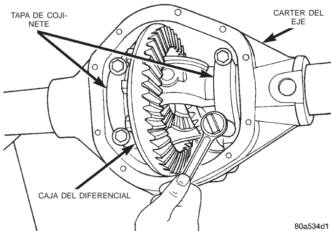
Fig. 51 Apretado de pernos que sujetan las tapas de cojinetes
