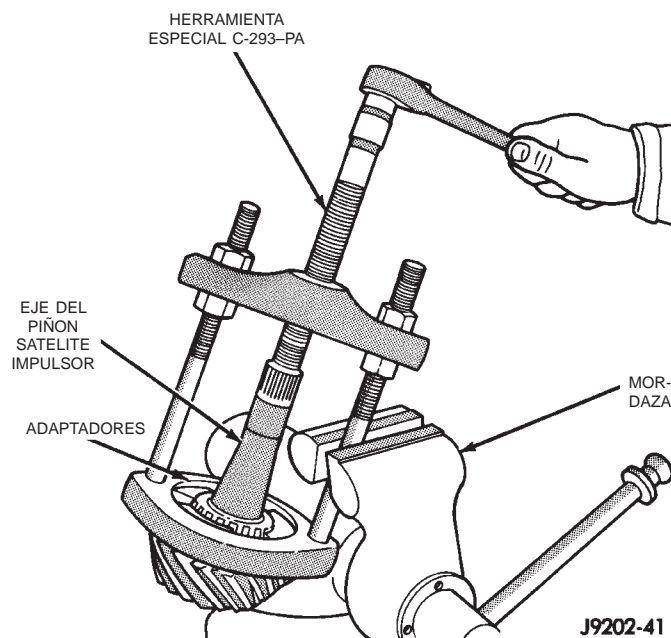
Fig. 32 Desmontaje del cojinete interior
