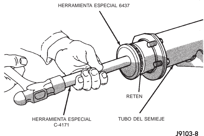
Fig. 22 Instalación de la junta del semieje
