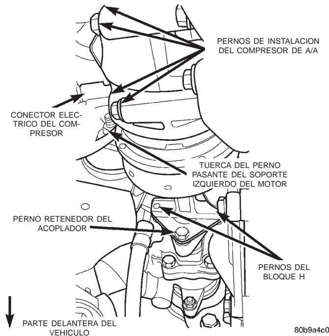
Fig. 12 Posición y orientación del compresor de A/A
