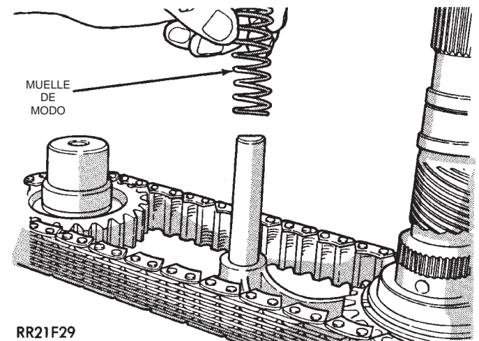
Fig. 21 Desmontaje del muelle de horquilla de modo
