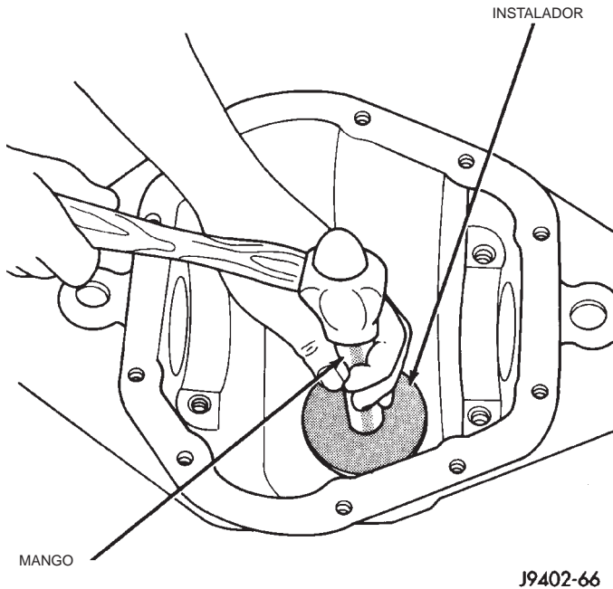
Fig. 33 Instalación de la cubeta del cojinete trasero del piñón
