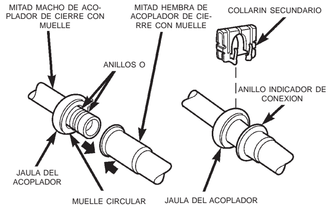
Fig. 5 Acoplador de cierre con muelle - Característico
