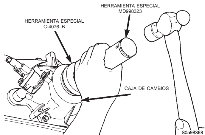
Fig. 78 Instalación de la junta trasera
