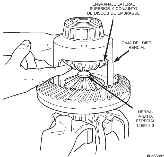
Fig. 63 Instalación de discos de embrague y engranaje lateral superior
