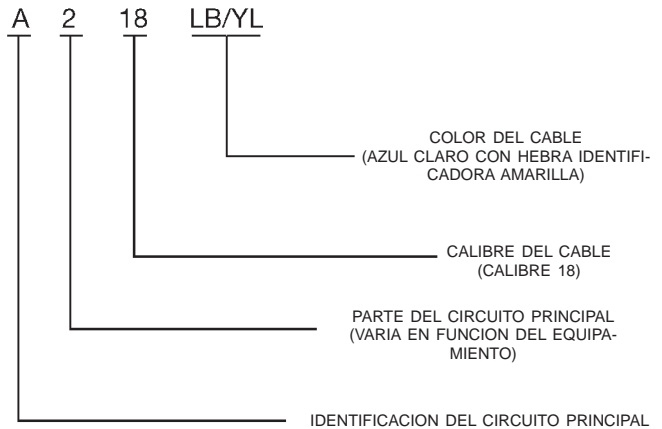
Fig. 1 Identificación de códigos de cables
