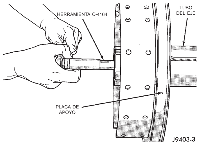
Fig. 57 Herramienta de ajustador roscado
