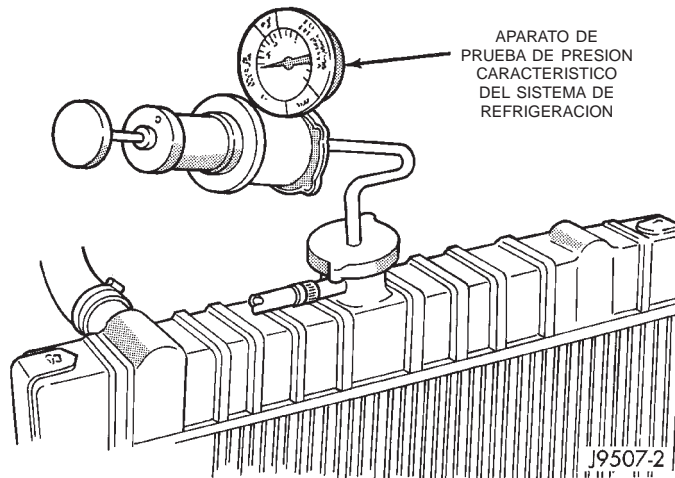
Fig. 12 Sistema de presurización—Característico
