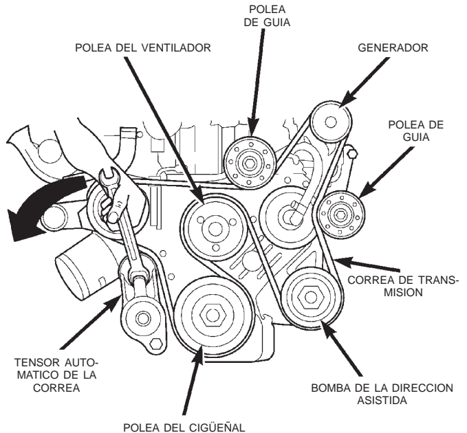
Fig. 8 Conjunto de tensor automático de correa
