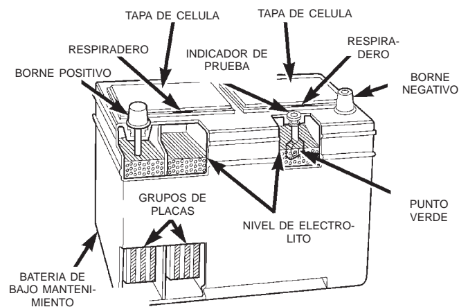
Fig. 1 Batería de bajo mantenimiento - Característica
