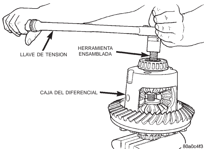
Fig. 57 Apriete de herramienta compresora de muelles Belleville
