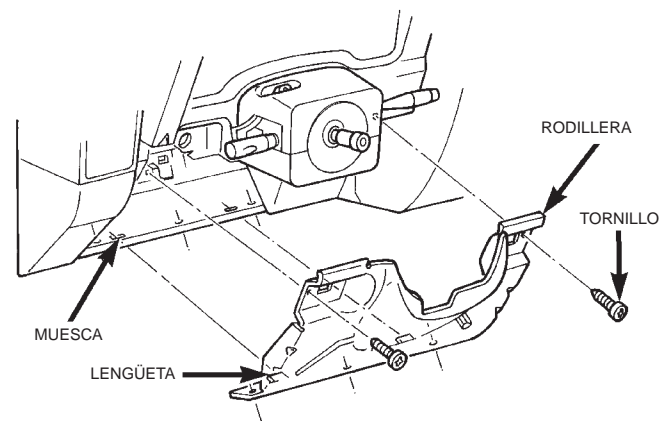
Fig. 5 Desmontaje e instalación de la rodillera
