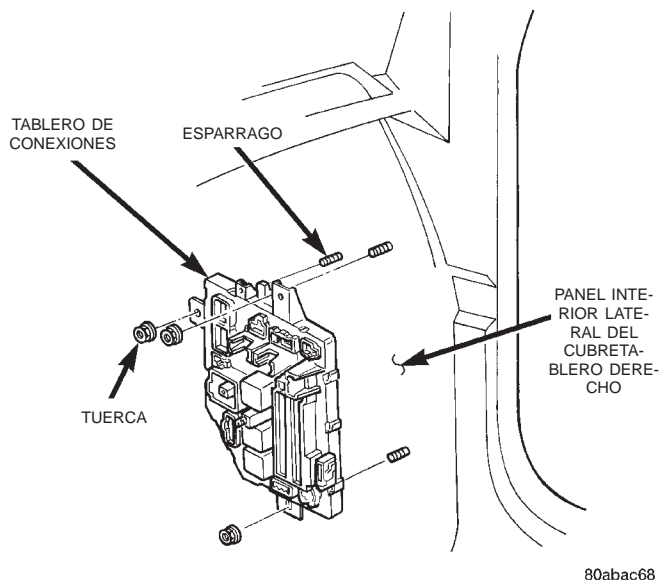
Fig. 7 Desmontaje e instalación del tablero de conexiones
