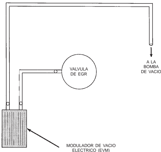
Fig. 1 Recorrido de manguera característico
