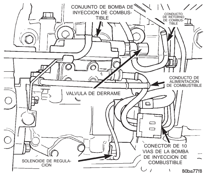
Fig. 22 Válvula de derrame
