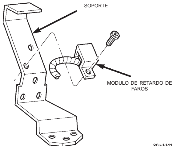
Fig. 1 Módulo de retardo de faros
