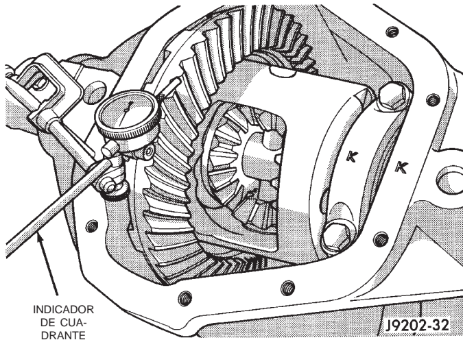
Fig. 59 Medición de holgura entre dientes de la corona
