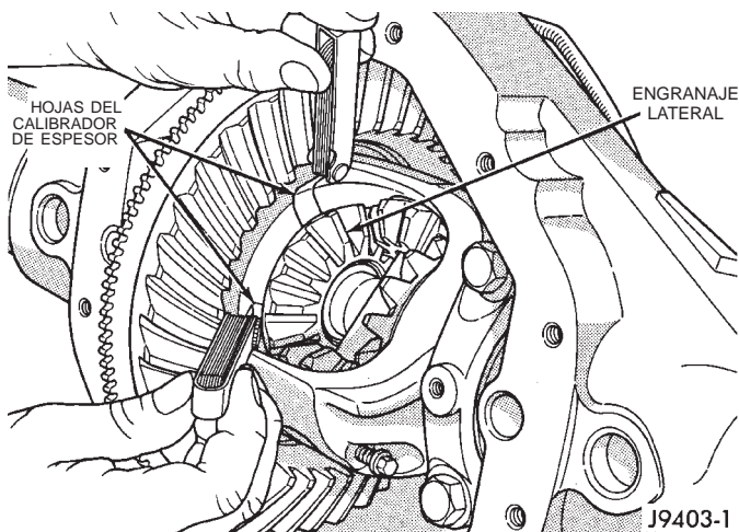
Fig. 60 Medición de luz de engranaje lateral
