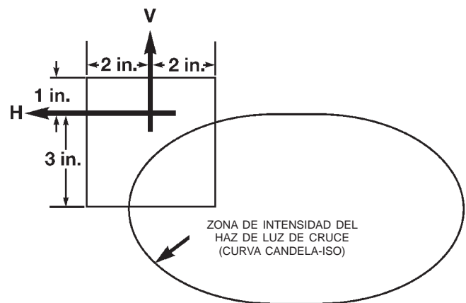
Fig. 1 Pantalla de alineación de faros—Característica
