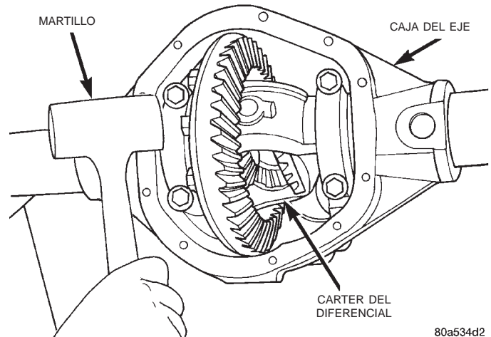
Fig. 72 Asentamiento de los cojinetes laterales falsos de diferencial en el lado del piñón satélite
