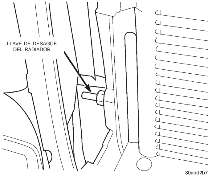
Fig. 32 Llave de desagüe del radiador—Característica
