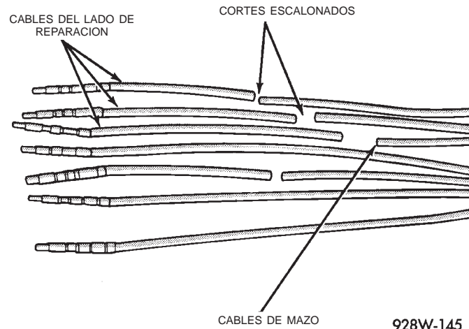
Fig. 18 Corte escalonado de cables
