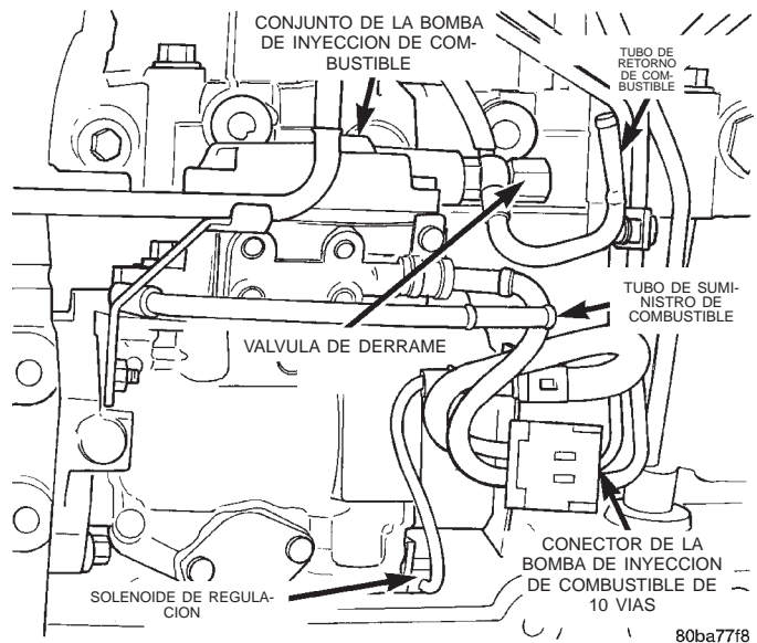
Fig. 3 Bomba de inyección de combustible
