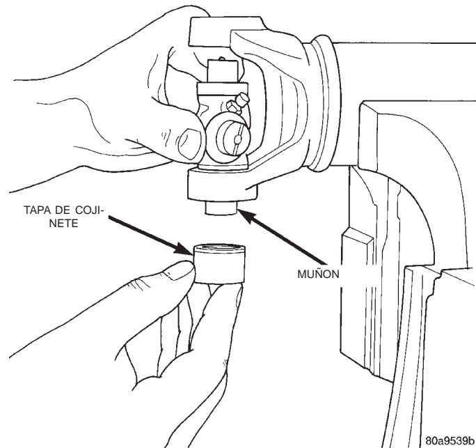
Fig. 21 Instalación del cojinete en el muñón
