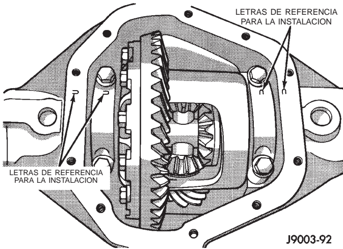
Fig. 23 Identificación de tapa de cojinete
