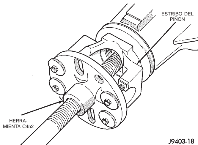
Fig. 24 Desmontaje del estribo del piñón
