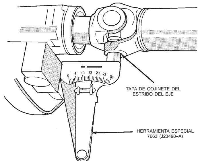
Fig. 9 Medición del ángulo del eje propulsor (C)
