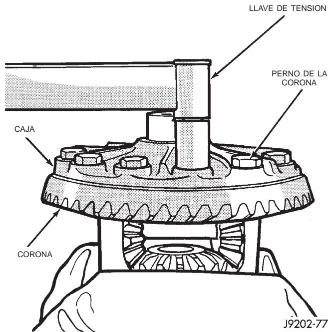
Fig. 27 Instalación de pernos de la corona
