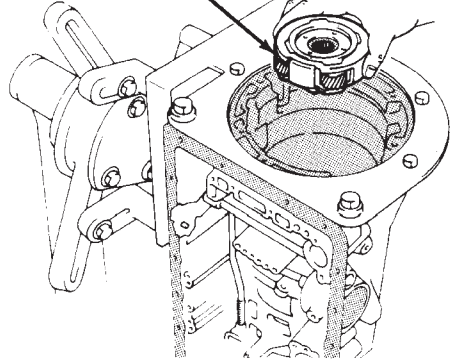
Fig. 110 Desmontaje del anillo de muelle y corona del planetario
