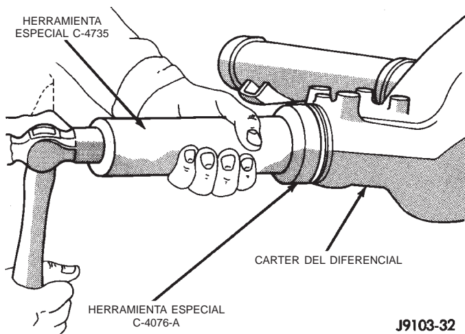
Fig. 32 Instalación de la junta del piñón
