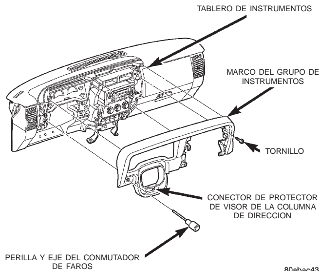
Fig. 10 Desmontaje e instalación del marco del grupo de instrumentos
