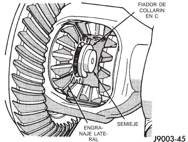
Fig. 9 Fiador de collarín en C del semieje
