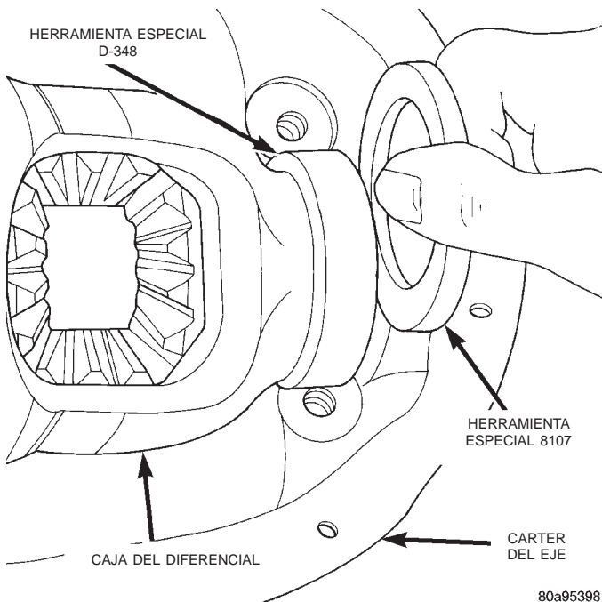
Fig. 71 Inserción de espaciadores de punto inicial
