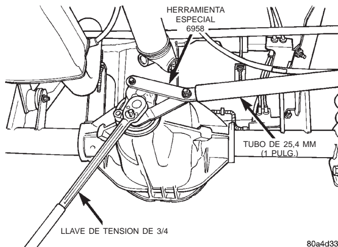
Fig. 11 Apriete de la tuerca del eje del piñón—Característico
