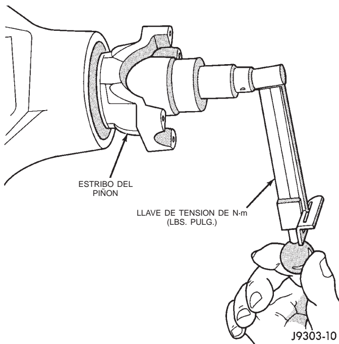
Fig. 16 Comprobación de torsión de rotación del piñón
