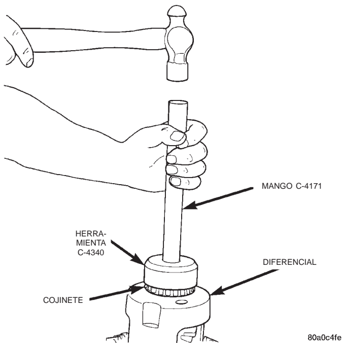
Fig. 21 Instalación de cojinetes laterales del diferencial
