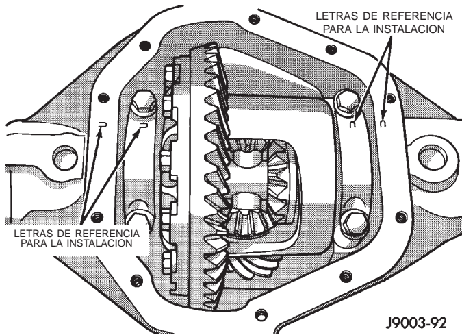
Fig. 29 Letras de referencia de tapas de cojinetes del diferencial
