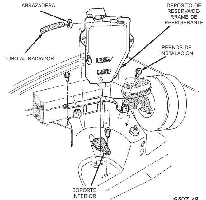
Fig. 3 Depósito de reserva y derrame—Con conducción a la derecha
