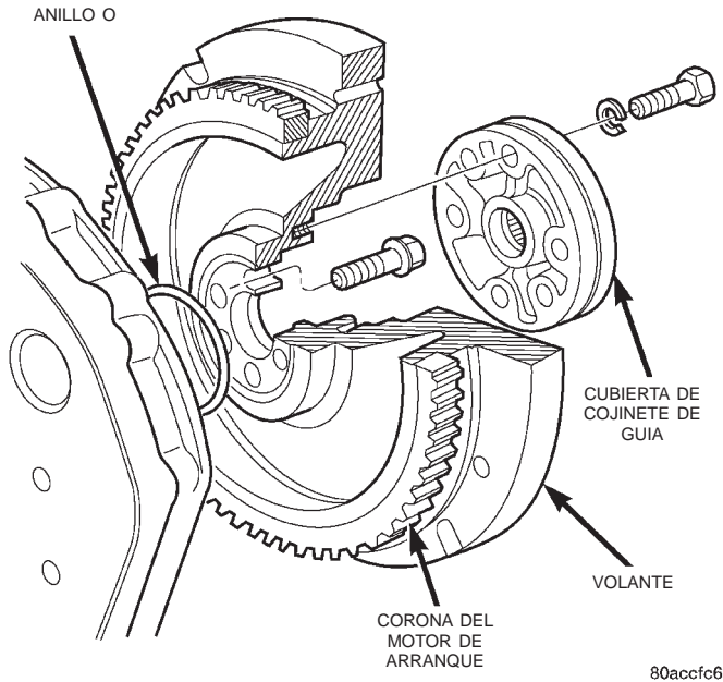
Fig. 9 Instalación del volante (VM diesel)
