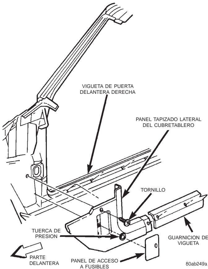
Fig. 9 Desmontaje e instalación del panel tapizado lateral derecho del cubretablero
