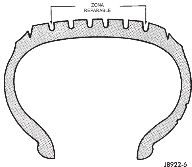
Fig. 11 Zona de reparación del neumático
