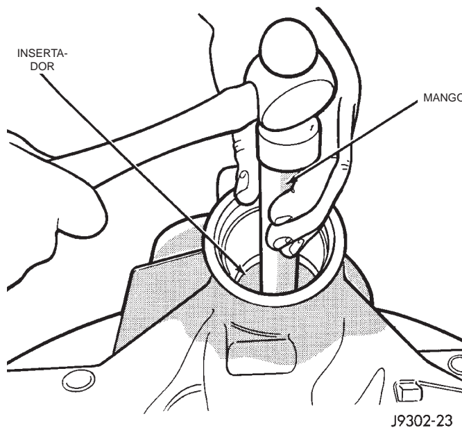
Fig. 27 Desmontaje de la cubeta del cojinete trasero
