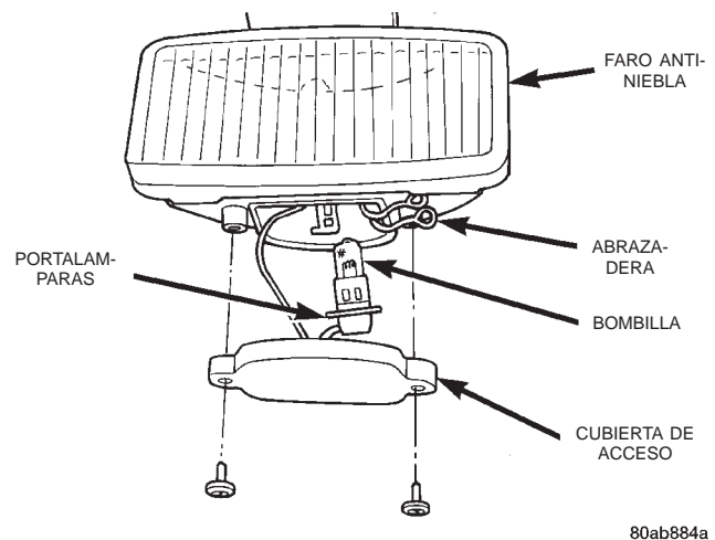
Fig. 2 Componentes del faro antiniebla
