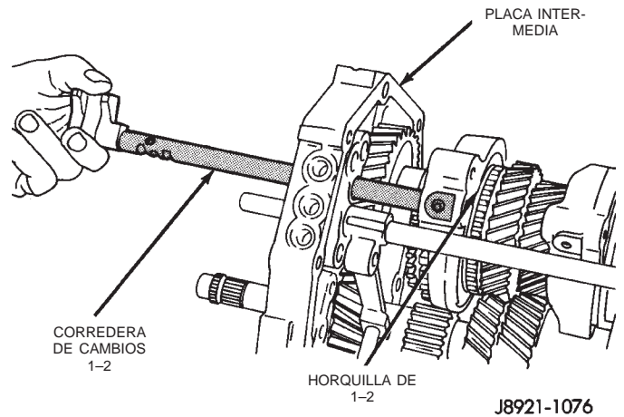
Fig. 74 Desmontaje de corredera de cambios 1-2
