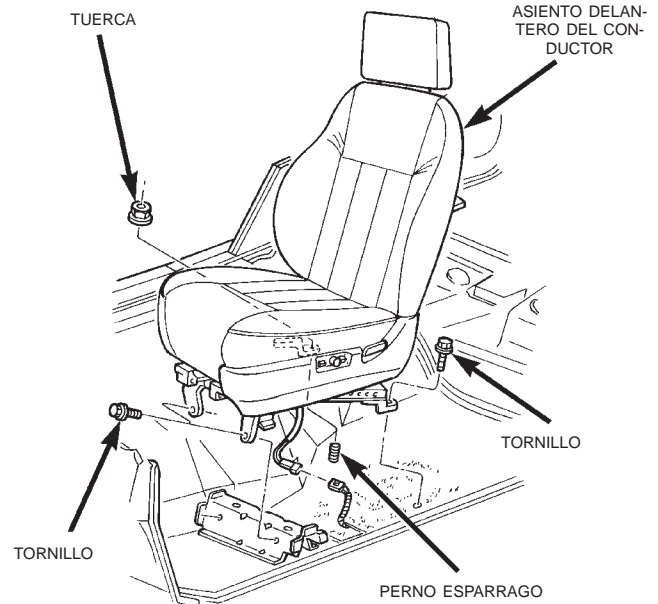
Fig. 4 Desmontaje e instalación de asiento servoasistido
