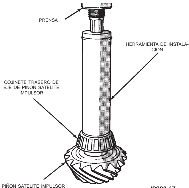
Fig. 33 Instalación de cojinete trasero del eje
