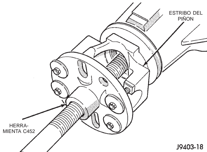
Fig. 13 Desmontaje del estribo
