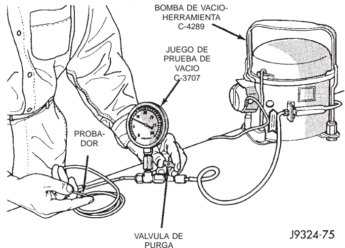
Fig. 8 Ajuste de la válvula de purga de prueba de vacío
