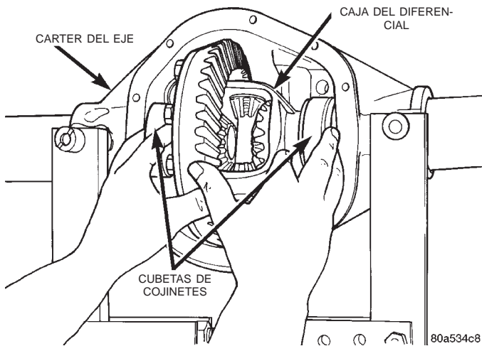
Fig. 27 Desmontaje de caja del diferencial
