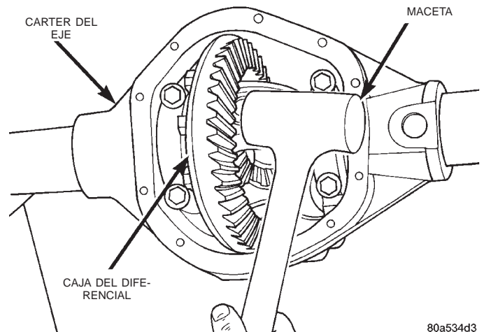
Fig. 53 Calce de cojinete lateral del diferencial en el lado de la corona
