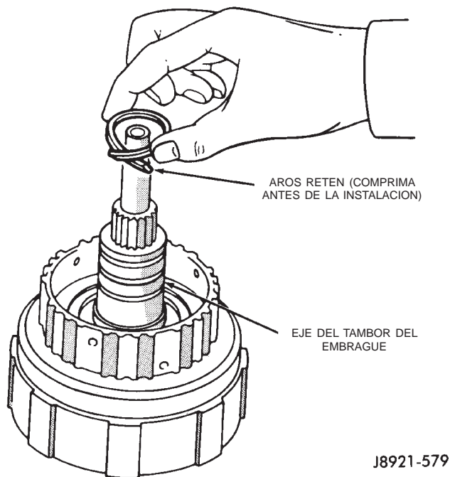
Fig. 252 Instalación de los aros retén del eje del tambor del embrague
