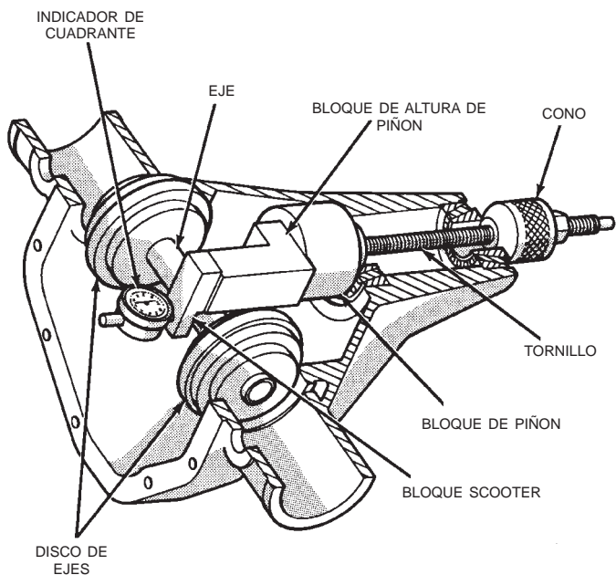
Fig. 46 Herramientas calibradoras de profundidad de piñón satélite—Características
