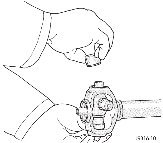
Fig. 27 Instalación de tapa de cojinete
