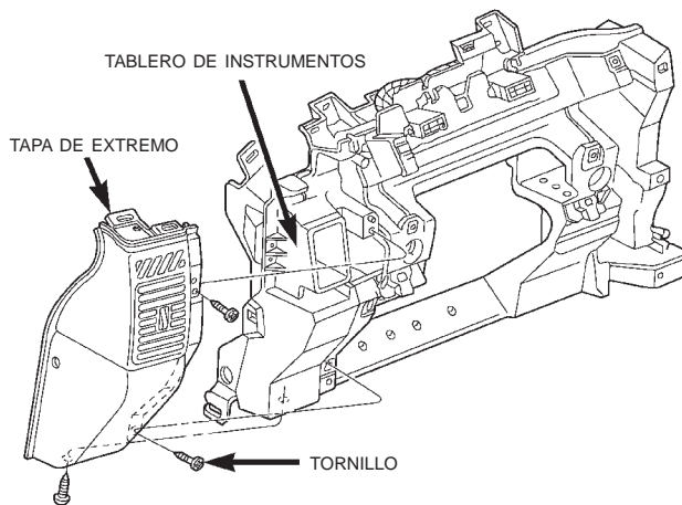
Fig. 21 Desmontaje e instalación de tapa de extremo del tablero de instrumentos
