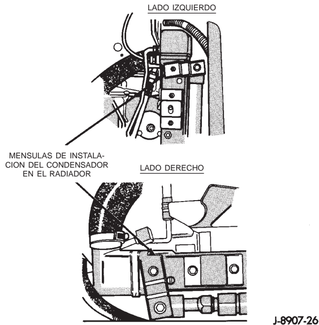
Fig. 34 Ménsulas de instalación del condensador en el radiador—Motor 4.0L
