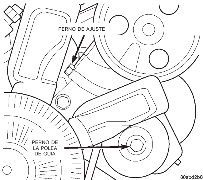
Fig. 47 Soporte de la bomba de la dirección asistida y polea de guía
