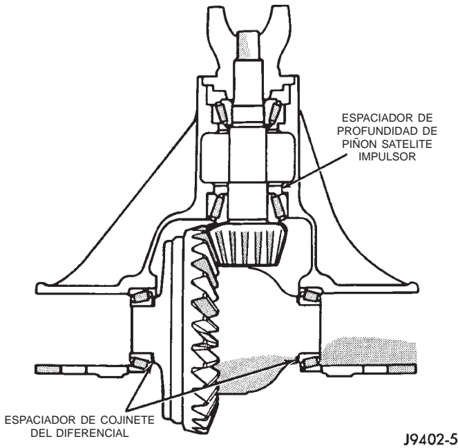
Fig. 50 Posiciones de espaciadores de ajuste del eje
