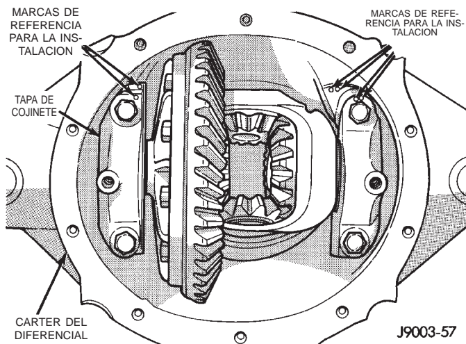
Fig. 17 Marcas de referencia para la instalación
