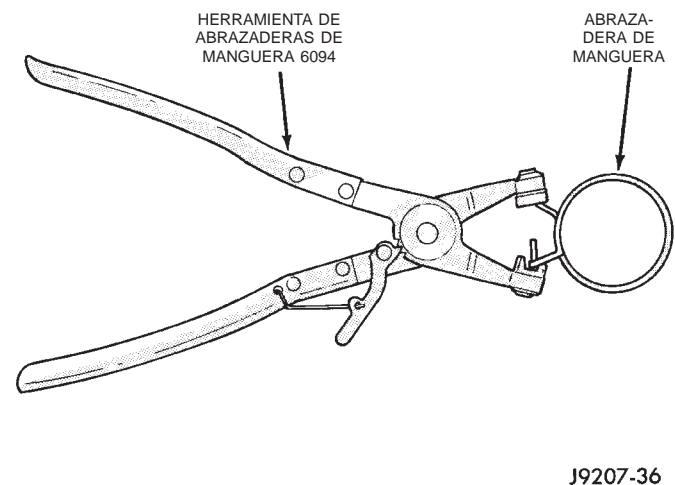
Fig. 6 Herramienta de abrazaderas de manguera—Característico
