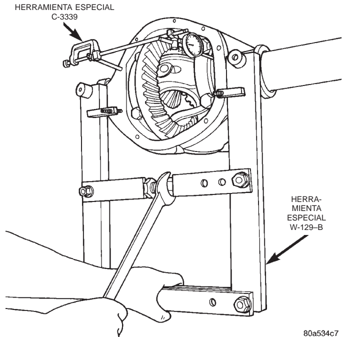
Fig. 26 Separación del cárter del eje
