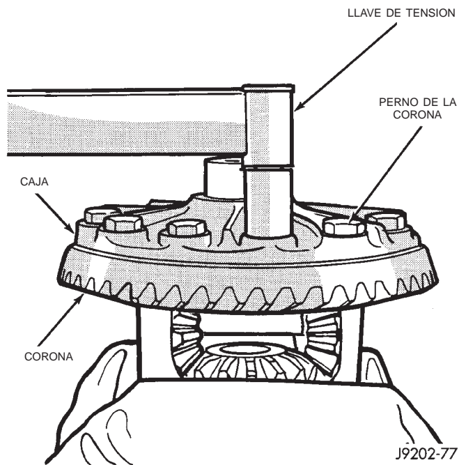
Fig. 33 Instalación de pernos de la corona
