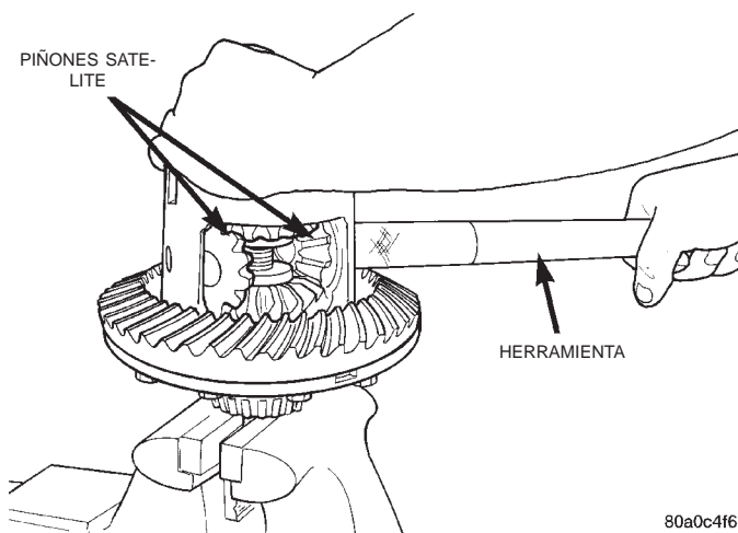
Fig. 59 Desmontaje de piñones satélite
