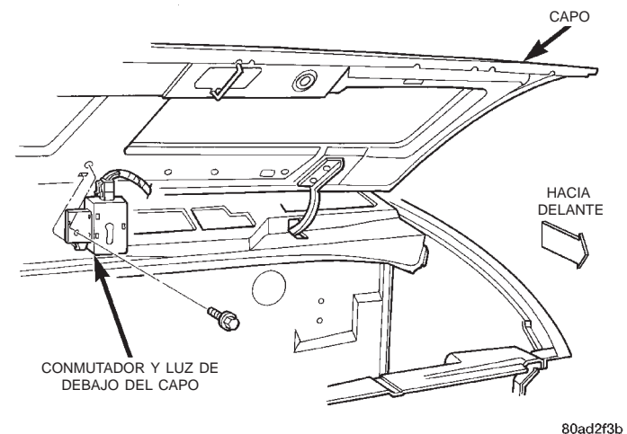
Fig. 8 Luz de debajo del capó
