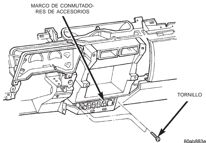
Fig. 8 Desmontaje e instalación del marco de conmutadores de accesorios del tablero de instrumentos
