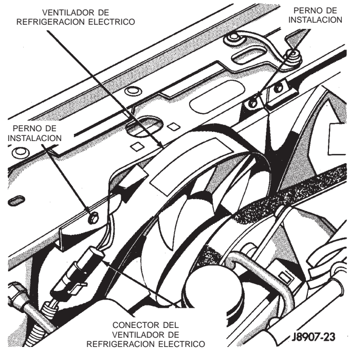
Fig. 38 Ventilador de refrigeración auxiliar— Desmontaje e instalación—Característico
