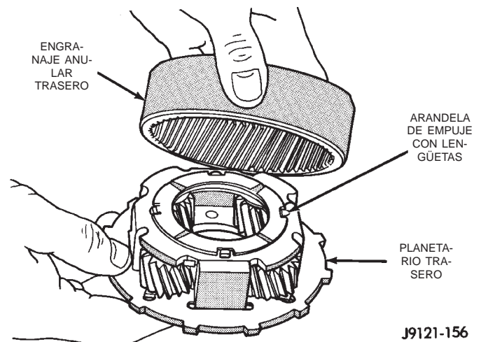
Fig. 152 Ensamblaje del engranaje anular y planetario trasero
