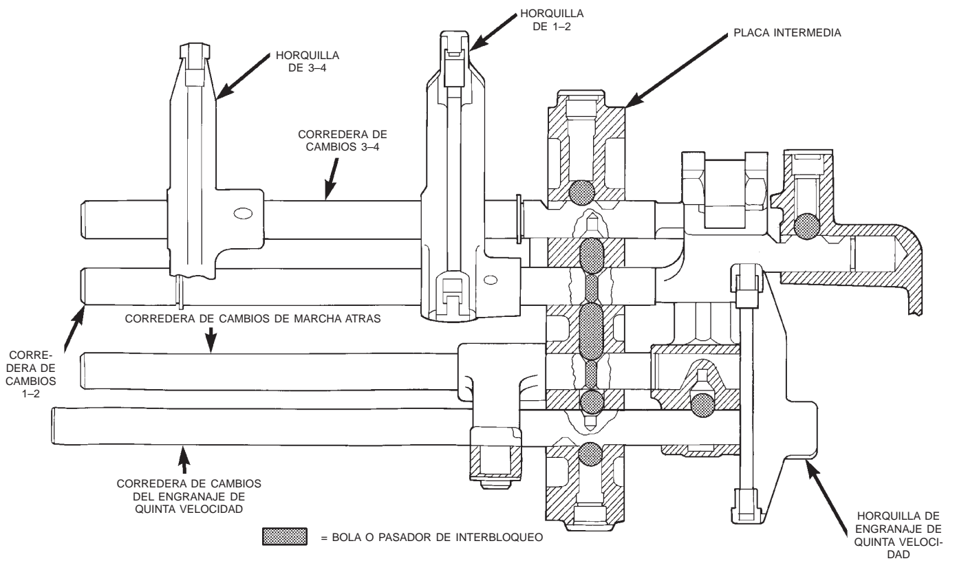
Fig. 75 Componentes de correderas de cambio
