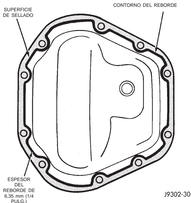
Fig. 43 Tapa de cárter característica con sellante
