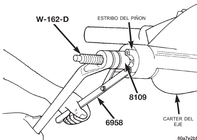
Fig. 8 Instalación del estribo del piñón
