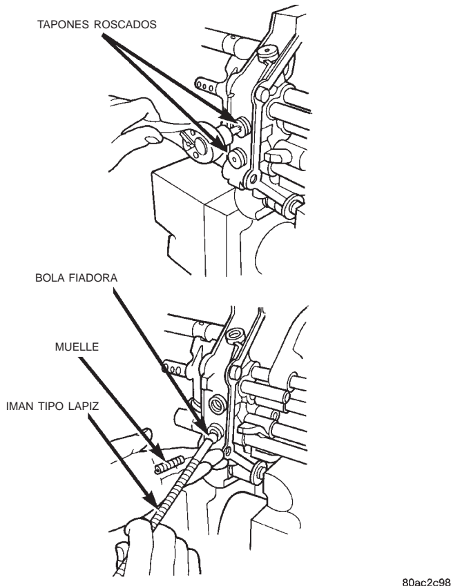
Fig. 66 Desmontaje de bola fiadora y muelle
