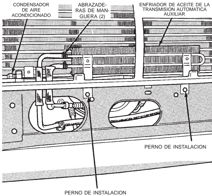
Fig. 16 Enfriador de aceite por aire auxiliar
