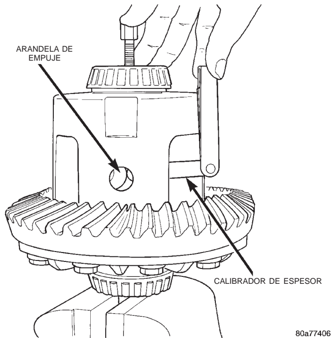
Fig. 45 Desmontaje de arandela de empuje de piñón satélite
