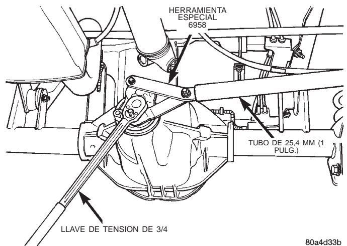
Fig. 46 Apriete de la tuerca del piñón – Característico
