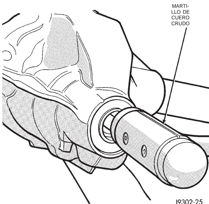
Fig. 25 Desmontaje del piñón satélite
