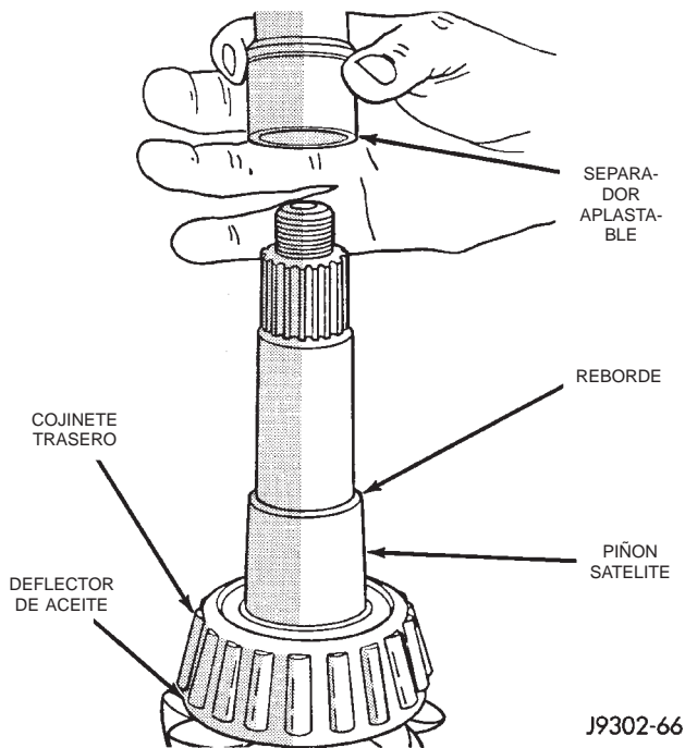
Fig. 28 Separador aplastable
