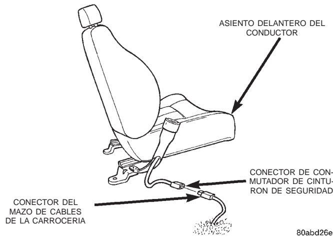
Fig. 3 Conector de conmutador de cinturón de seguridad del conductor
