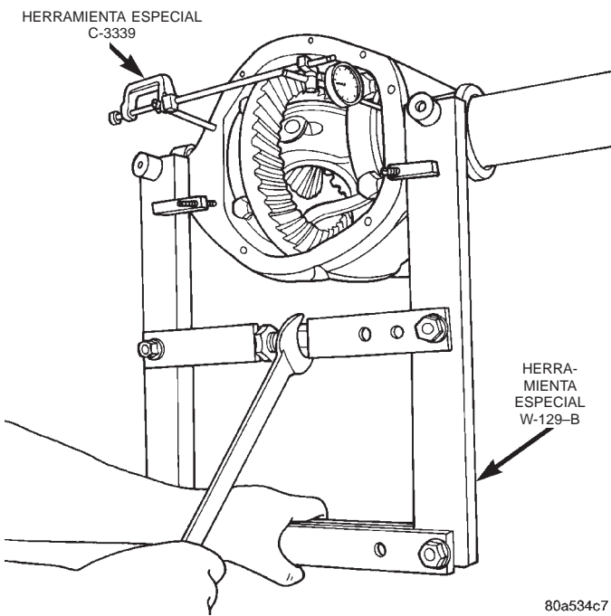
Fig. 19 Separación del cárter del eje
