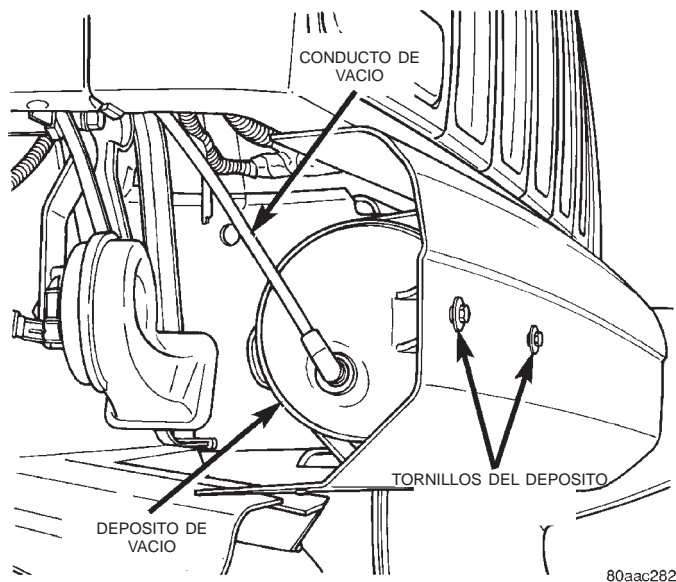
Fig. 7 Desmontaje e instalación del depósito de vacío
