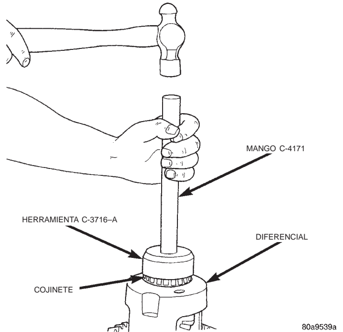
Fig. 31 Instalación de cojinetes laterales del diferencial
