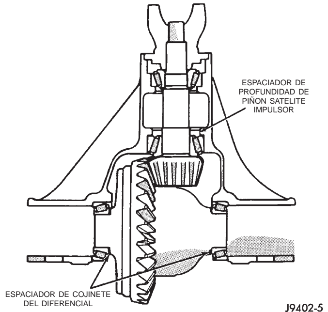
Fig. 45 Emplazamientos de espaciadores
