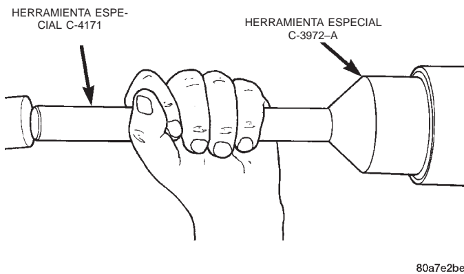
Fig. 7 Instalación de junta del piñón
