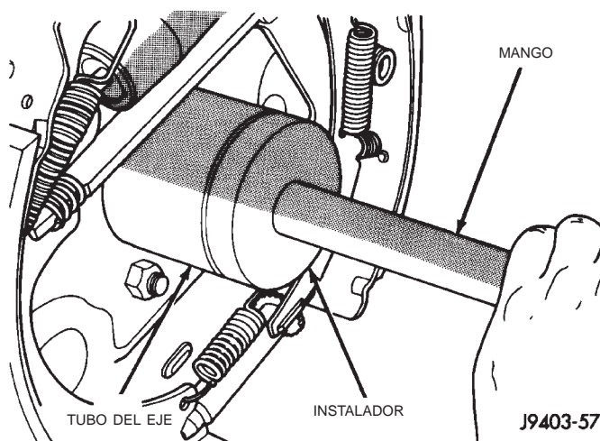
Fig. 12 Instalación de la junta del eje y el cojinete
