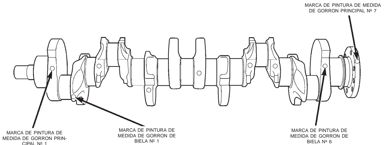
Fig. 20 Localización de pintura de identificación de medida de gorrón de cigüeñal
