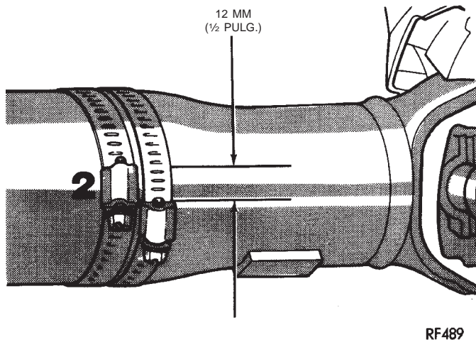
Fig. 7 Tornillos de abrazadera separados
