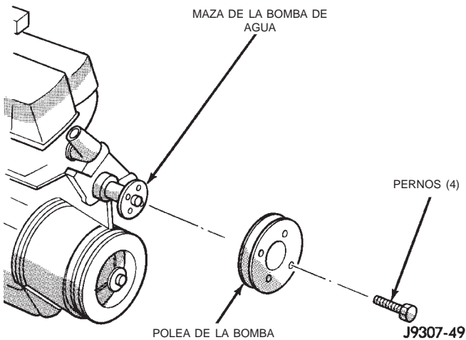
Fig. 23 Pernos de la polea de la bomba de agua
