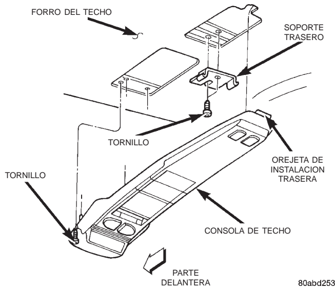
Fig. 3 Desmontaje e instalación de la consola de techo
