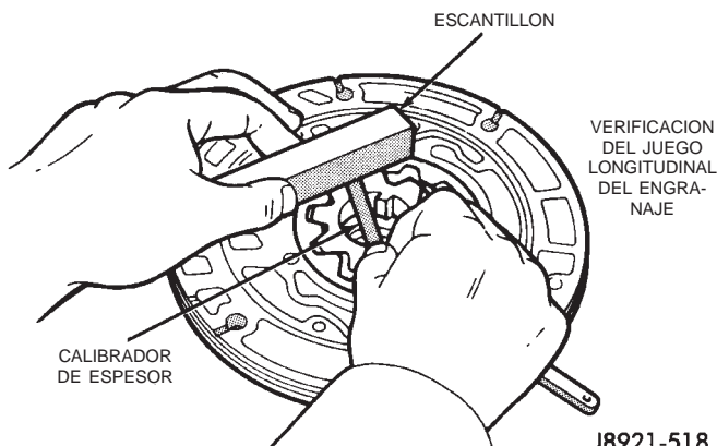
Fig. 189 Verificación de las holguras de los engranajes de la bomba
