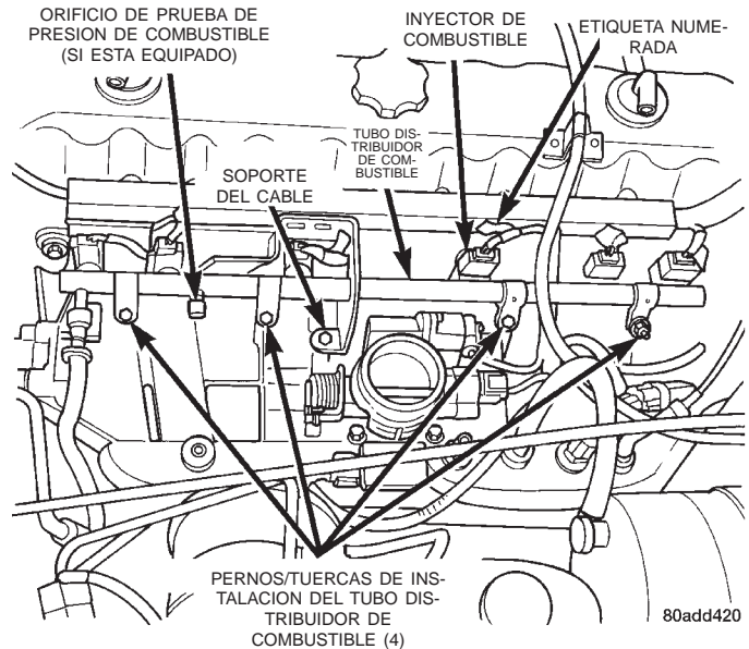
Fig. 30 Montaje del tubo distribuidor de combustible—Motor 4.0L
