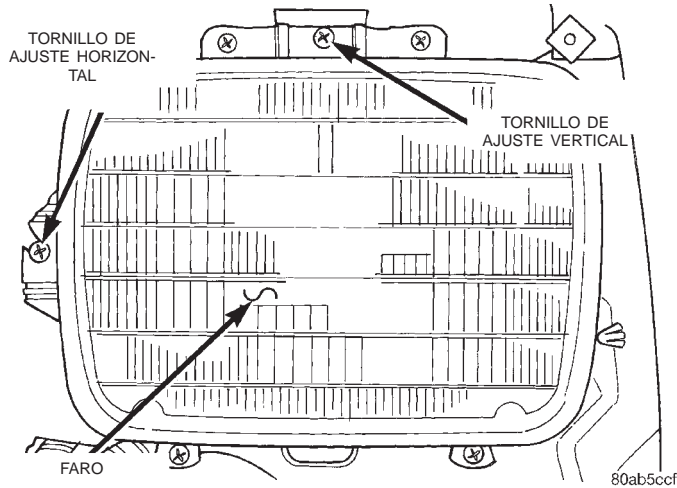
Fig. 3 Tornillos de ajuste del haz de luz de los faros
