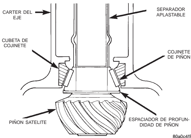
Fig. 52 Emplazamientos de espaciadores
