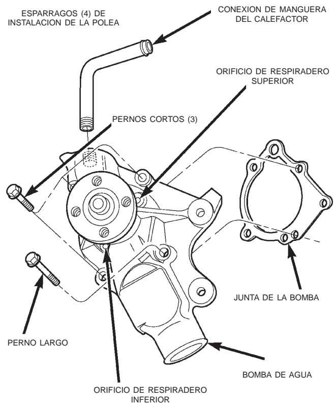
Fig. 22 Desmontaje e instalación de la bomba de agua—Característico
