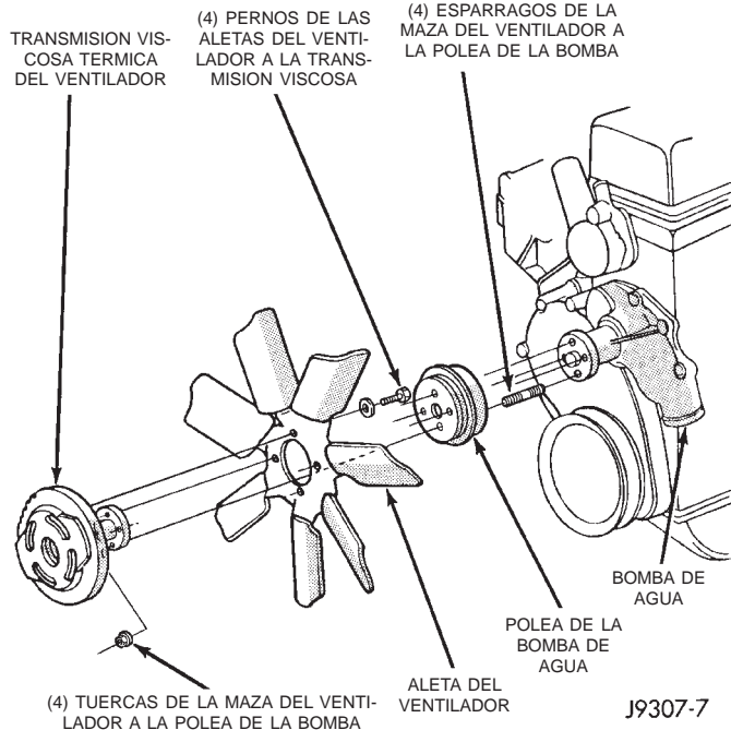
Fig. 49 Ventilador de refrigeración instalado en la bomba de agua
