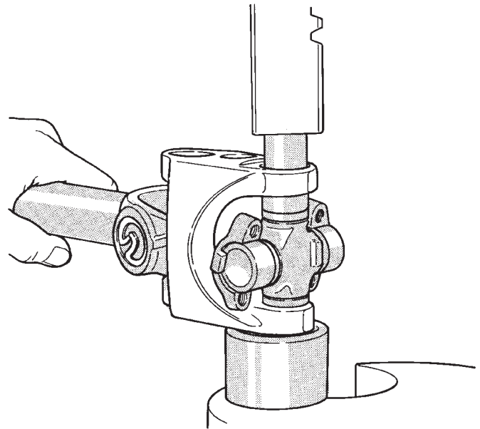
Fig. 23 Extracción del cojinete
