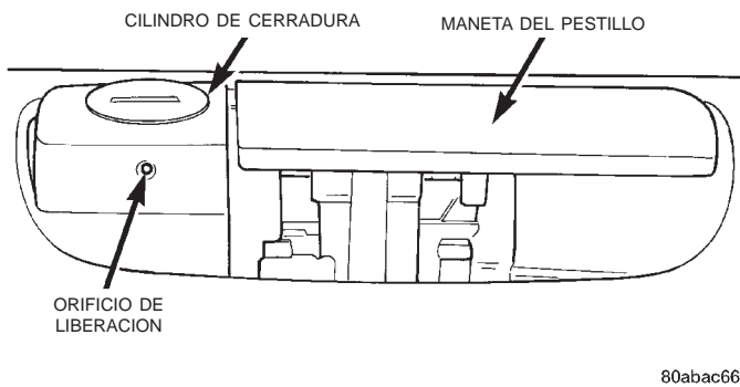
Fig. 19 Desmontaje e instalación del cilindro de cerradura de la guantera
