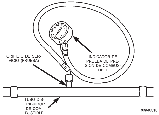
Fig. 7 Indicador de prueba de presión de combustible (Instalación característica del indicador en el orificio de prueba)
