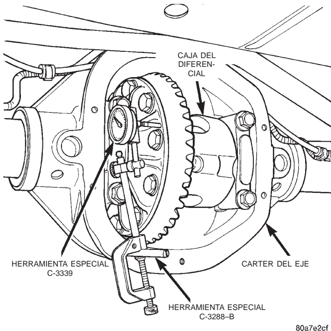
Fig. 74 Medición de juego lateral del diferencial
