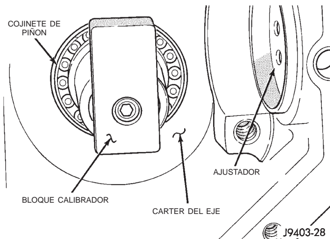
Fig. 54 Bloque calibrador
