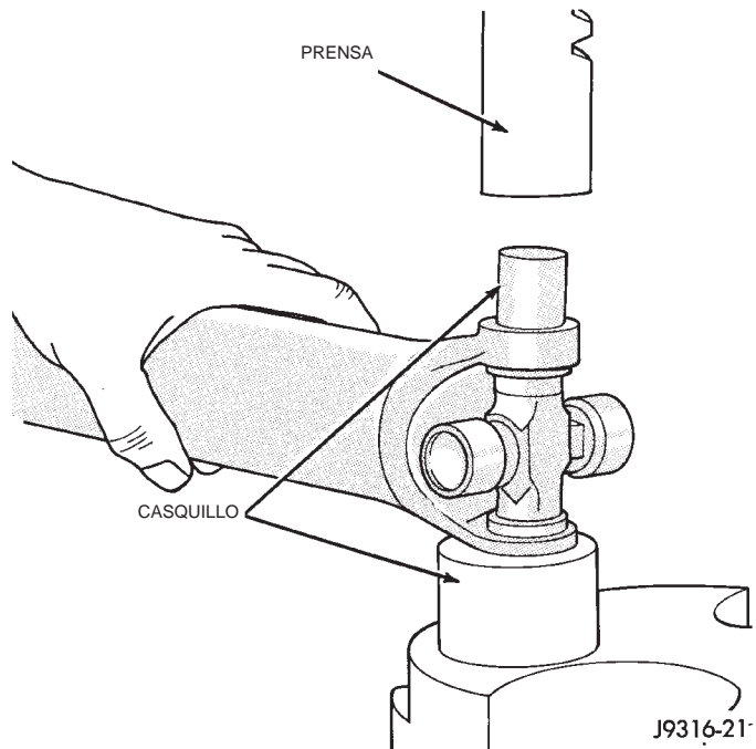
Fig. 18 Extracción del cojinete
