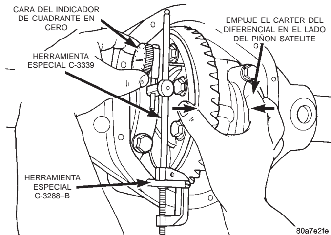
Fig. 75 Sujeción del cárter del diferencial y puesta en cero del indicador de cuadrante
