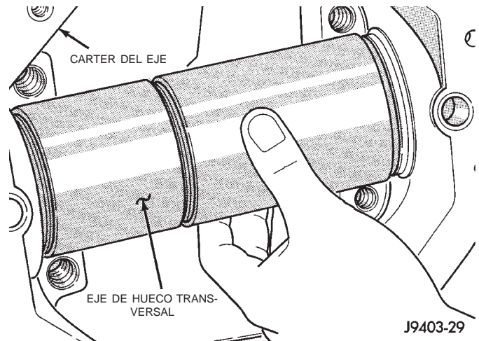
Fig. 55 Eje de hueco transversal
