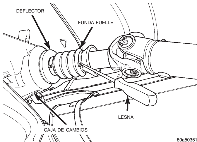
Fig. 14 Abrazadera de funda guardapolvo
