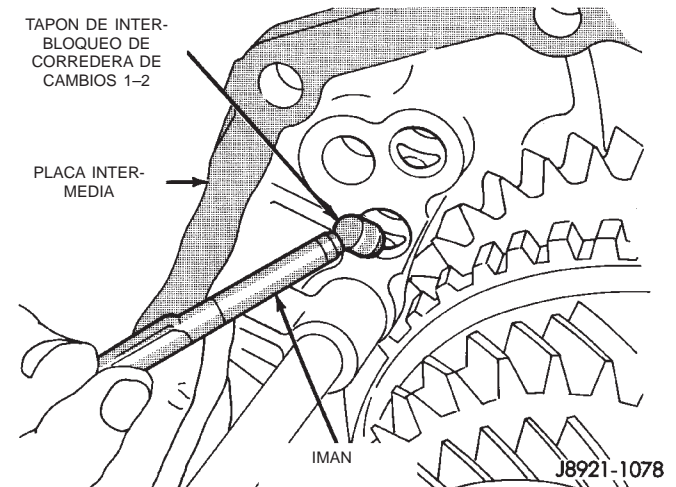
Fig. 85 Instalación de tapón de interbloqueo de corredera de cambios 1-2
