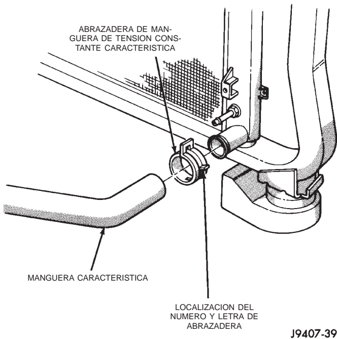
Fig. 7 Localización del número/letra de abrazadera
