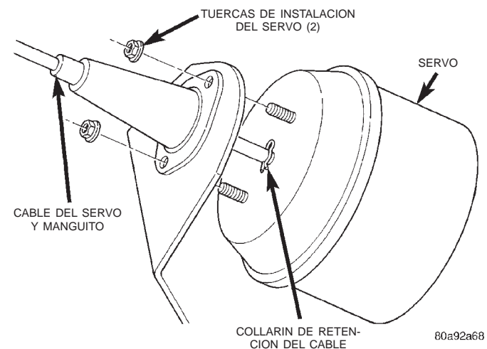
Fig. 2 Desmontaje e instalación del collarín del cable del servo—Característico
