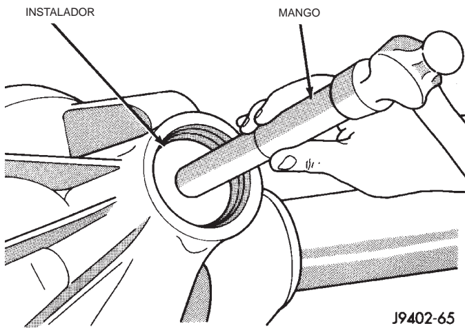
Fig. 34 Instalación de la cubeta del cojinete exterior del piñón
