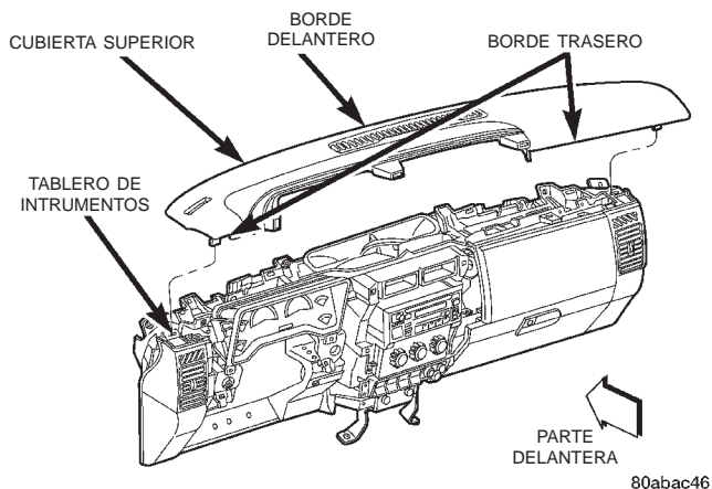
Fig. 15 Desmontaje e instalación de la cubierta superior del tablero de instrumentos
