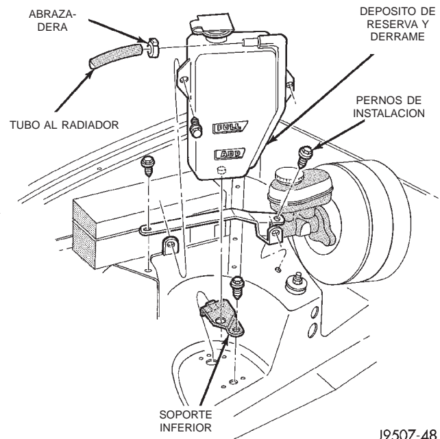
Fig. 18 Depósito de reserva y derrame—Con conducción a la derecha
