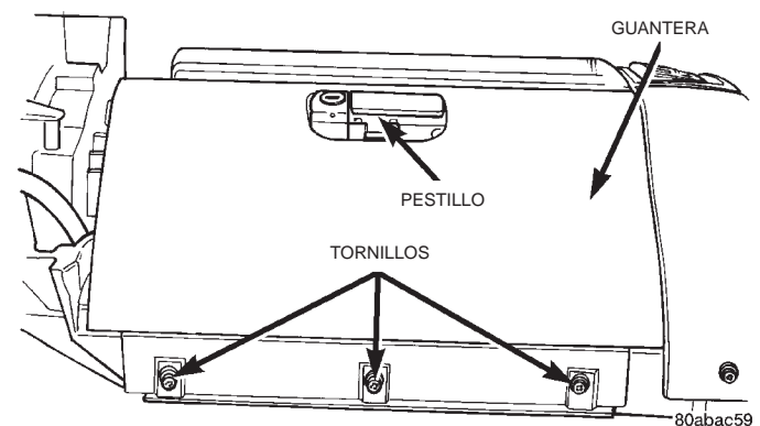
Fig. 17 Desmontaje e instalación de la guantera
