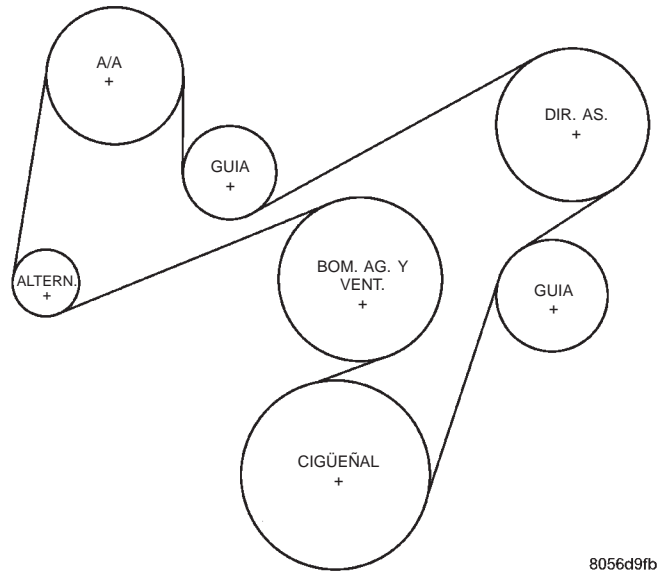
Fig. 41 Modelos con motor 2.5L—Con A/A REEMPLAZO O AJUSTE DE CORREA—VOLANTE A LA IZQUIERDA
