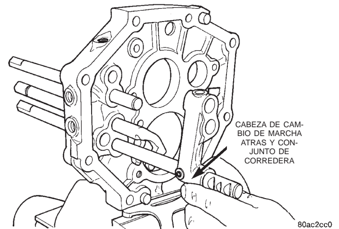
Fig. 69 Desmontaje de cabeza de cambio de marcha atrás y conjunto de corredera
