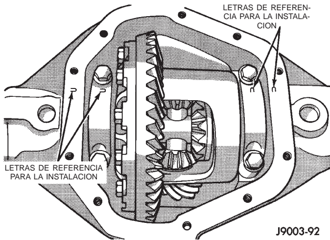
Fig. 16 Identificación de la tapa de cojinete
