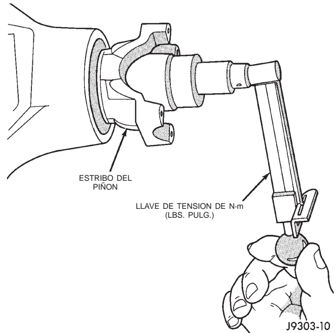
Fig. 9 Comprobación de torsión de rotación del piñón
