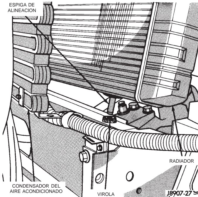
Fig. 31 Espigas de alineación del radiador— Características
