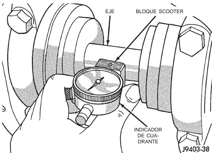
Fig. 69 Medición de profundidad de piñón satélite—Característica
