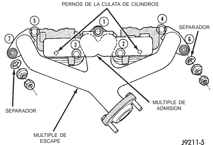
Fig. 29 Desmontaje e instalación de los múltiples de admisión y escape—motor 2.5L
