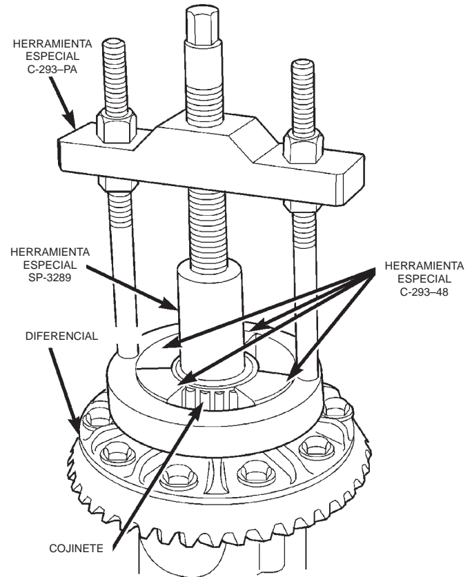
Fig. 20 Desmontaje de cojinete del diferencial
