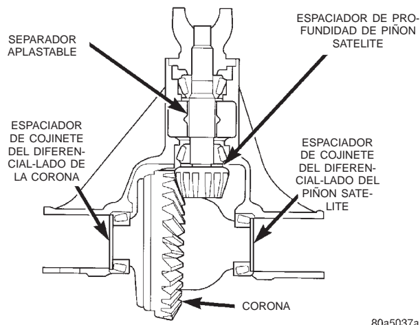
Fig. 65 Emplazamientos de espaciadores
