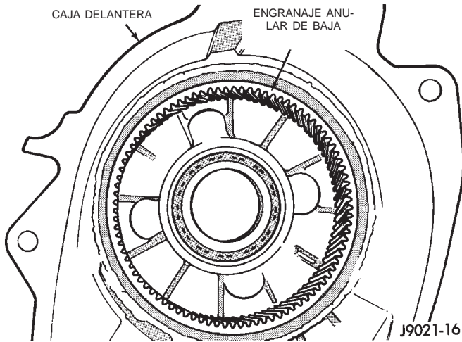
Fig. 86 Engranaje anular de baja
