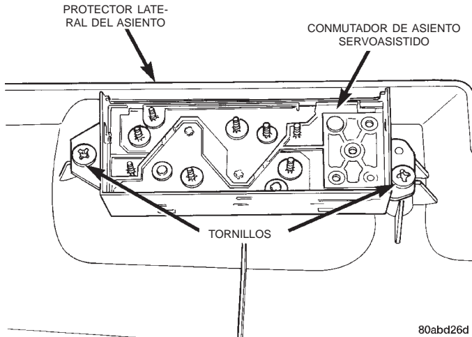
Fig. 2 Desmontaje e instalación del conmutador de asiento servoasistido
