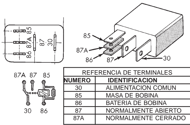
Fig. 30 Terminales de relés de ASD y de la bomba de combustible
