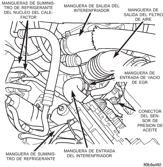
Fig. 17 Compartimiento del motor, Volante a la izquierda — Diesel
