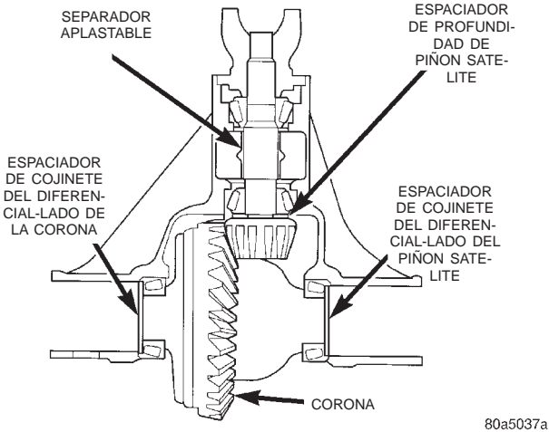
Fig. 1 Emplazamientos de espaciadores
