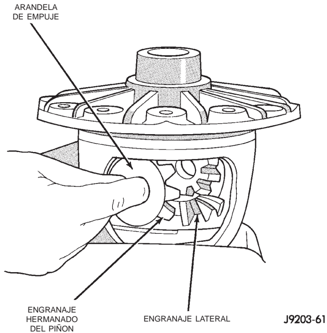
Fig. 50 Desmontaje de engranaje hermanado del piñón
