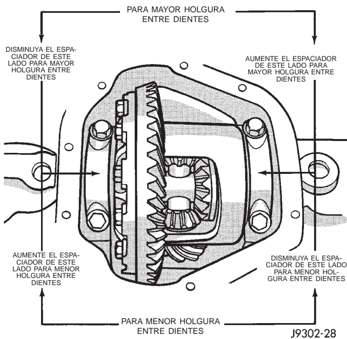
Fig. 60 Ajuste de espaciador de holgura entre dientes
