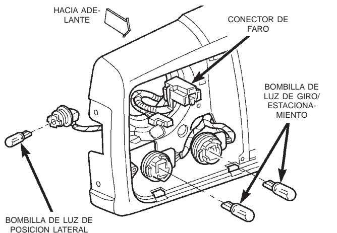
Fig. 1 Conector de faro
