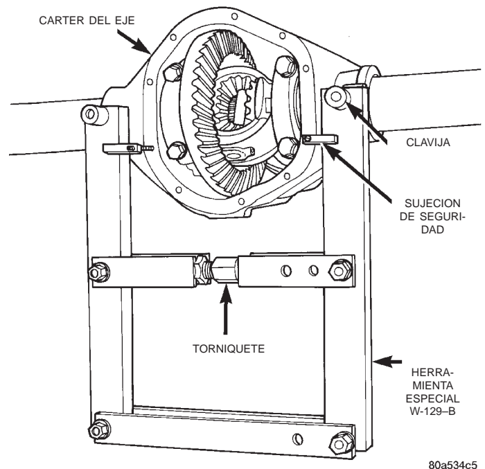
Fig. 21 Instalación de separador del cárter del eje
