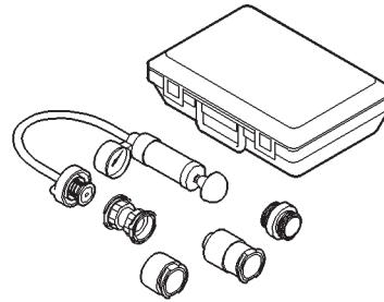
Aparato de prueba de presión del sistema de refrigeración—7700-A
