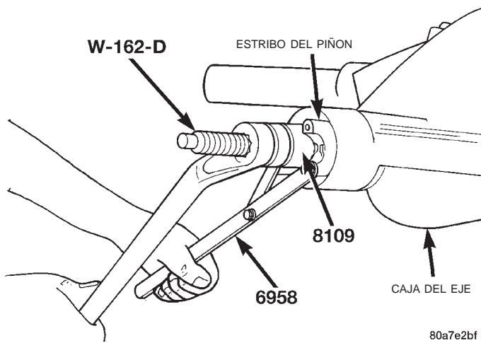
Fig. 38 Instalación del estribo del piñón
