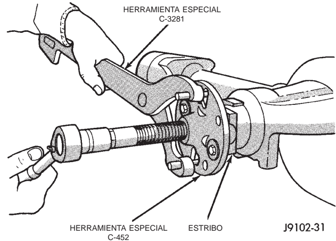
Fig. 28 Desmontaje del estribo del piñón
