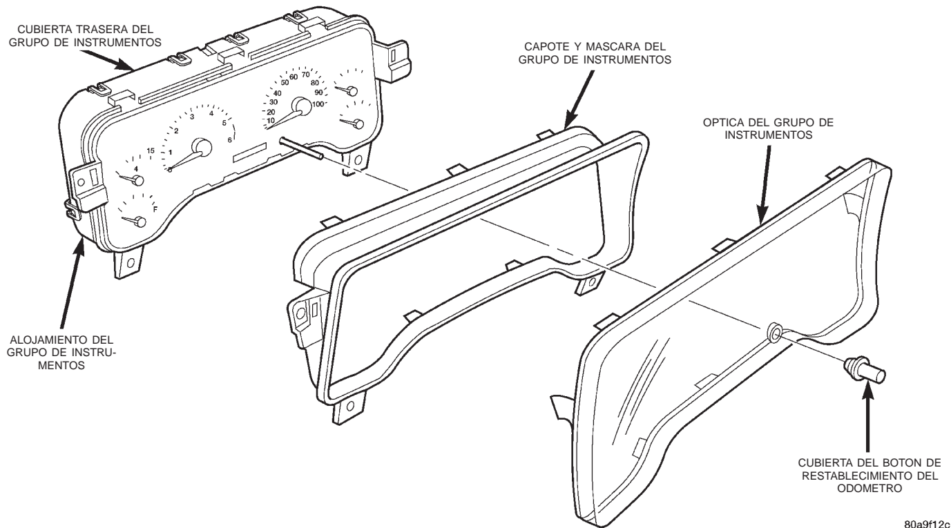
Fig. 14 Componentes del grupo de instrumentos
