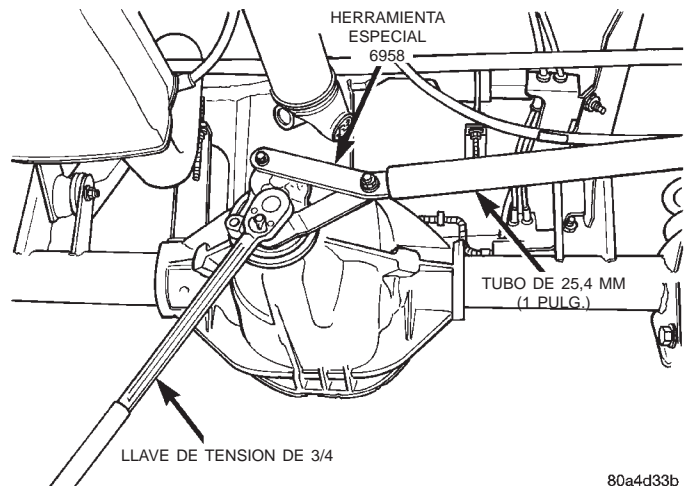
Fig. 17 Apriete de la tuerca del eje del piñón-Characterístico
