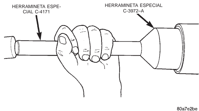
Fig. 42 Instalación de la junta del piñón necesario, consulte Profundidad del piñón satélite para seleccionar el espaciador del espesor correcto antes de instalar el cojinete trasero del piñón.
