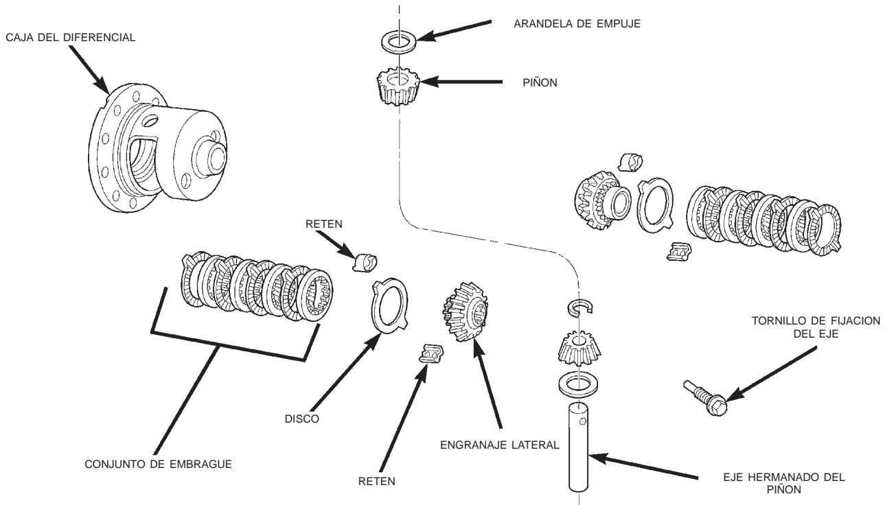
Fig. 38 Componentes del diferencial Trac-Lok
