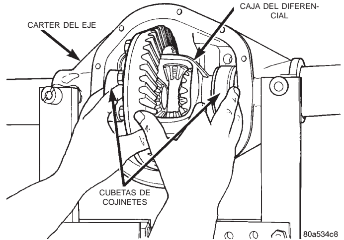
Fig. 20 Desmontaje de caja del diferencial
