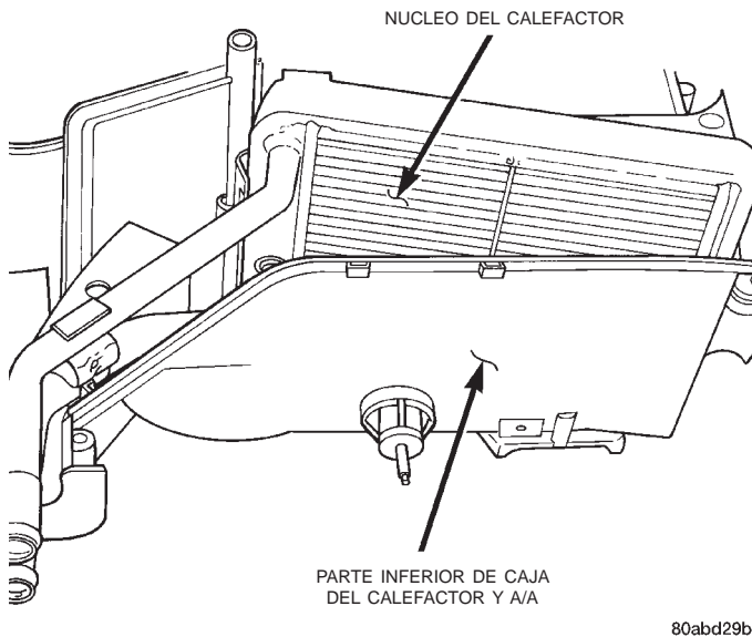
Fig. 48 Desmontaje e instalación del núcleo del calefactor
