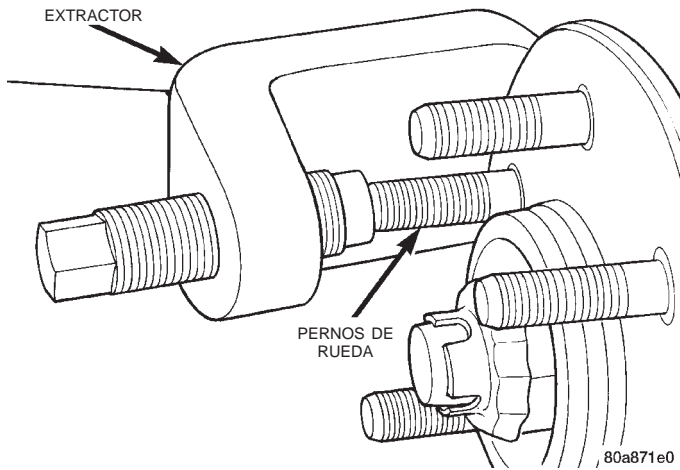
Fig. 9 Desmontaje de los pernos de la rueda
