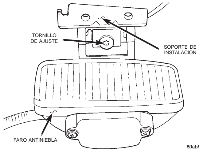
Fig. 5 Ajuste del faro antiniebla
