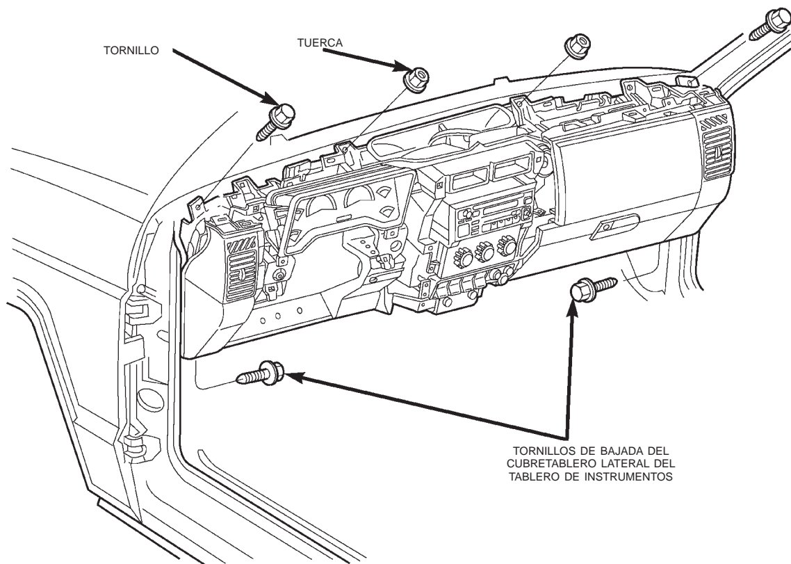
Fig. 23 Desmontaje e instalación del conjunto del tablero de instrumentos
