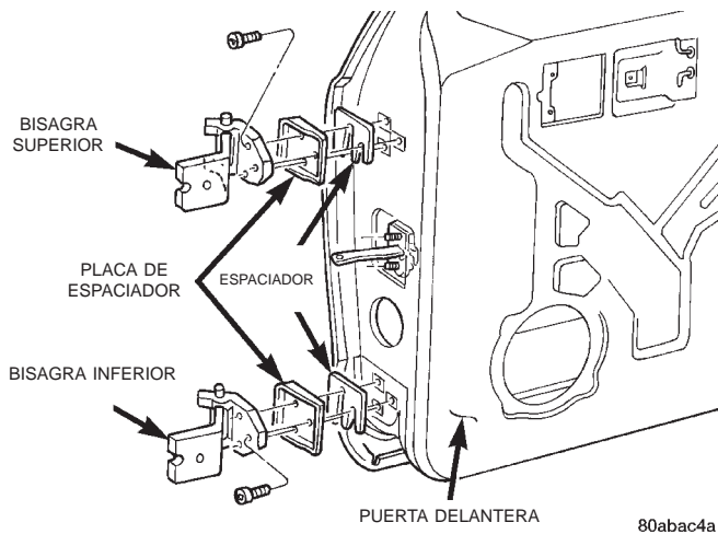
Fig. 26 Bisagra de puerta delantera
