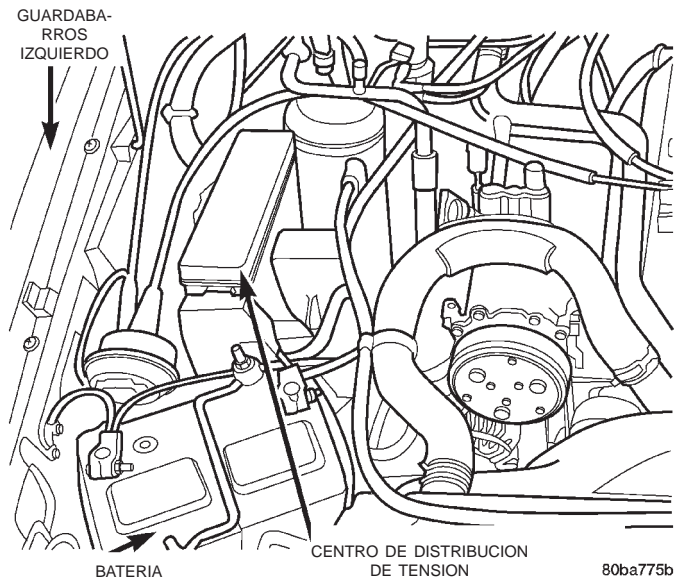
Fig. 1 Centro de distribución de tensión
