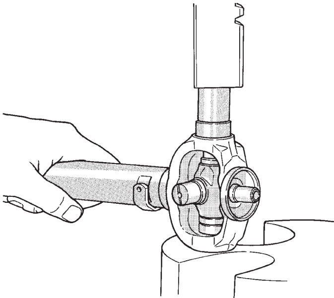
Fig. 29 Colocación de tapa de cojinete
