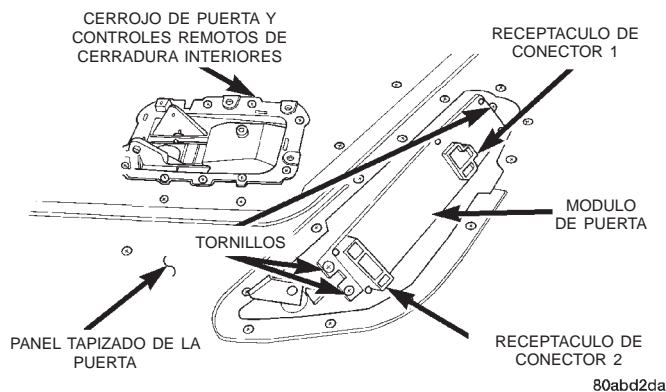
Fig. 4 Desmontaje/instalación de módulo de puerta
