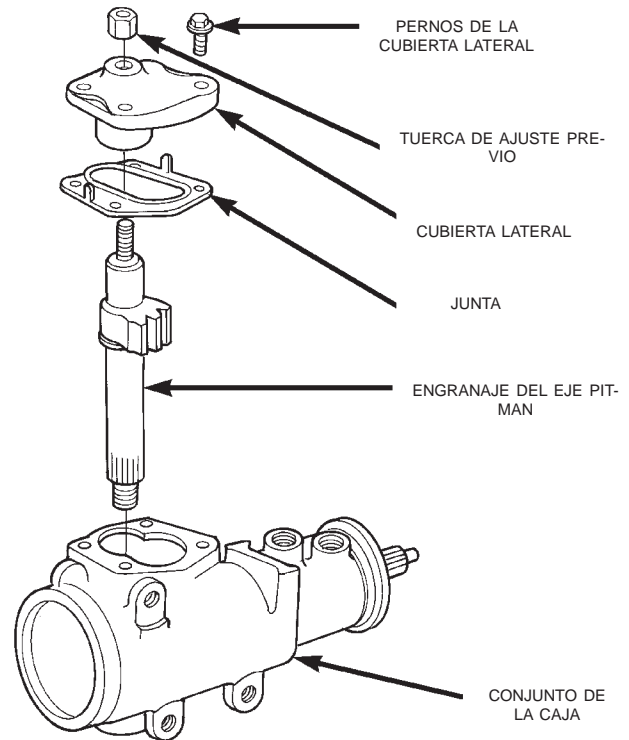
Fig. 6 Cubierta lateral y eje pitman
