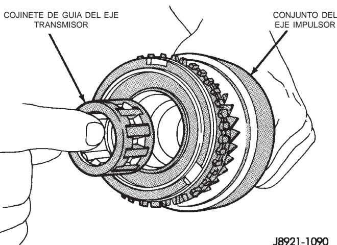
Fig. 107 Desmontaje de cojinete de guía del eje transmisor
