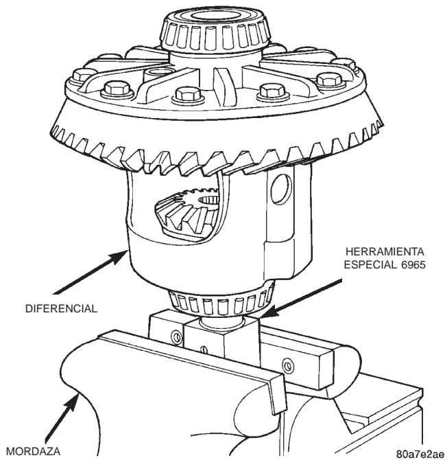
Fig. 52 Herramienta de sujeción de caja del diferencial
