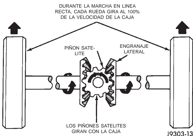
Fig. 3 Funcionamiento del diferencial—Marcha en línea recta
