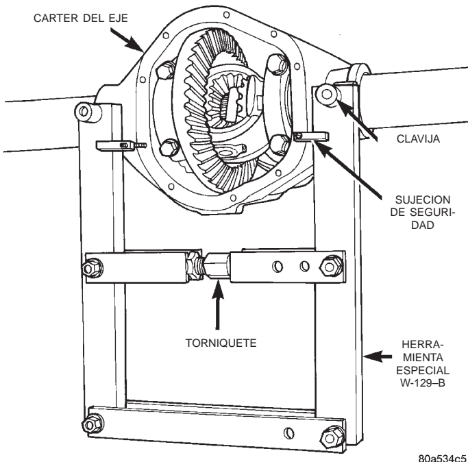
Fig. 24 Instalación del separador del cárter del diferencial
