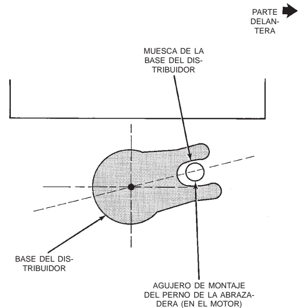
Fig. 32 Posición del distribuidor acoplado—Motor de 2.5L 4 cilindros
