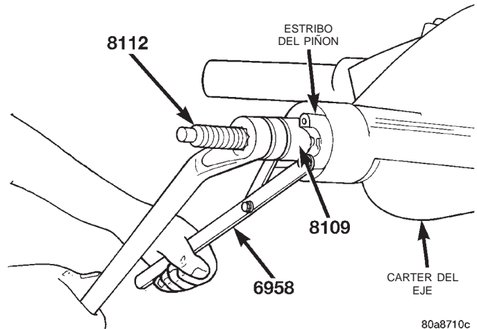
Fig. 16 Instalación del estribo del piñón
