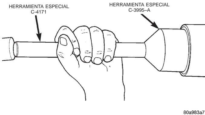
Fig. 10 Instalación de la junta retén trasera
