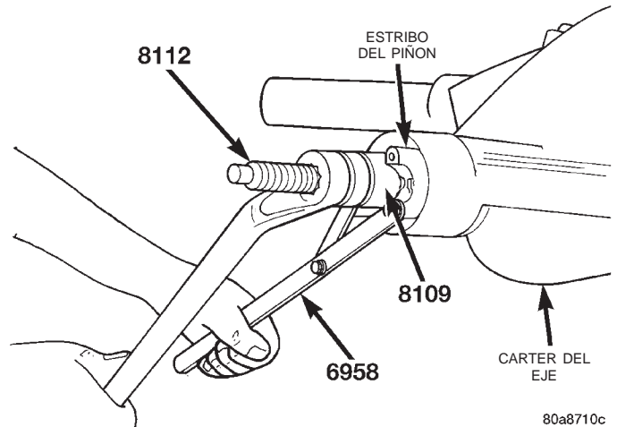
Fig. 45 Instalación del estribo del piñón
