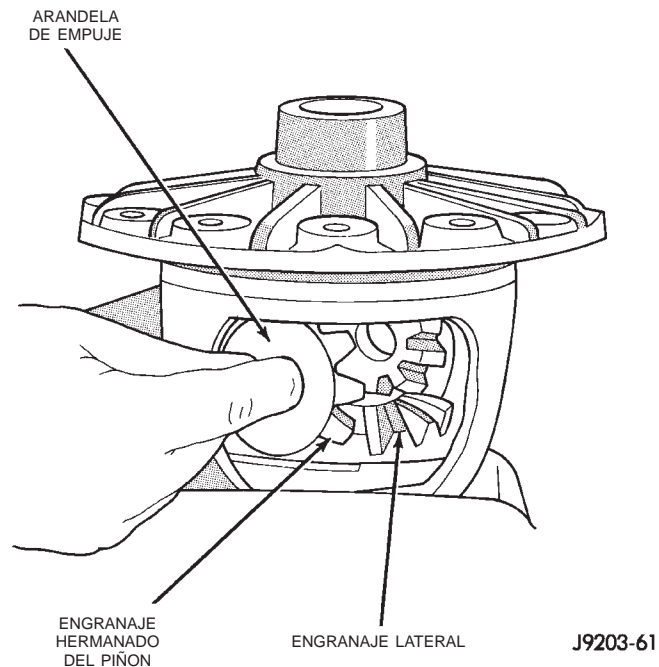
Fig. 37 Desmontaje de engranaje hermano del piñón
