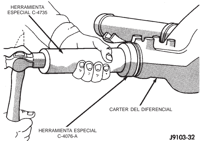
Fig. 14 Instalación de junta de piñón del eje 8 1/4
