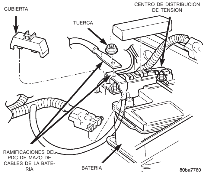
Fig. 3 Conexiones del centro de distribución de tensión
