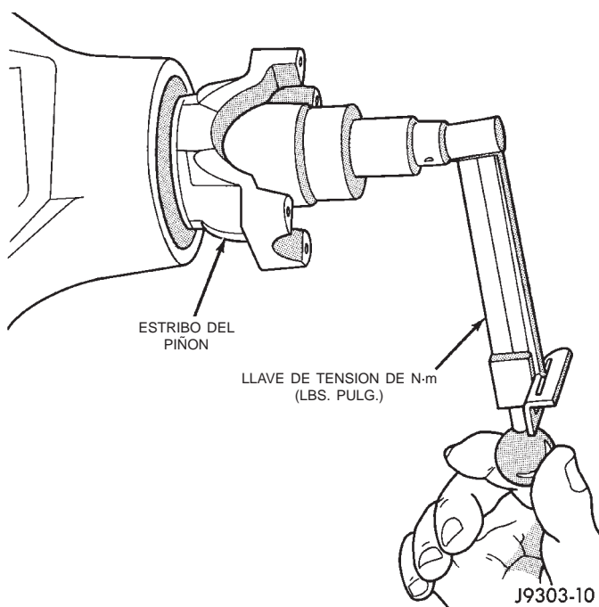
Fig. 47 Comprobación de torsión de rotación del piñón satélite
