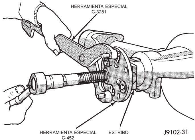
Fig. 7 Desmontaje del estribo del piñón
