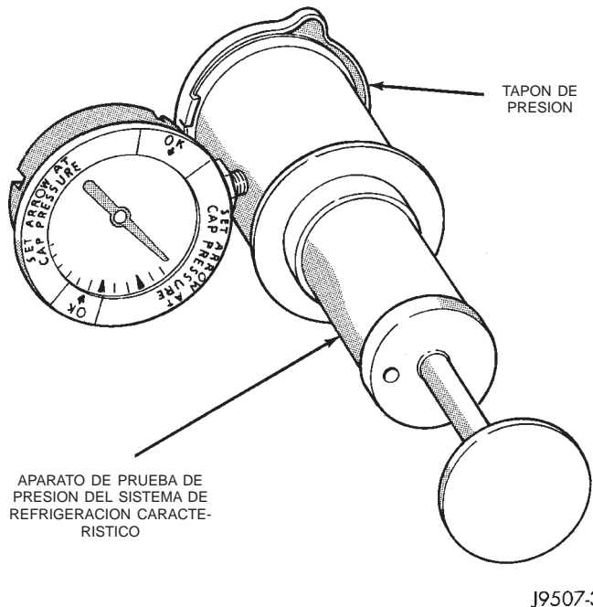
Fig. 11 Aparato de prueba de presión del sistema de refrigeración característico
