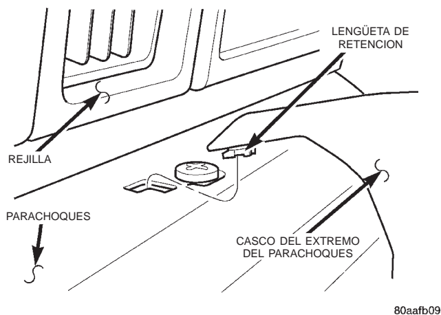
Fig. 2 Casco del extremo del parachoques GANCHO DE TRACCION DELANTERO
