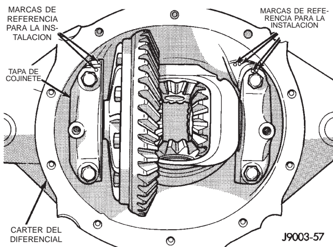
Fig. 19 Tapas y pernos de cojinetes
