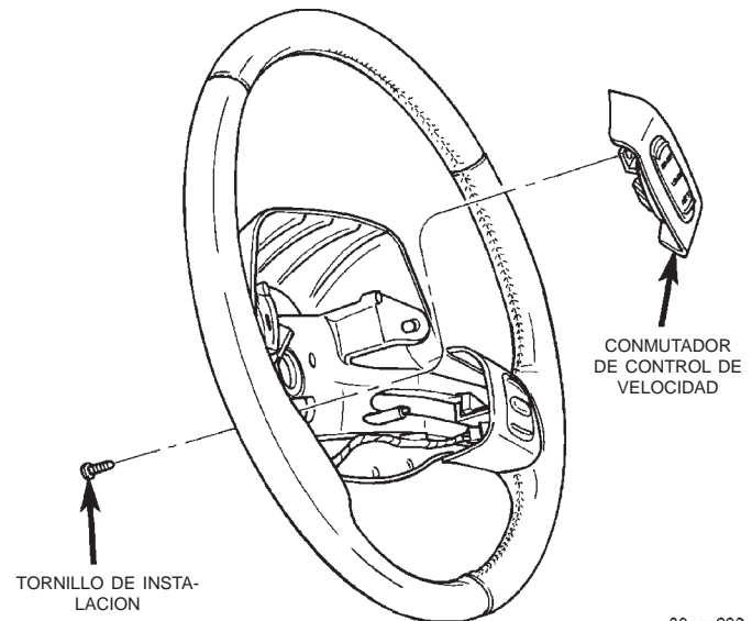
Fig. 3 Desmontaje e instalación del conmutador de control de velocidad
