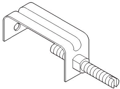
Retenedor de bola de detenedor y muelle—6583
