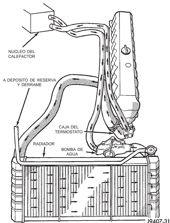
Fig. 1 Circulación de refrigerante—Motores 2.5L y 4.0L
