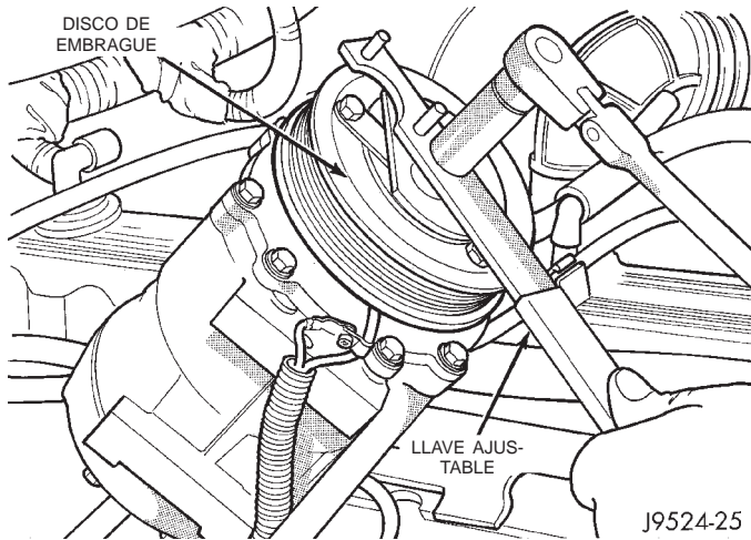
Fig. 23 Desmontaje de la tuerca de embrague
