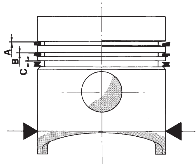
Fig. 57 Luz del aro de pistón a la acanaladura
