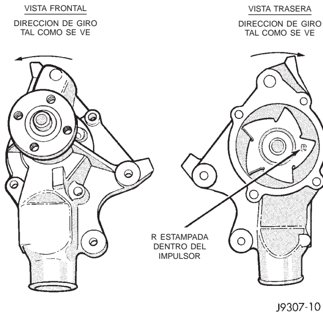
Fig. 19 Bomba de agua de giro a la inversa— Característica
