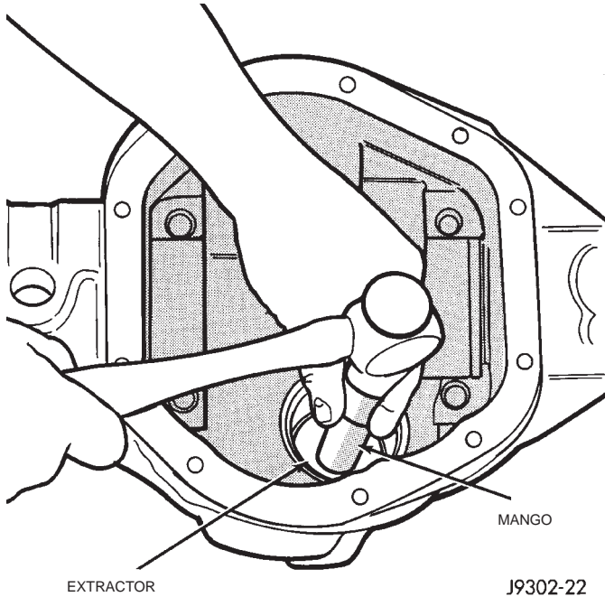
Fig. 36 Desmontaje de la cubeta del cojinete delantero
