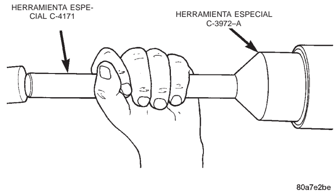
Fig. 35 Instalación de la junta del piñón
