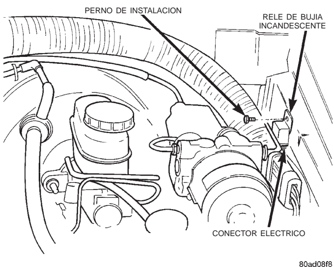
Fig. 24 Localización del relé de bujías incandescentes
