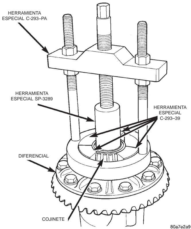
Fig. 30 Desmontaje de cojinete del diferencial
