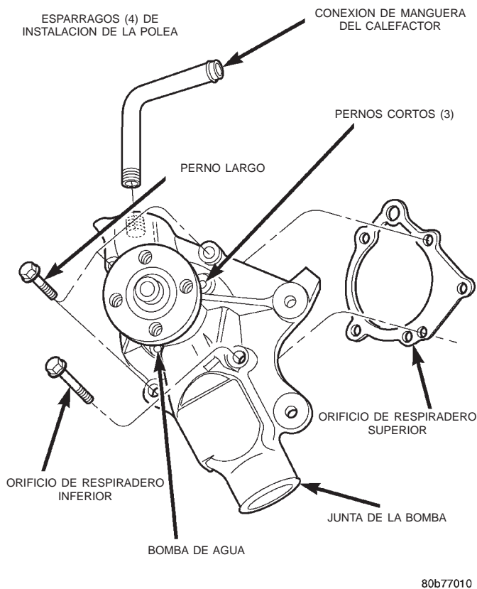
Fig. 25 Desmontaje e instalación de la bomba de agua—Característico
