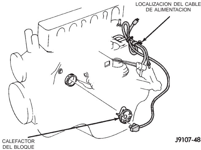
Fig. 39 Calefactor y cable— Motor de 2.5L y 4 cilindros
