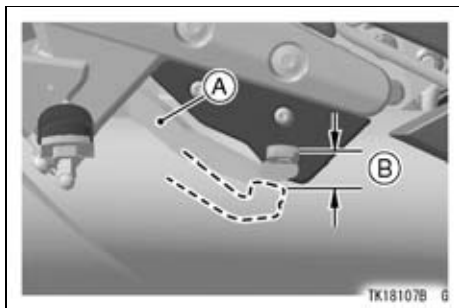
A. Pedal de freno B. Recorrido del pedal
