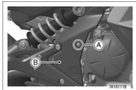
A. Perno B. Cubierta del lado derecho del chasis
