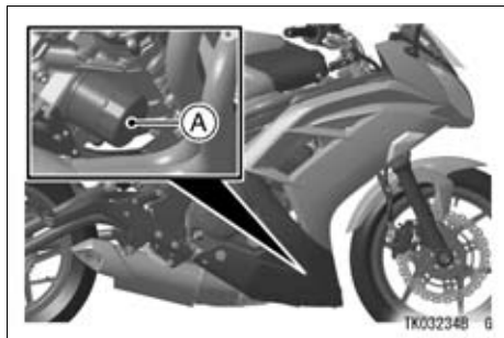
A. Cartucho del filtro de aceite
