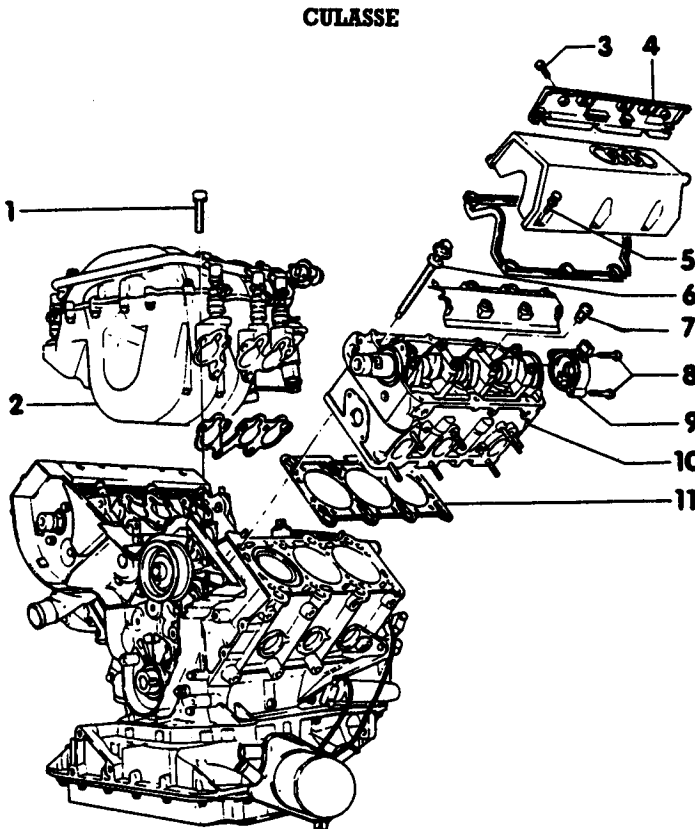
1 : Vis de fixation collecteur. - 2 : Tubulure d'admission. - 3 : Vis de protection. - 4 : Protecteur. - 5 : Vis de couvre-culasse. - 6 : Vis de culasse. - 7 : Soupape de limitation de pression. - 8 : Vis de transmetteur Hall. - 9 : Boîtier du transmetteur de Hall. - 10 : Culasse. - 11 : Joint de culasse.
