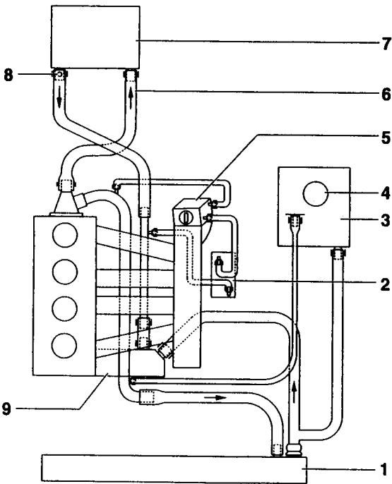
1 : Radiateur. - 2 : Radiateur d'huile. - 3 : Vase d'expansion. - 4 : Bouchon. - 5 : Ajutage papillon. - 6 : Conduite d'arrivée radiateur de chauffage. - 7 : Radiateur de chauffage. - 8 : Orifice de purge. - 9 : Pompe à eau.
