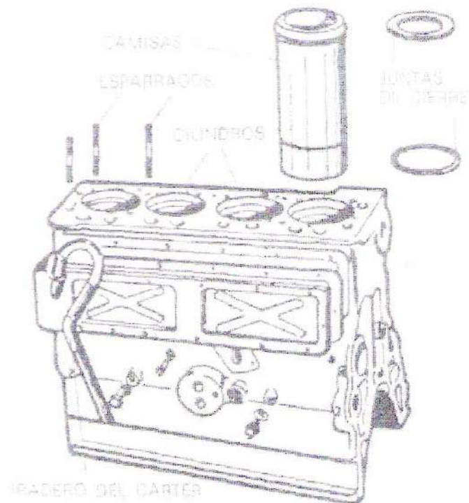
Fig. 3. Bloque y algunas de las piezas que contiene.
