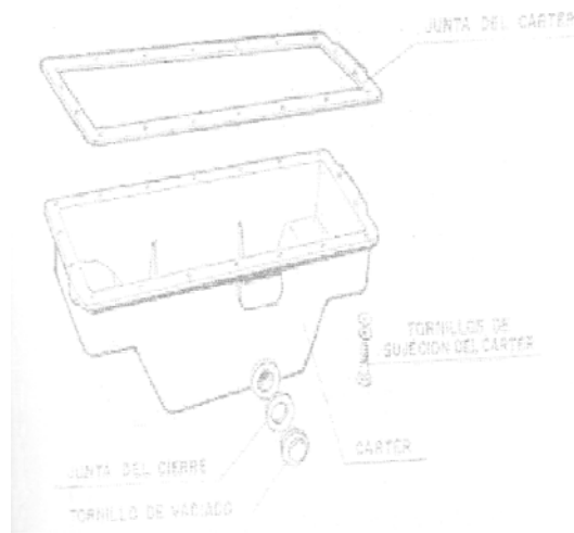
Fig. 15. Cárter. Arriba, la junta del cárter
