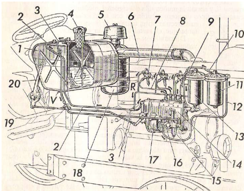
Fig. 192. Instalación completa del equipo de inyección y sus accesorios.
