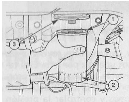
1.- sello de goma. 2.-cartucho. 3.-cabezal.
