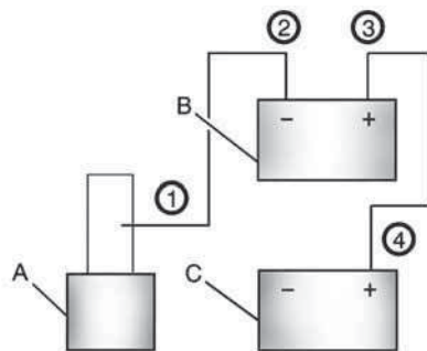
Desconexión de los cables de arranque
