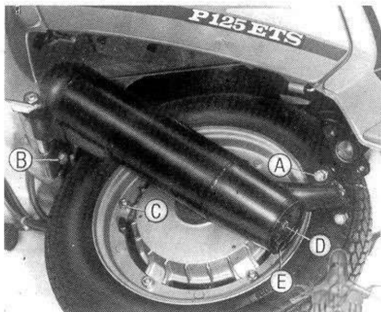
Fig. 2 - Smontaggio ruota posteriore del motorhelp.com
