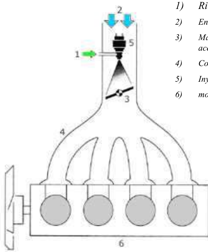
Monopunto
