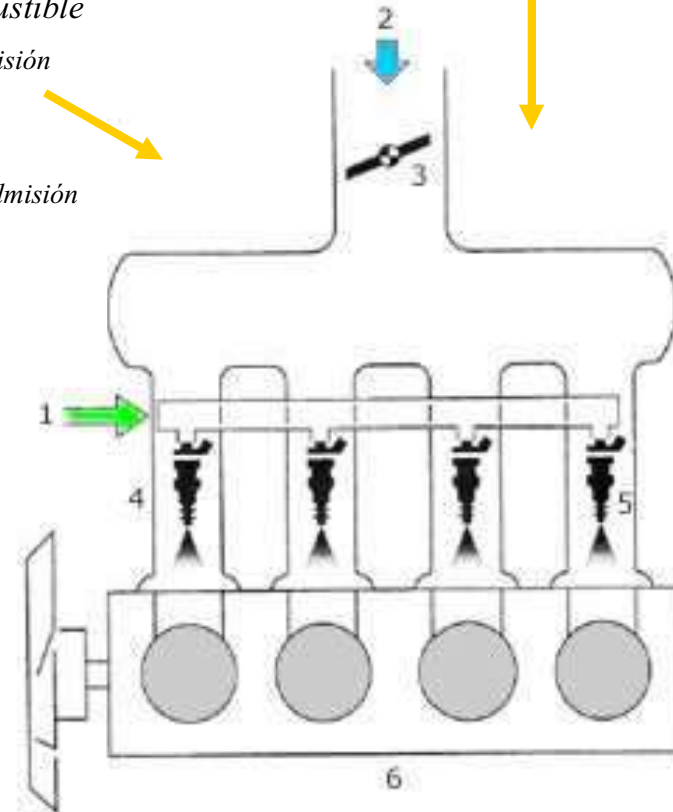
Multipunto
