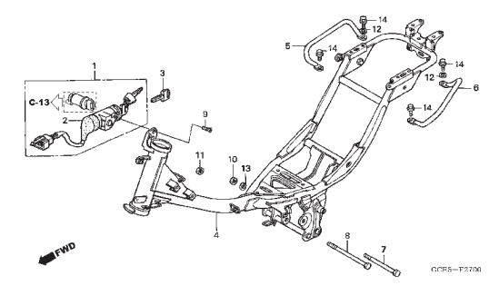
C-27 Bastidor
