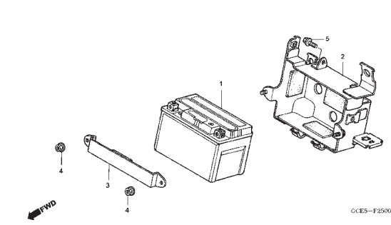
C-25 Bateria
