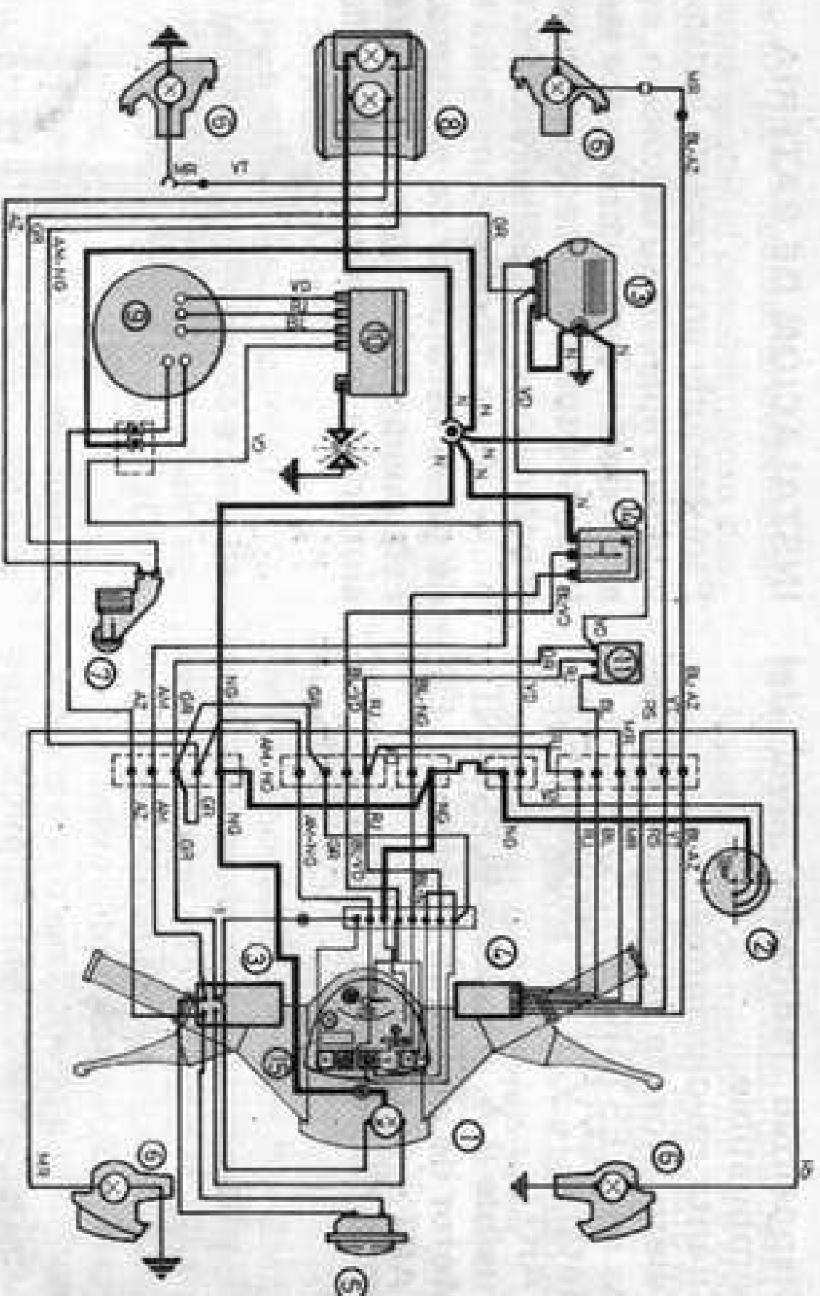
Fig. 17 Esquema eléctrico Vespa TX 200
