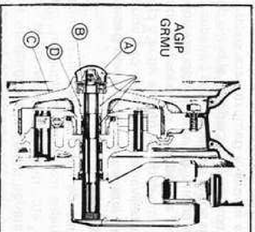
Fig. 38 Engrase tambor freno delantero.
