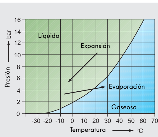
Curva de presión de vapor R134a
