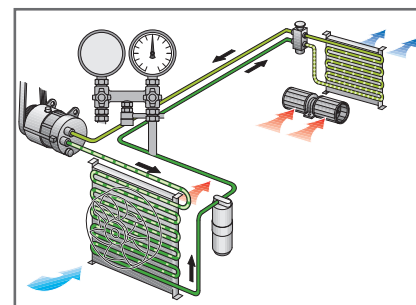
Empalme para Servicio, alta presión
