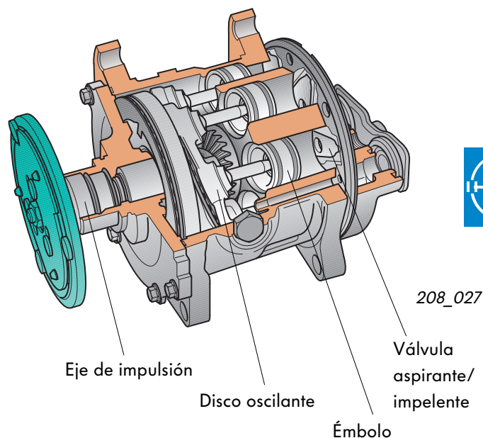
Compresor de disco oscilante, no autorregulado Ángulo constante del disco oscilante Cilindrada constante
