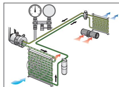
Empalme para Servicio, baja presión
